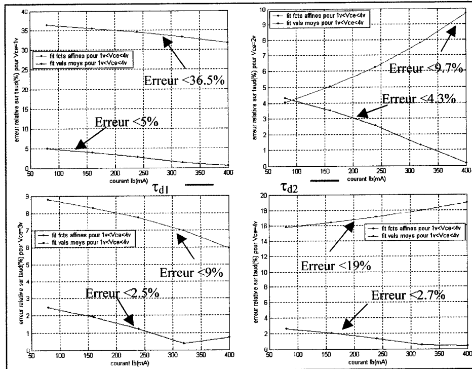
Figure 4-61: Erreurs de \tau_{d1} et de \tau_{d2} par rapport à \tau_{d\_ed} pour 1\text{V} < V_{ce} < 4\text{V}
