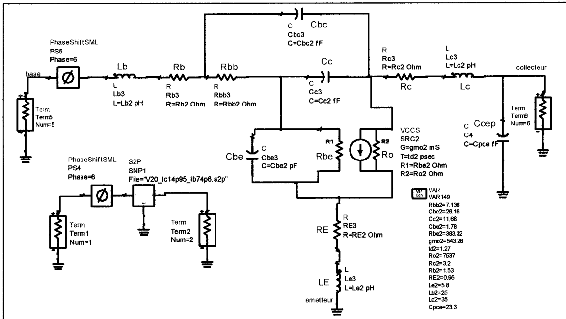
Figure 4-28: Simulation des paramètres-S pour le point V_{ce}=2\text{v} et I_b=74.6\mu\text{A}
