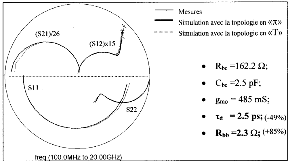
Figure 4-13: Optimisation des paramètres \tau_d et R_{bb} de la topologie en «π»
