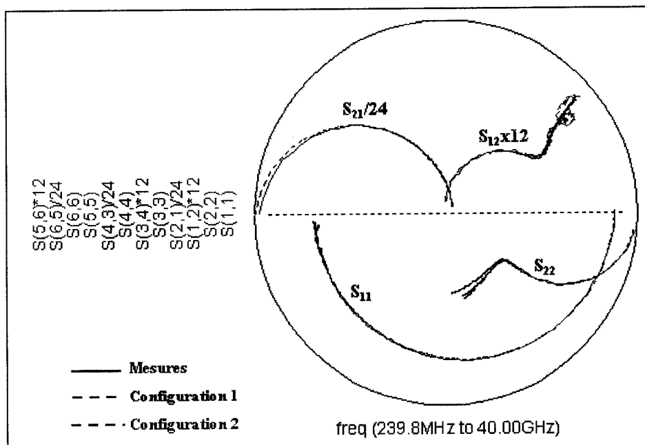
Figure 3-25: Simulation des paramètres-S pour le V_{cc}=4\text{v} et I_b=50.6\mu\text{A}
