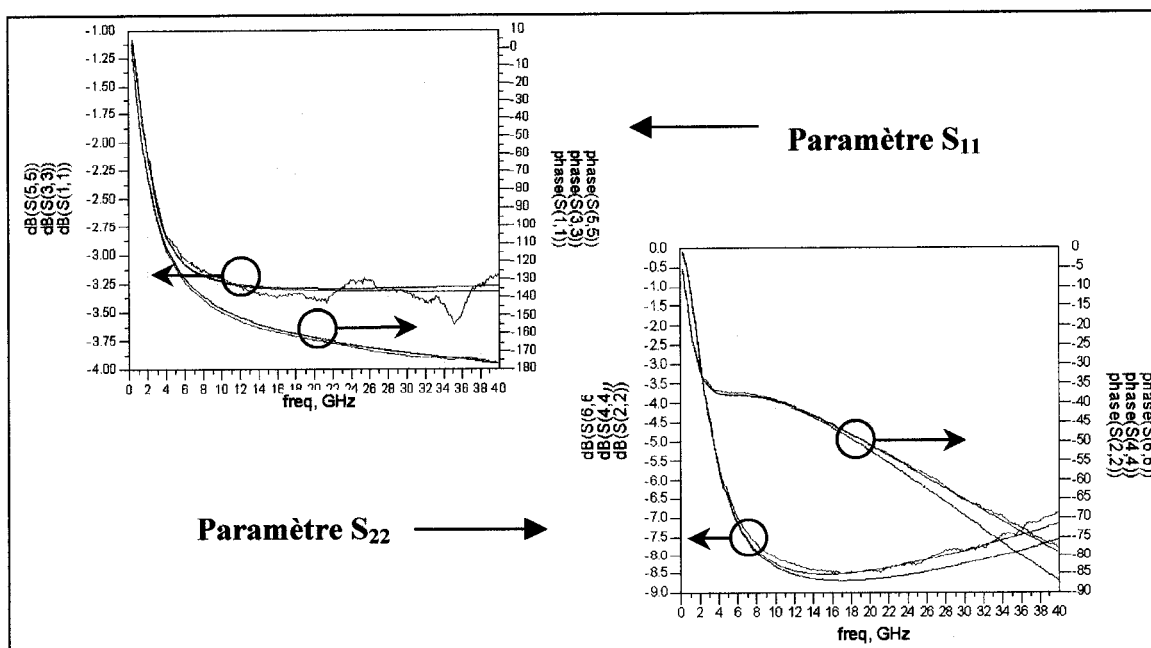
Figure 3-26: Module et phase des paramètres S_{11} et S_{22} à V_{cc}=4\text{v} , I_b=50.6\mu\text{A}
