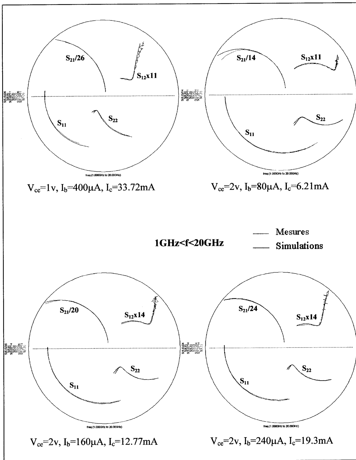
Figure 5-2: Simulations paramètres-S pour ( V_{ce}=1V , I_b=400\mu A ) et ( V_{ce}=2V et 80\mu A < I_b < 240\mu A )
