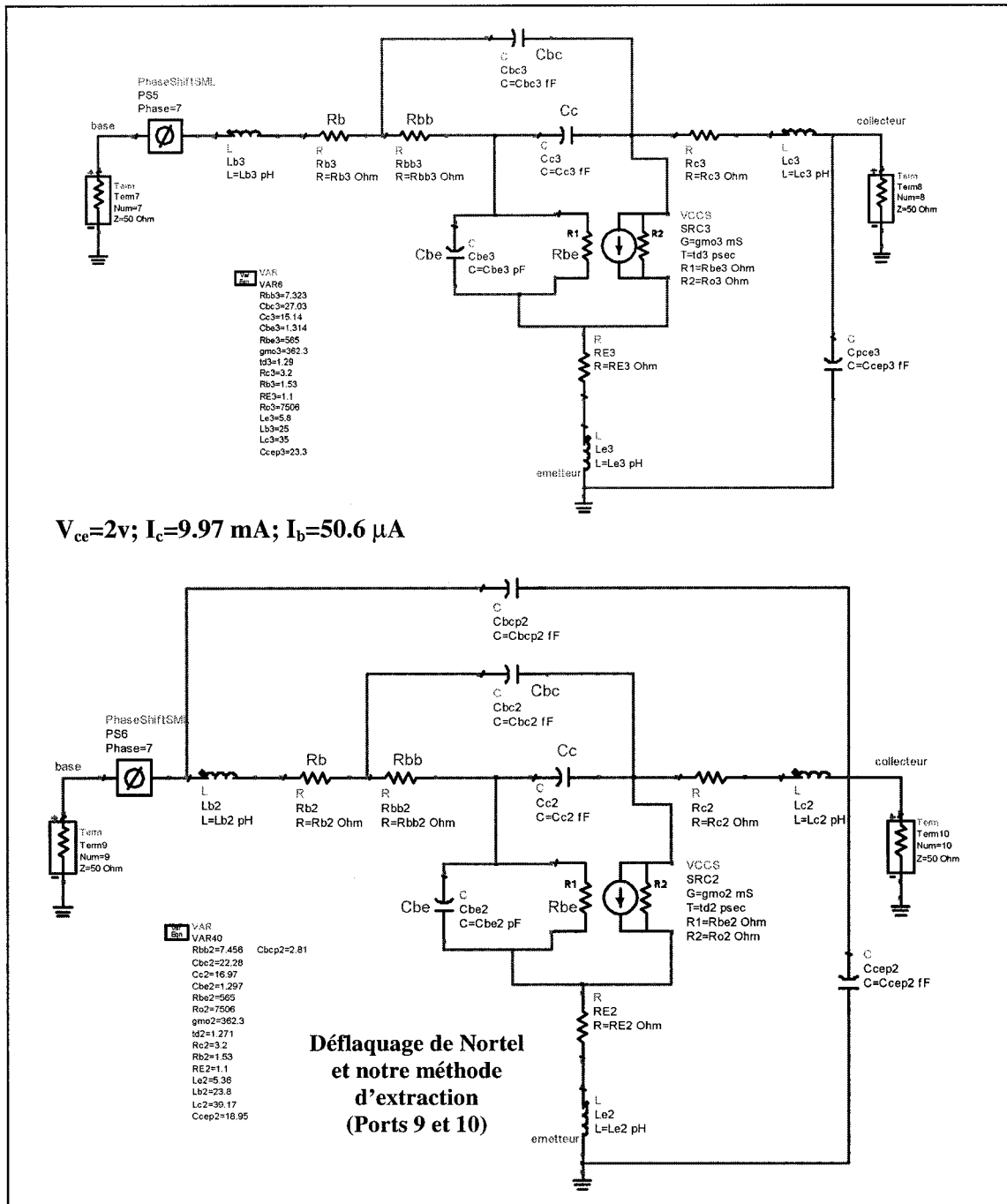
Figure 3-15: Simulation en paramètres-S pour les 2 méthodes de déflaage
