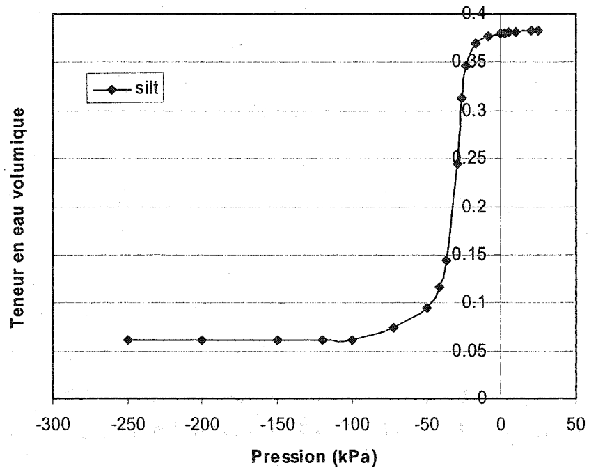
Figure 4.11 : Courbe de rétention d'eau : teneur en eau volumique vs. succion pour les silts (matériaux 2 a à 2 d)
