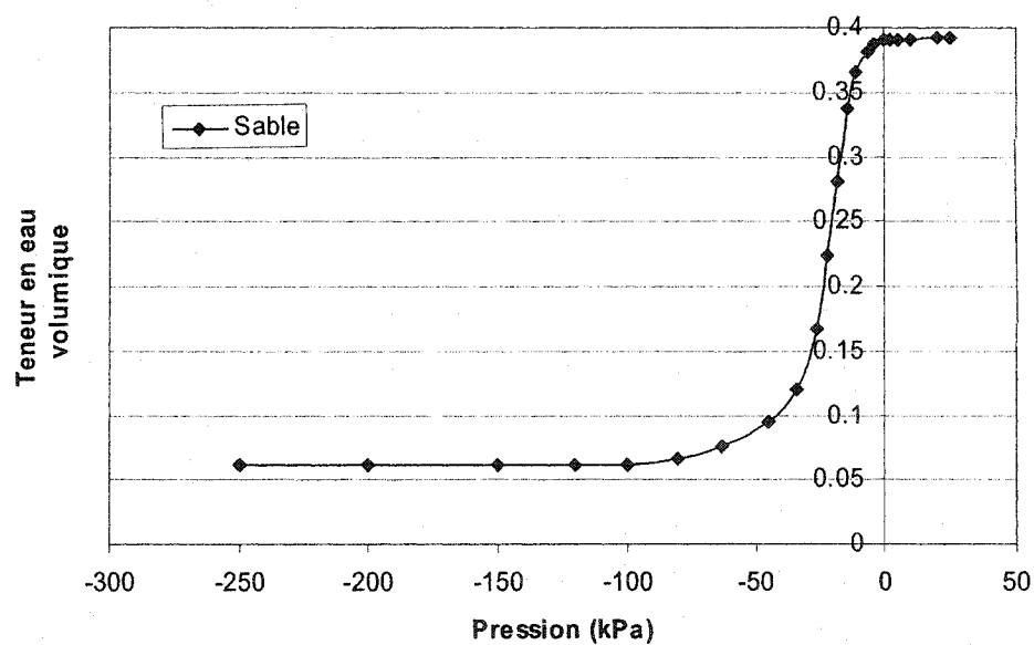
Figure 4.13 : Courbe de rétention d'eau : teneur en eau volumique vs. succion du sable
