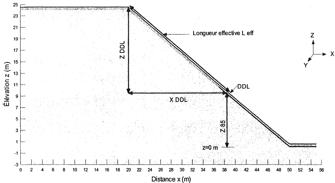
Figure 4.60 : CEBC incluant les indications sur la longueur effective et le point DDL.
