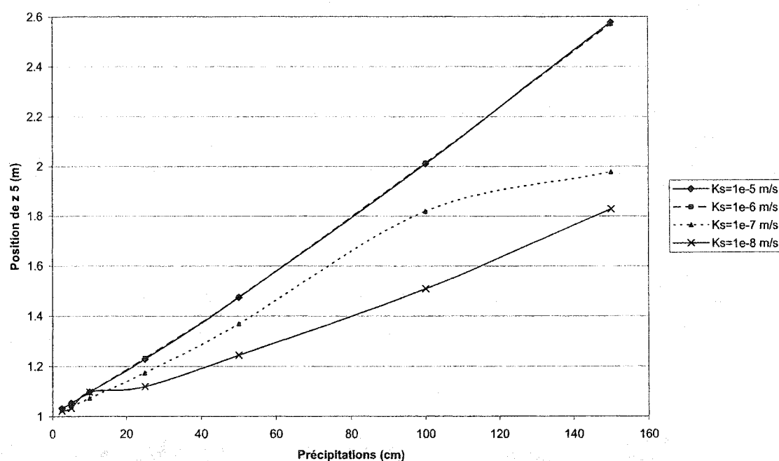
Figure 4.26 : Évolution de la position de z_5 par rapport à la quantité totale de précipitations après cinq jours à 12,5 cm au-dessus de l'interface silt-sable, pour diverses valeurs de k_s pour le silt de la couverture.
