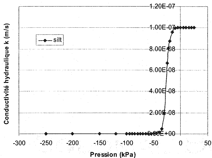
Figure 4.9 : Fonction de perméabilité : conductivité hydraulique vs. succion du matériau 2 c avec k_s = 1 \cdot 10^{-7} m/s
