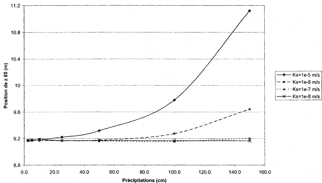
Figure 4.25 : Évolution de la position de z_{85} par rapport à la quantité totale de précipitations après cinq jours à 1 m au-dessous de l'interface silt-sable.
