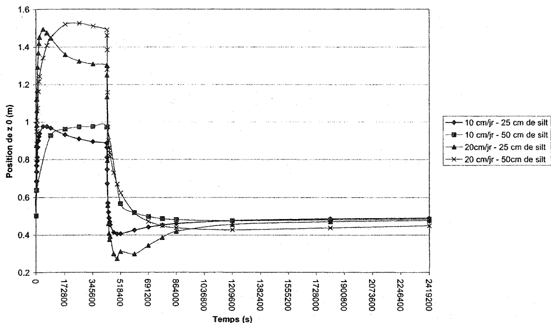
Figure 4.33 : Comparaisons entre les valeurs de z_0 en fonction du temps avec une épaisseur de couverture et des précipitations variables
