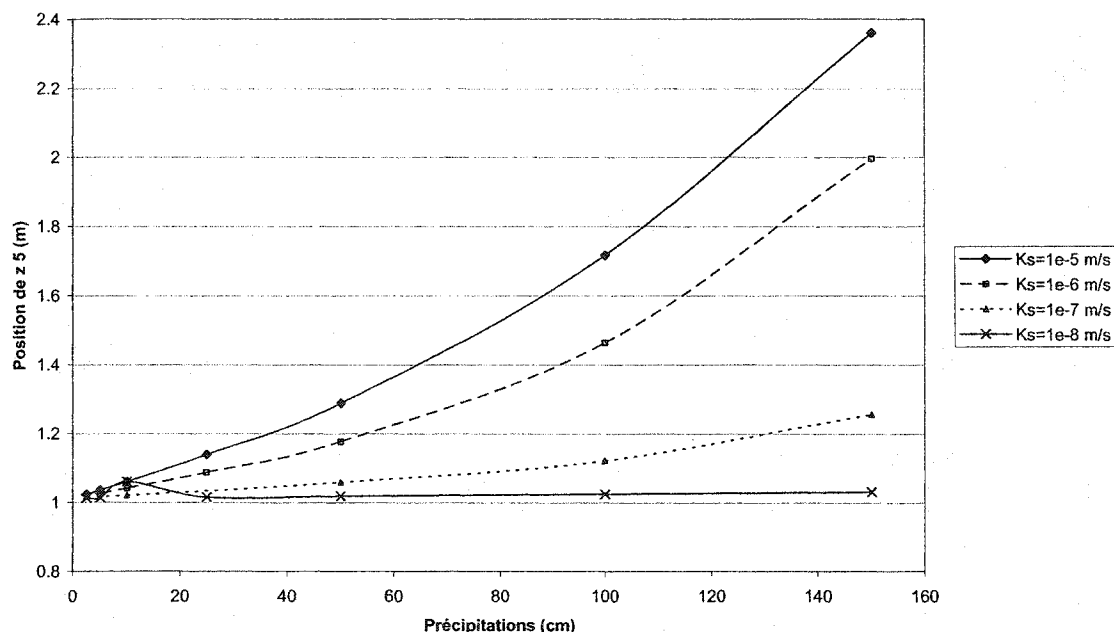
Figure 4.27 : Évolution de la position de z_5 par rapport à la quantité totale de précipitations après cinq jours à 1 m au-dessous de l'interface silt-sable pour diverses valeurs de k_s pour le silt de la couverture.
