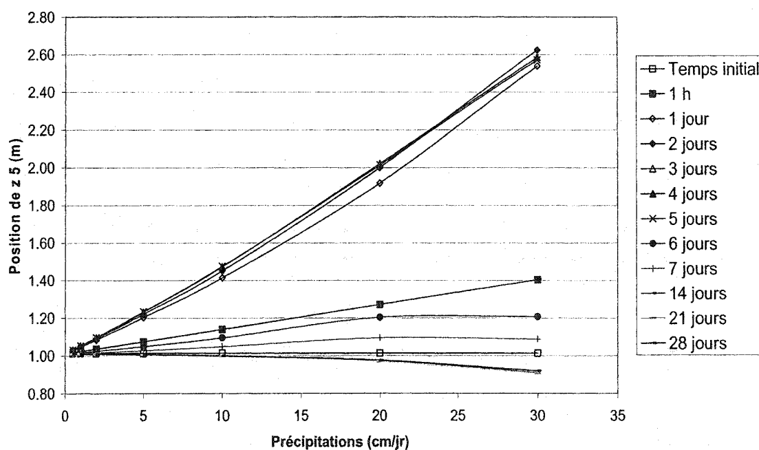
Figure 4.20 : Évolution de la position de z_5 en fonction des intensités de précipitations - k_s du silt = 1 \cdot 10^{-6} m/s.
