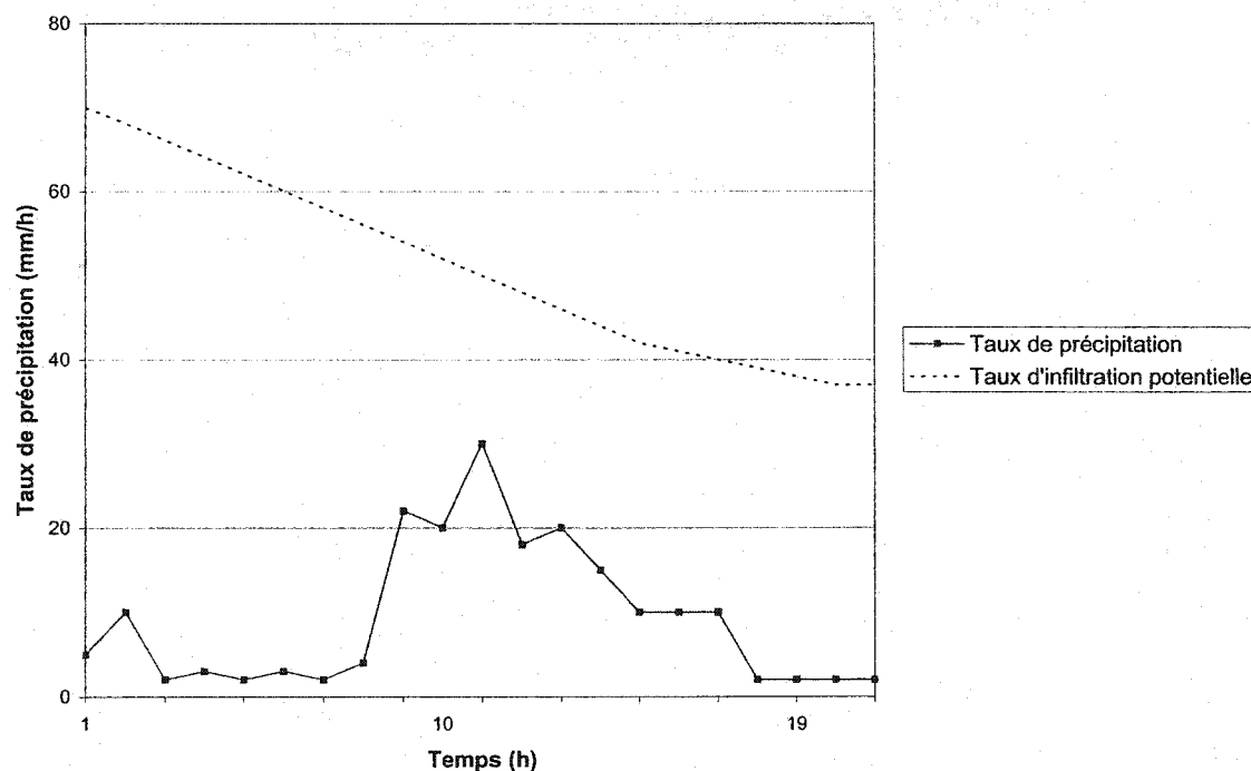
Figure 3.3 : Taux de précipitation et infiltration potentielle par rapport au temps – exemple 2 (adaptée d'après Blight, 1997).
