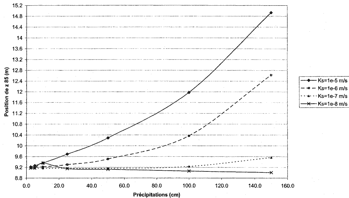
Figure 4.24 : Évolution de la position de z_{85} par rapport à la quantité totale de précipitations après cinq jours à 12,5 cm au-dessus de l'interface silt-sable.
