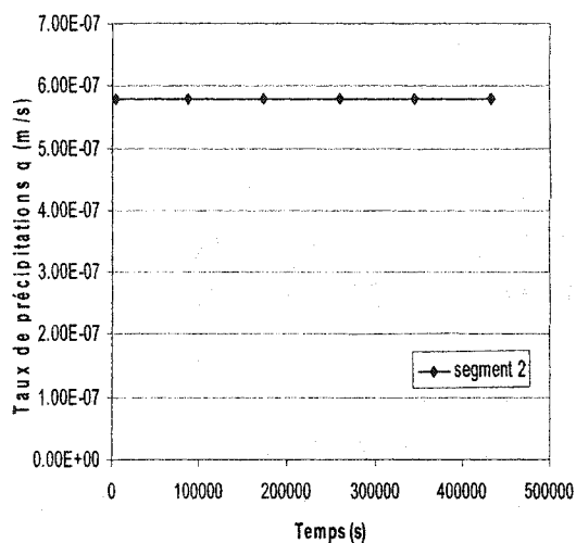
Figure 4.15b : 5 cm/jr pendant 5 jours : « plateau »
