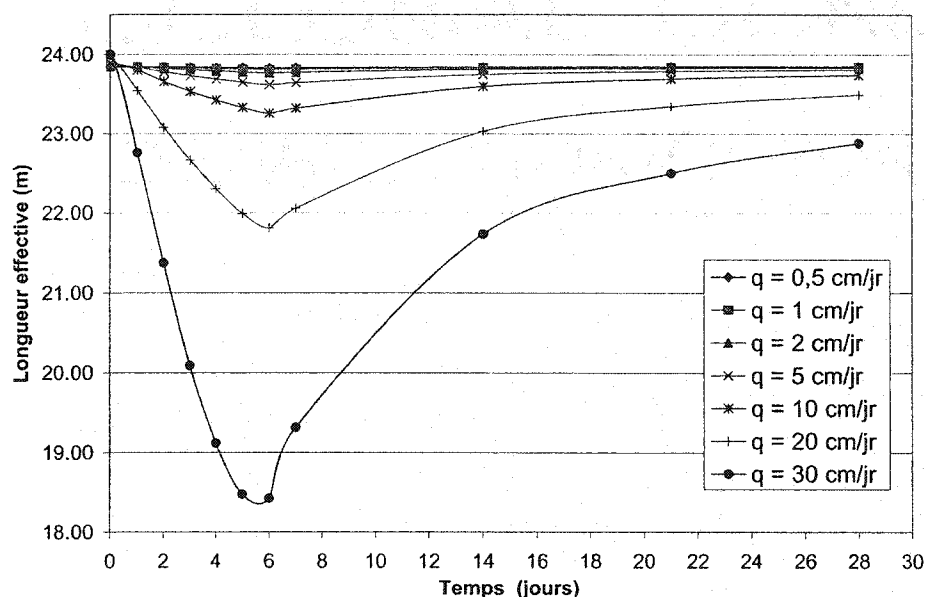
Figure 4.61 : Évolution de la longueur effective par rapport au taux de précipitation, lorsqu'il y a cinq jours de précipitations suivies d'un drainage libre jusqu'au 28ème jour.
