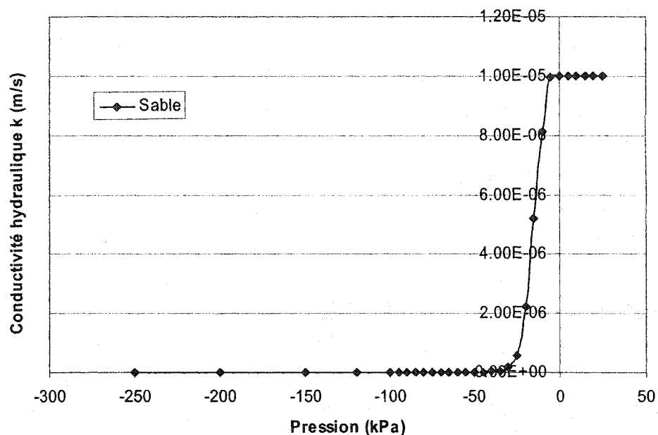
Figure 4.12 : Fonction de perméabilité : conductivité hydraulique vs. succion du sable
