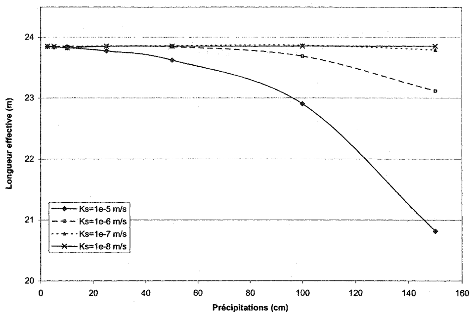
Figure 4.64 : Évolution de la longueur effective pour diverses valeurs de k_s du silt, selon le taux de précipitation (cinq jours de précipitations suivies d'un drainage libre jusqu'au 28ème jour) ; basée sur \psi_{85} en-dessous de l'interface silt-sable.
