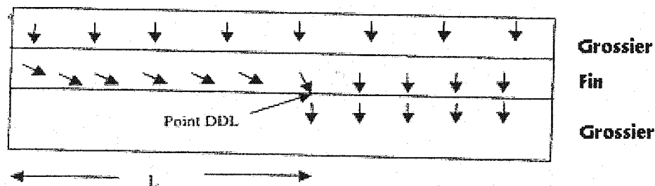
Figure 4.59 : Représentation schématique de l'écoulement de l'eau dans une couverture avec effets de barrière capillaire inclinée formée de sols fins et grossiers (adaptée de Bussière 1999).
