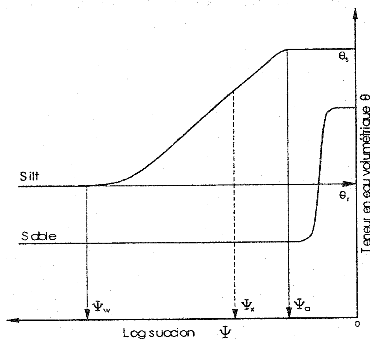
Figure 3.5 : Courbes de rétention d'eau schématisées pour un sable et un silt (adaptée d'après Aubertin et al., 1995)
