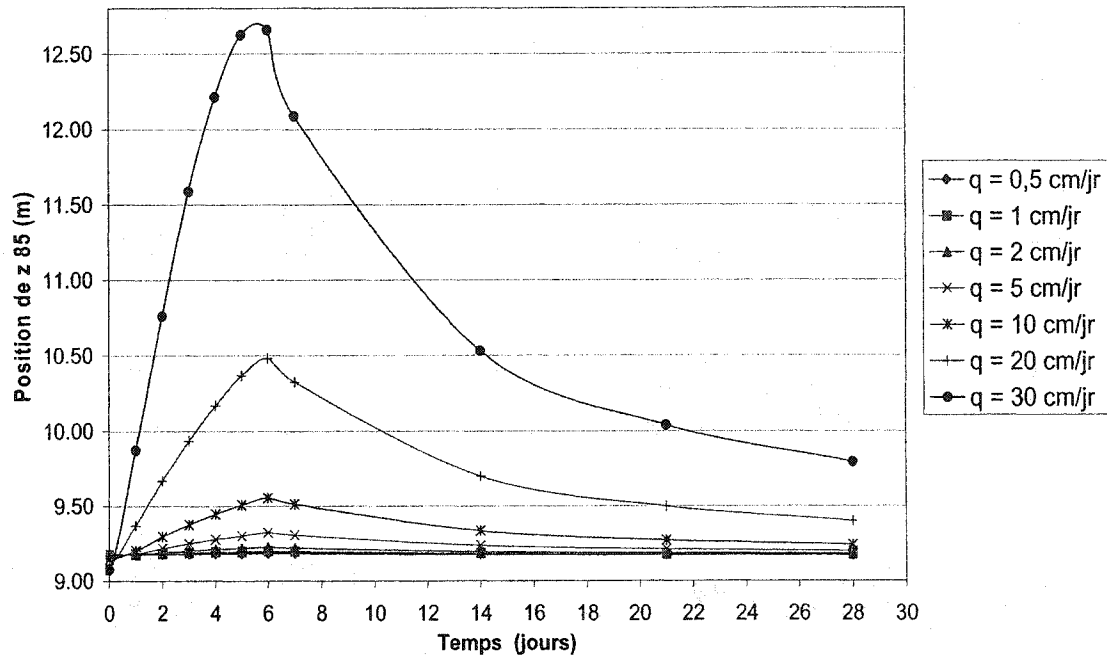
Figure 4.19 : Évolution de la position z_{85} en fonction des intensités et de la durée des précipitations (avec k_s du silt = 1 \cdot 10^{-6} m/s).
