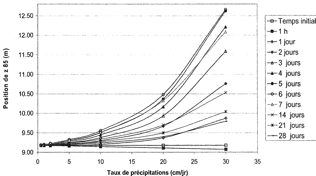
Figure 4.18 : Évolution de la position de z_{85} en fonction des intensités de précipitations (avec k_s du silt = 1 \cdot 10^{-6} m/s).
