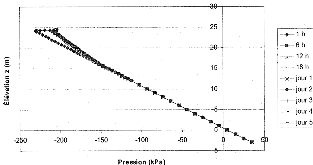
Figure 4.40 : Variation de la pression en fonction de l'élévation pour une section prolongée de x_1 pendant 5 jours de précipitations et une intensité de 10 cm/jr.
