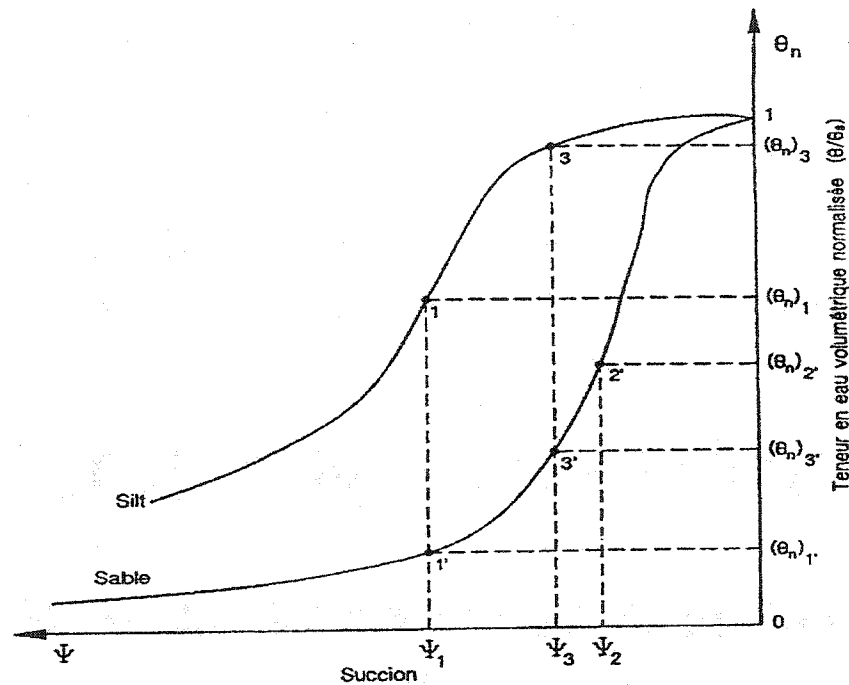
Figure 3.8 : Courbes de rétention d'eau pour un sable et un silt, présentées dans un plan \psi - \theta_n (tirée de Aubertin et al. 1995)
