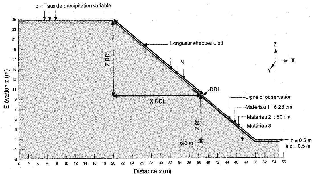
Figure 4.1 : Schéma du modèle de référence montrant la géométrie, les matériaux et certaines conditions aux frontières ( q , h ), la position du DDL, x_{DDL} , L_{eff} , z_{85} et les lignes d'observation.
