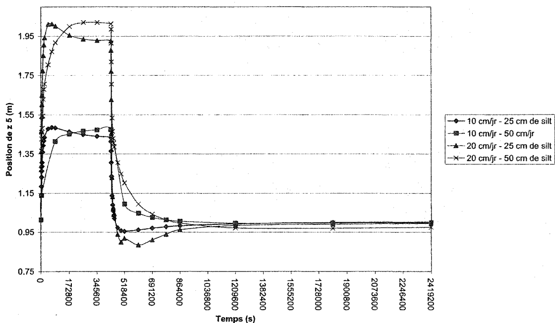
Figure 4.32 : Comparaisons entre les valeurs de z_5 en fonction du temps avec une épaisseur de couverture et des précipitations variables.
