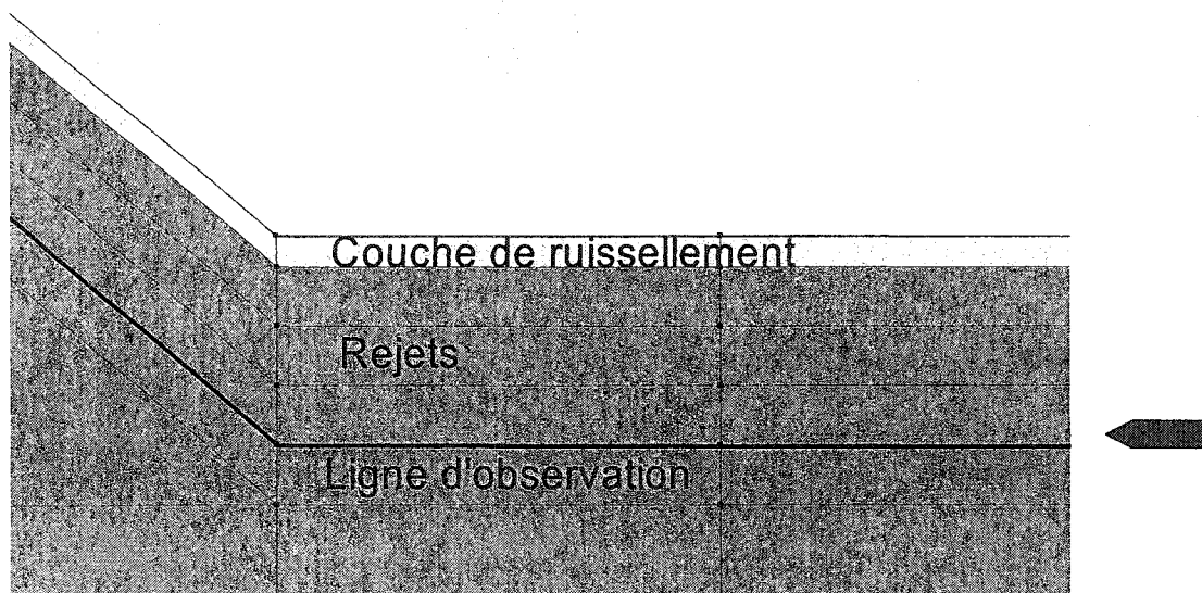
Figure 4.34 : Géométrie d'une partie du modèle pour le cas sans couverture, avec la ligne d'observation utilisée pour observer l'évolution du milieu.
