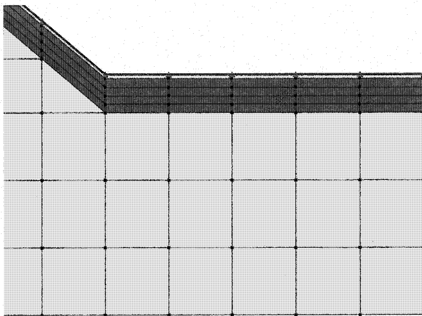
Figure 4.4 : Maillage au bas de la pente et drain de pied (point rouge) au niveau de l'interface entre le matériau drainant et le silt à x = 55 m, z = 0,5 m et h = 0,5 m.
