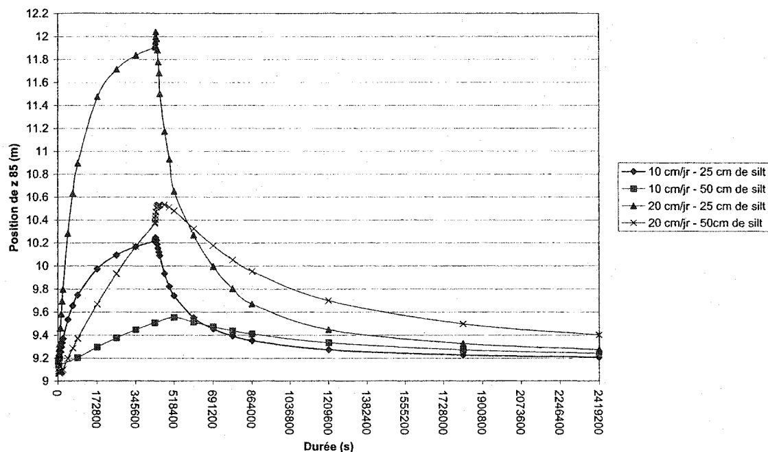
Figure 4.31 : Comparaisons entre les valeurs de z_{85} en fonction du temps avec une épaisseur de couverture et des précipitations variables.
