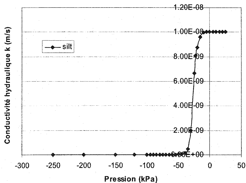
Figure 4.10 : Fonction de perméabilité : conductivité hydraulique vs. succion du matériau 2 d avec k_s = 1 \cdot 10^{-8} m/s
