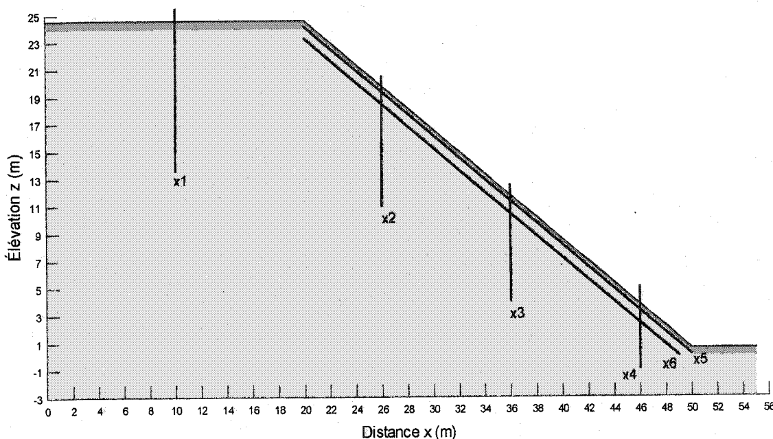
Figure 4.36 : Sections x_1 , x_2 , x_3 , x_4 , x_5 et x_6 effectuées dans la CEBC.
