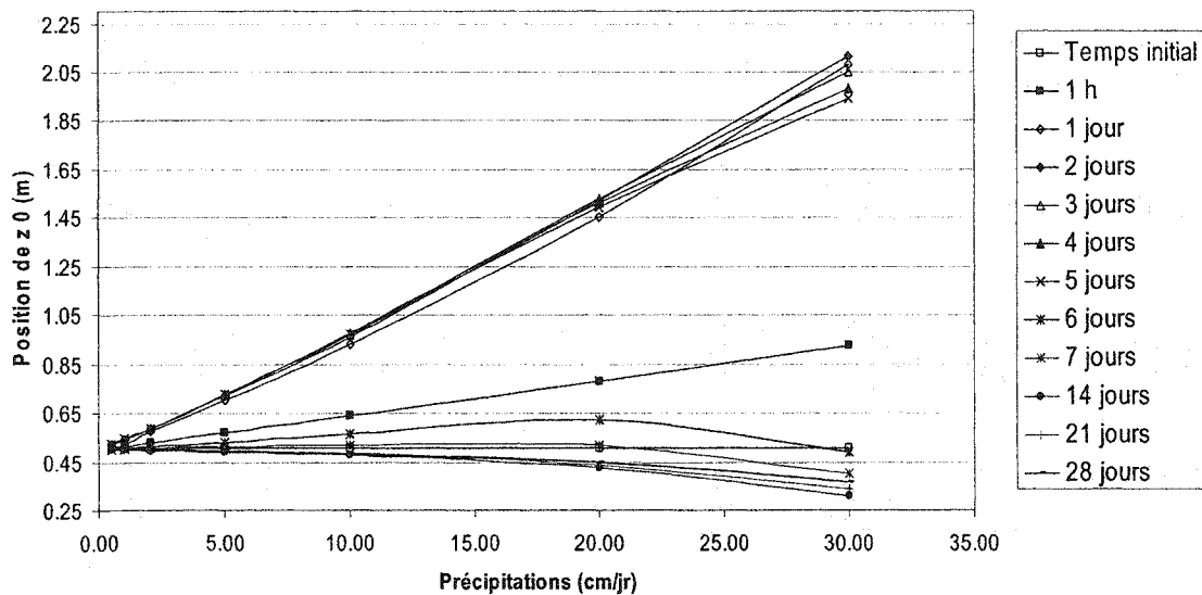
Figure 4.22 : Évolution de z_0 en fonction des intensités de précipitations ( k_s du silt = 1 \cdot 10^{-6} m/s).
