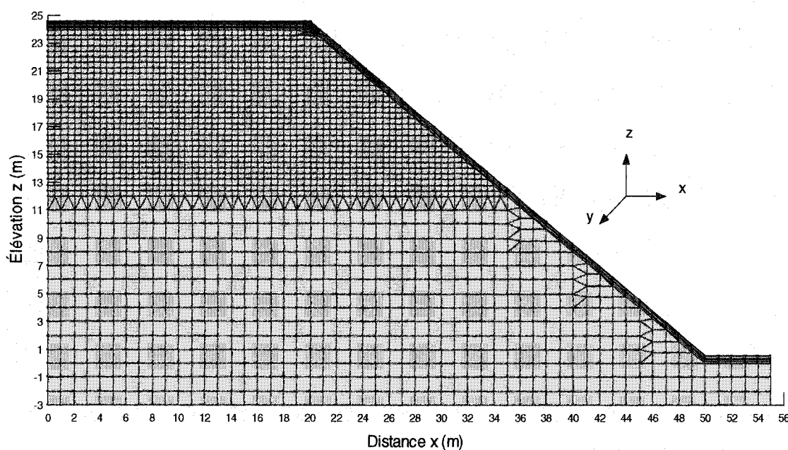
Figure 4.2 : Schéma du modèle de référence avec le maillage.
