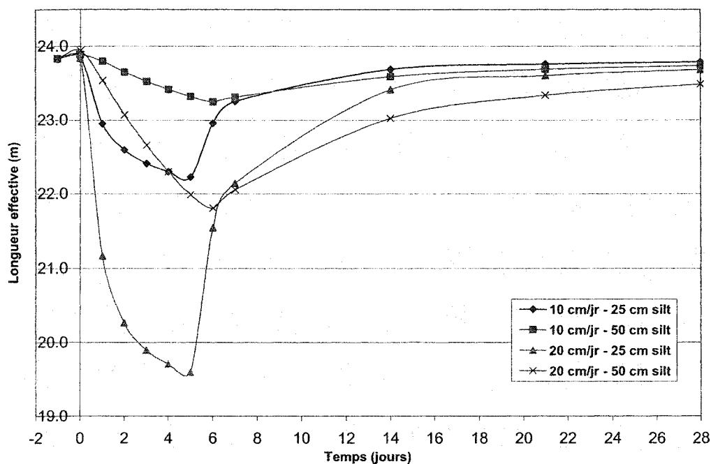
Figure 4.62 : Évolution de la longueur effective par rapport à l'épaisseur du silt et au taux de précipitations, lorsqu'il y a cinq jours de précipitations suivies d'un drainage libre jusqu'au 28ème jour.
