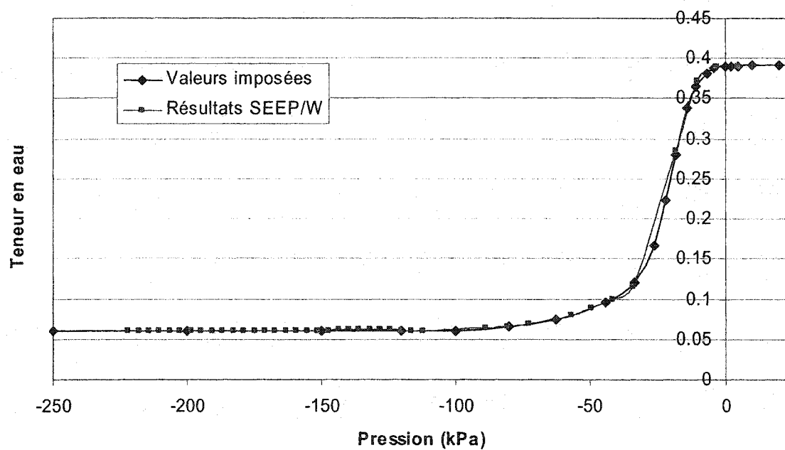
Figure 4.17 : Exemples de courbes de rétention d'eau imposées dans le modèle et ressorties avec les résultats.
