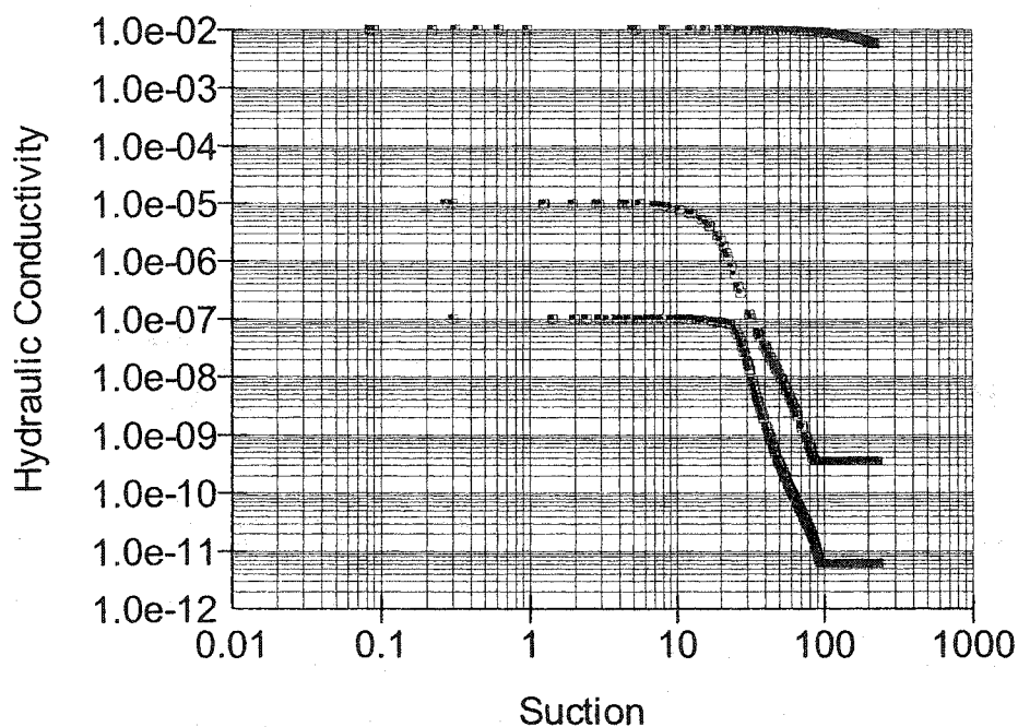
Figure 4.16 : Courbes de la conductivité hydraulique vs la succion imposées dans le modèle et ressorties avec les résultats. Graphique fait par SEEP/W avec en abscisse : succion en kPa ; en ordonnée : conductivité hydraulique en m/s. De bas en haut : silt, sable, matériau drainant.
