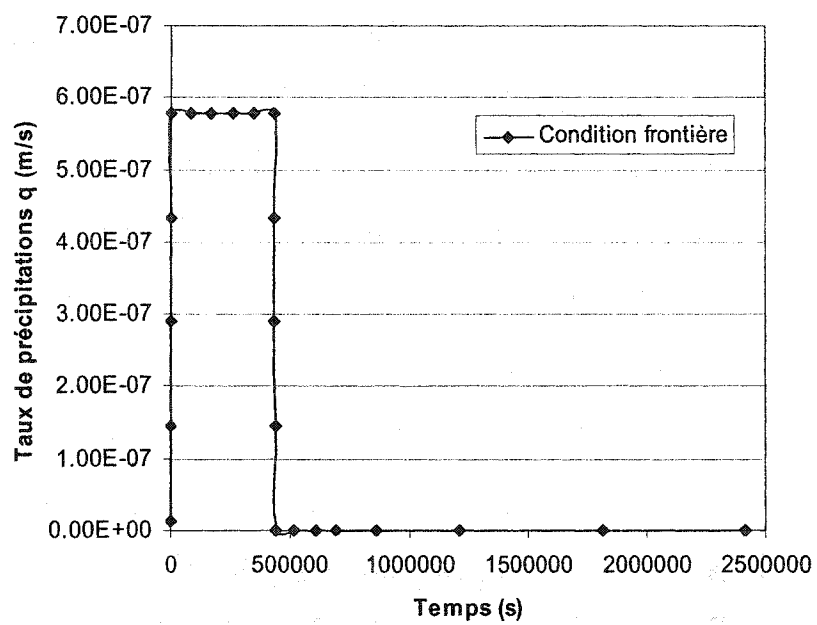
Figure 4.14 : Évolution du taux de précipitations pendant 28 jours avec cinq jours de pluie (5 cm/jr) et 23 jours de drainage
