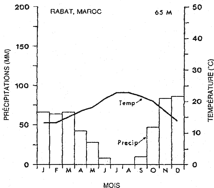
Figure 2.1a : Précipitations et températures annuelles à Rabat, Maroc (tirée de FAO, 1992).
