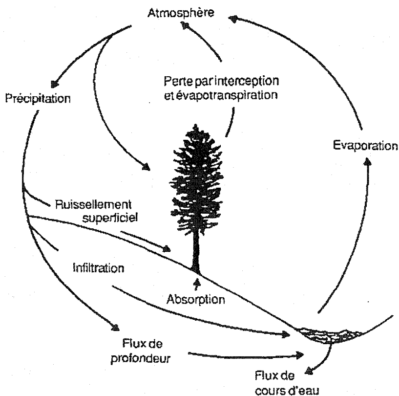
Figure 2.3 : Le cycle hydrologique (tirée de FAO, 1992).
