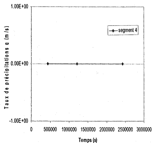
Figure 4.15d : 0 cm/jr de pluie pendant 28 jours : « plateau 2 »
