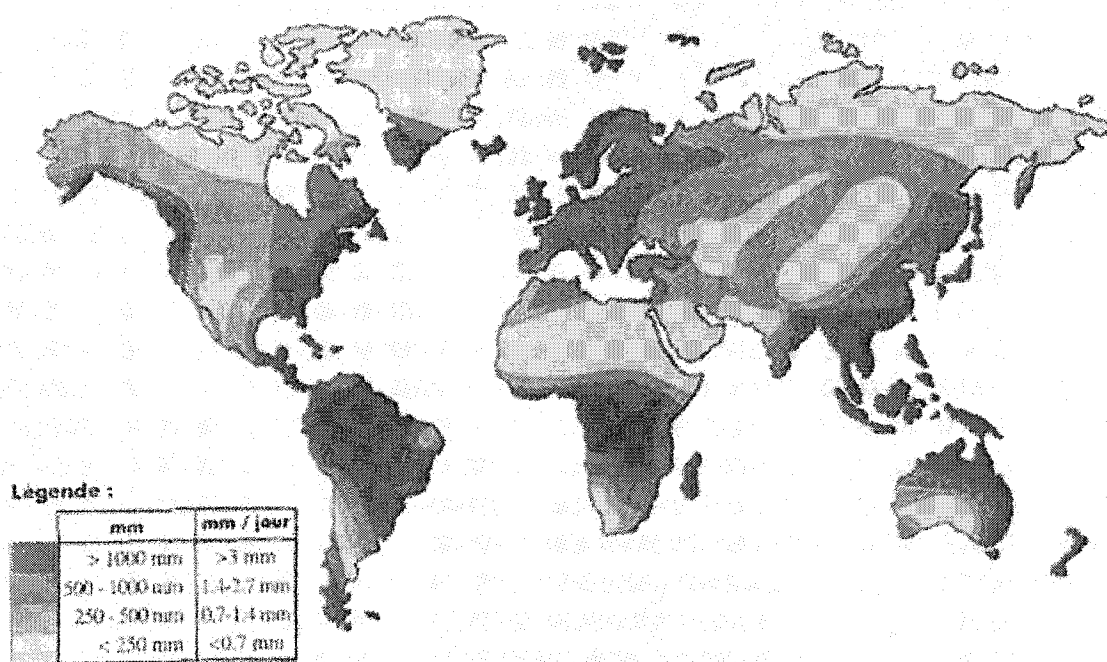
Figure 2.4 : Précipitations moyennes annuelles et journalières.
