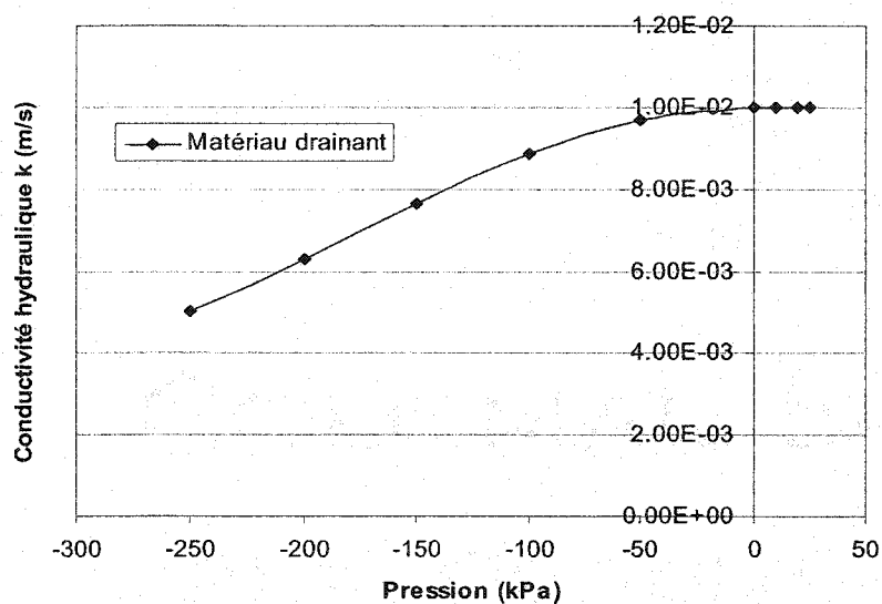
Figure 4.5 : Fonction de perméabilité : conductivité hydraulique vs. succion du matériau drainant avec k_s = 1 \cdot 10^{-2} m/s
