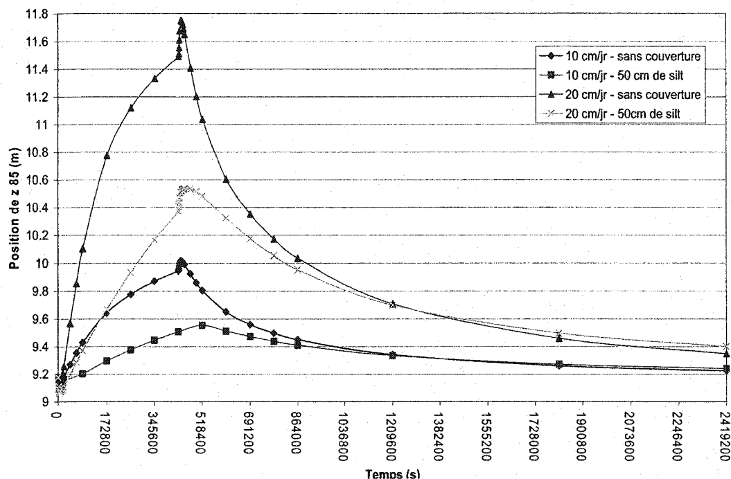
Figure 4.35 : Comparaisons entre les valeurs de z_{85} en fonction du temps en présence et en absence de couverture et avec des précipitations variables.
