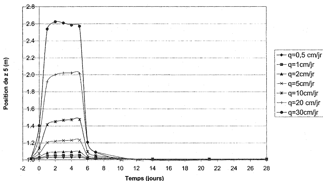
Figure 4.21 : Évolution de la position de z_5 en fonction des intensités et de la durée des précipitations (avec k_s du silt = 1 \cdot 10^{-6} m/s).
