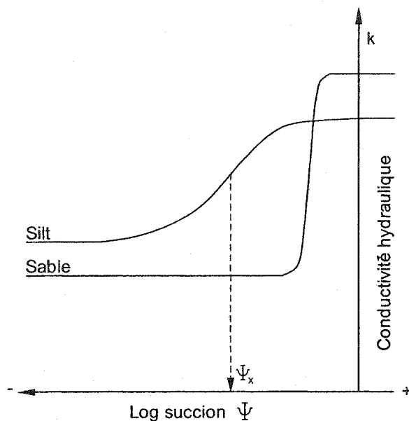
Figure 3.7 : Fonctions de perméabilité schématisées pour un sable et un silt (tirée d'Aubertin et al., 1995)
