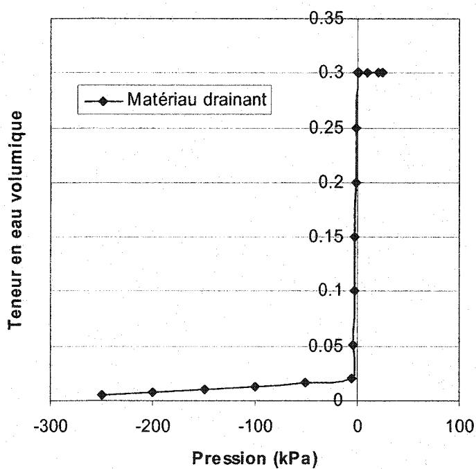
Figure 4.6 : Courbe de rétention d'eau : teneur en eau volumique vs. succion du matériau drainant
