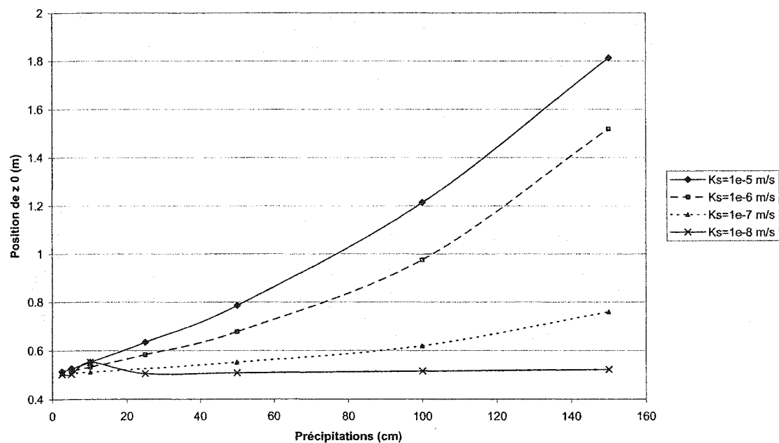
Figure 4.29 : Évolution de la position de z_0 par rapport à la quantité totale de précipitations après cinq jours à 1 m au-dessous de l'interface silt-sable.
