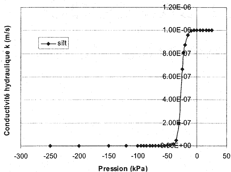
Figure 4.8 : Fonction de perméabilité : conductivité hydraulique vs. succion du matériau 2 b avec k_s = 1 \cdot 10^{-6} m/s
