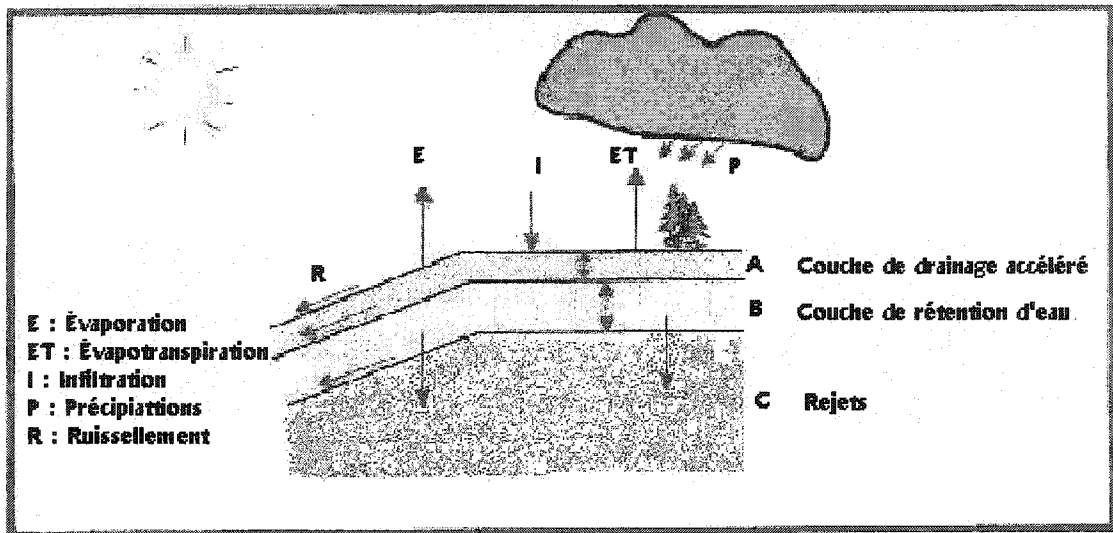
Figure 3.6: Échanges sol - atmosphère dans une couverture à effet de barrière capillaire.
