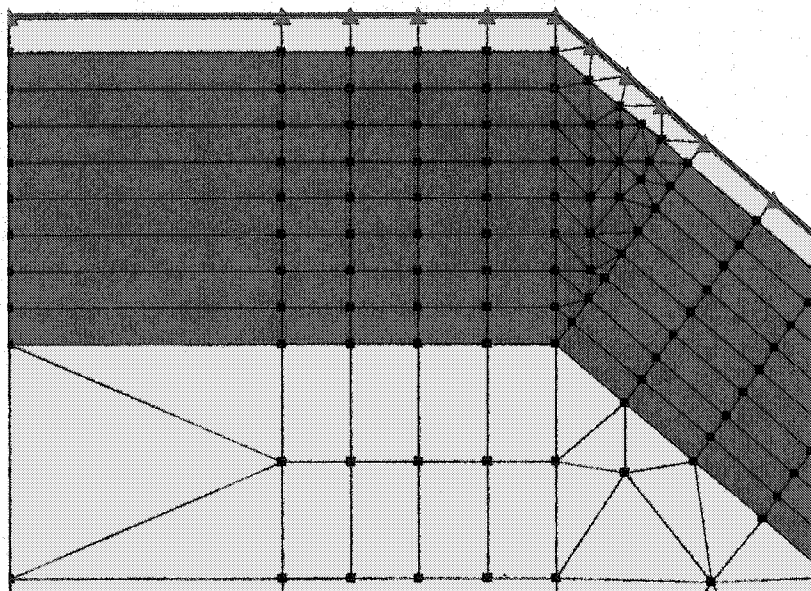
Figure 4.3 : Maillage au haut de la pente ; on voit la couche de ruissellement, la couverture de silt et les rejets (du haut vers le bas).
