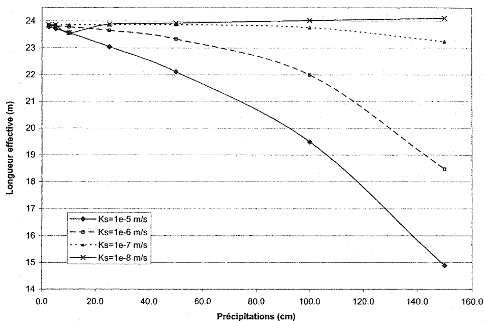
Figure 4.63 : Évolution de la longueur effective pour diverses valeurs de k_s du silt, selon le taux de précipitation (cinq jours de précipitations suivies d'un drainage libre jusqu'au 28ème jour) ; basée sur \psi_{85} au-dessus de l'interface silt-sable.
