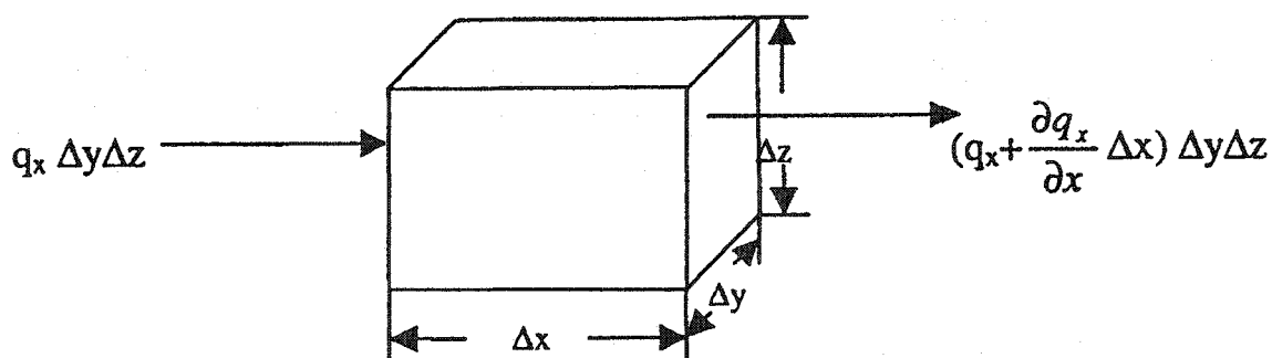
Figure 3.4 : Volume élémentaire de sol avec le bilan des débits (tirée de Hillel, 1998).
