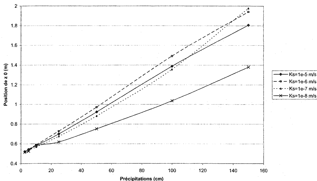
Figure 4.28 : Évolution de la position de z_0 par rapport à la quantité totale de précipitations après cinq jours à 12,5 cm au-dessus de l'interface silt-sable.
