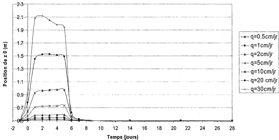
Figure 4.23 : Évolution de la position z_0 en fonction des intensités et de la durée des précipitations ( k_s du silt = 1 \cdot 10^{-6} m/s).
