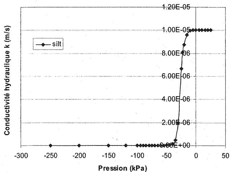
Figure 4.7 : Fonction de perméabilité : conductivité hydraulique vs. succion du matériau 2 a avec k_s = 1 \cdot 10^{-5} m/s
