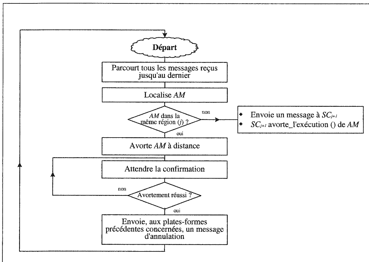
Figure 3.9 Organigramme de avorte_exécution() , exécuté par AS_j
