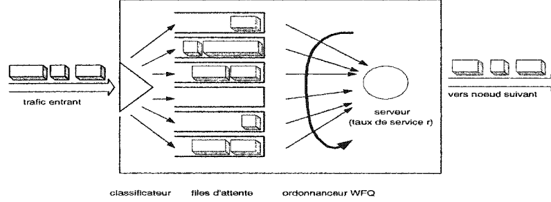
FIG. 3.2 – Ordonnanceur WFQ
