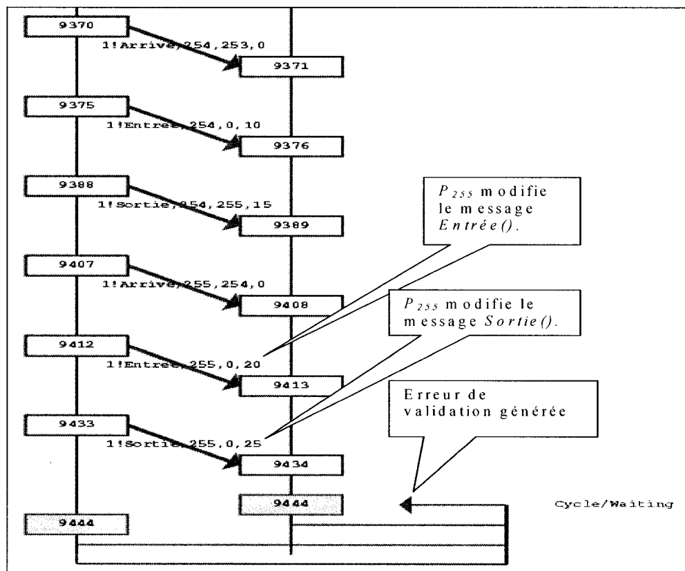
Figure 4.5 Explication de l'erreur de validation de la quatrième propriété, premier cas
