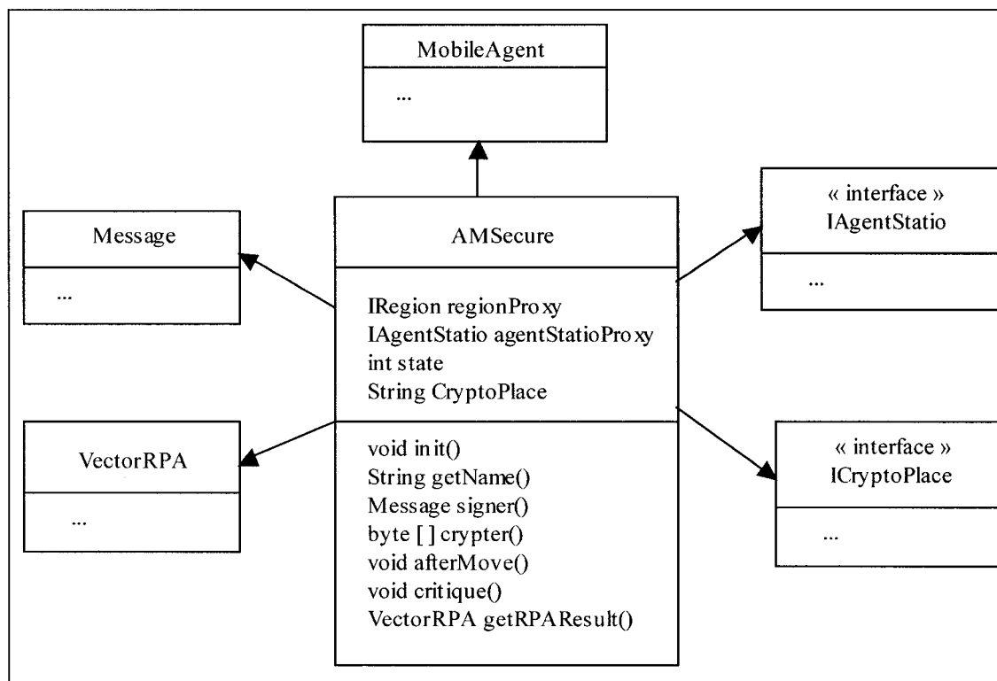
Figure 4.12 Diagramme de classe de l'agent AM
