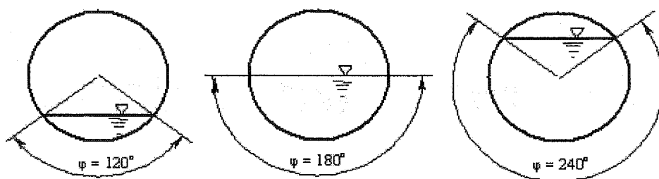
Figure 3.6 Niveaux de remplissage avec du liquide
