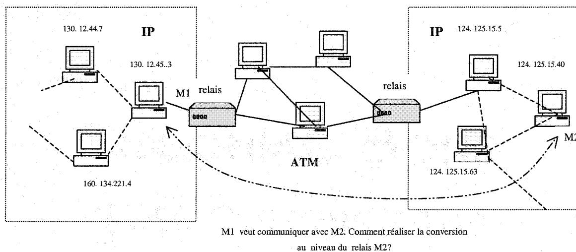
Figure 3.5 Problème de conversion d'adresses au niveau du relais
