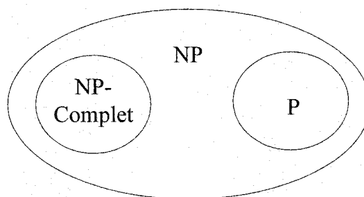
Figure 2.6 Les différentes classes de problèmes
