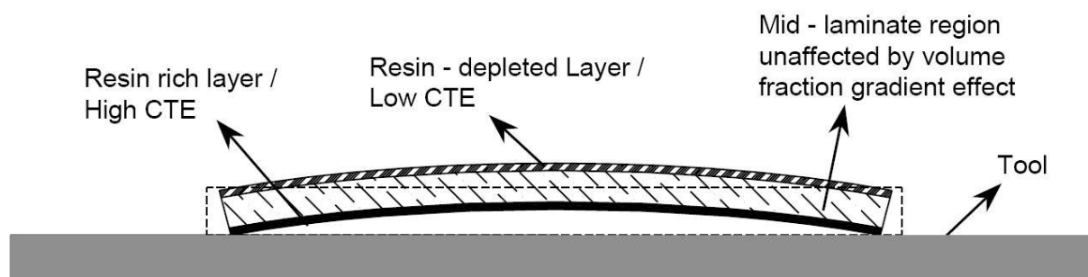
Figure 1-14 : Phénomène de gauchissement causé par un gradient de taux de fibres à travers l'épaisseur du composite (Bapanapalli et Smith, 2005).
