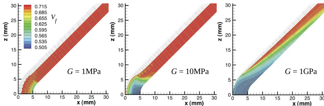
Figure 1-9 : Influence du comportement en cisaillement à travers l'épaisseur sur la consolidation d'un composite courbé prédite par simulation numérique (Li et Tucker III, 2002).
