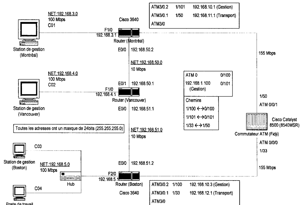
Figure 4.12 Réseau en triangle pour les tests de diagnostic
