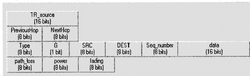
Figure 4.6 Format de l'entête d'un paquet DATA
