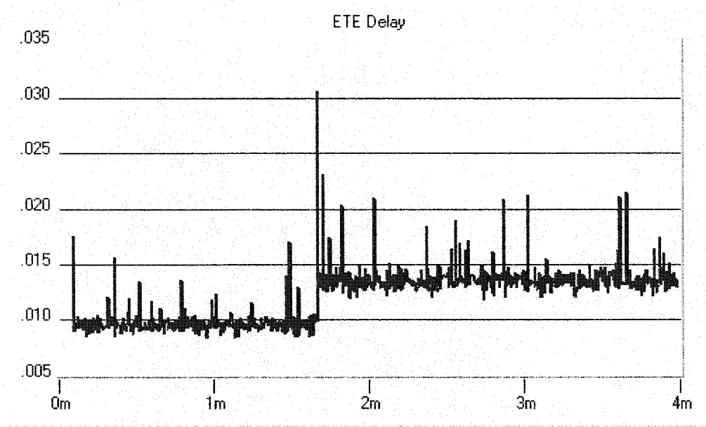
Figure 4.12 Délai ETE – départ du nœud 4 – cas 1 & 2
