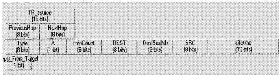
Figure 4.5 Format d'un paquet RREP
