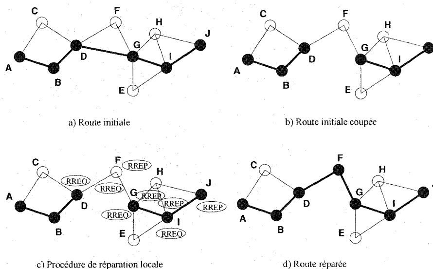
Figure 3.1 Restauration de route par re-routage partiel
