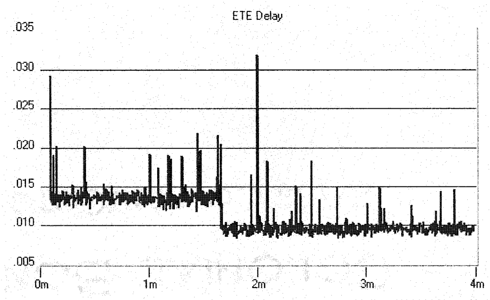
Figure 4.16 Délai ETE – départ du nœud 17 – cas 3
