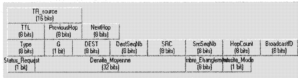
Figure 4.10 Représentation d'un paquet RREQ
