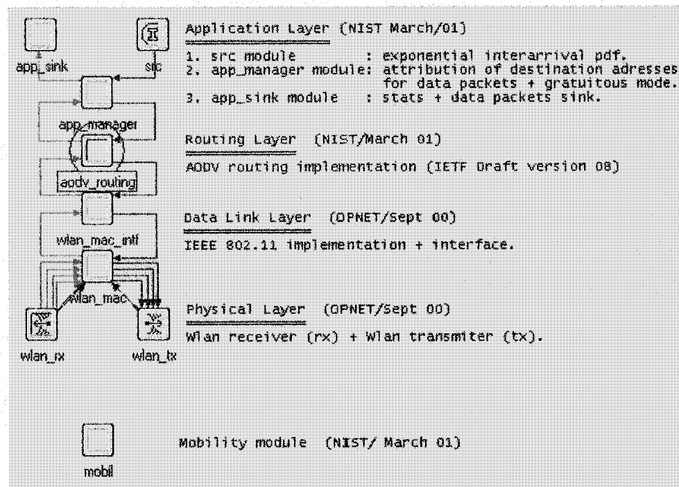
Figure 4.2 Modèle d'un nœud AODV
