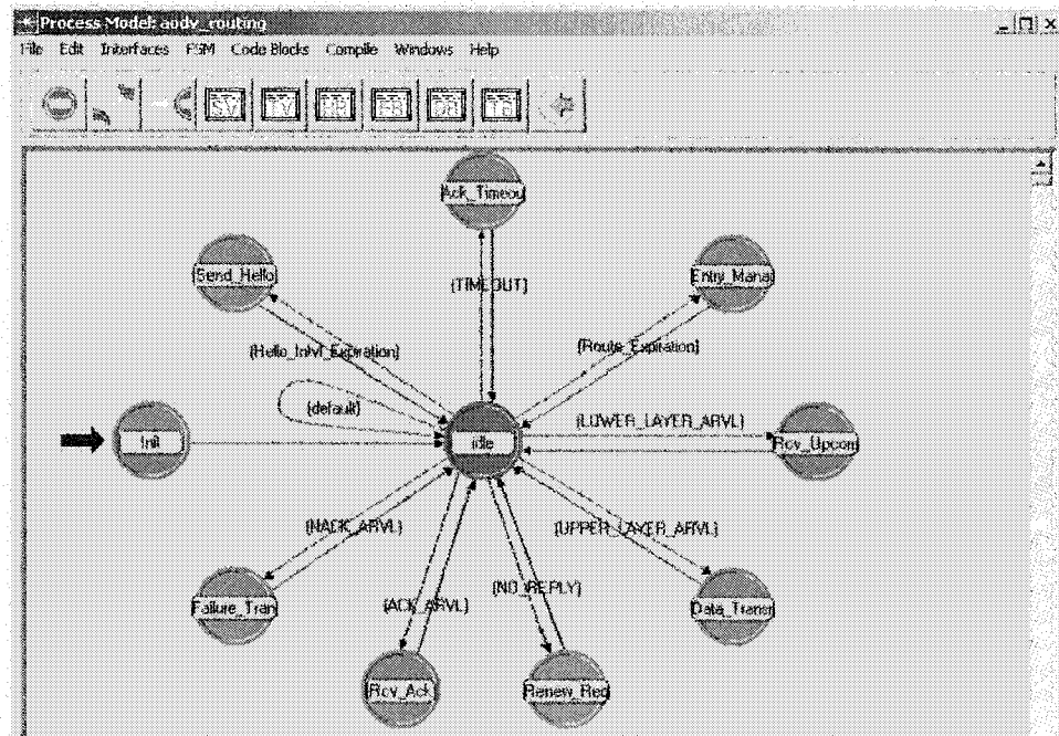
Figure 4.7 Représentation de la machine à états finis initiale
