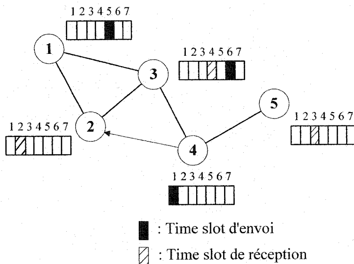
Figure 2.5 Affectation des slots dans l'algorithme de routage basé sur TDMA
