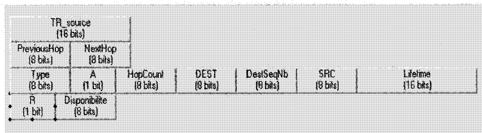
Figure 4.8 Représentation d'un paquet RREP
