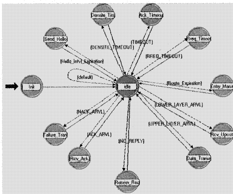
Figure 4.9 Représentation de la nouvelle machine à états finis
