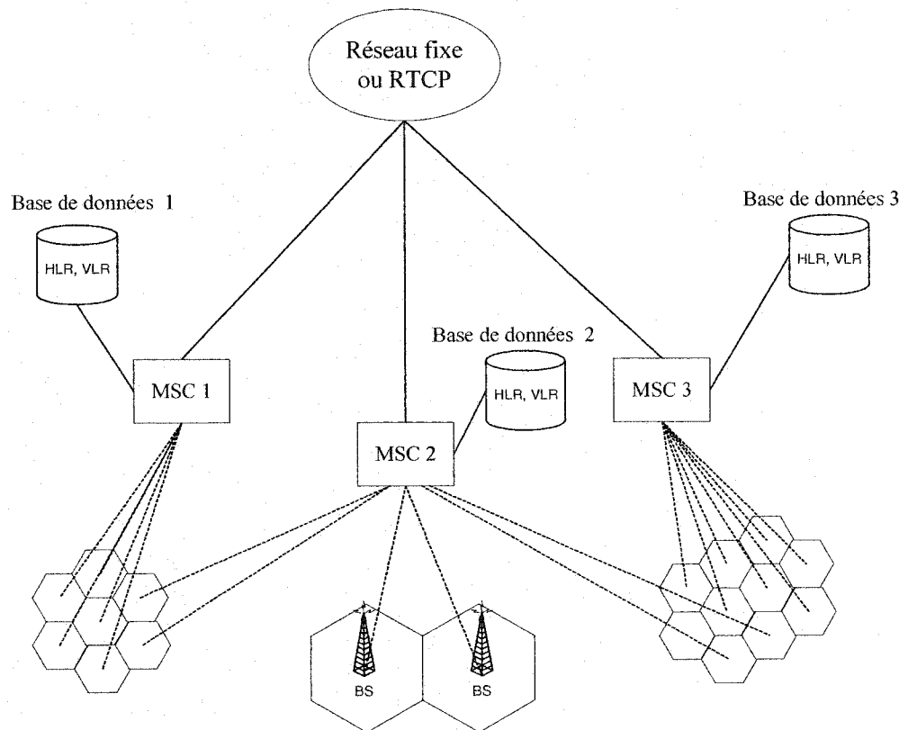
Figure 1.1 Architecture d'un réseau mobile cellulaire
