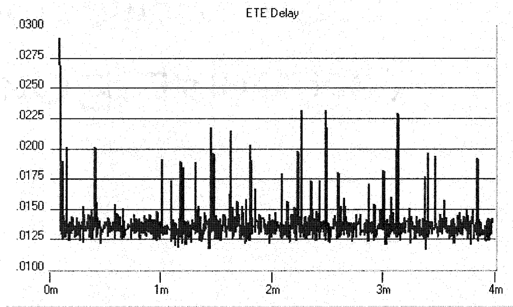
Figure 4.13 Délai ETE – départ du nœud 4 – cas 3
