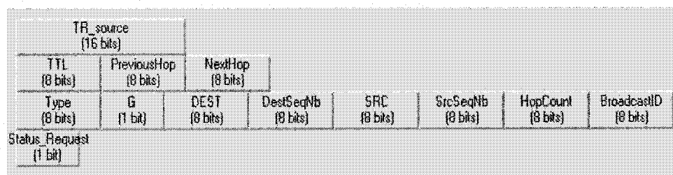
Figure 4.4 Format d'un paquet RREQ
