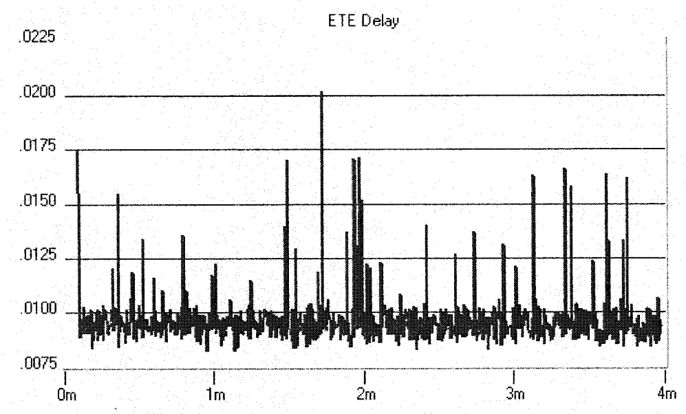
Figure 4.14 Délai ETE – départ du nœud 12 – cas 1 & 2
