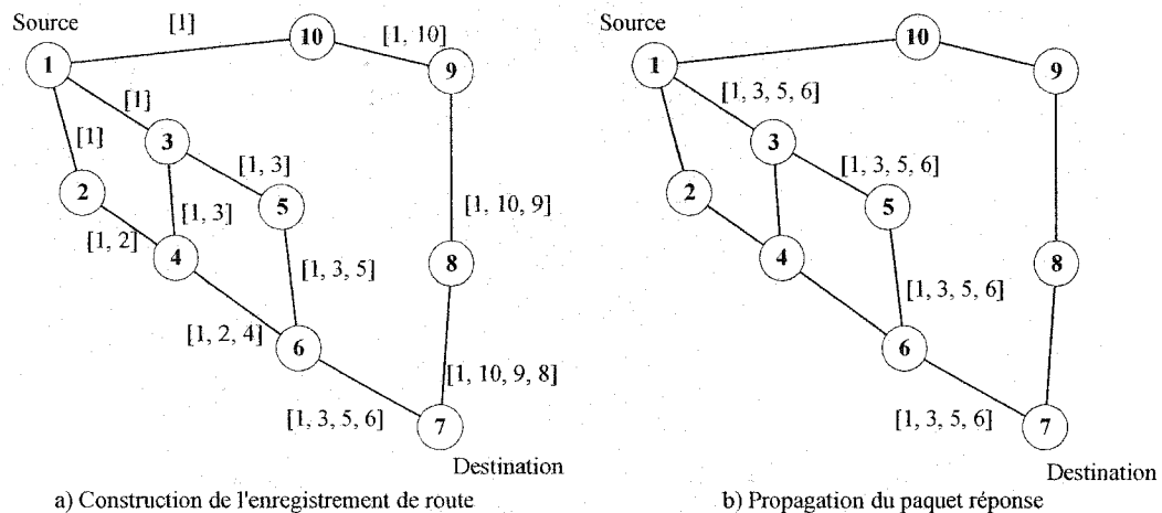
Figure 2.3 Découverte de chemins dans DSR
