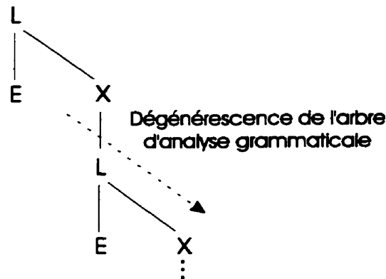
Figure 4.7 Dégénérescence de l'arbre d'analyse syntaxique avec la méthode LL(k)
