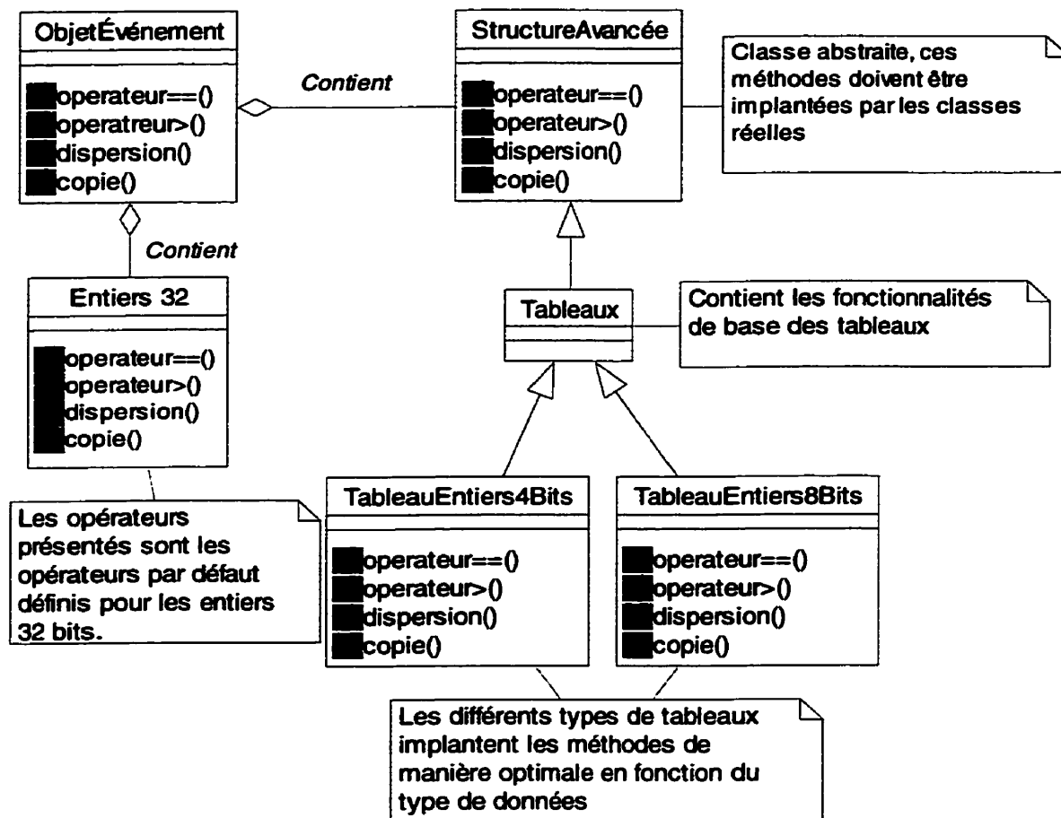
Figure 4.3 Hiérarchie des classes de l'objet événement
