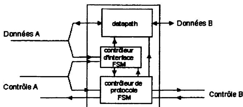
Figure 1.3. Architecture du module d'interface utilisé dans [SuBr92]
