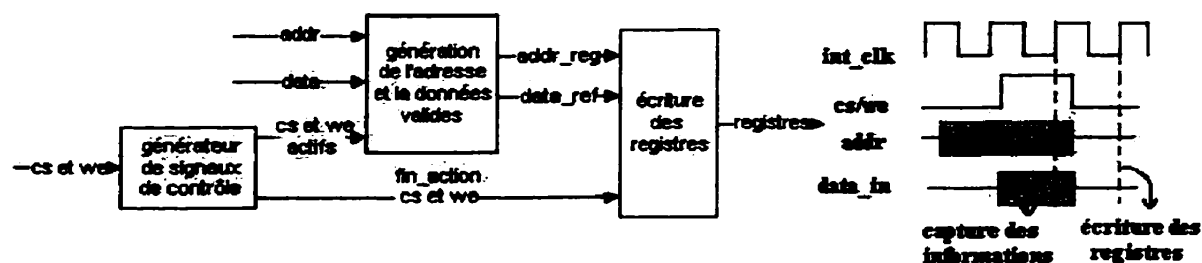
Figure 3.11. Schéma logique et diagramme temporel du bloc d'écriture
