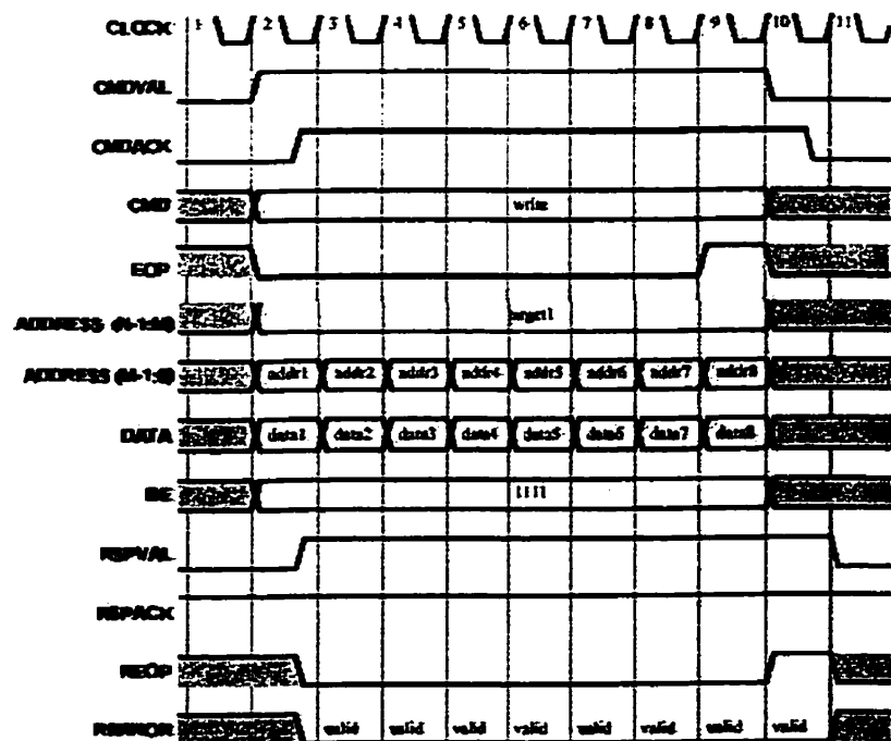
Figure H.4. Diagramme temporel d'une opération d'écriture
