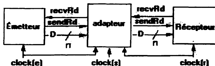
Figure F.2. Adapteur pour des processus d'horloges reliées
