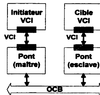
B) Connexion à travers un bus
