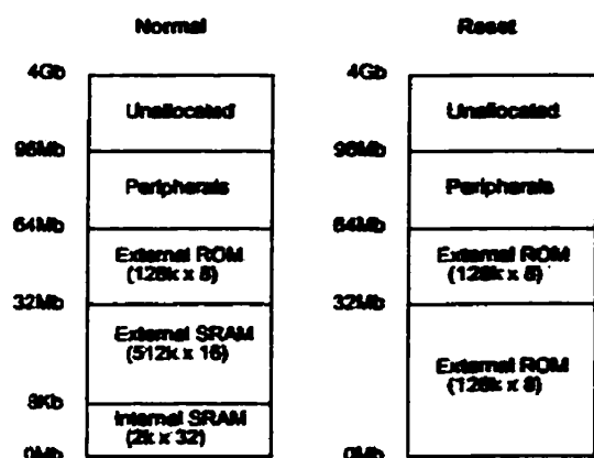
Figure G.8. Définition d'un espace d'adressage typique
