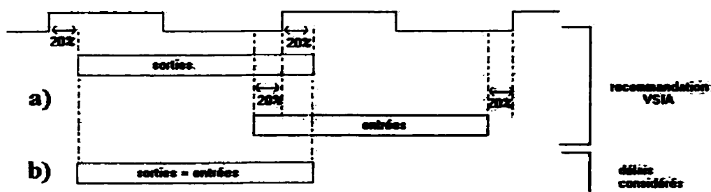
Figure 3.1. Spécifications des délais du protocole BVCI a) proposées par VSIA, b) utilisées dans le projet
