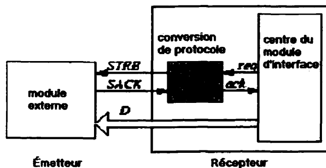
Figure F.4. Module d'interface synthétisée avec Integral
