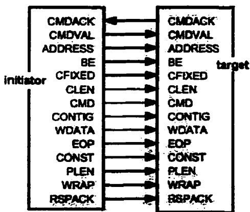
Figure H.1. Signaux du transfert d'une requête BVCI
