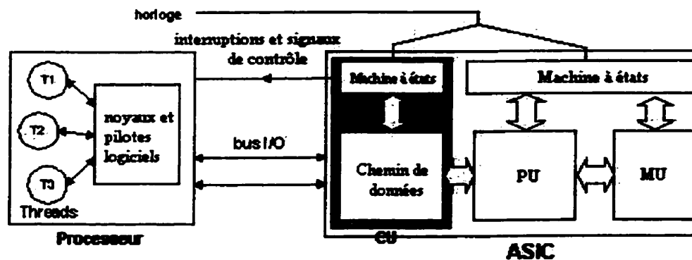
Figure 1.4. Architecture type du système proposé dans [BPM98]
