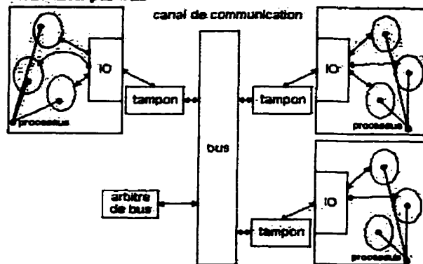
Figure 2.4. Modèles de communication
