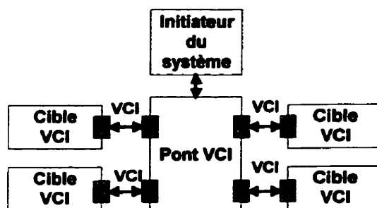
Figure 2.9. Topologies proposées par VSIA
