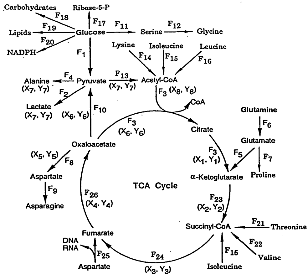
Figure 1.1 : Diagramme simplifié du réseau de réactions impliquant le glucose et la glutamine d'après Xie et Wang (1996).
