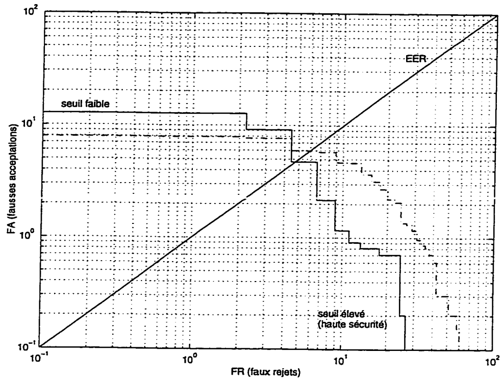
Figure 6.24: Courbes DET. Schème 4545. Modèle à 16 gaussiennes. Fichier test tronqué à 30 secondes. Normalisation: muselière (trait plein: -) et cohorte (trait pointillé: -.).
