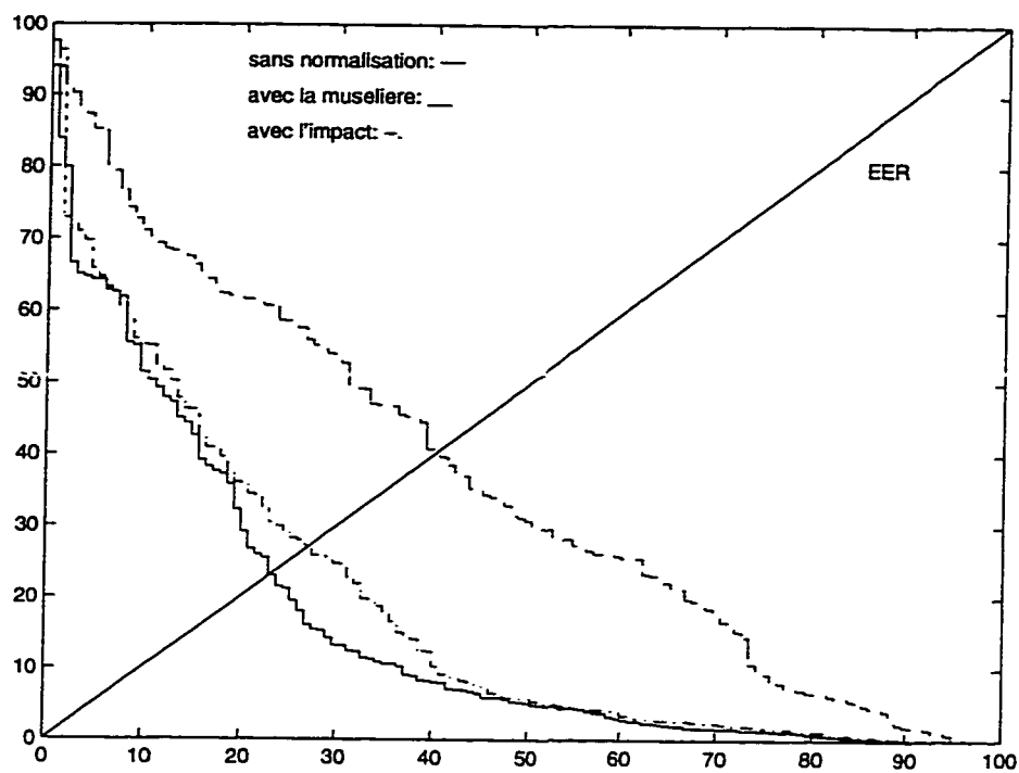
Figure 6.21: Courbes ROC. Schème 13545. Modèle à 16 gaussiennes. Fichier test tronqué à 03 secondes.
