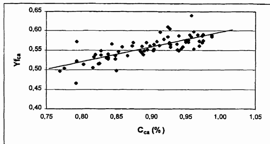
Figure 1.5: Fraction de fines dans la caisse d'arrivée versus consistance.
