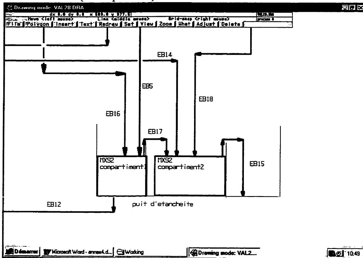
Figure IV.13: Puit d'étanchéité (CADSIM® Plus PAPDYN®).
