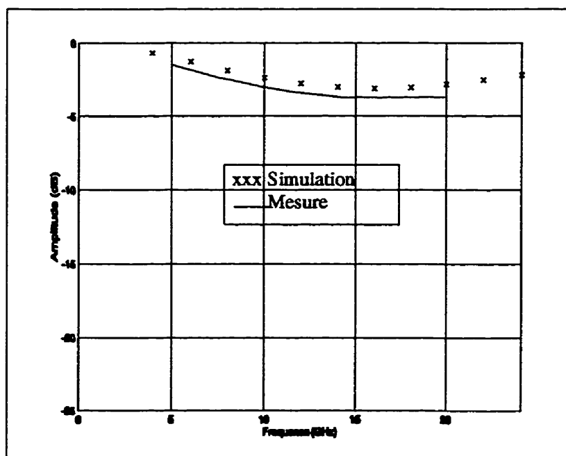
Figure 4.25: Transmission du coupleur multioctaves
