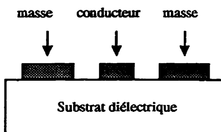
Figure 4.1: Vue de dessus et coupe transversale d'une ligne coplaire
