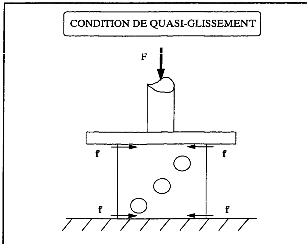
Figure 5.2 : Condition de quasi-glissement. F : force de compression ; f : force de frottement.
