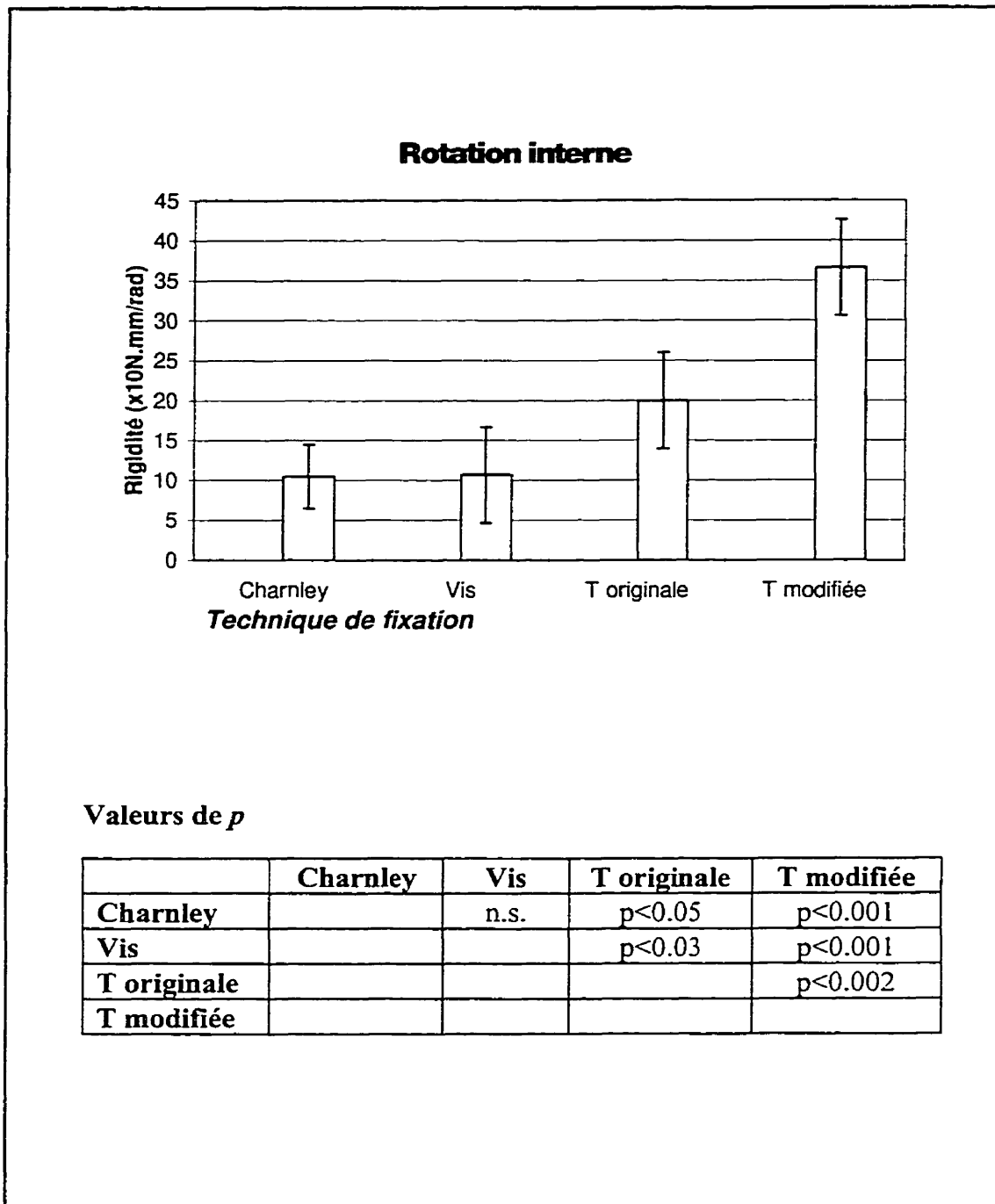
Figure 16 - Résultats de rigidité en rotation interne
