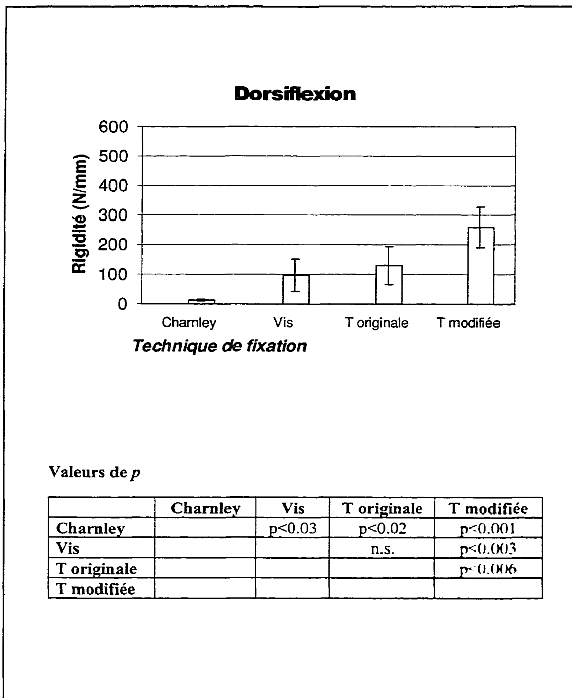
Figure 14 - Résultats de rigidité en dorsiflexion
