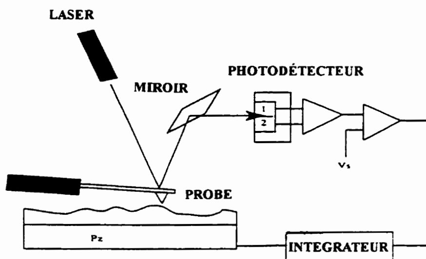
Figure 3.4 Le microscope à force atomique, l'instrument [93].
