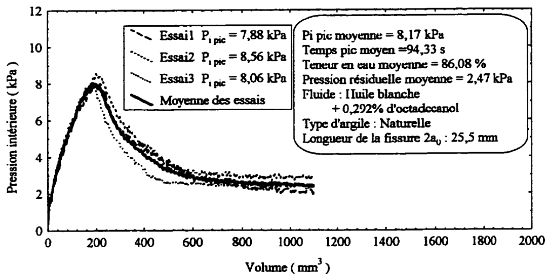
Figure A.5 : Courbe de fracturation (PHCFT) avec l'huile blanche +0,292% d'octadecanol, pour une argile naturelle et 2a_0 = 25,5 \text{ mm}
