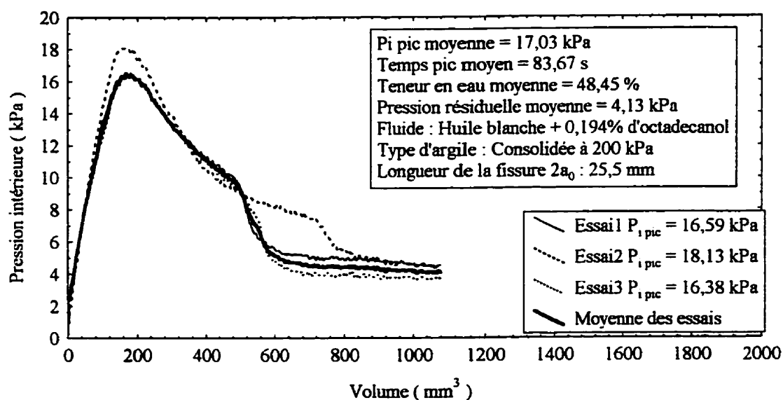
Figure A.11 : Courbe de fracturation (PHCFT) avec l'huile blanche +0,194% d'octadecanol, pour une argile consolidée à 200 kPa et 2a_0 = 25,5 \text{ mm}
