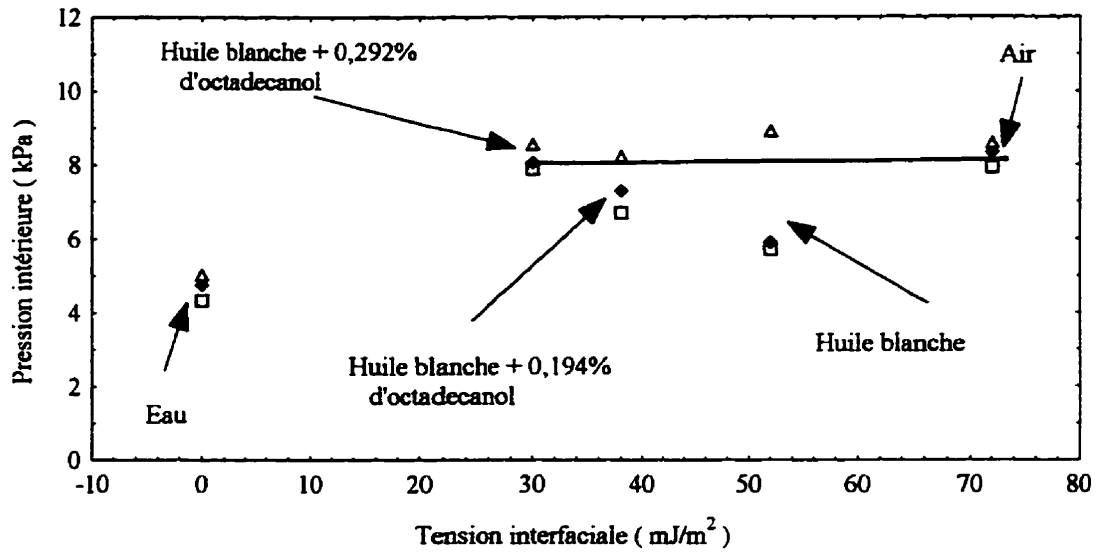
Figure 6.6 : Influence de la tension interfaciale sur la pression au pic avec une argile naturelle et 2a_0 = 25,5 mm
