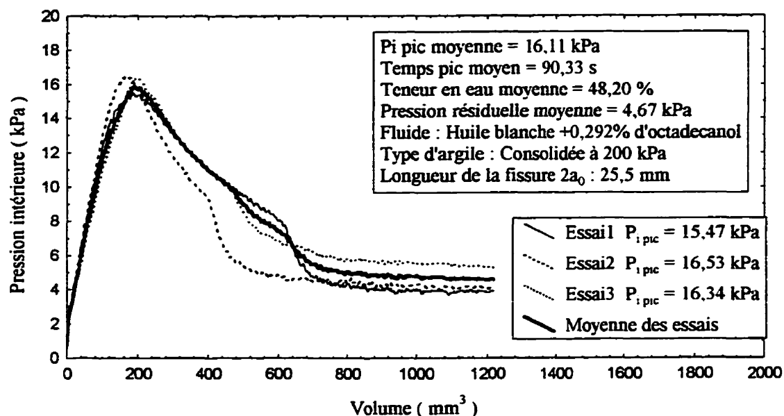
Figure A.13 : Courbe de fracturation (PHCFT) avec l'huile blanche +0,292% d'octadecanol, pour une argile consolidée à 200 kPa et 2a_0 = 25,5 \text{ mm}
