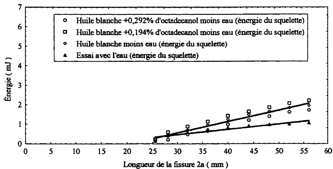
Figure 7.23 : Comparaison de l'énergie de fissuration du squelette et celle de l'eau pour 2a_0 = 25,5 mm
