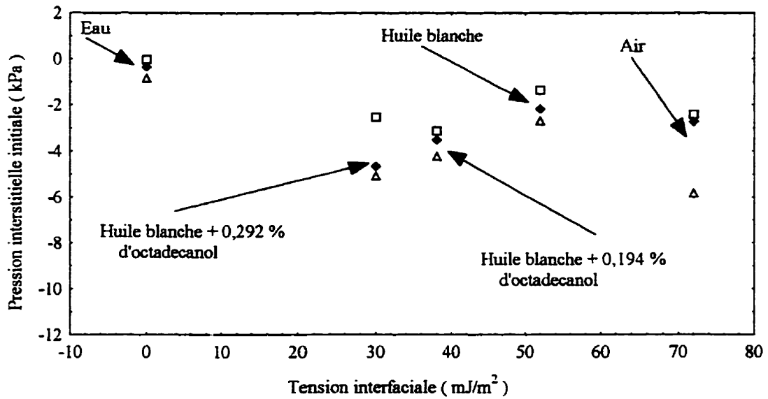
Figure 6.7: Influence de la tension interfaciale sur la pression interstitielle avec une argile naturelle et 2a_0 = 25,5 mm
