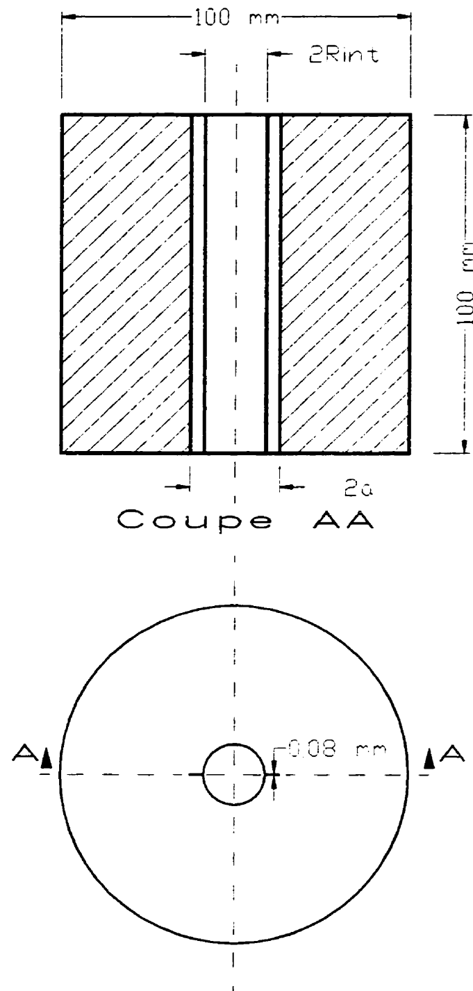
Figure 5.1 : Représentation schématique de l'échantillon cylindrique creux
