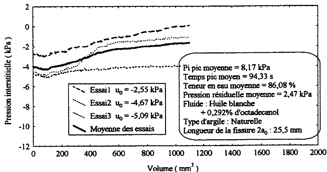
Figure A.6 : Variation de la pression interstitielle pendant l'essai avec l'huile blanche +0,292% d'octadecanol, pour une argile naturelle et 2a_0 = 25,5 \text{ mm}
