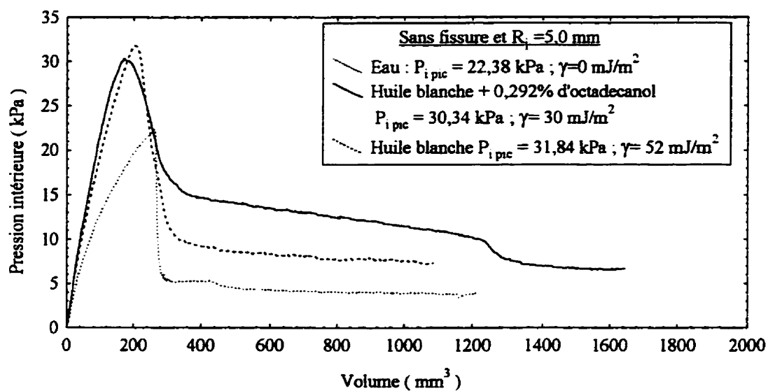
Figure 6.24 : Courbe de fracturation (PHCFT) avec tous les fluides, pour une argile consolidée à 200 kPa et sans fissure
