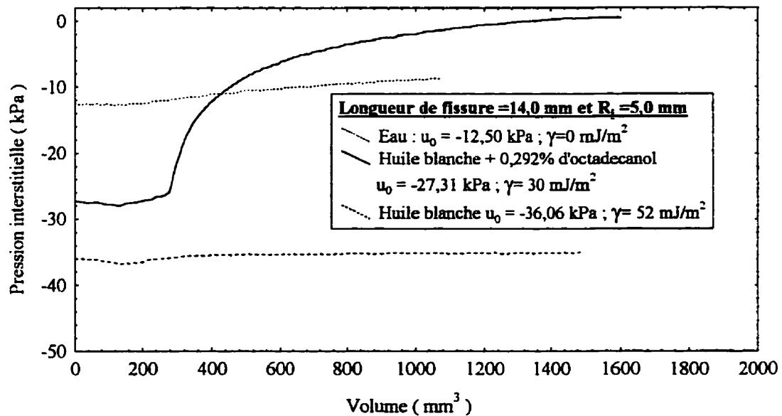
Figure 6.19 : Variation de la pression interstitielle pour tous les fluides (sauf l'air) pour une argile consolidée à 200 kPa et 2a_0 = 14,0 mm
