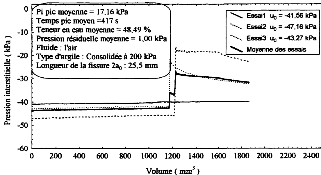
Figure A.16 : Variation de la pression interstitielle pendant l'essai avec l'air, pour une argile consolidée à 200 kPa et 2a_0 = 25,5 \text{ mm}
