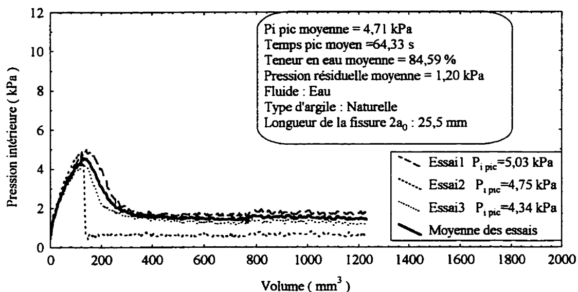
Figure 6.2 : Courbe de fracturation (PHCFT) avec l'eau, pour une argile naturelle et 2a_0 = 25,5 \text{ mm}
