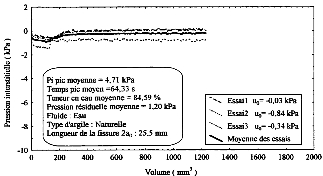
Figure 6.3 : Variation de la pression interstitielle pendant l'essai avec l'eau, pour une argile naturelle et 2a_0 = 25,5 \text{ mm}
