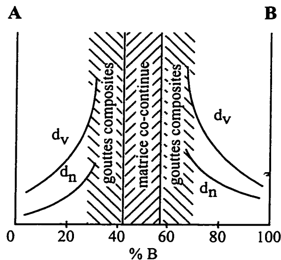
Figure I.2. Variation du diamètre moyen en nombre d_n et en volume d_v dans un système biphasé A-B selon la teneur en phase B; le diagramme montre la région où les gouttes composites sont observées ainsi que le domaine de co-continuité.
