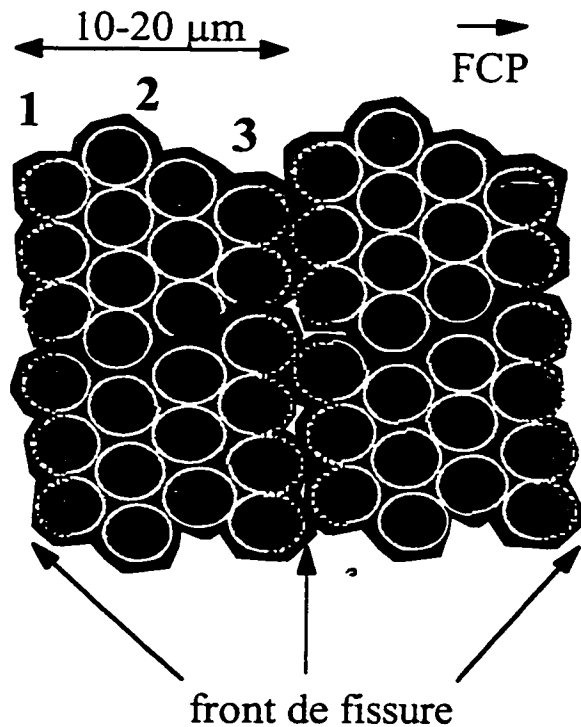
Figure II.5. Modèle de formation des super-cupules observées à da/dN relativement élevé dans les mélanges polystyrène/polyéthylène.
