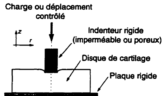
Figure 1.4: Le test d'indentation
