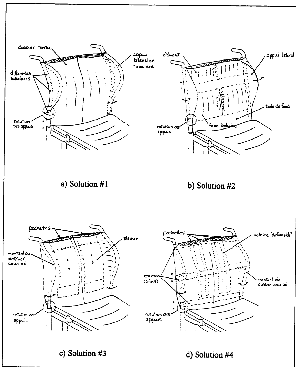
Figure 2.4 – a) Dossier à tubulures profilées; b) Dossier flexible avec éléments de forme; c) Dossier flexible avec plaques intégrées; d) Dossier contour flexible
