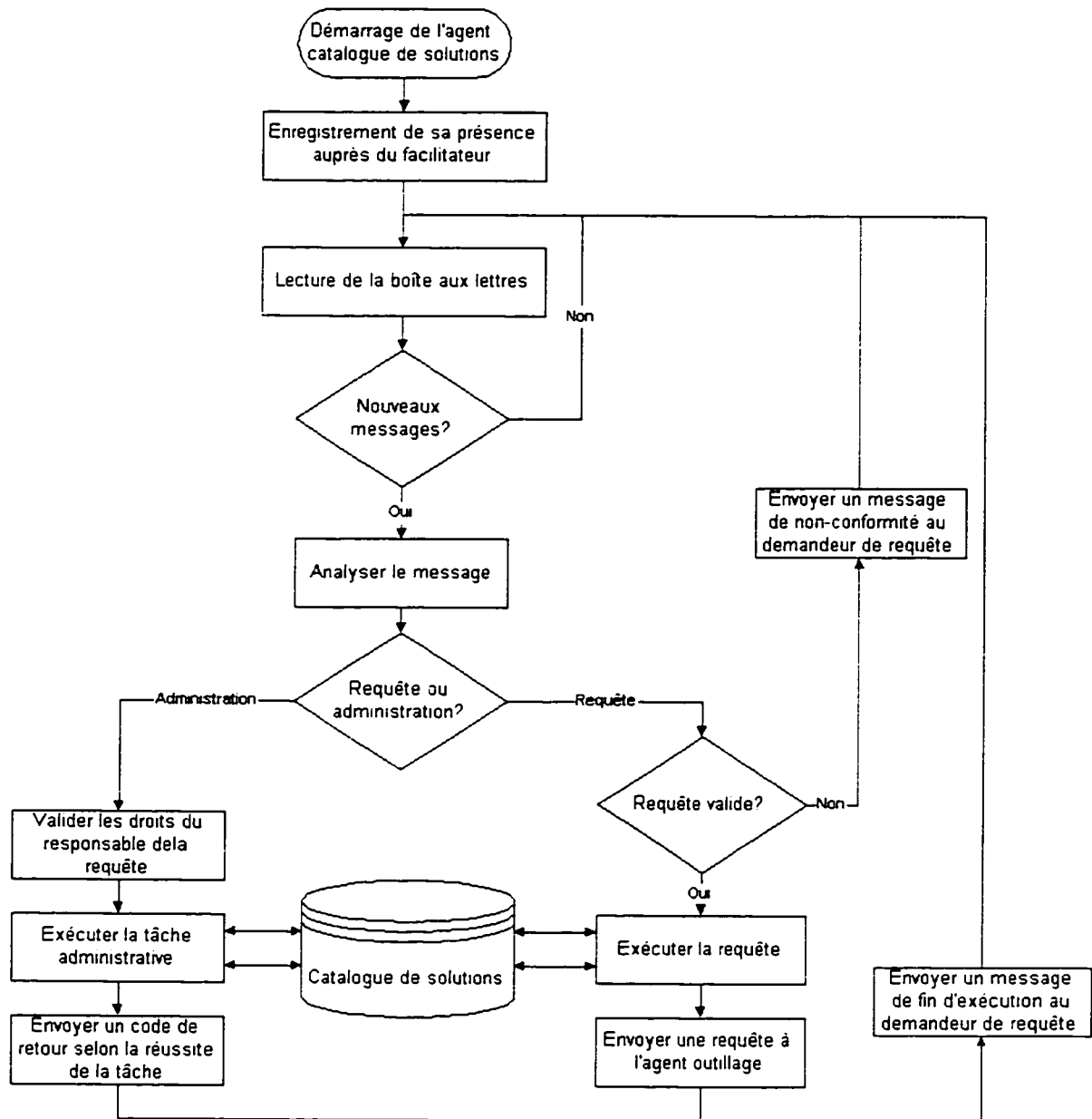
Figure 3.14 : Diagramme logique de l'agent catalogue de solutions d'assemblage
