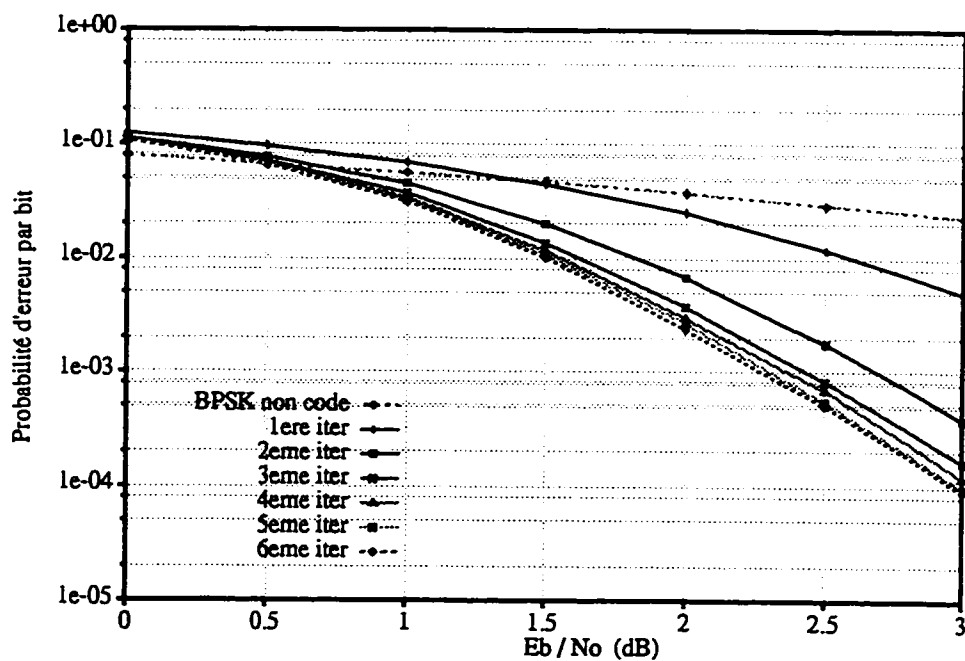
Figure A1.1.5 Performances d'erreur du code turbo de taux R=1/2 , avec K=3 , G=(1, 5/7) , N=196 , Entrel. aléatoire
