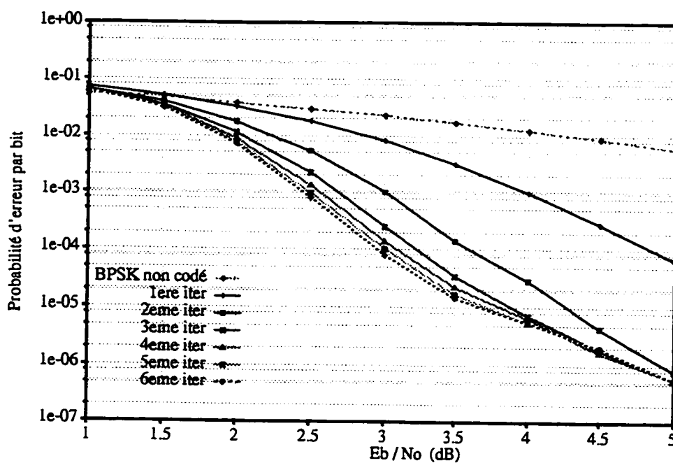
Figure A2.1.6 Performances d'erreur du code turbo de taux R=4/6 , avec K=3 , G=(1, 5/7) , N=900 , Entrel. aléatoire
