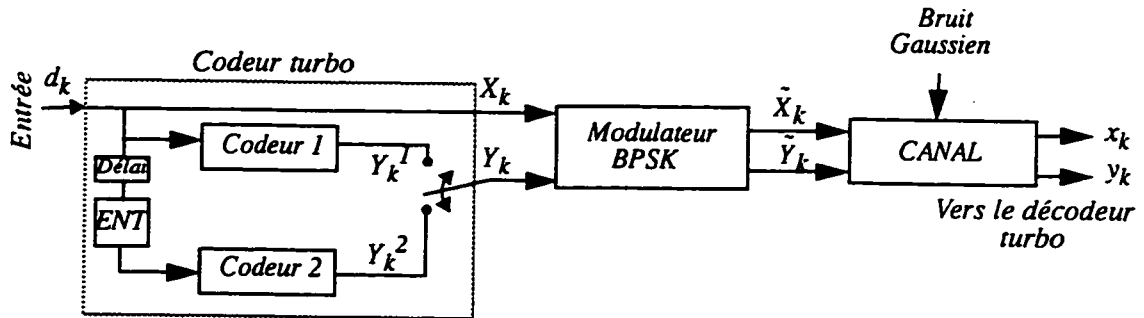
Figure 2.8 Structure du système à l'émission, codage turbo, R=1/2
