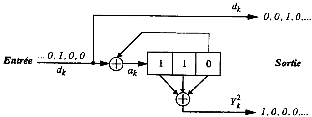
Figure 2.4 Codeur convolutionnel récursif systématique R=1/2, K=3, G=(1, 7/5) .
