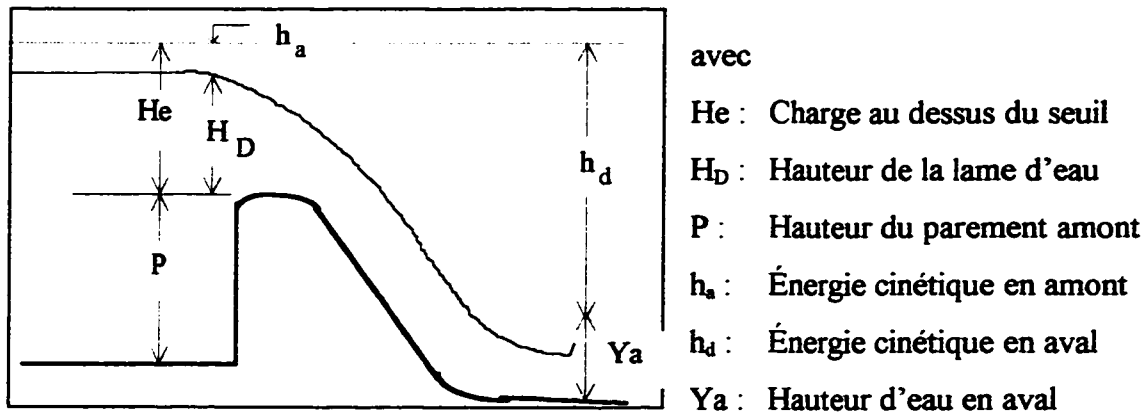
Figure 3.2: Coefficients hydrauliques utilisés
