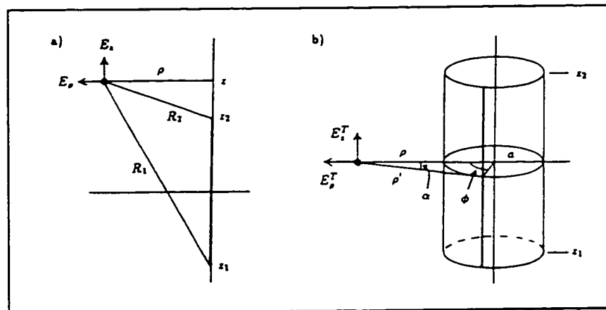
Figure 1.2: Evaluation du champ électrique crée par la distribution tubulaire de courant sur les segments (fig. extraite de Burke (1992)).
