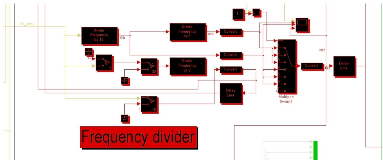
Figure 3-28 : Modèle Simulink du contrôle temporel de la matrice.
