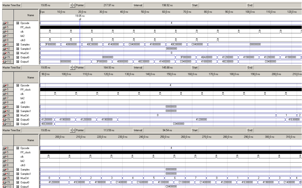
Figure 3-23 : Contrôle temporel de l'algorithme FFT radical-4, ordre N=16 .
