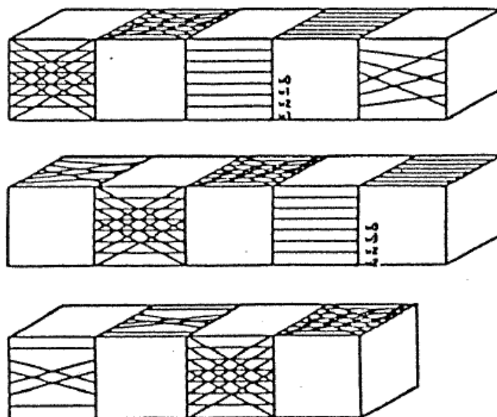
Figure 2-30 : Processeur d'image à géométrie constante parallèle utilisant un UPE base 2 [10].
