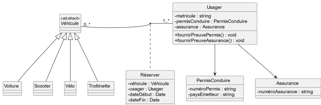
Fig. 1. Exemple de diagramme de classes fourni dans le Guide UML [13].
