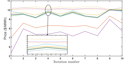
(d) DSO's pricing strategy in Scenario 7.
