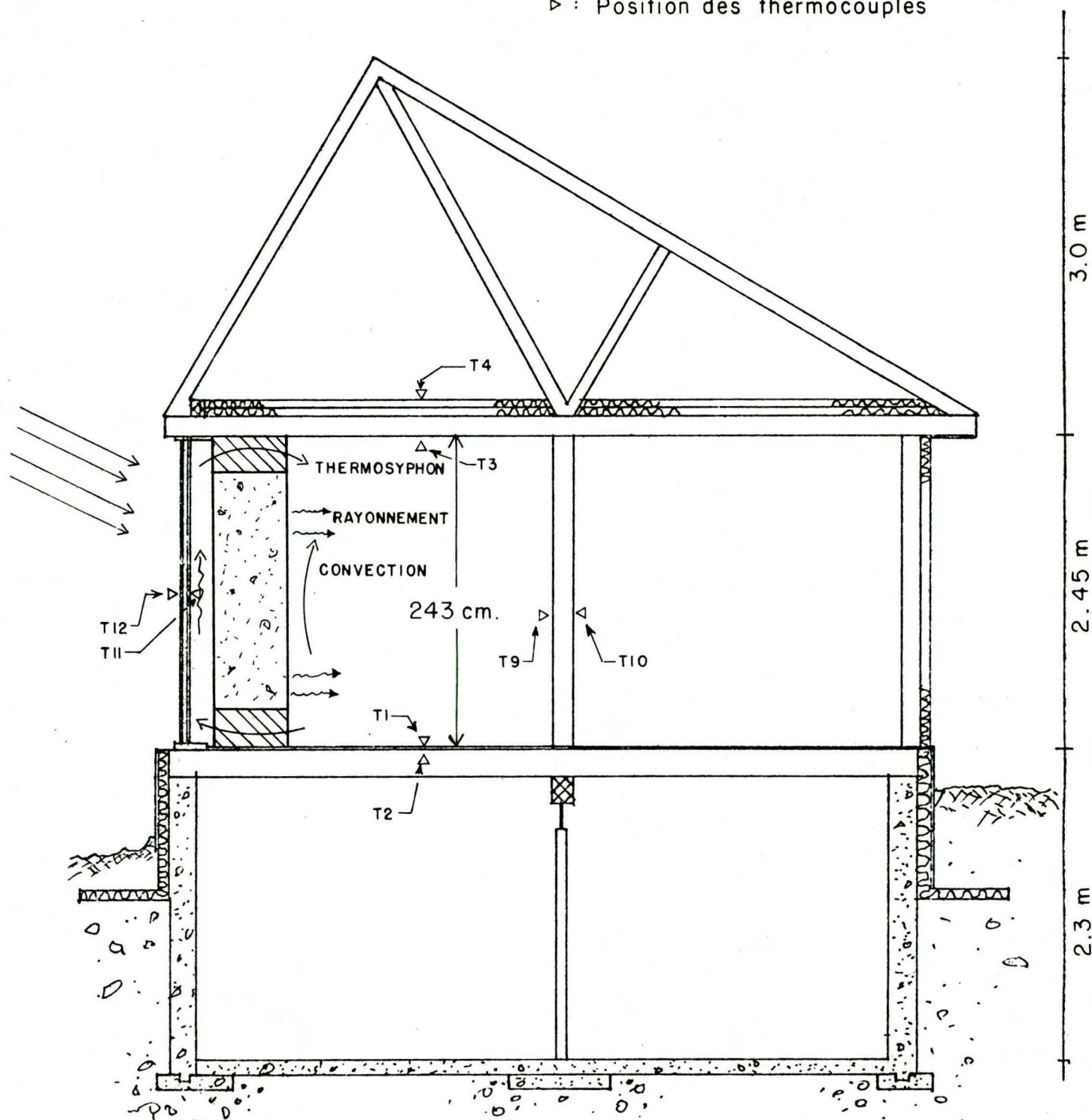
FIG. 3 Cellule du mur Trombe, vue en coupe
