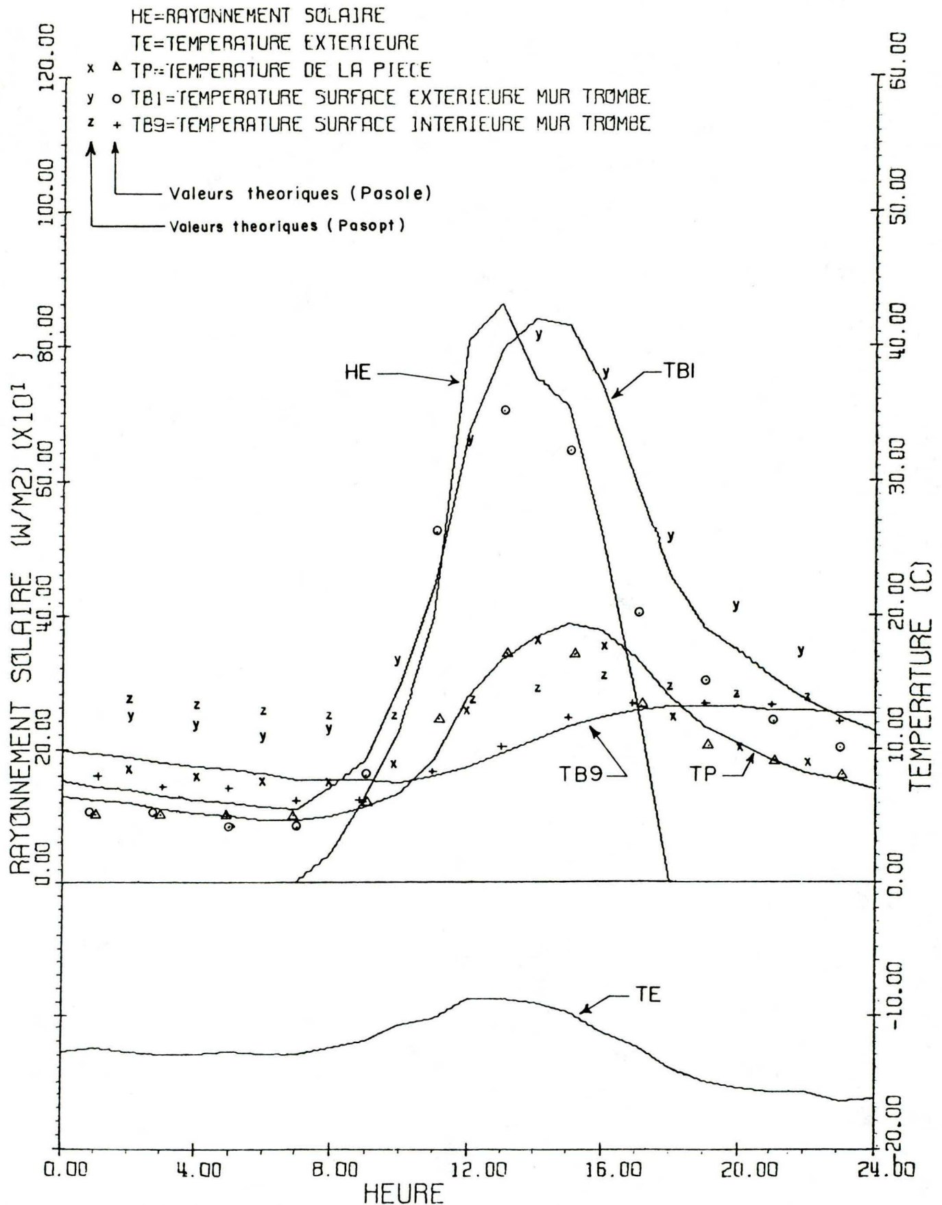
FIG. 8 Variation du rayonnement et des températures
