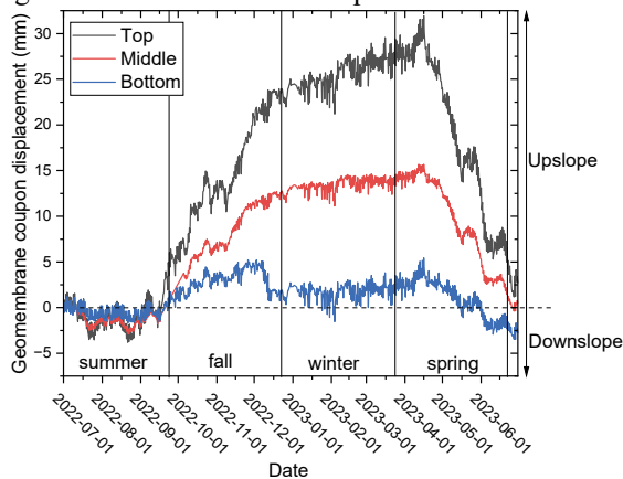
Fig. 9. Geomembrane coupon displacement.
