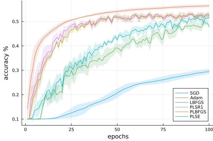
Figure 0.7 Précision au cours des époques pour différentes méthodes d’entraînement considérant PSNet et \mathcal{L}^{\text{PSL}} sur CIFAR10, L = 100 .
