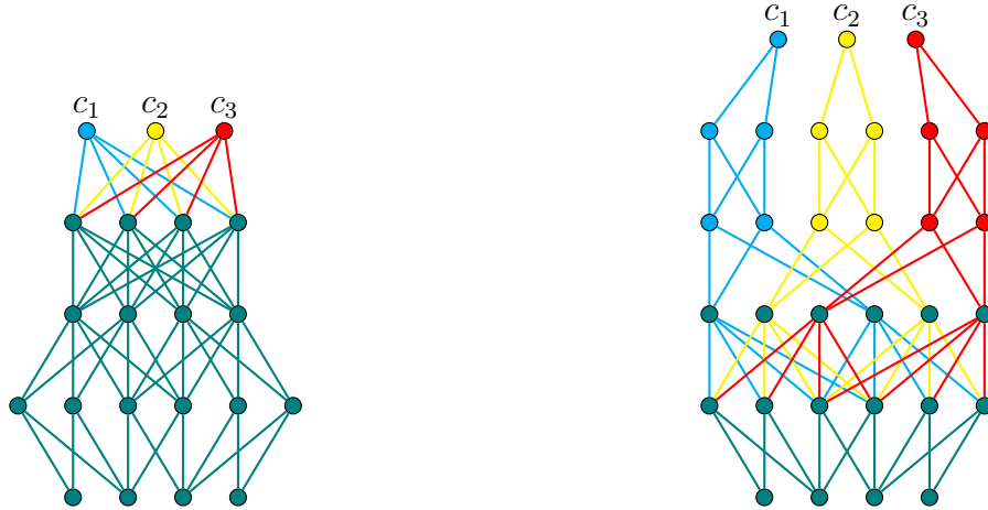
Figure 0.3 Dépendance des poids de chaque score, pour des réseaux LeNet (gauche) et PSNet (droite) simplifiés.
