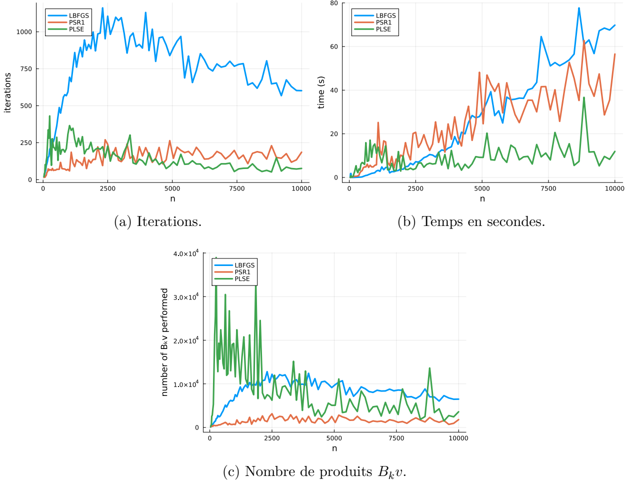
Figure 0.1 Performance des méthodes quasi-Newton minimisant f^{\text{limit}} (4).
