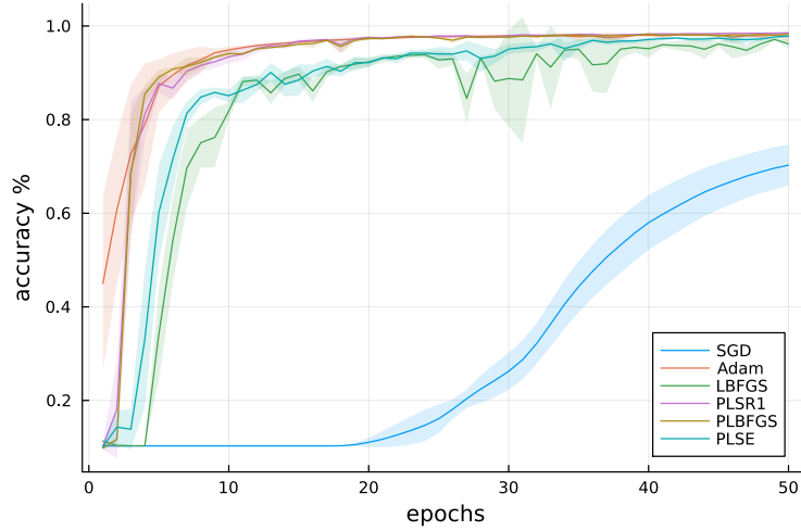
Figure 0.6 Précision au cours des époques pour différentes méthodes d'entraînement considérant PSNet et \mathcal{L}^{\text{PSL}} sur MNIST, L = 100 .
