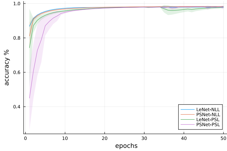
Figure 0.4 Précision au cours des époques de LeNet et PSNet pour \mathcal{L}^{\text{NLL}} et \mathcal{L}^{\text{PSL}} sur MNIST L = 100 .
