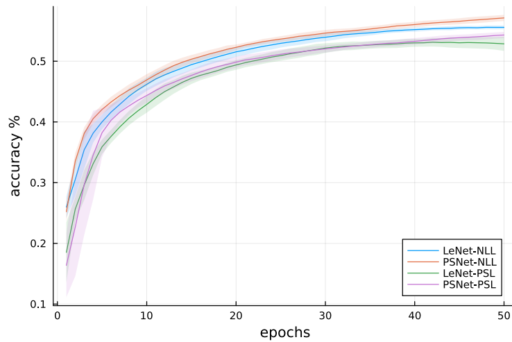
Figure 0.5 Précision au cours des époques de LeNet et PSNet pour \mathcal{L}^{\text{NLL}} et \mathcal{L}^{\text{PSL}} sur CIFAR10 L = 100 .
