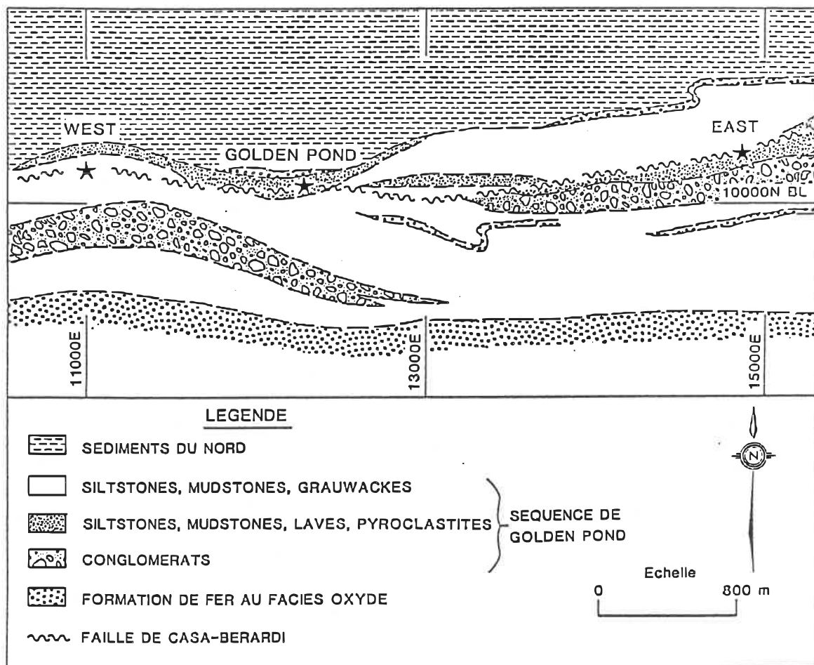
Figure 3.1: Géologie locale autour des trois gisements de Golden Pond (Modifié d'après Pattison et al. , 1986)
