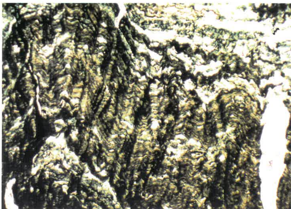
Figure 4.10: Schiste à séricite, graphite et carbonate extrêmement crénulé. Remarquez la limpidité de la veine de quartz recoupant la foliation (à droite) comparativement aux bandes de quartz et de carbonate (en haut, à droite) (éch. CB60738, 31,25X, L.N.).
