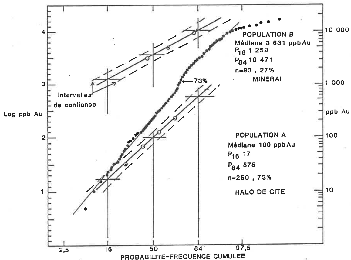
Figure 6.3: Diagramme de probabilité-fréquence cumulée de la section 14 960 E
