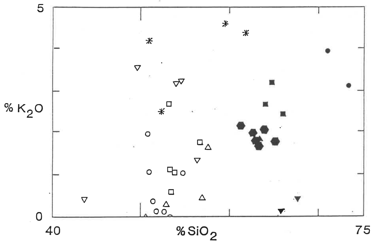
Figure 5.11: Diagramme \text{K}_2\text{O} vs \text{SiO}_2 . Légende en page 68
