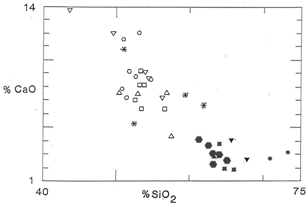
Figure 5.9: Diagramme CaO vs SiO 2 . Légende en page 68
