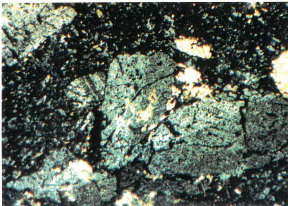
Figure 4.6: Lave mafique gloméroporphyrique. Phénocristaux d'albite fracturés et légèrement carbonatisés baignant dans une matrice de microlites de plagioclases, de chlorite et de clinozoïsité (éch. C860715, 31,25X, L.P.).
