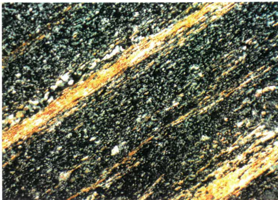
Figure 4.1: Siltstone (unité 2a) composé de quartz microcristallin, de chlorite, de carbonates et de séricite concentrée en lamines (éch. C860666, 31,25X, L.P.).
