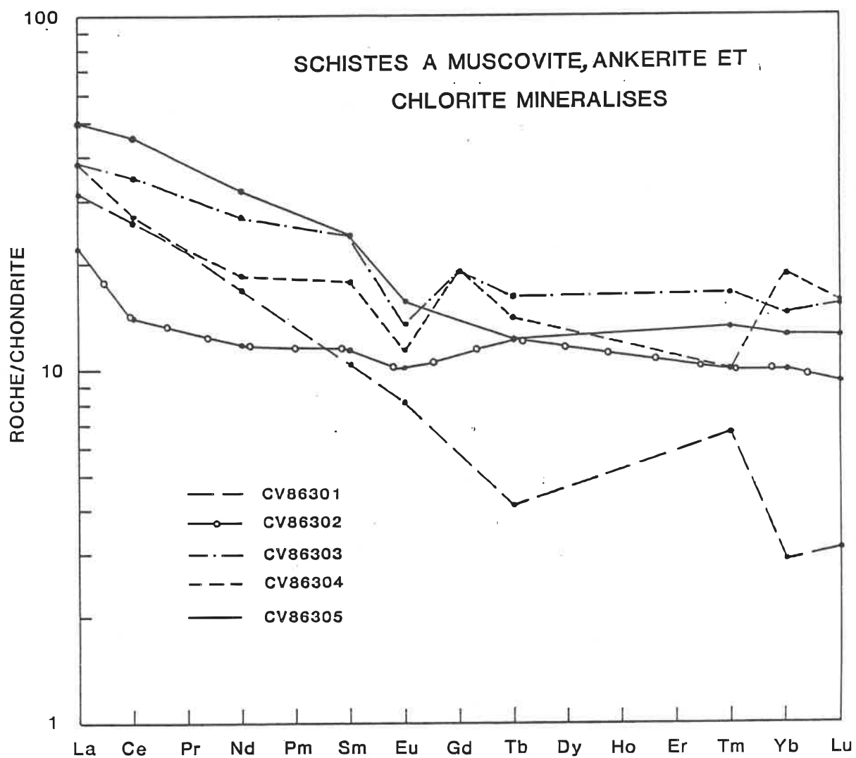
Figure 5.14: Patrons de terres rares des schistes à muscovite, ankérite et chlorite minéralisés (unité 3)
