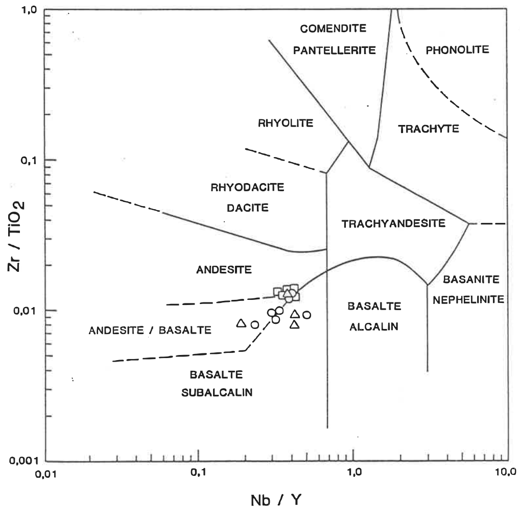
Figure 5.3: Diagramme Zr/TiO_2 vs Nb/Y . D'après Winchester et Floyd, 1977. Légende en page 68
