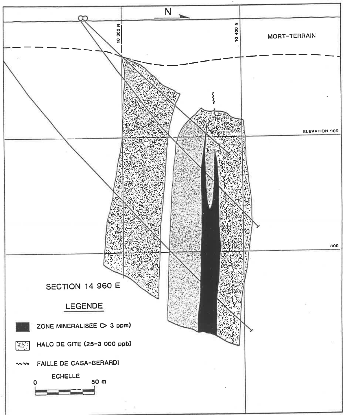
Figure 6.6: Contour des halos de gîte et de la zone minéralisée de la section 14 960 E
