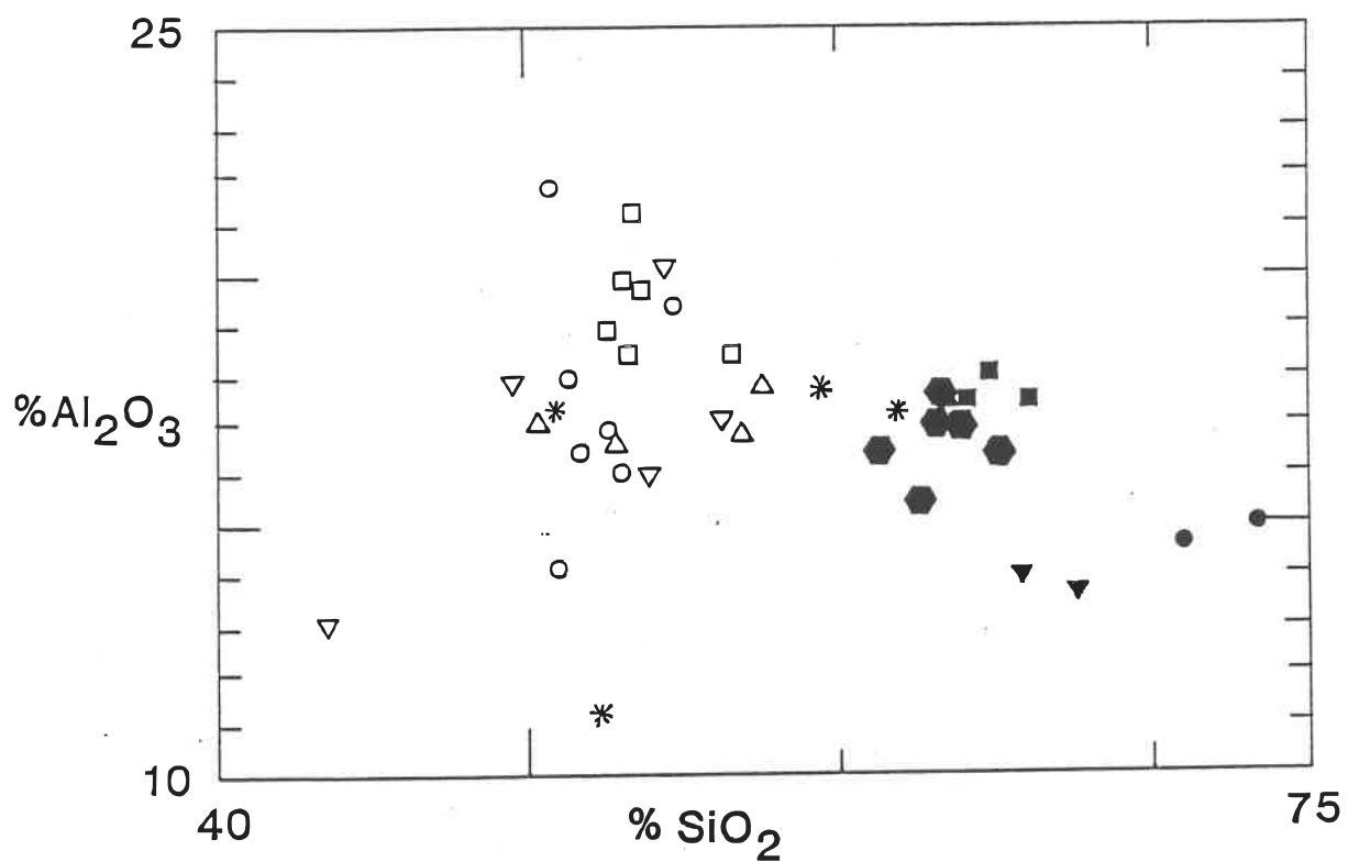
Figure 5.5: Diagramme \text{Al}_2\text{O}_3 vs \text{SiO}_2 . Légende en page 68
