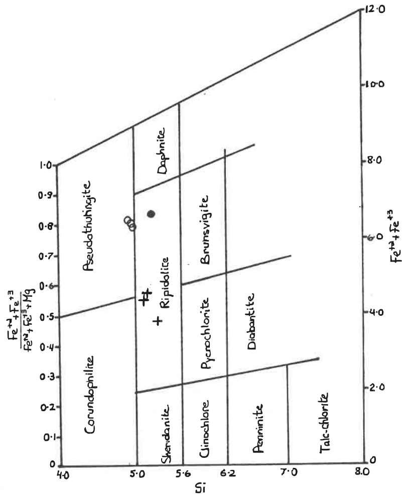
Figure 4.B: Classification des chlorites d'après Hey (1954)
