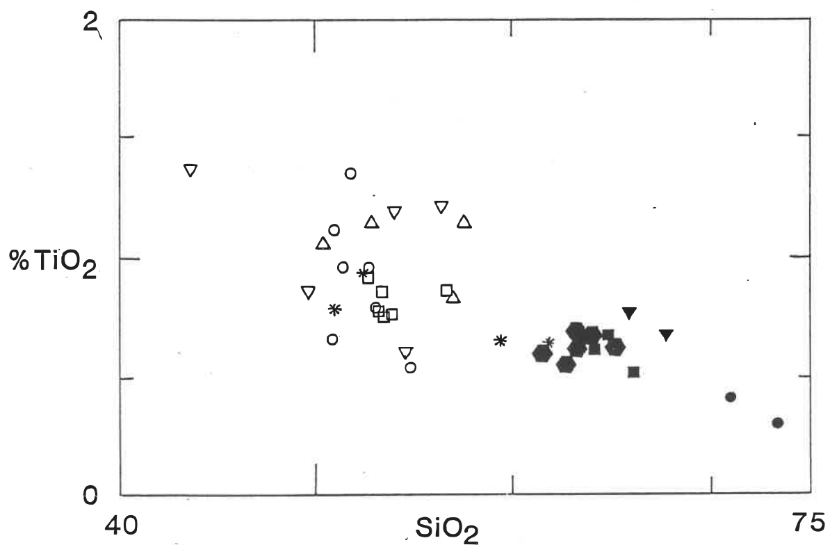
Figure 5.4: Diagramme \text{TiO}_2 vs \text{SiO}_2 . Légende en page 68
