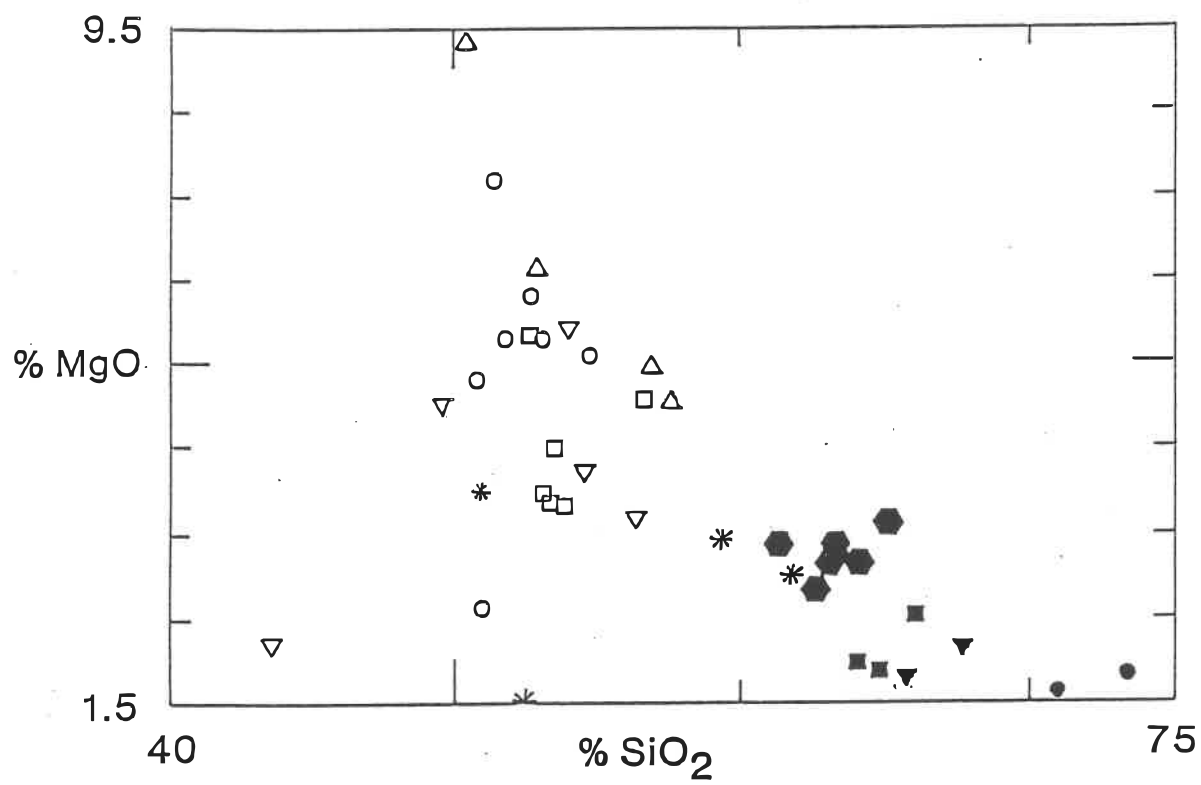
Figure 5.7: Diagramme \text{MgO} vs \text{SiO}_2 . Légende en page 68
