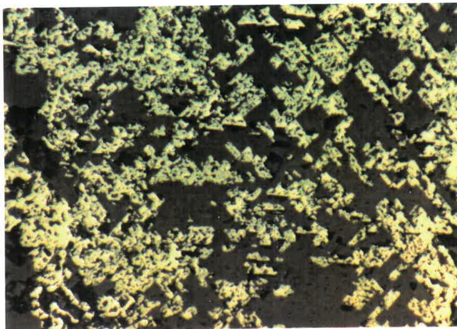
Figure 4.11: Cas extrême de pyrite à texture graphique avec le quartz (éch. CB60880, 100X, L.R.).
