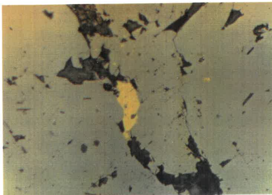
Figure 4.12: Grain d'or (0,05 mm de long) coincé entre un cristal de pyrite au centre et un cristal d'arsénopyrite à gauche. Remarquez la multitude de gouttelettes d'or ( d < 0,0025 mm) incluses dans la pyrite et les trois inclusions d'or dans les cristaux d'arsénopyrite à gauche et à droite (éch. CB60886, 500X, L.R.).
