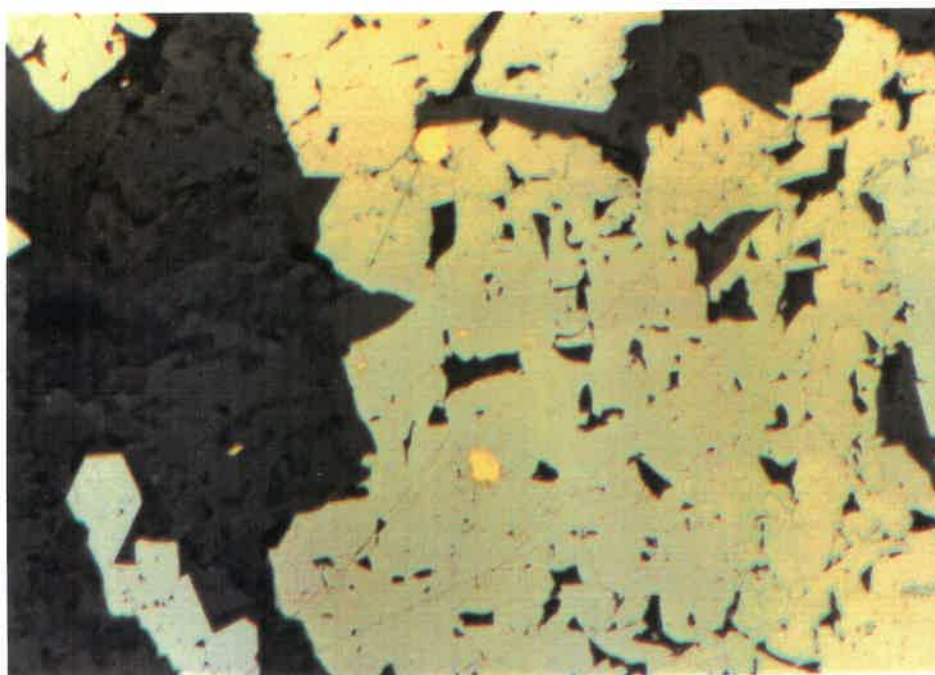
Figure 4.13: Gouttelettes d'or ( d_{\max} = 0,03 \text{ mm} ) incluses dans un cristal de pyrite poecilitique (inclusions de gangue). Remarquez le minuscule grain d'or libre dans le quartz à gauche (éch. C860895, 200X, L.R.).
