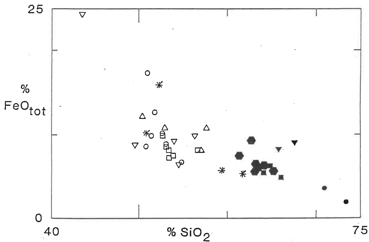
Figure 5.6: Diagramme \text{FeO}_{\text{tot}} vs \text{SiO}_2 . Légende en page 68
