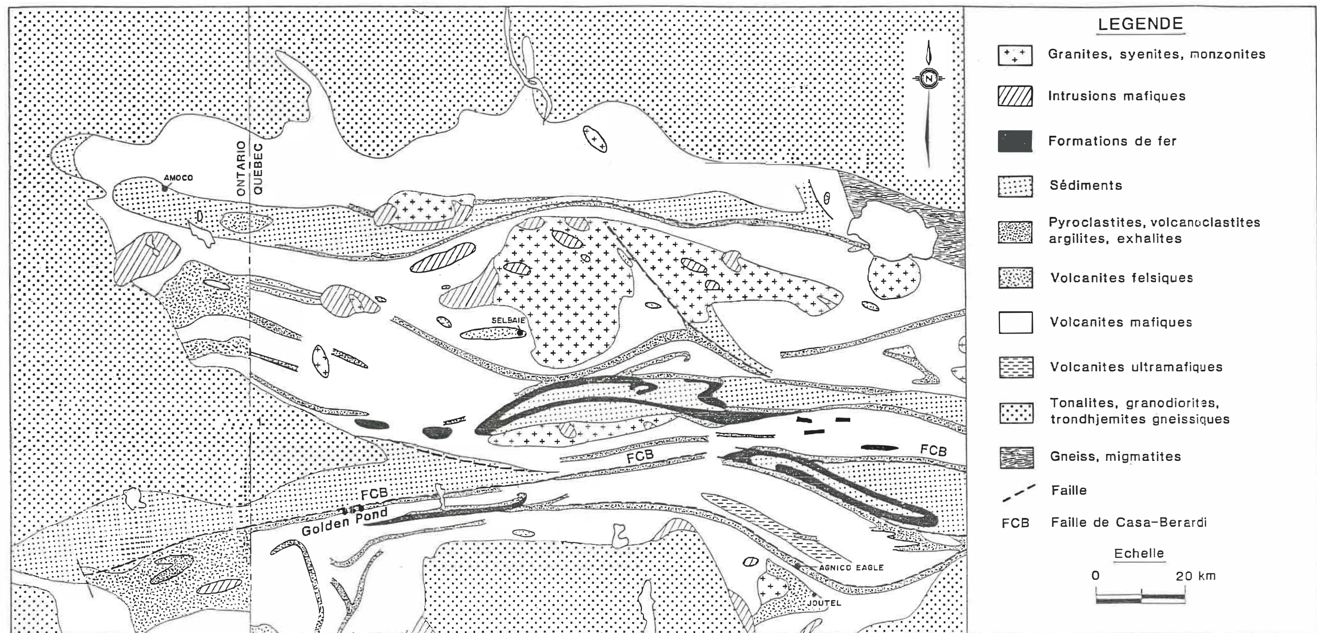
Figure 2.3 – Géologie du sillon Harricana-Turgeon. (Modifié d'après Lacroix, 1986b)
