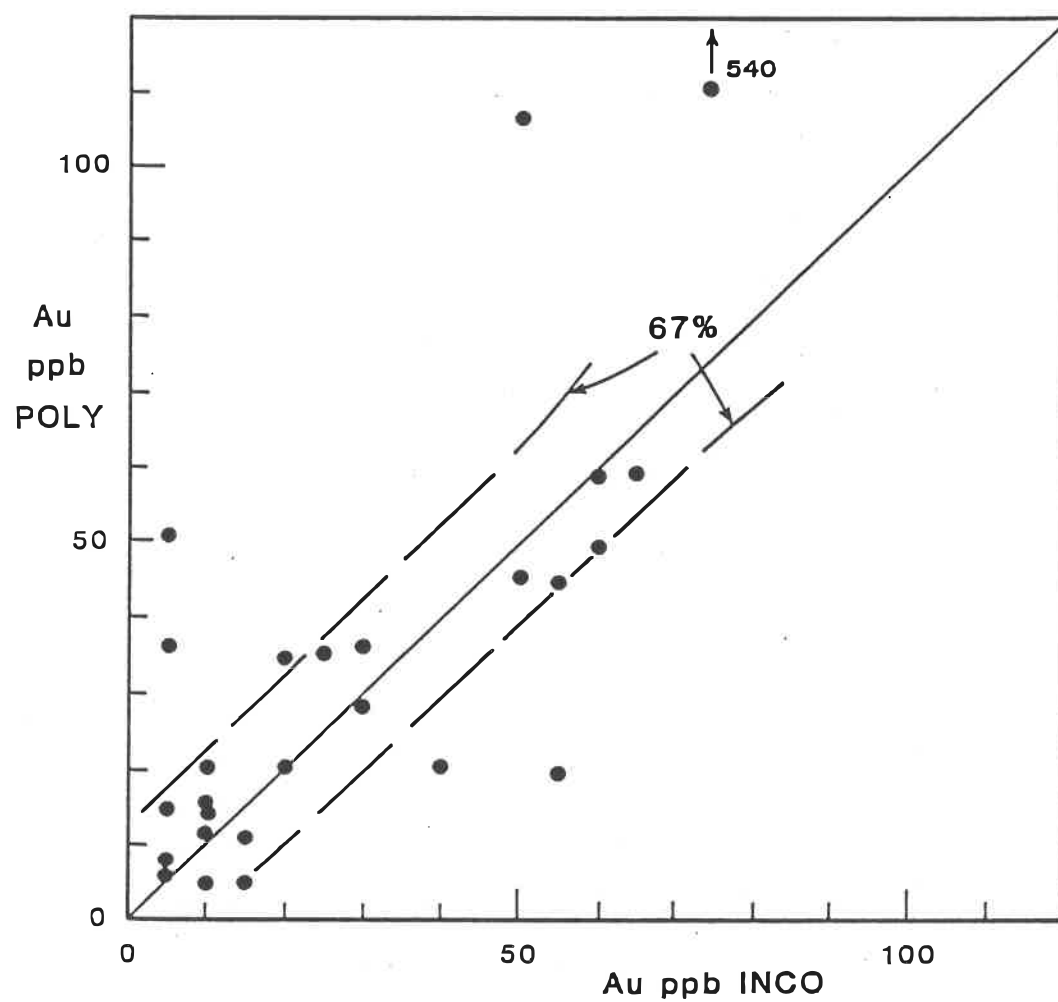
Figure 6.1: Comparaison des résultats analytiques obtenus par absorption atomique (INCO) et par AANI (Poly). (ppb Au)
