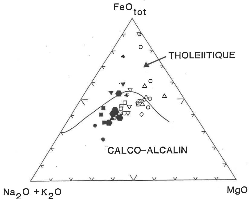
Figure 5.2: Diagramme AFM. Division d'après Irvine et Baragar, 1971. Légende en page 68
