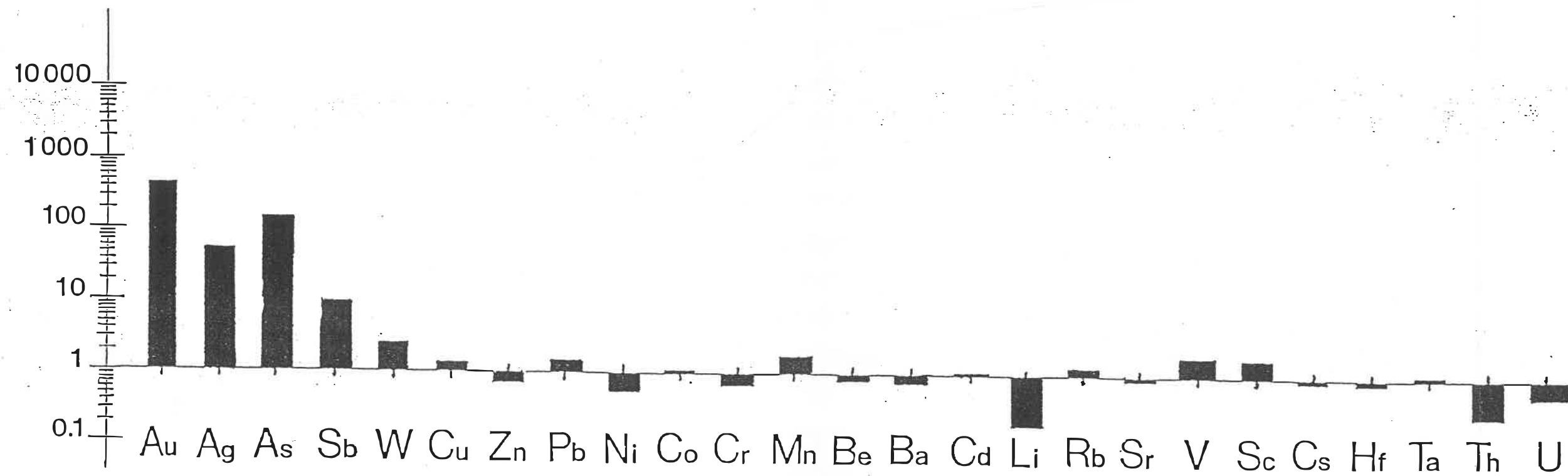
Figure 5.12: Diagramme d'enrichissement et de perte relatifs des éléments traces. Les enrichissements et les pertes sont définis d'après la moyenne obtenue pour les schistes minéralisés divisée par la moyenne obtenue pour les siltstones non minéralisés (unité 3)
