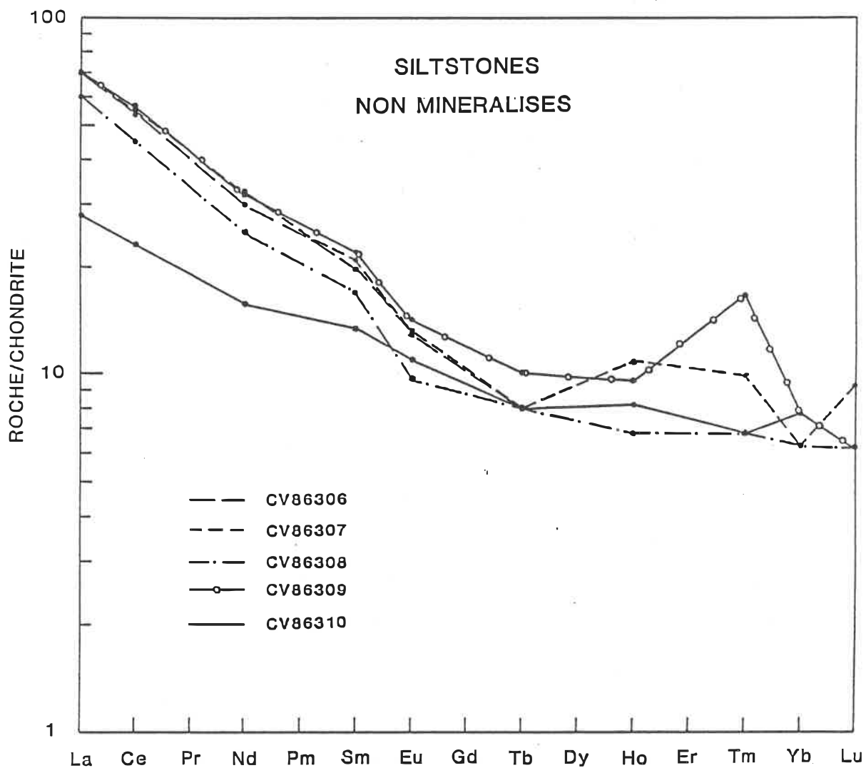
Figure 5.13: Patrons de terres rares des siltstones non minéralisés (unité 3)
