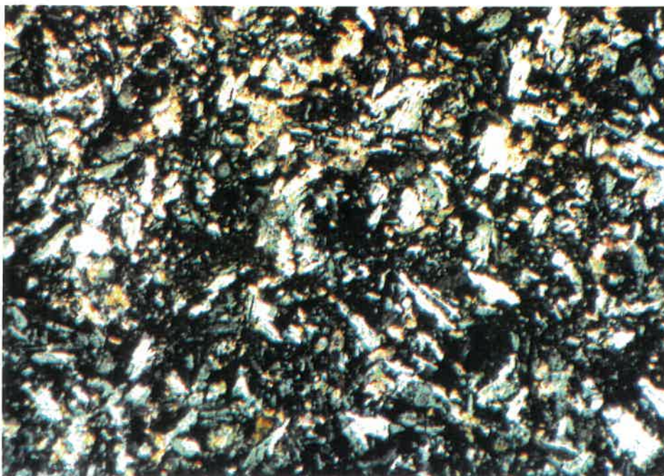
Figure 4.4: Lave mafique aphanitique à texture interstitielle. Interstices entre les microlites de plagioclases remplis de chlorite, de clinozoïsité, de carbonates, de rutile et de leucoxène (éch. C860705, 31,25X, L.P.).
