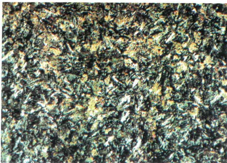
Figure 4.5: Lave mafique aphanitique altérée. Cristallisation de carbonates et de séricite aux dépens des plagioclases, de la chlorite et de la clinozoïsité (éch. C860723, 31,25X, L.P.).
