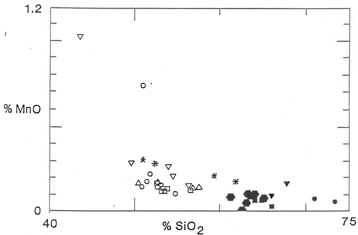
Figure 5.8: Diagramme MnO vs SiO 2 . Légende en page 68
