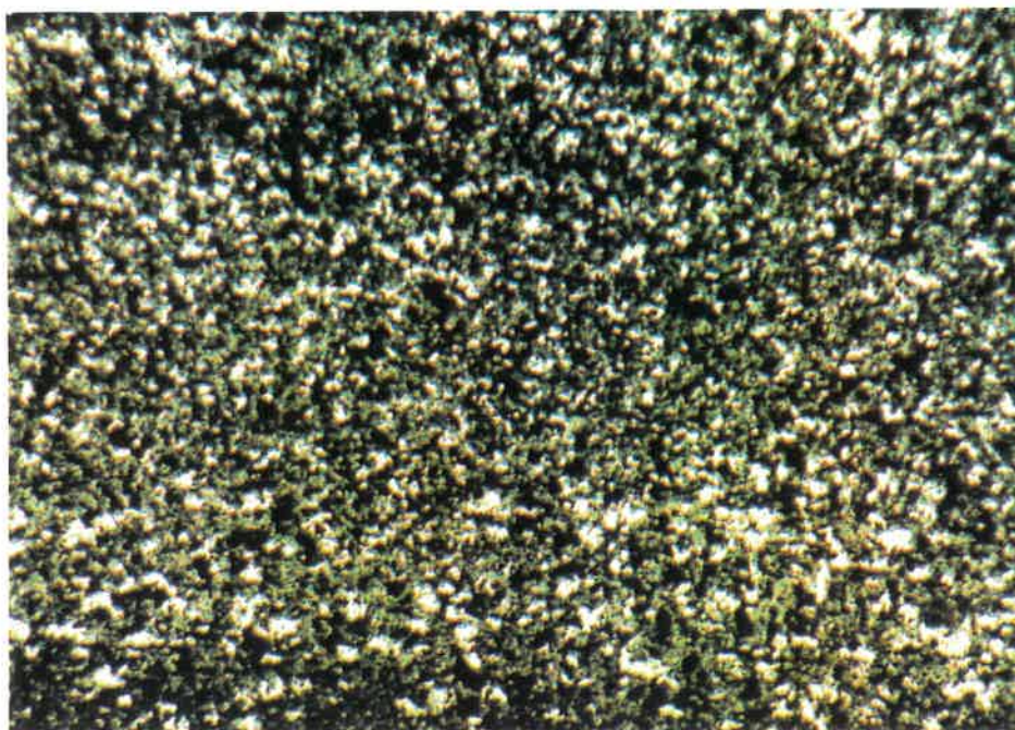
Figure 4.2: Formation de fer au faciès oxyde (unité 2b). Détail d'un lit riche en chlorite et en magnétite (éch. C860664, 31,25X, L.N.).
