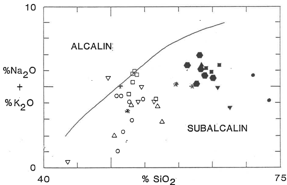
Figure 5.1: Diagramme \text{Na}_2\text{O} + \text{K}_2\text{O} vs \text{SiO}_2 . Division d'après MacDonald et Katsura, 1964. Légende en page 68
