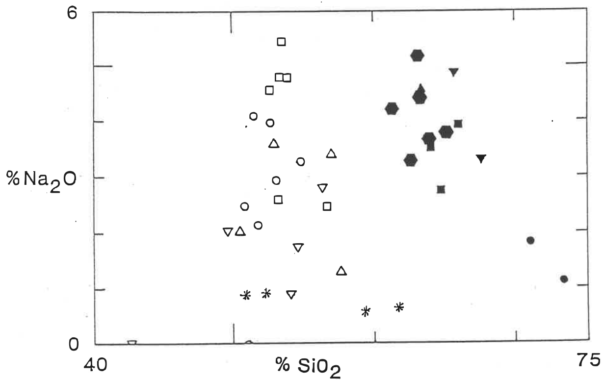
Figure 5.10: Diagramme \text{Na}_2\text{O} vs \text{SiO}_2 . Légende en page 68
