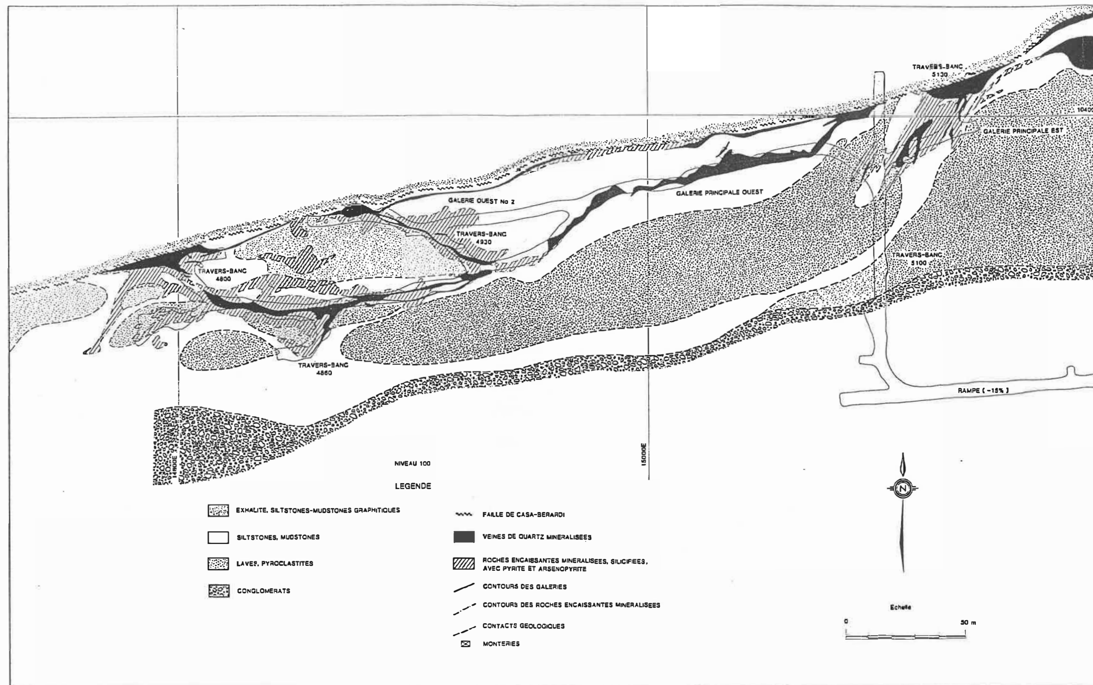
Figure 3.2 - Géologie du niveau 100 à Golden Pond East. (Modifié d'après Sauerbrey, 1986)
