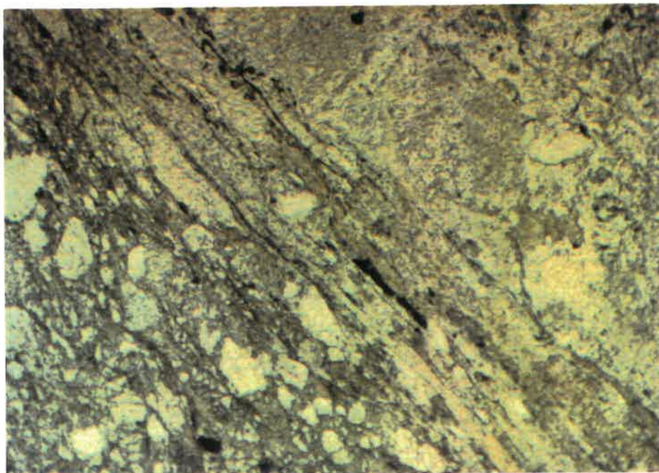
Figure 4.3a: Conglomérat polymicte lithique. Contact micacé entre un fragment de siltstone gréseux (à gauche) et un fragment de lave gloméroporphyrique à droite (éch. CB606B1, 31,25X, L.N.).
