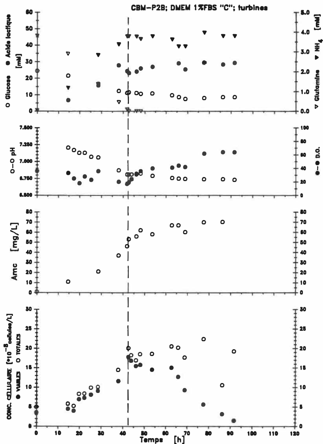
Figure 19 Courbe de croissance des cellules CBM-P2-B cultivées en curvée dans le Celligen dans le DMEM supplémenté de 1% FBS, agitation fournie par l'agitateur à hélices. Expérience C
