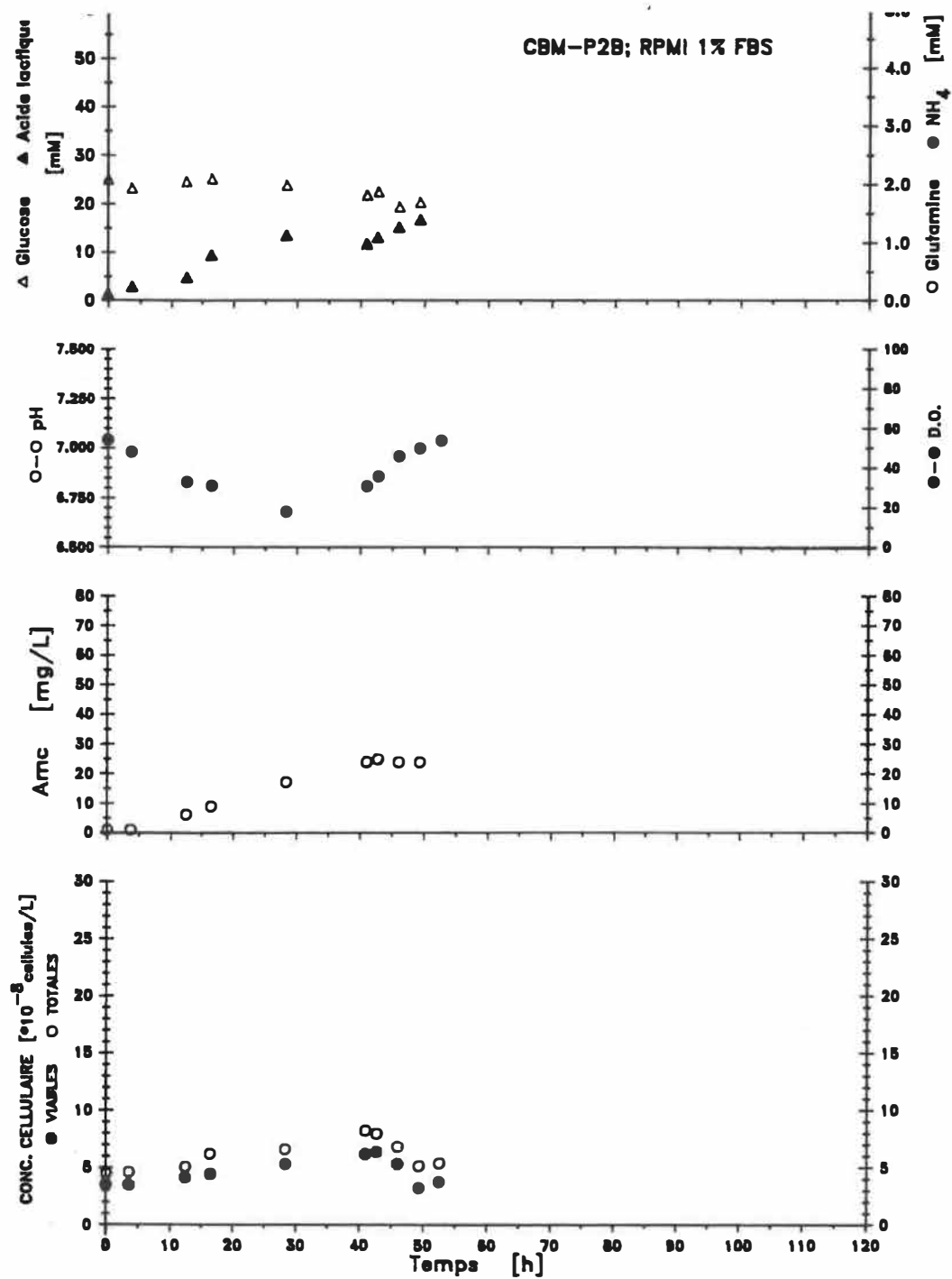
Figure A7 Evolution des concentrations d'une culture de cellules de la lignée CBM-P2-B, dans le Celligen, dans le RPMI 1640 + 1%FBS
