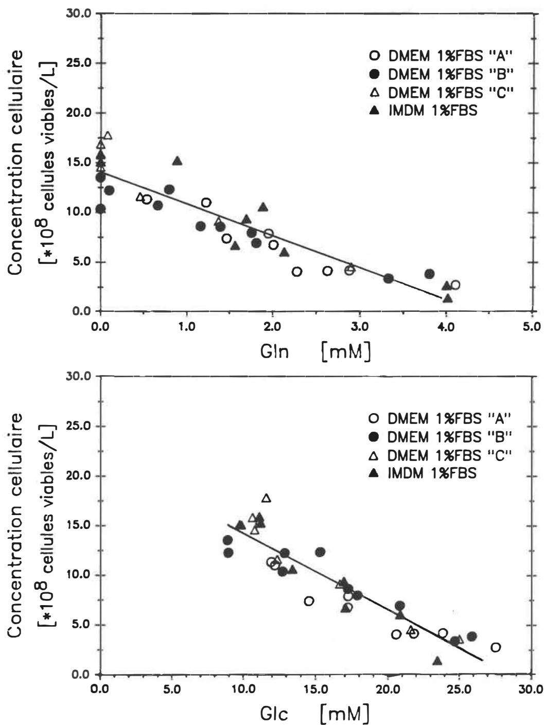
Figure 28 Evaluation des coefficients de rendement Y_{XV/Gln} et Y_{XV/Glc}
