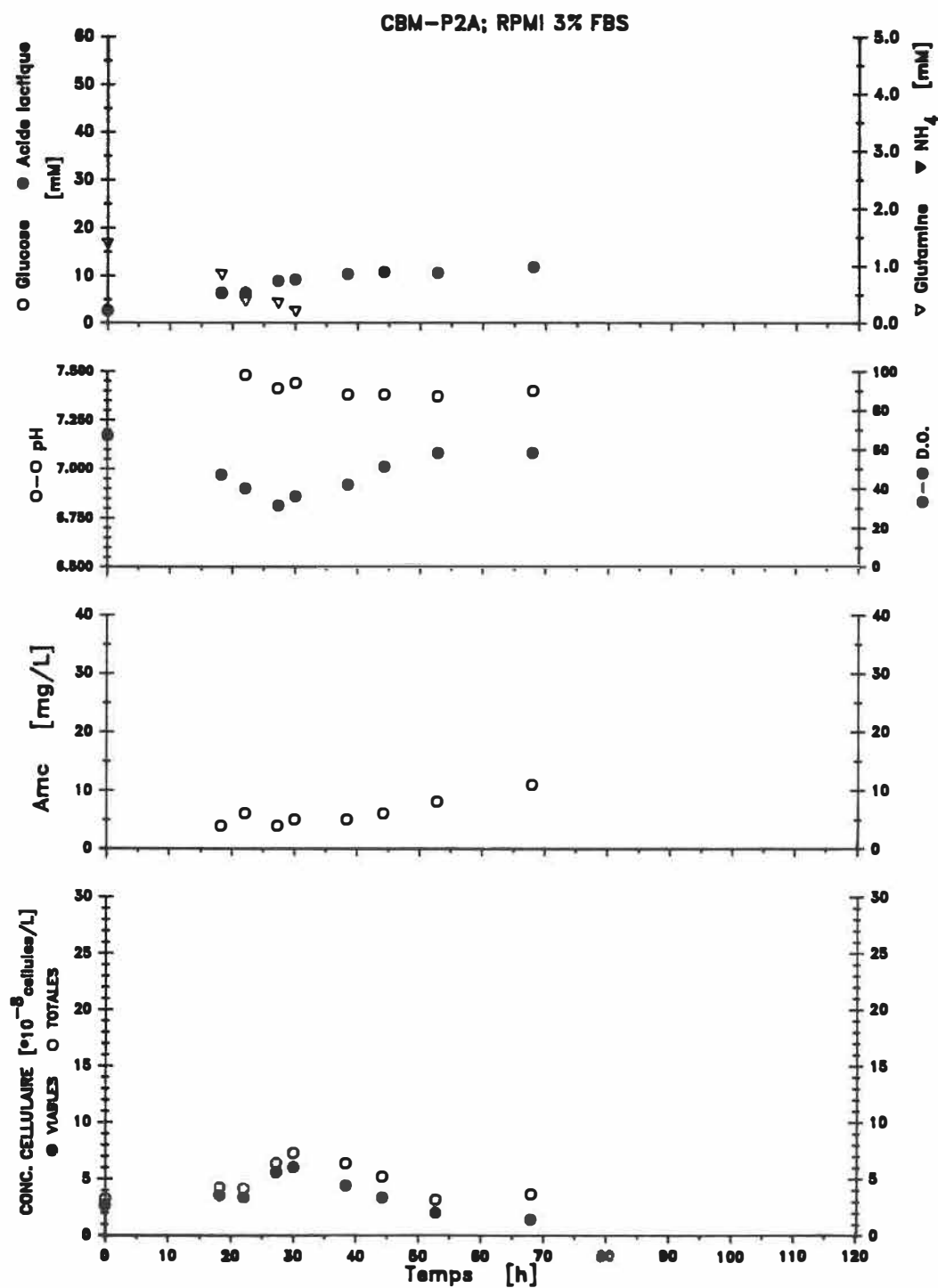
Figure 15 Courbe de croissance des cellules CBM-P2-A cultivées en cuvette dans le Celligen dans le RPMI 1640 supplémenté de 3% FBS
