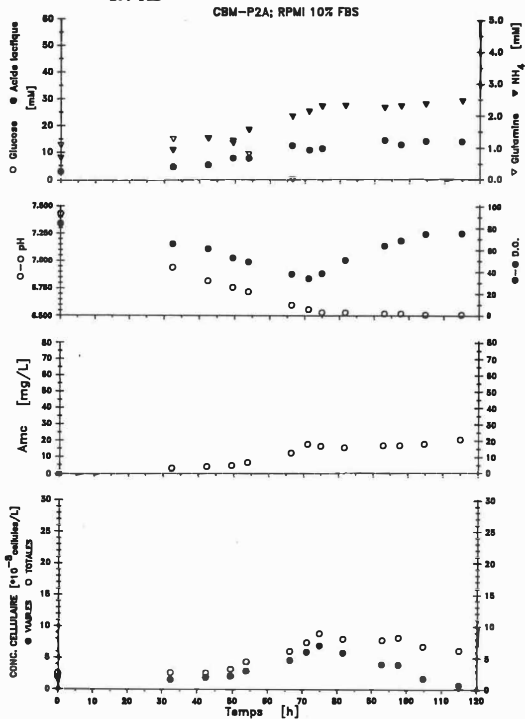
Figure 22 Courbe de croissance des cellules CBM-P2-A cultivées en curvée dans le Celligen dans le RPMI 1640 supplémenté de 10% FBS
