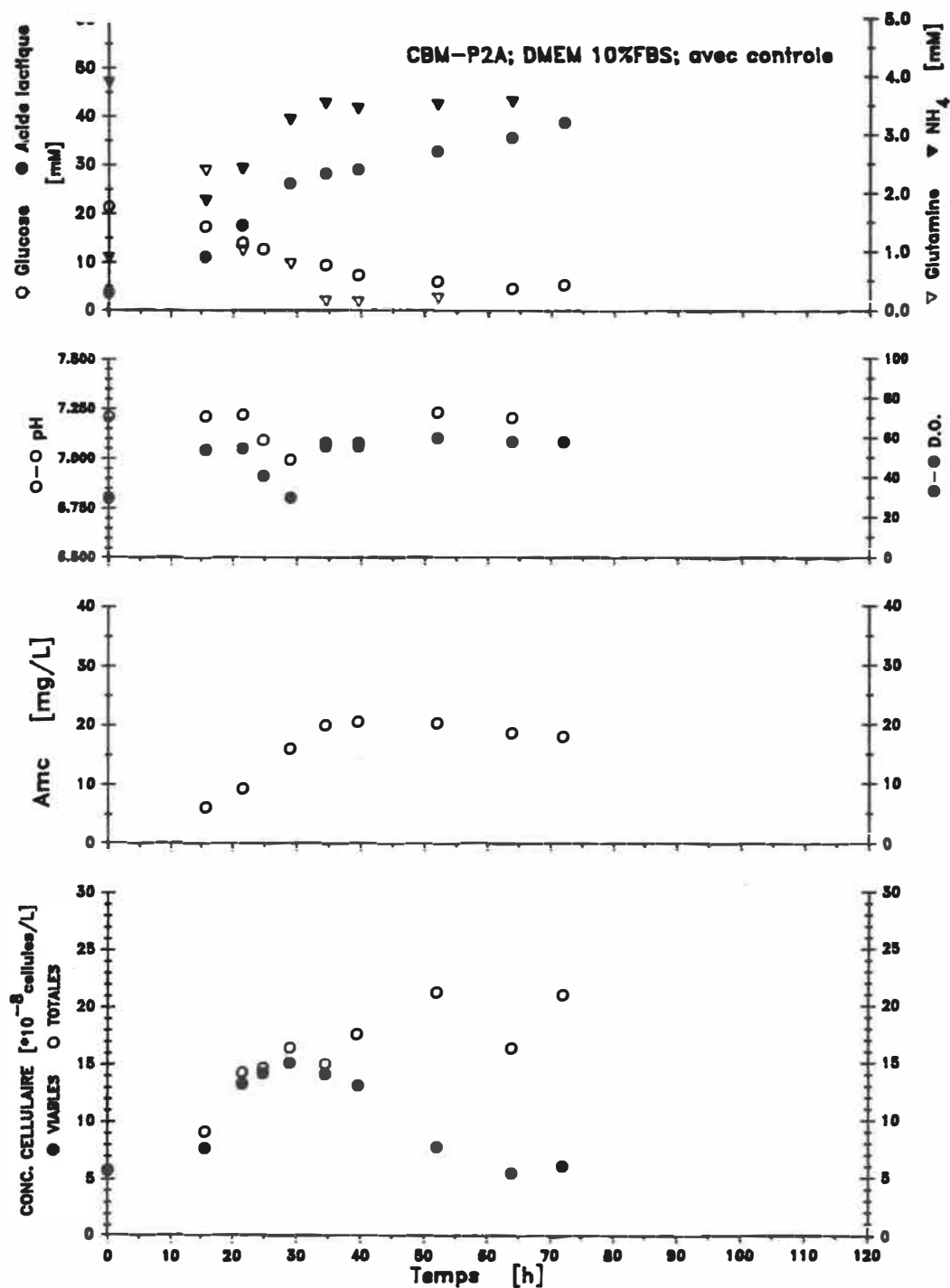
Figure A6 Evolution des concentrations d'une culture de cellules de la lignée CBM-P2-A, dans le Celligen, dans le DMEM + 10%FBS, avec contrôle de pH à 7,2 et de la DO à 60%
