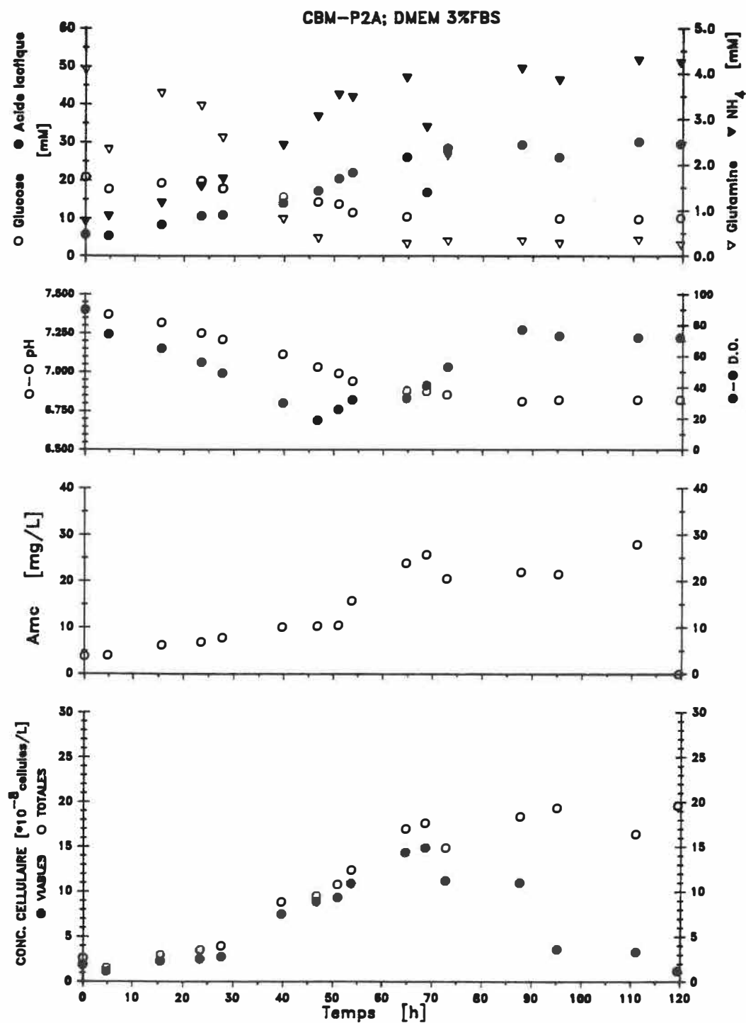
Figure 16 Courbe de croissance des cellules CBM-P2-A cultivées en cuvée dans le Celligen dans le DMEM supplémenté de 3% FBS
