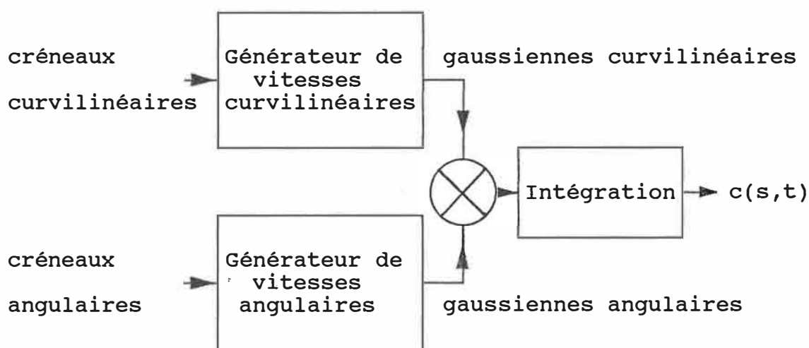
figure II.6 : Générateur de signatures
