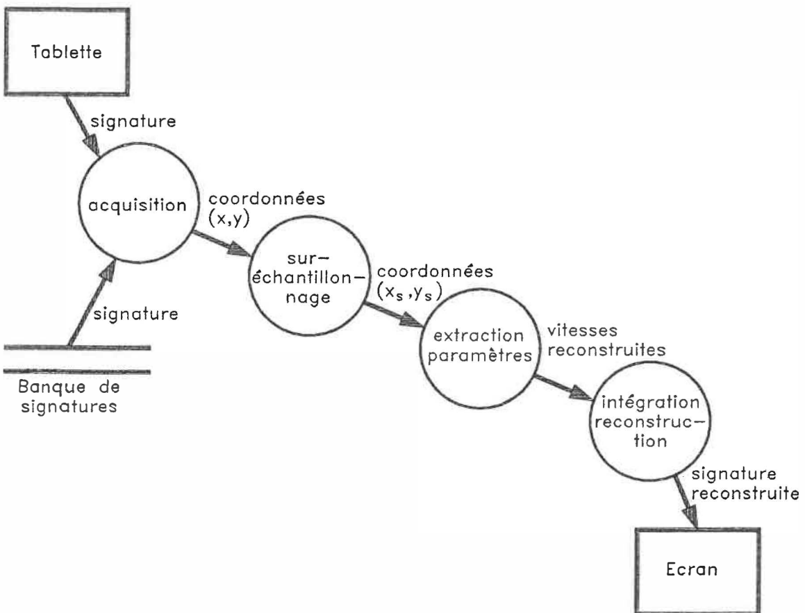
Figure IV.1 Diagramme de flux de données
