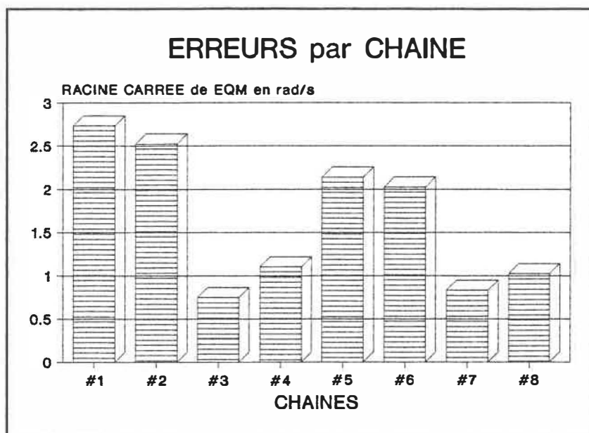
Figure VIII.9 Erreurs sur les vitesses angulaires.
