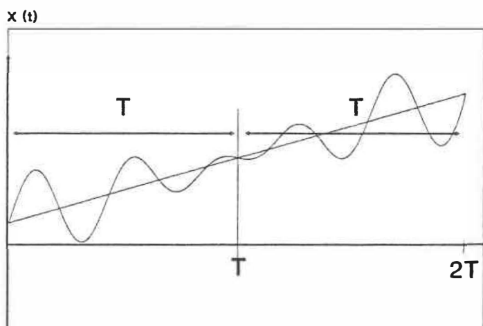
Figure V.2 Miroir inverse pour x(t) ou y(t)
