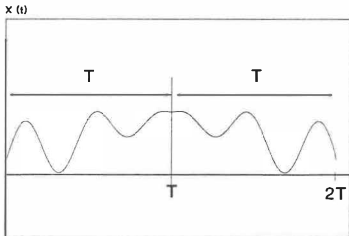
Figure V.1 Miroir du signal x(t) ou y(t)
