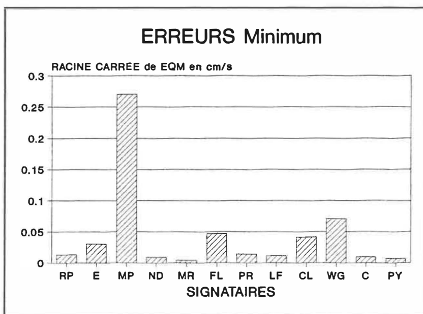
Figure VIII.13 Erreurs minimum sur la vitesse curvilinéaire
