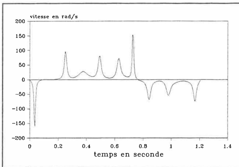
Figure VIII.7 Vitesse angulaire originale
