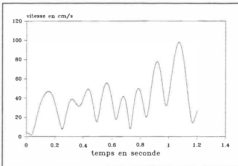
Figure VIII.4 Vitesse curvilinéaire originale
