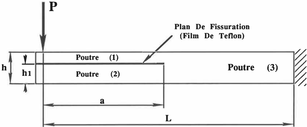
Figure A.1: Division de l'échantillon encastré en trois parties
