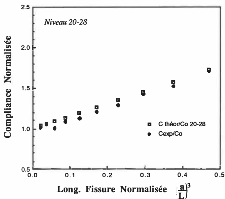
Figures C.3: Compliances théoriques et expérimentales du niveau 20/28
