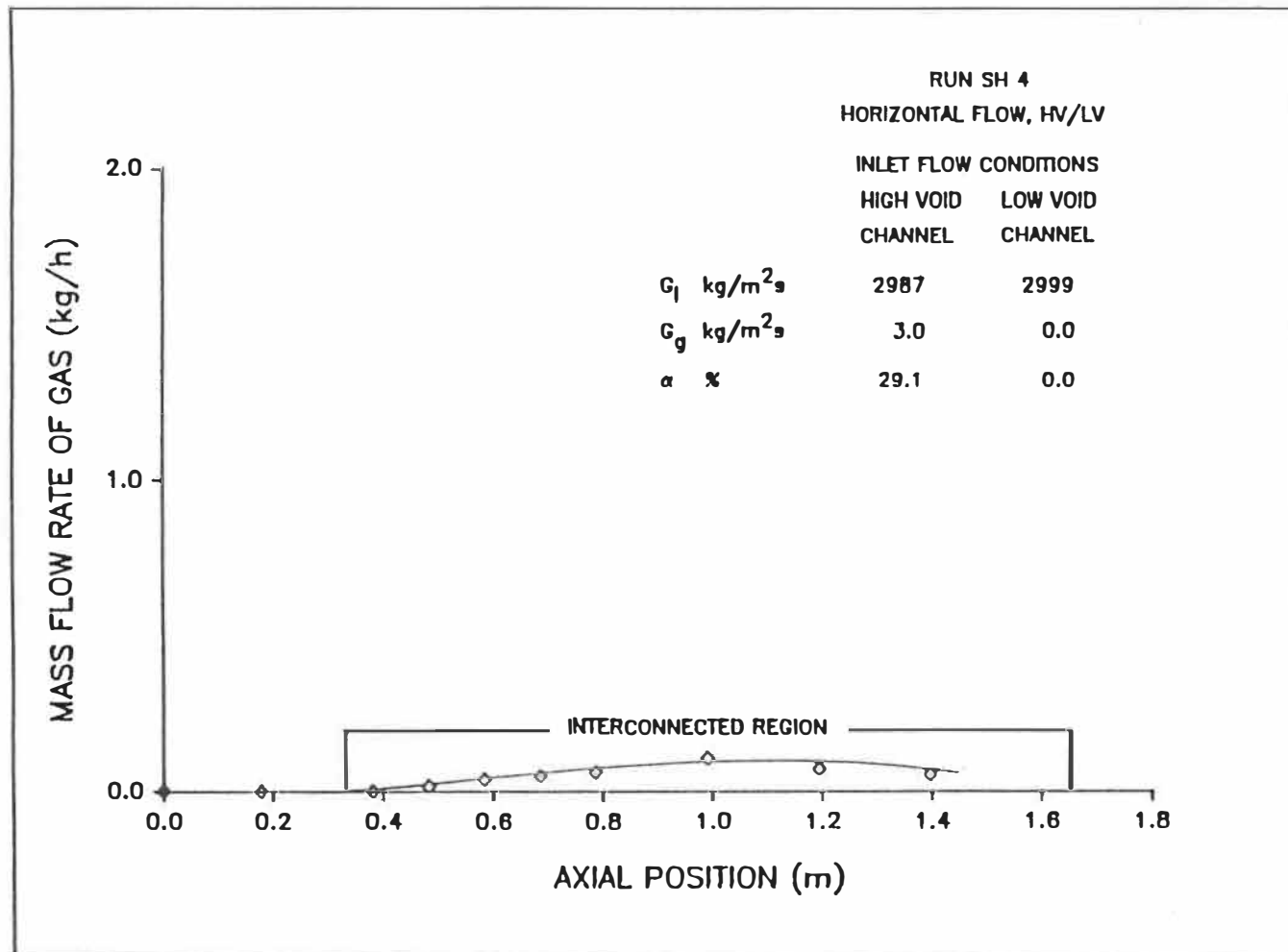
Figure 5.4c: Distribution axiale du débit massique du gaz.
