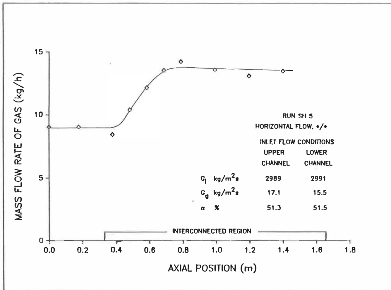
Figure 5.5c: Distribution axiale du débit massique du gaz.
