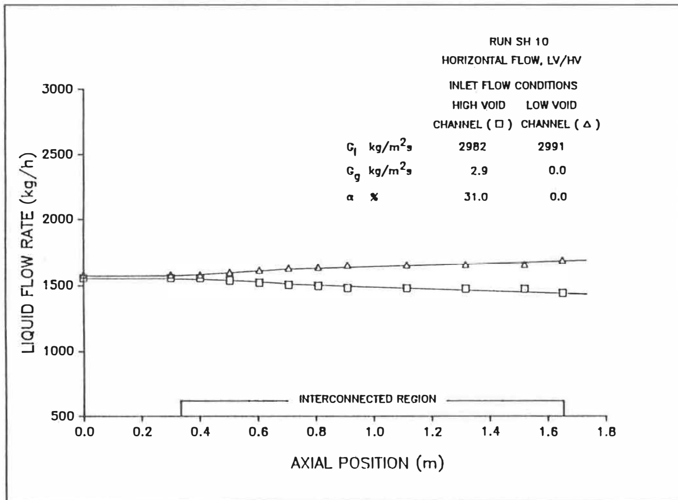
Figure 5.10b: Distribution axiale du débit massique du liquide.
