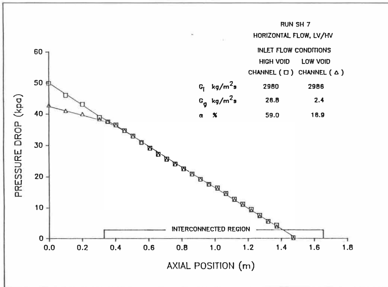
Figure 5.7d: Distribution axiale de la perte de pression axiale.
