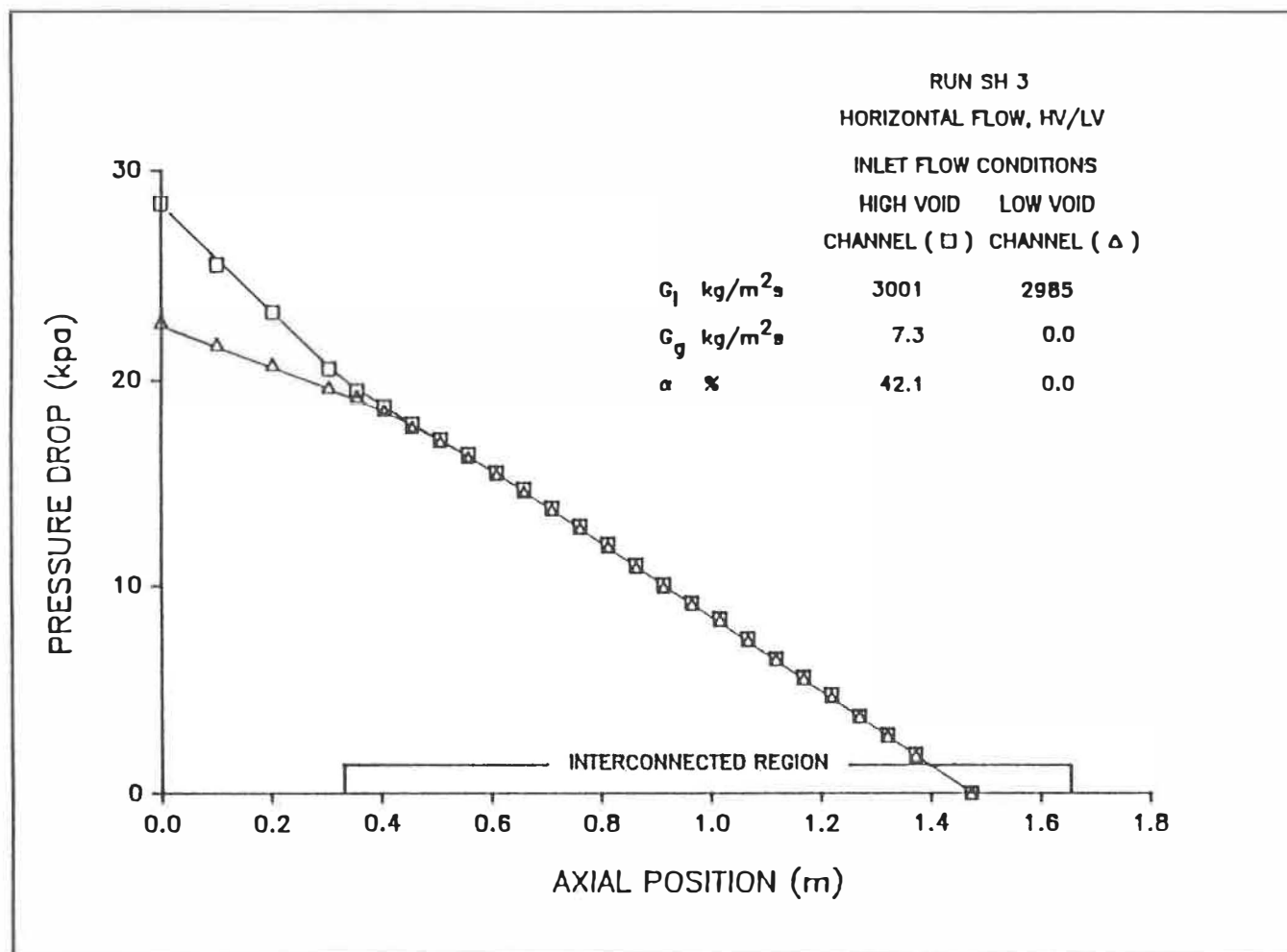
Figure 5.3d: Distribution axiale de la perte de pression axiale.
