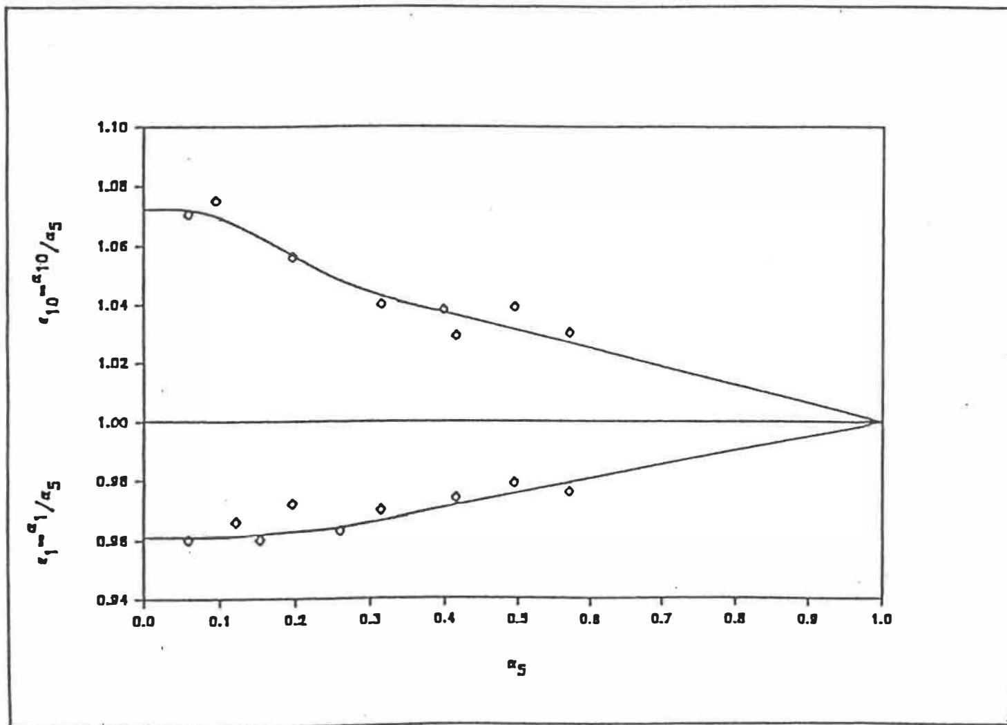
Figure 4.7: Courbe de correction du taux de vide.
