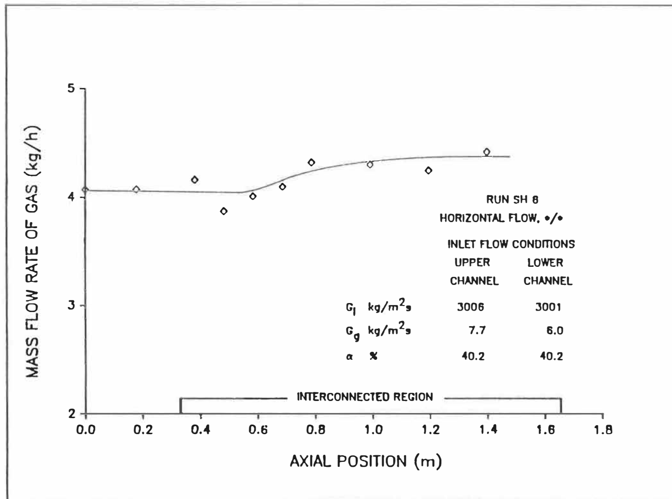
Figure 5.6c: Distribution axiale du débit massique du gaz.
