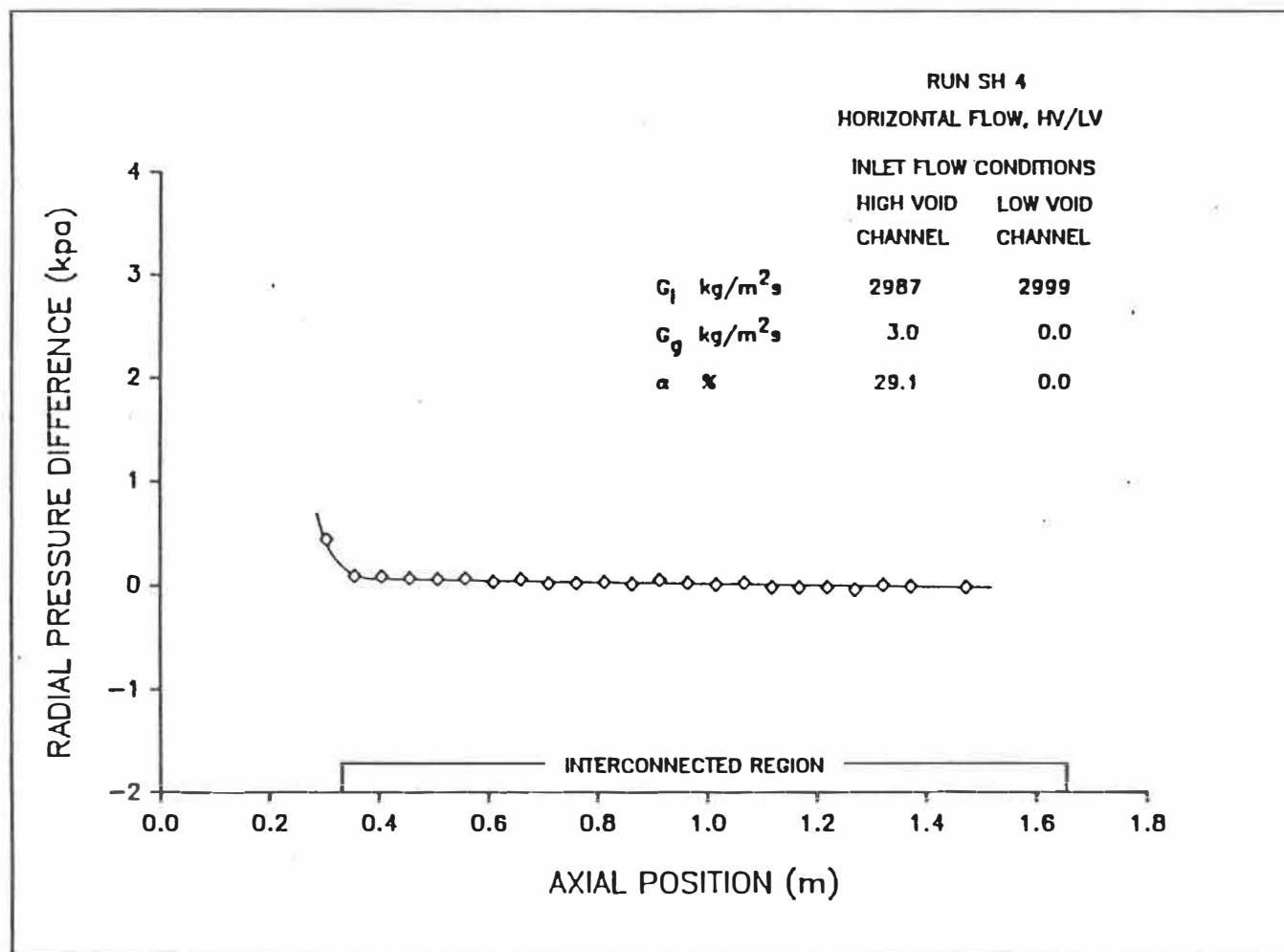
Figure 5.4e: Distribution axiale de la différence des pressions radiales.
