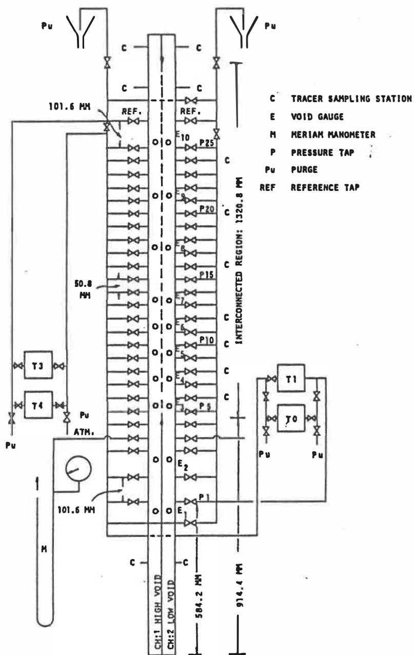
Figure 3.7: Positions des prises de pression, des stations d'échantillonnage du traceur.
