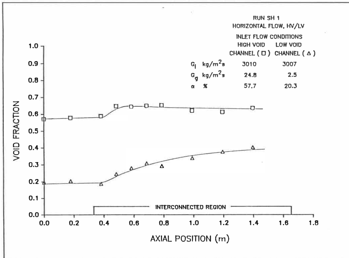
Figure 5.1a: Distribution axiale du taux de vide.
