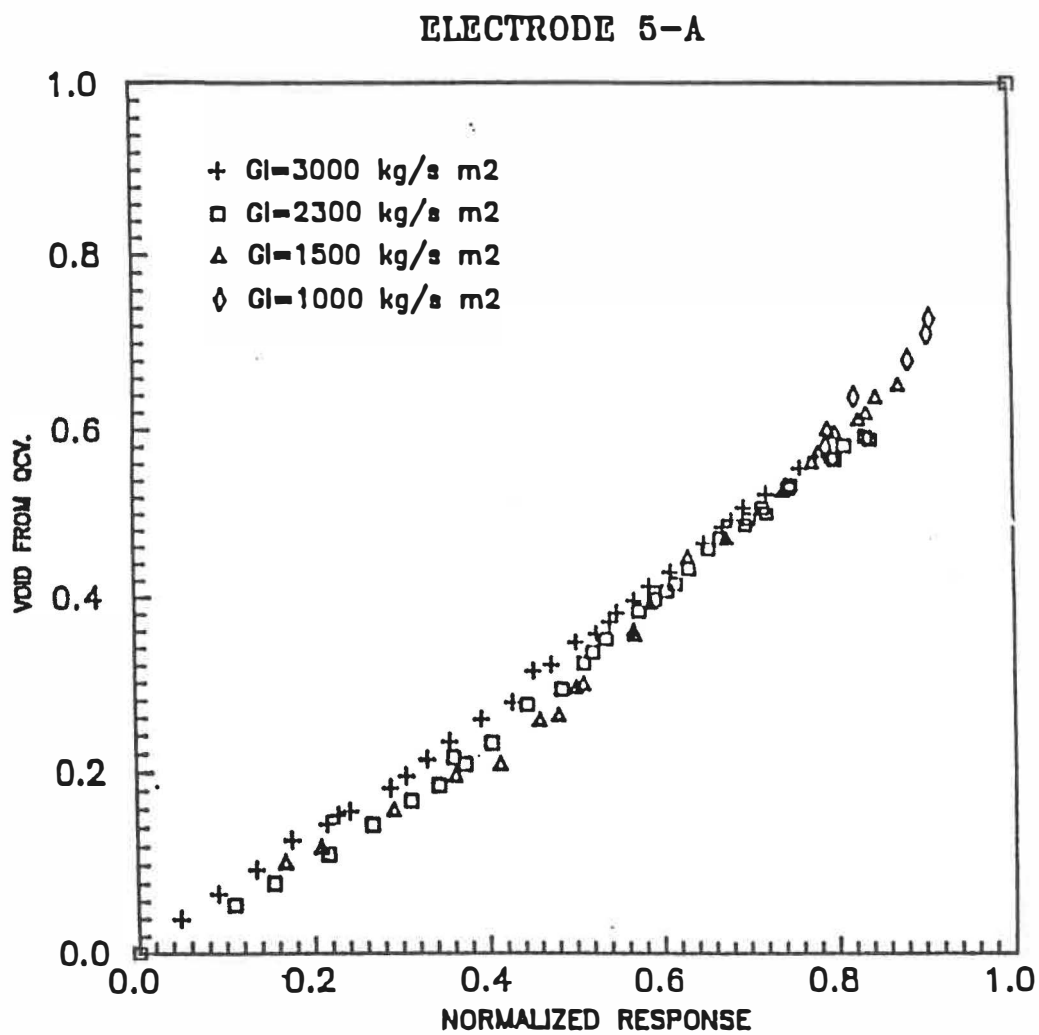
Figure 4.1a: Courbe de calibration de l'électrode (1-5).
