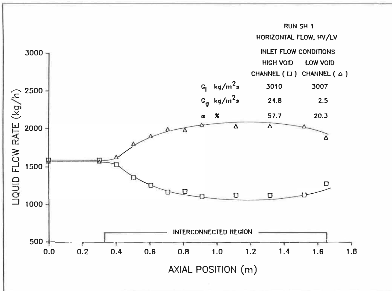
Figure 5.1b: Distribution axiale du débit massique du liquide.
