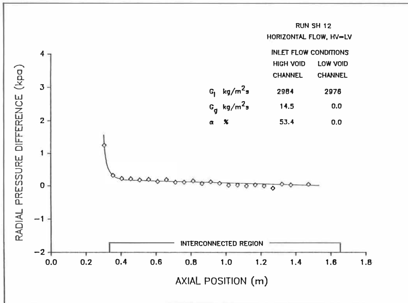
Figure 5.12e: Distribution axiale de la différence des pressions radiales.
