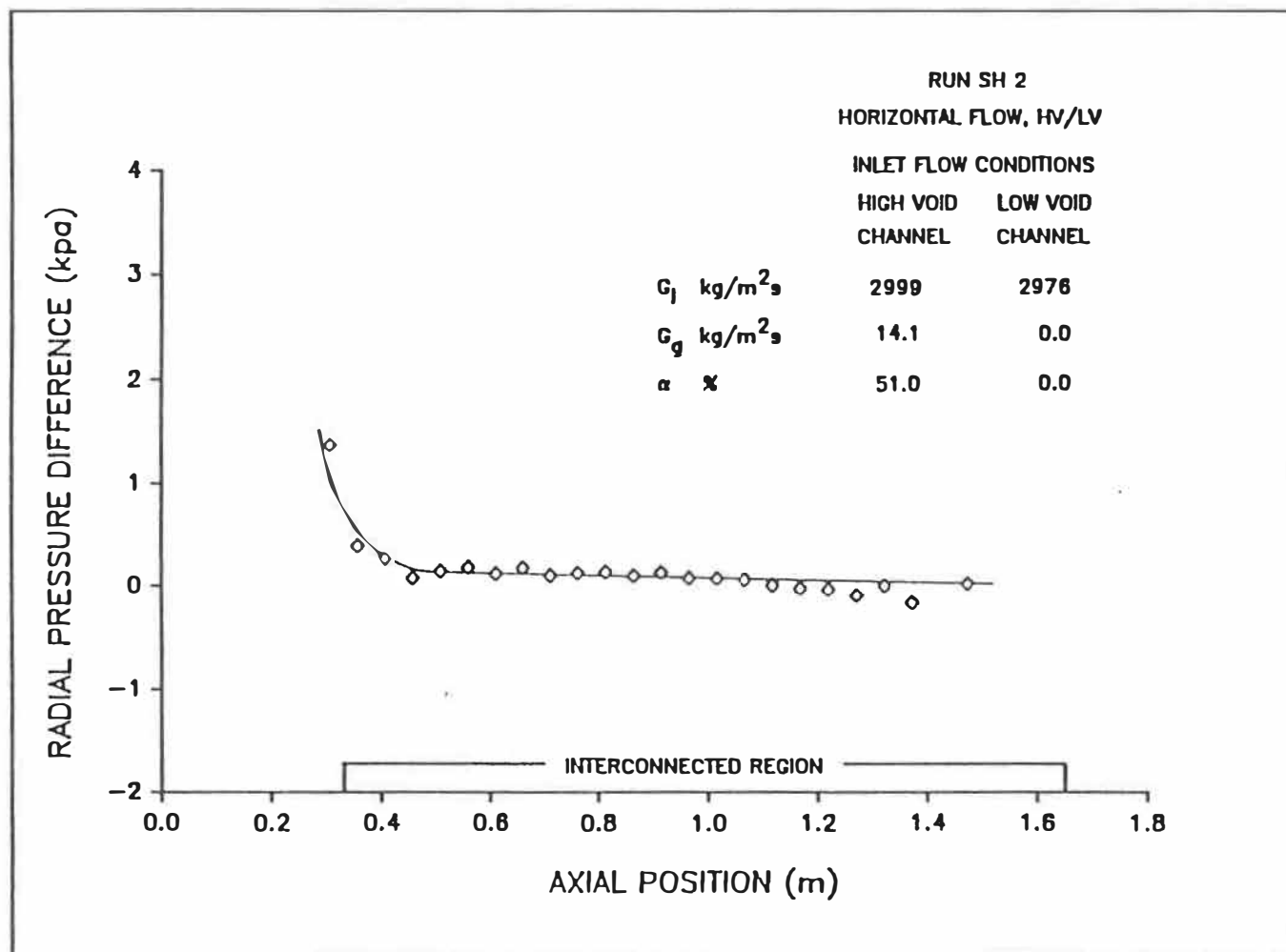
Figure 5.2e: Distribution axiale de la différence des pressions radiales.
