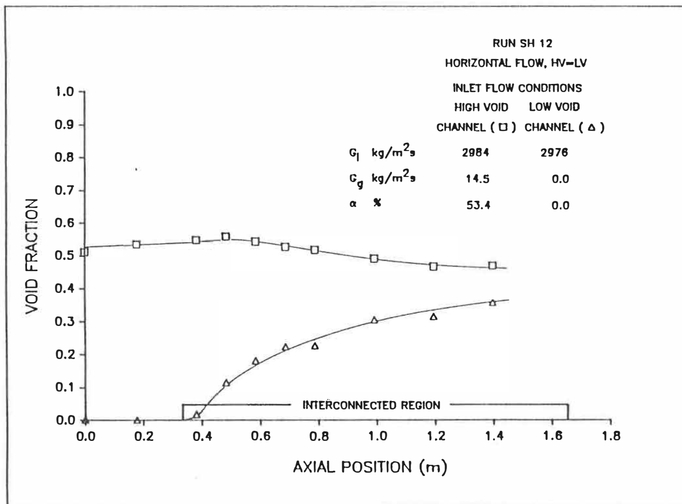
Figure 5.12a: Distribution axiale du taux de vide.
