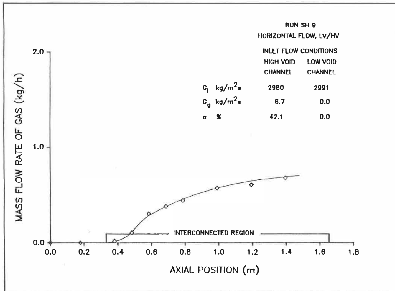
Figure 5.9c: Distribution axiale du débit massique du gaz.
