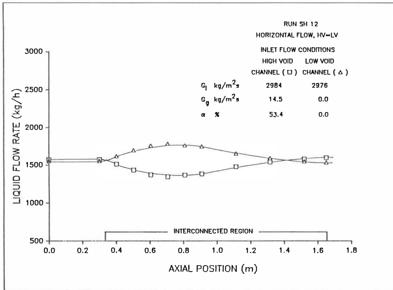
Figure 5.12b: Distribution axiale du débit massique du liquide.
