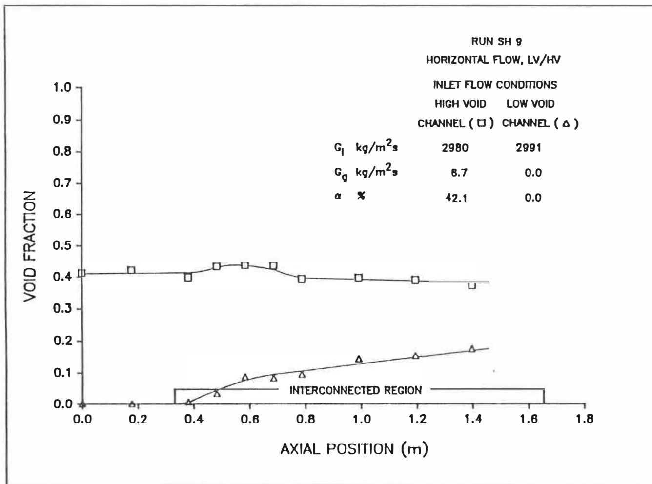
Figure 5.9a: Distribution axiale du taux de vide.
