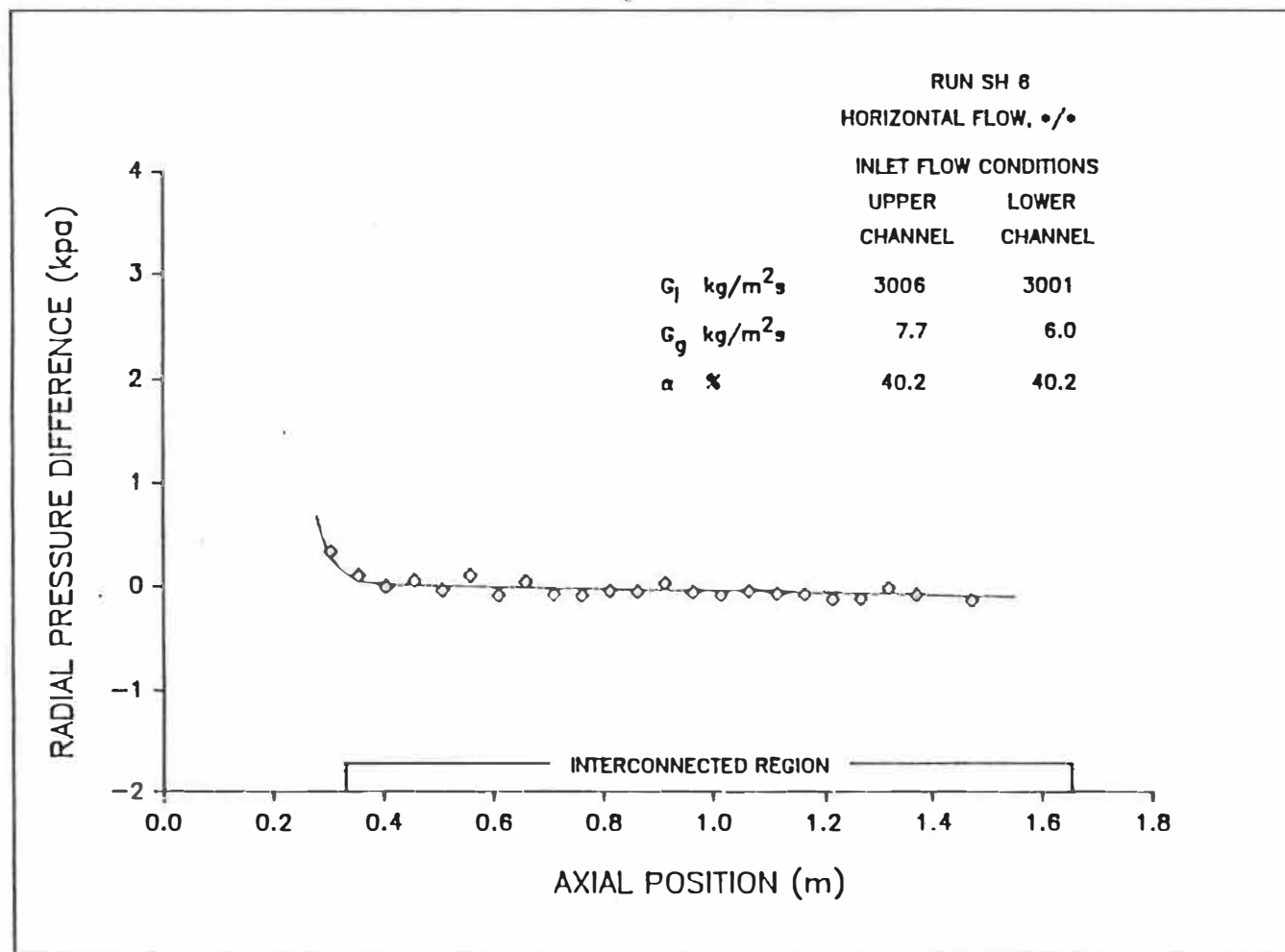
Figure 5.6e: Distribution axiale de la différence des pressions radiales.
