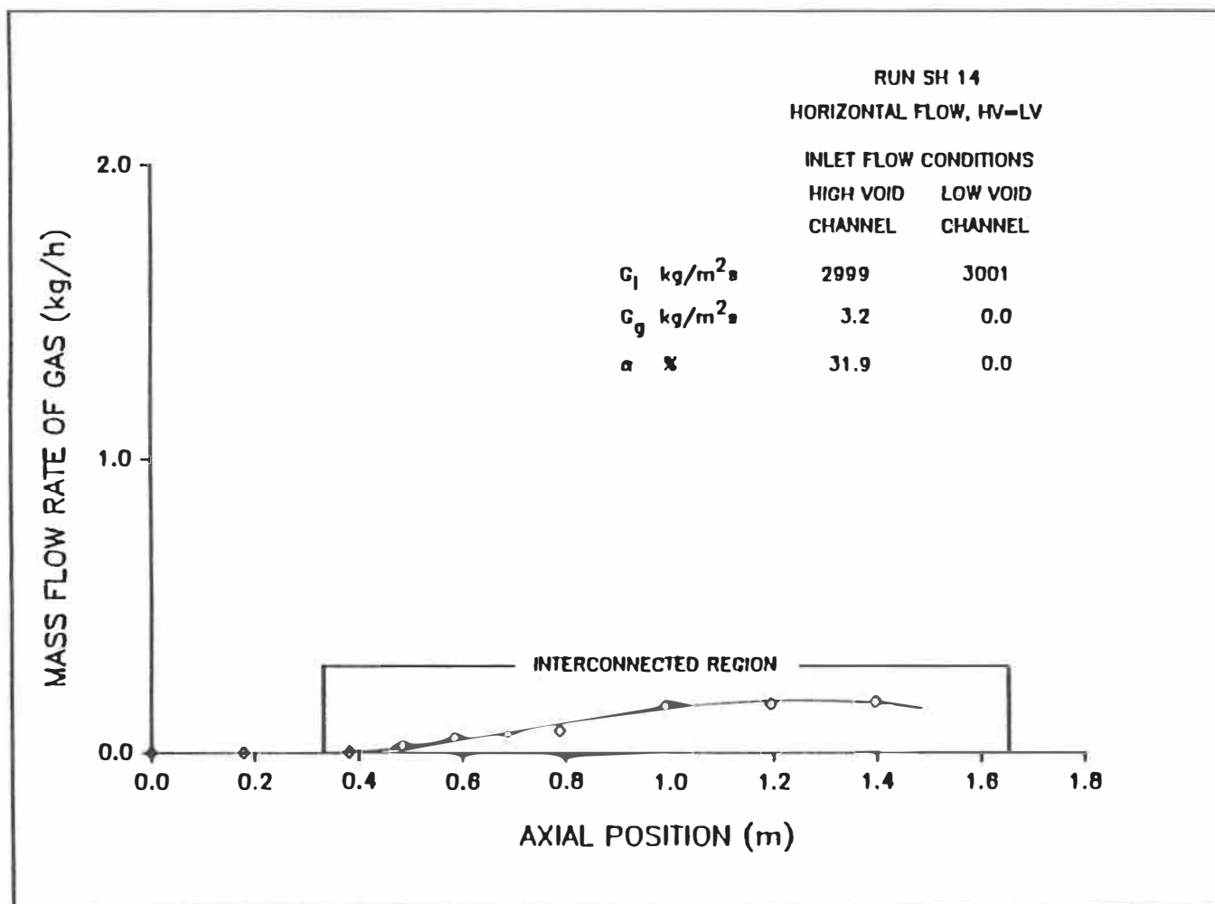
Figure 5.14c: Distribution axiale du débit massique du gaz.
