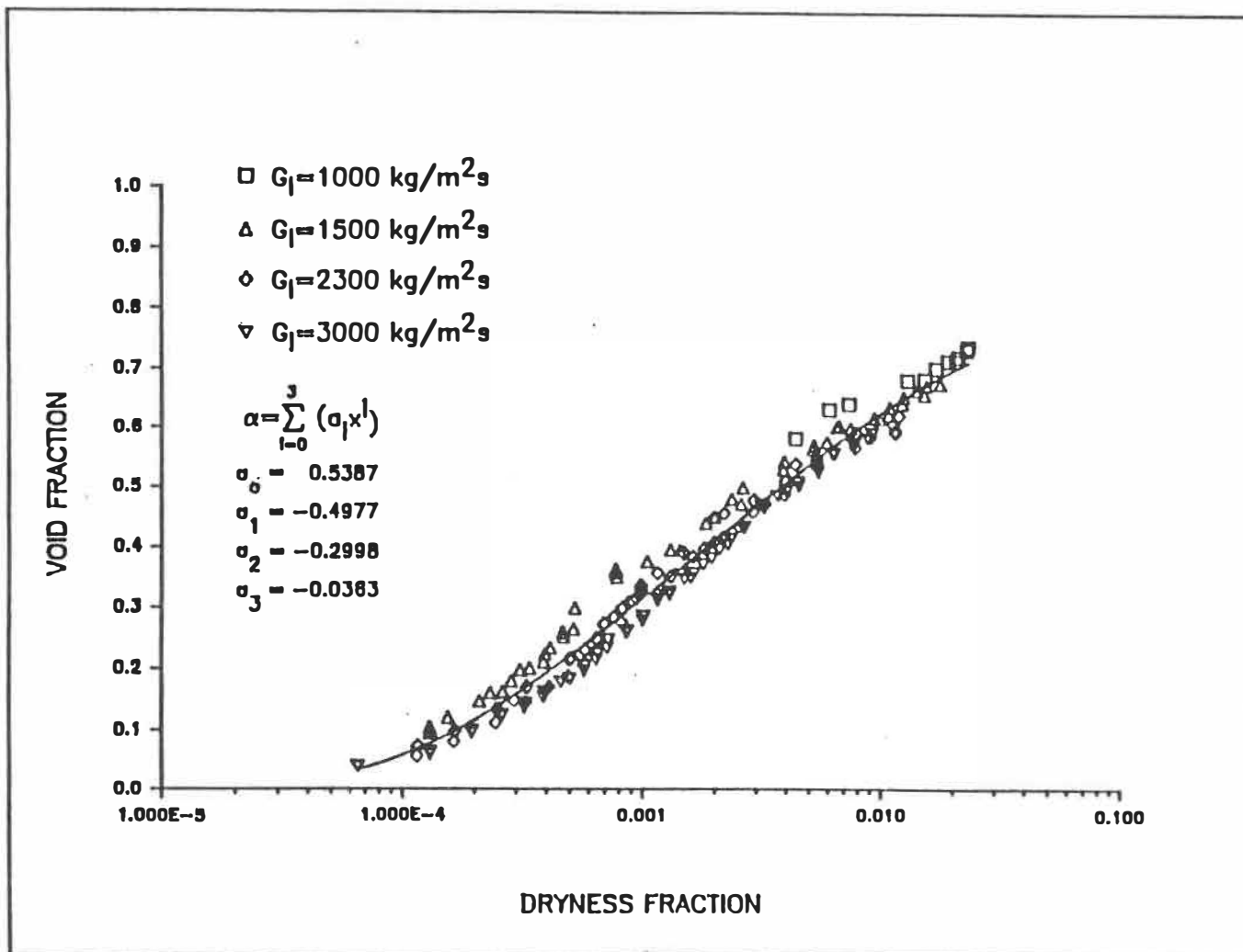
Figure 4.4: Relation entre le taux de vide et le titre de l'écoulement.
