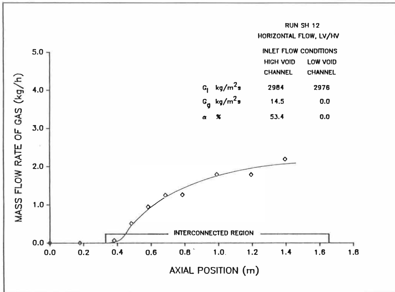
Figure 5.12c: Distribution axiale du débit massique du gaz.
