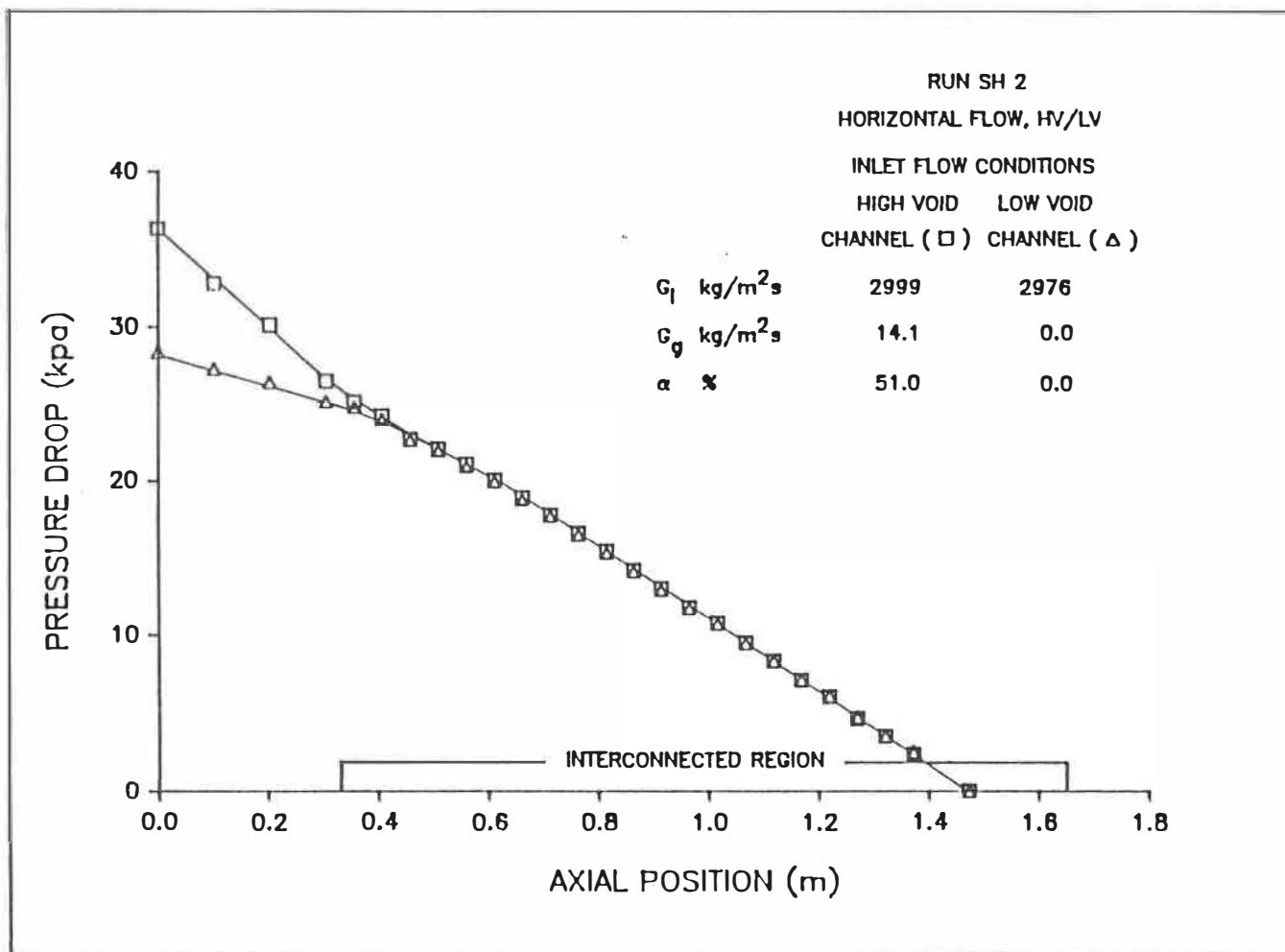
Figure 5.2d: Distribution axiale de la perte de pression axiale.
