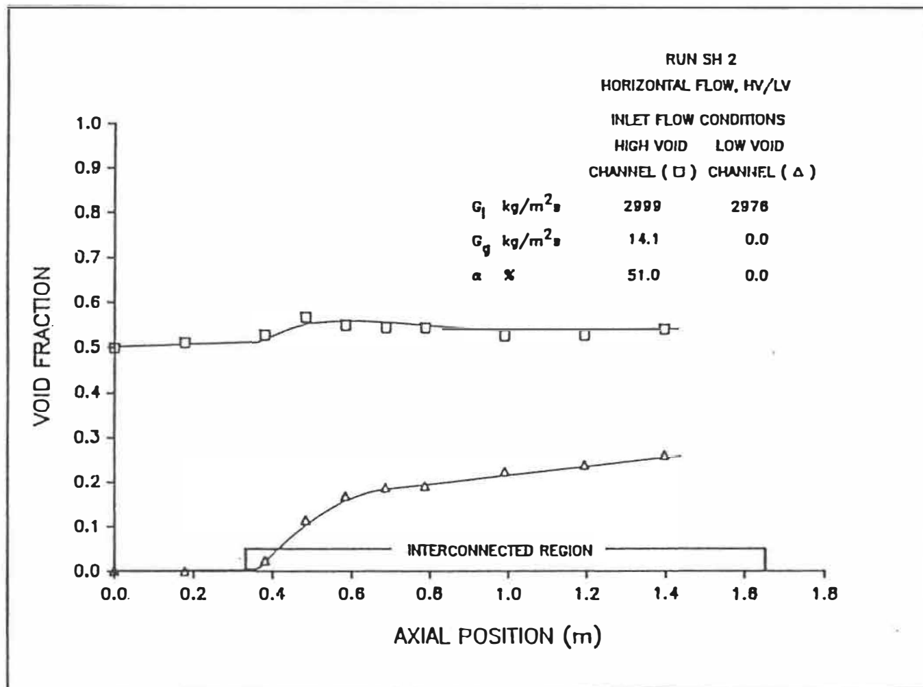
Figure 5.2a: Distribution axiale du taux de vide.
