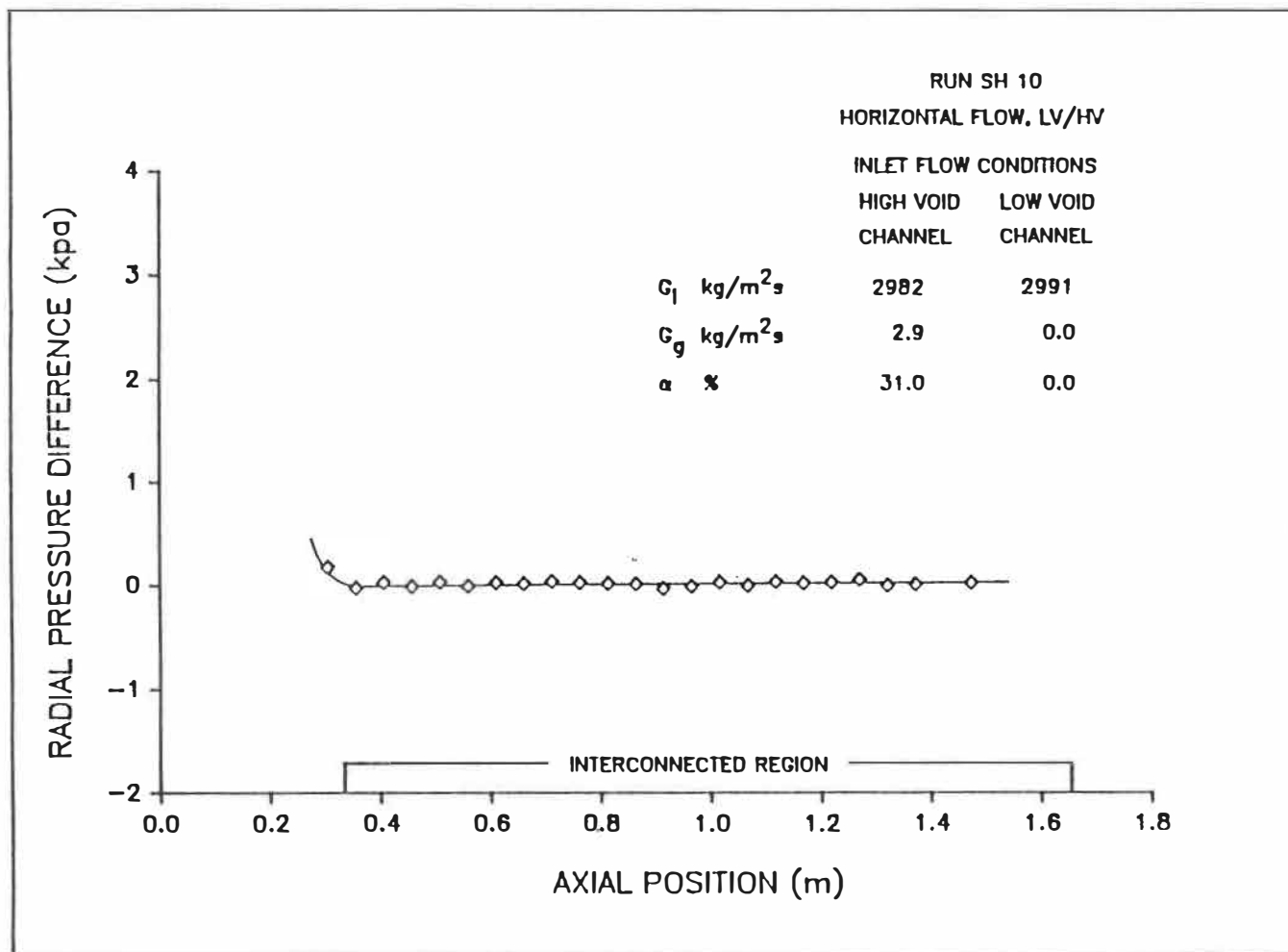
Figure 5.10e: Distribution axiale de la différence des pressions radiales.
