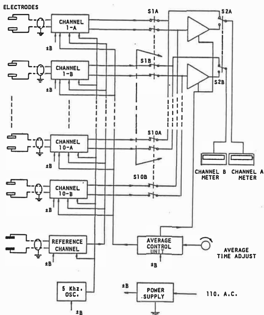
Figure 3.5: Schéma du système de mesure du taux de vide.
