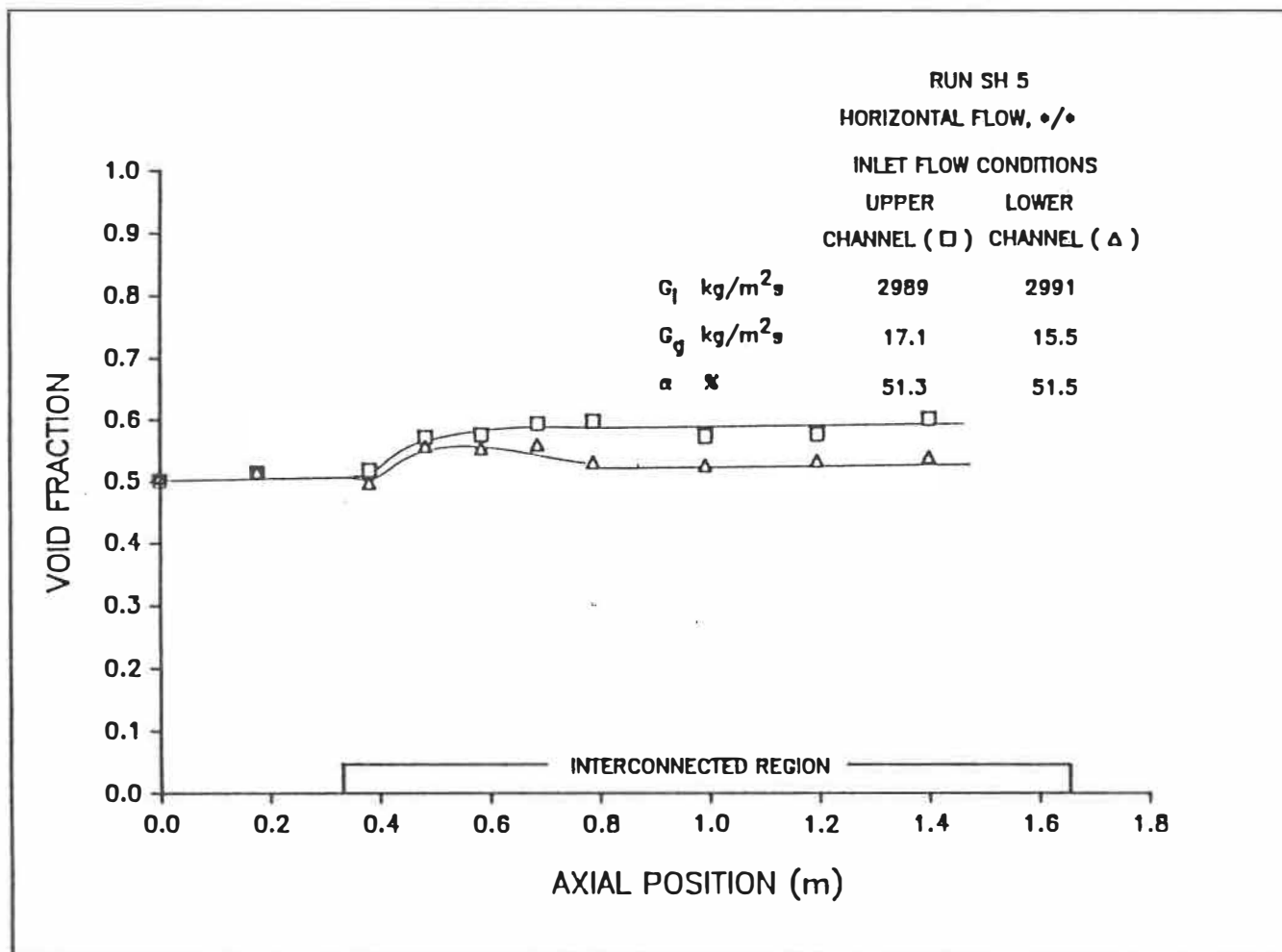
Figure 5.5a: Distribution axiale du taux de vide.
