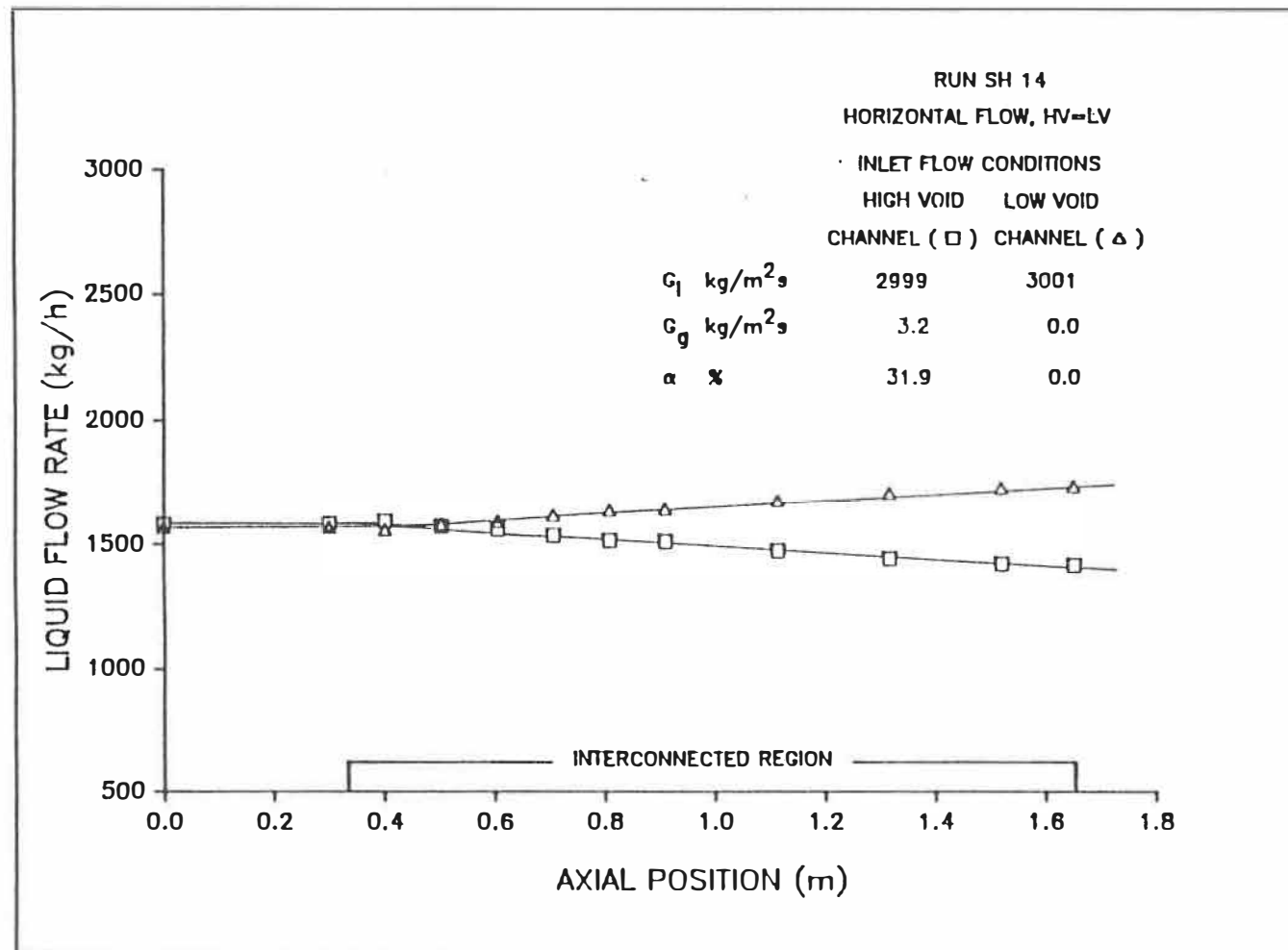
Figure 5.14b: Distribution axiale du débit massique du liquide.
