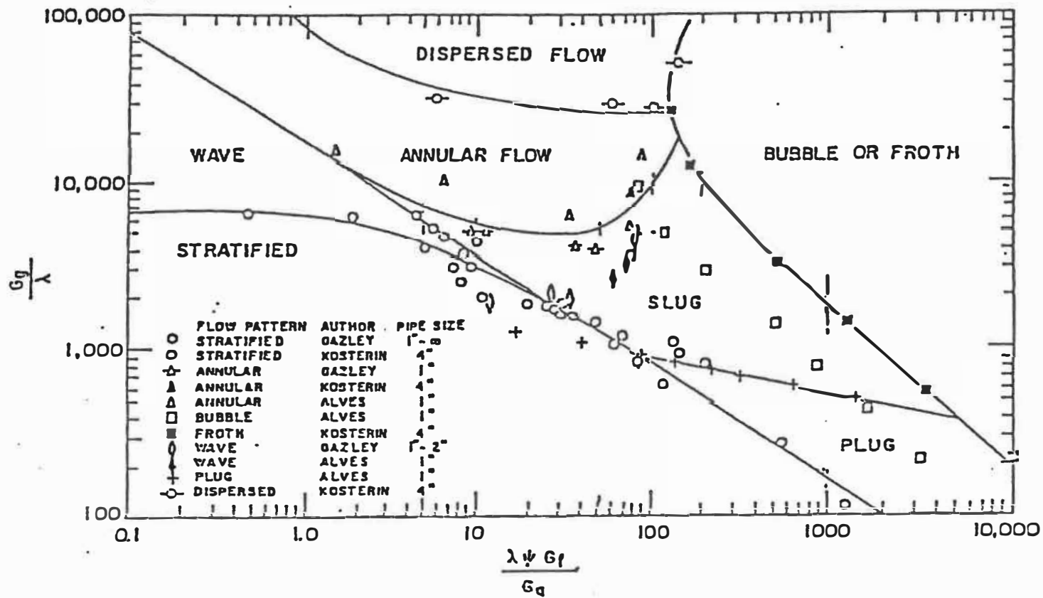
Figure 2.3: Carte des configurations de l'écoulement diphasique (eau-air) horizontal.
