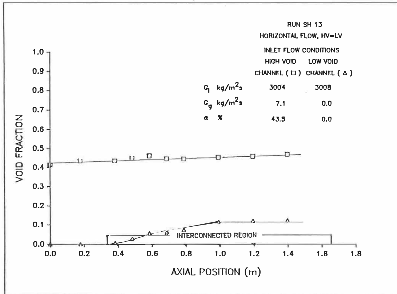
Figure 5.13a: Distribution axiale du taux de vide.
