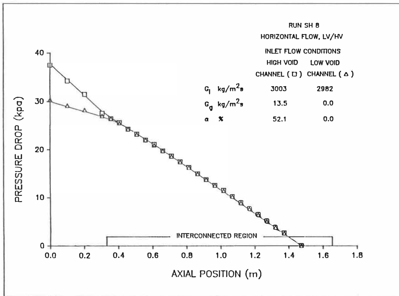
Figure 5.8d: Distribution axiale de la perte de pression axiale.
