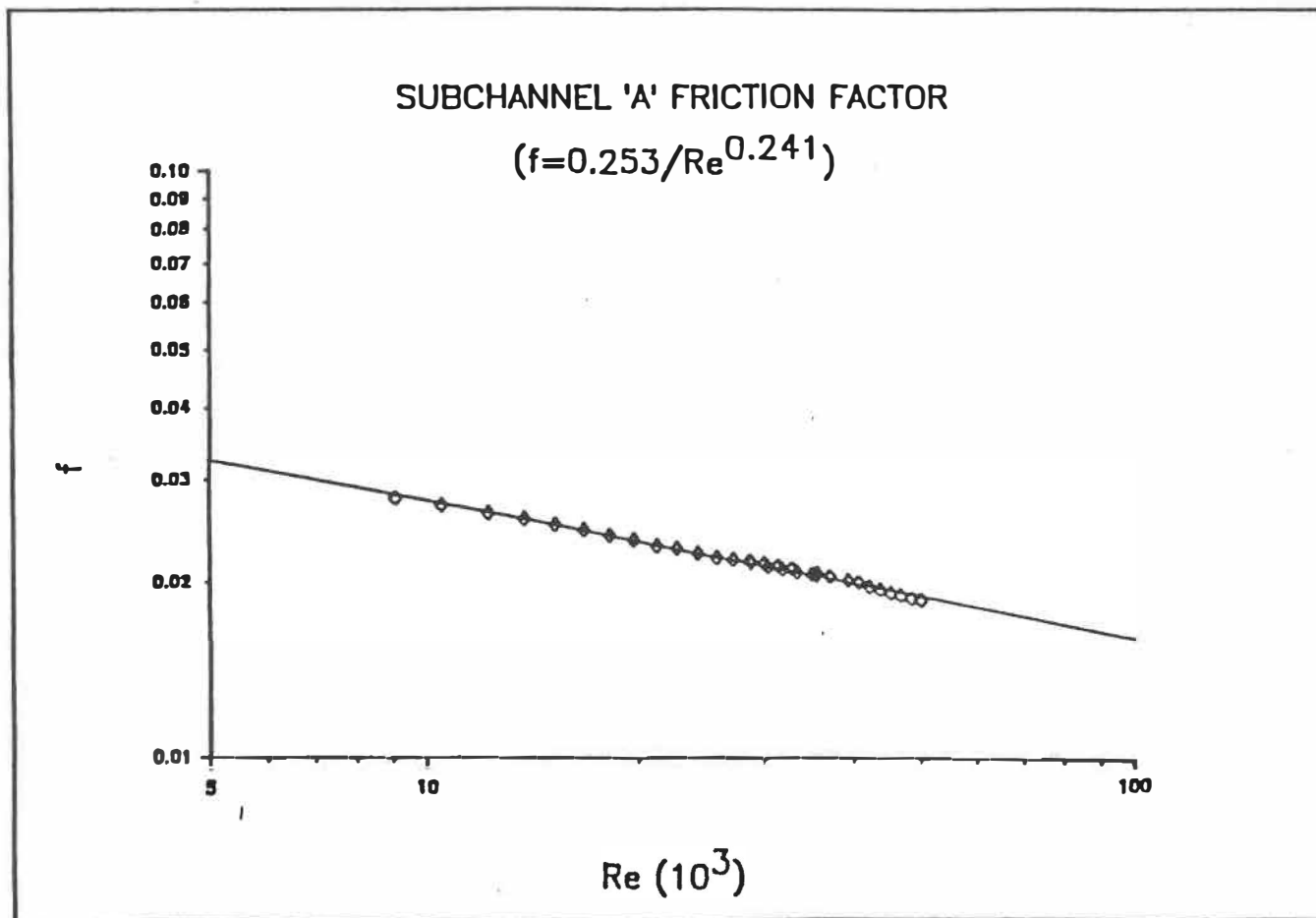
Figure 4.5: Variation du facteur de frottement f .vs. le nombre de Reynolds Re .
