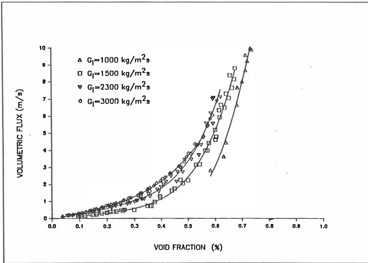
Figure 4.3: Relation entre le flux volumétrique du gaz j_g et le taux de vide moyen.
