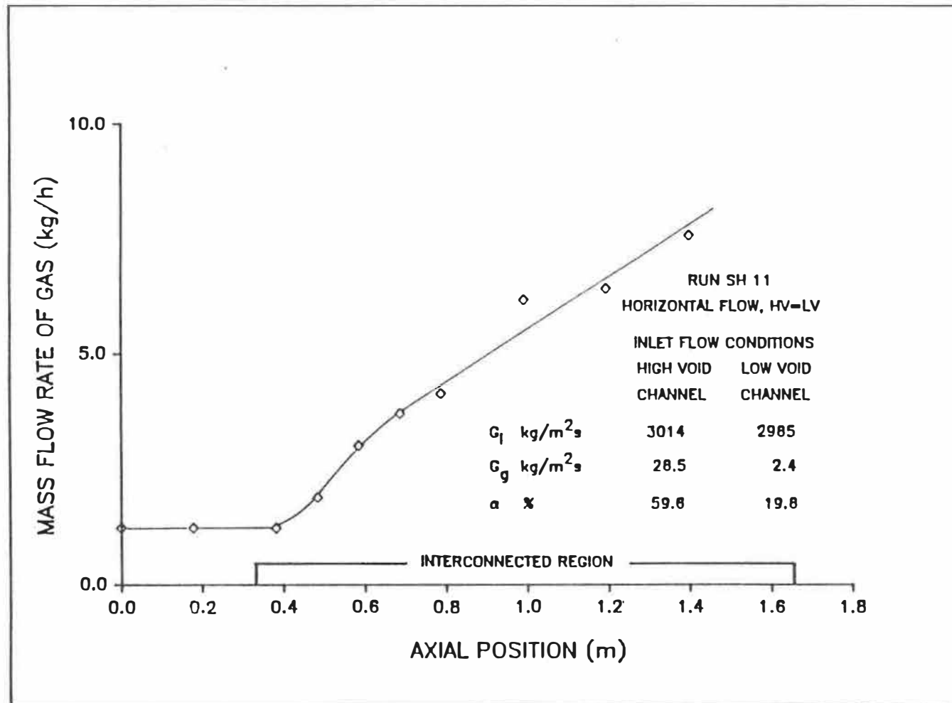
Figure 5.11c: Distribution axiale du débit massique du gaz.
