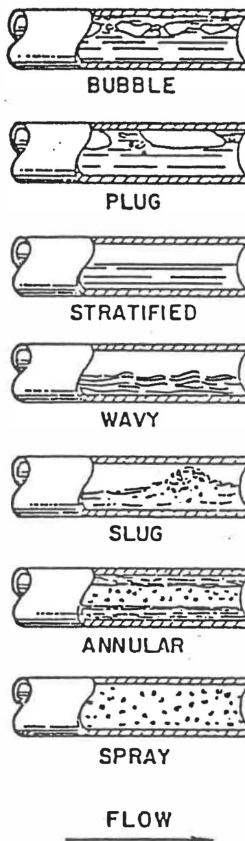
Figure 2.1: Les configurations de l'écoulement diphasique horizontal adiabatique.
