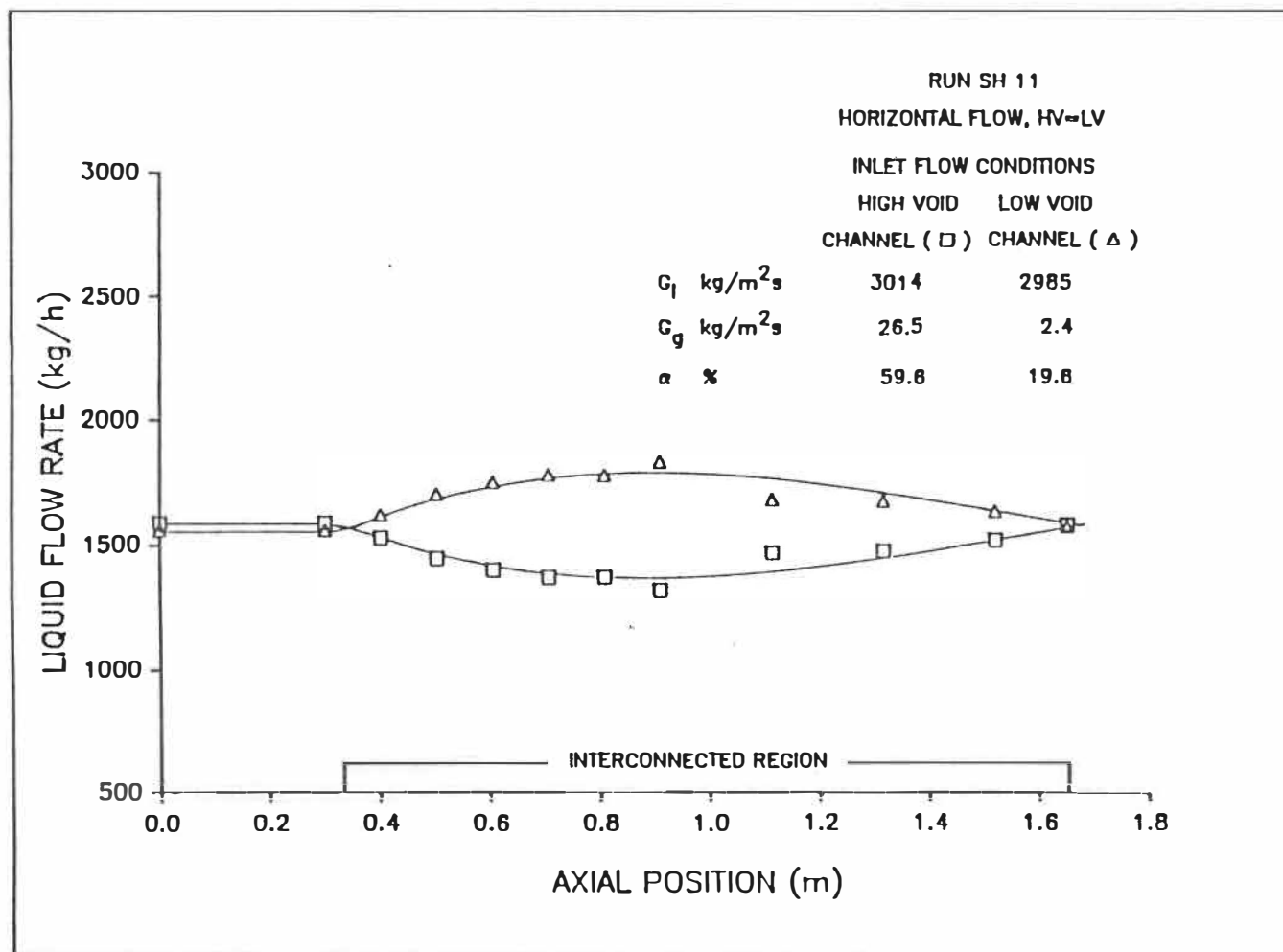
Figure 5.11b: Distribution axiale du débit massique du liquide.
