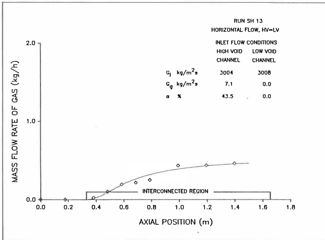
Figure 5.13c: Distribution axiale du débit massique du gaz.
