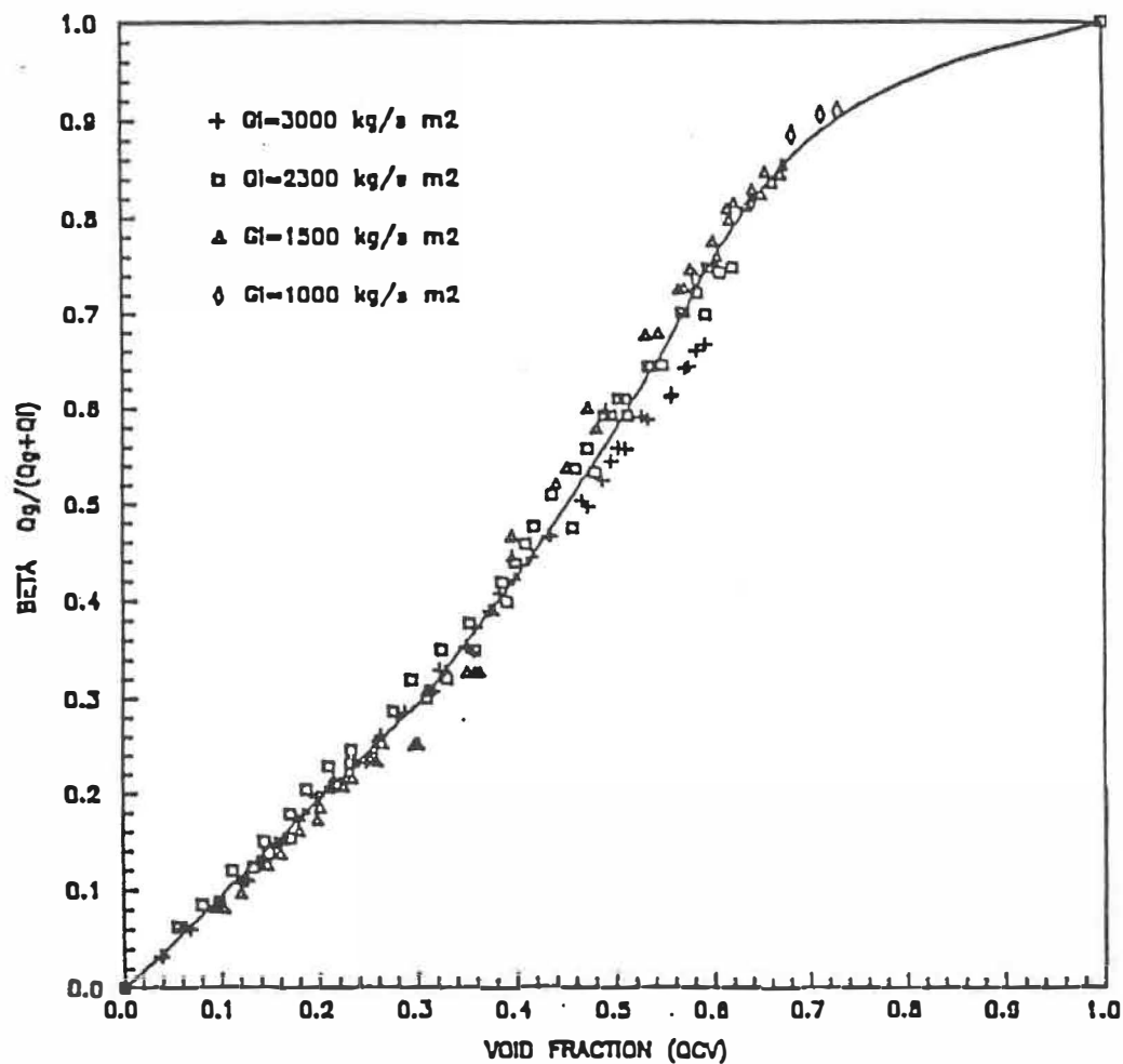
Figure 4.2: Relation entre le titre volumétrique \beta et le taux de vide \alpha .
