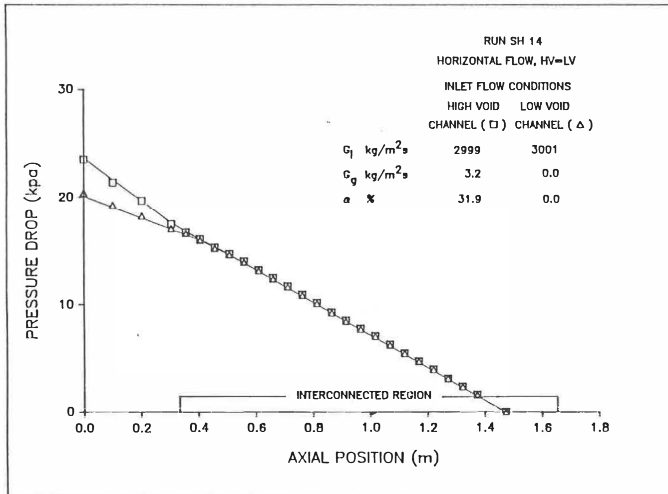
Figure 5.14d: Distribution axiale de la perte de pression axiale.
