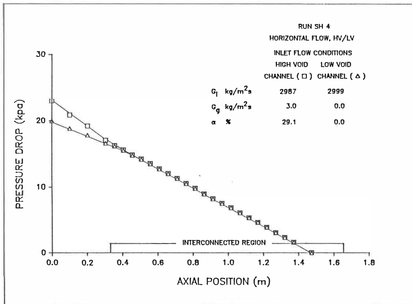
Figure 5.4d: Distribution axiale de la perte de pression axiale.
