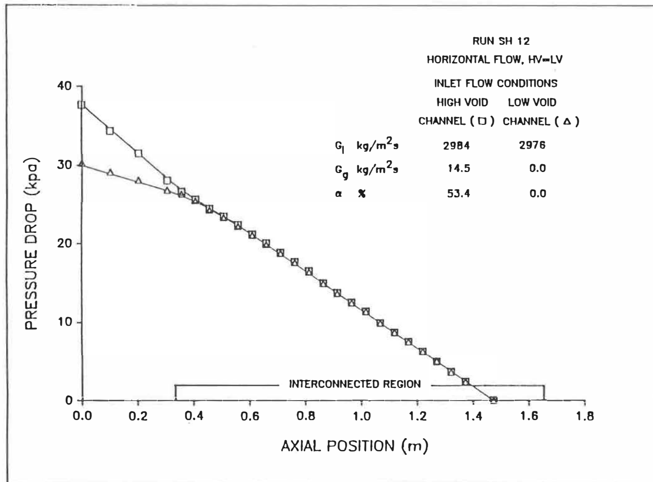
Figure 5.12d: Distribution axiale de la perte de pression axiale.
