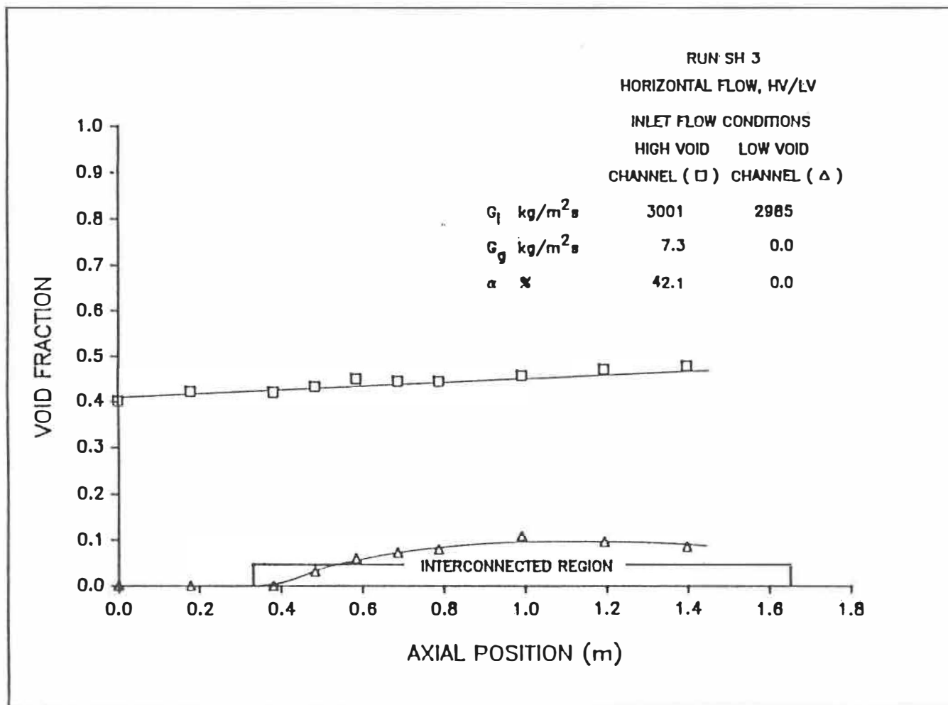
Figure 5.3a: Distribution axiale du taux de vide.
