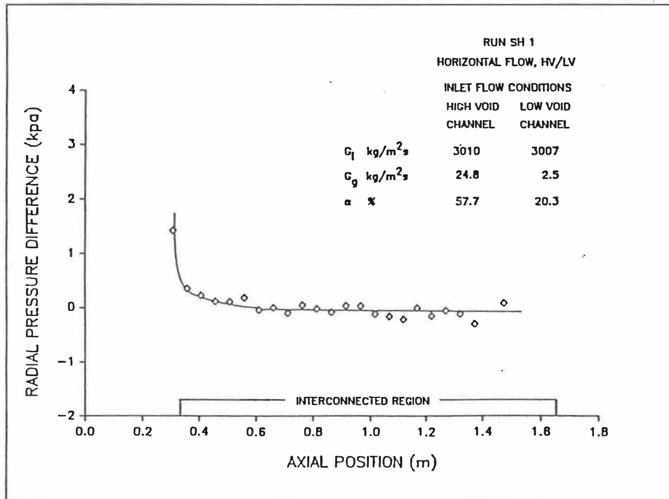
Figure 5.1e: Distribution axiale de la différence des pressions radiales.
