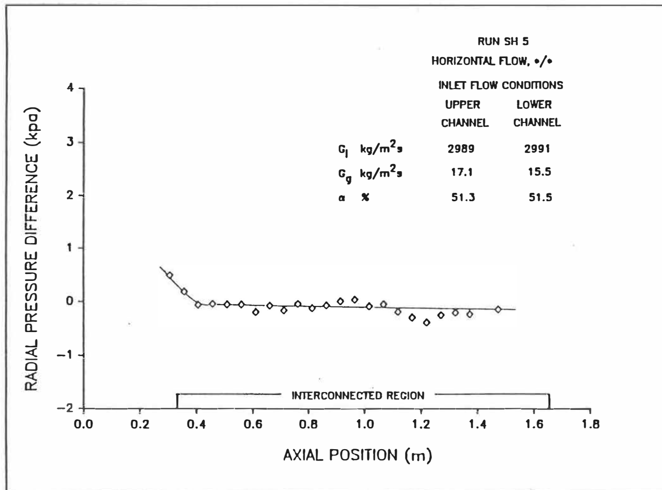
Figure 5.5e: Distribution axiale de la différence des pressions radiales.
