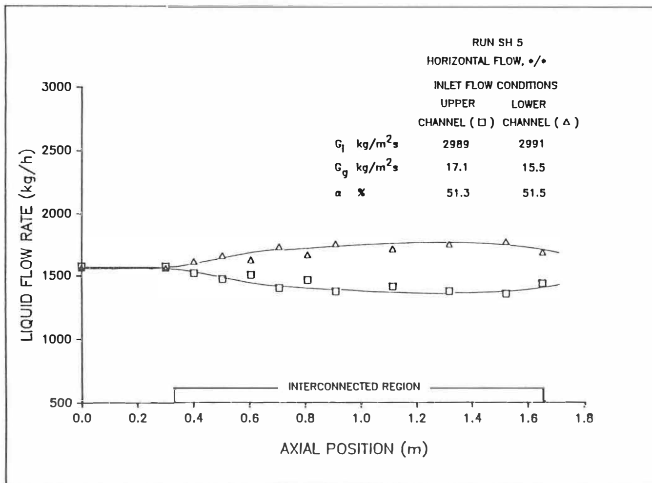
Figure 5.5b: Distribution axiale du débit massique du liquide.
