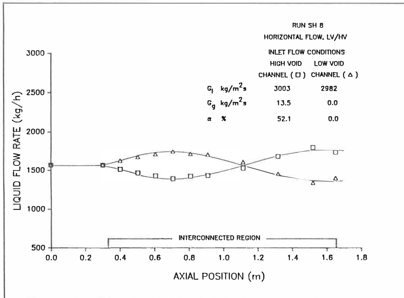
Figure 5.8b: Distribution axiale du débit massique du liquide.
