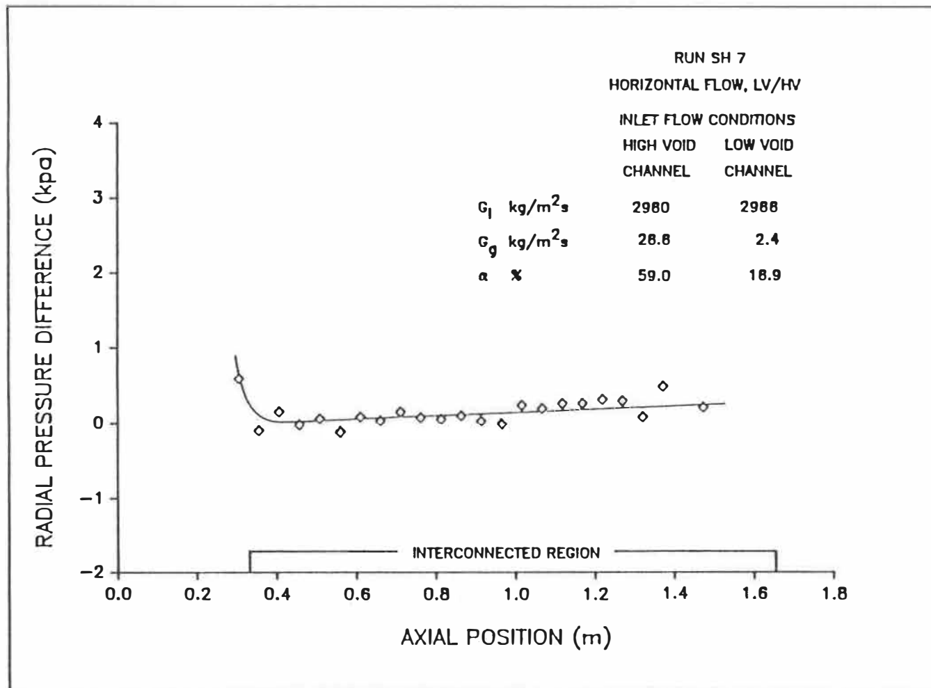
Figure 5.7e: Distribution axiale de la différence des pressions radiales.
