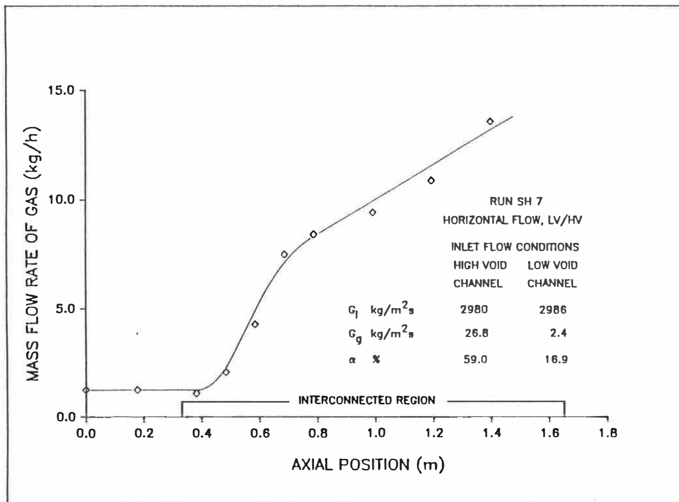
Figure 5.7c: Distribution axiale du débit massique du gaz.
