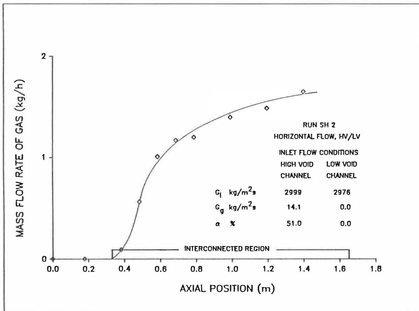
Figure 5.2c: Distribution axiale du débit massique du gaz.
