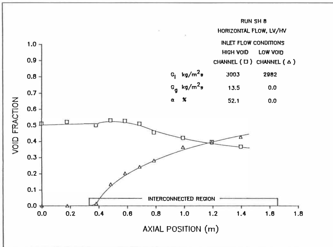
Figure 5.8a: Distribution axiale du taux de vide.
