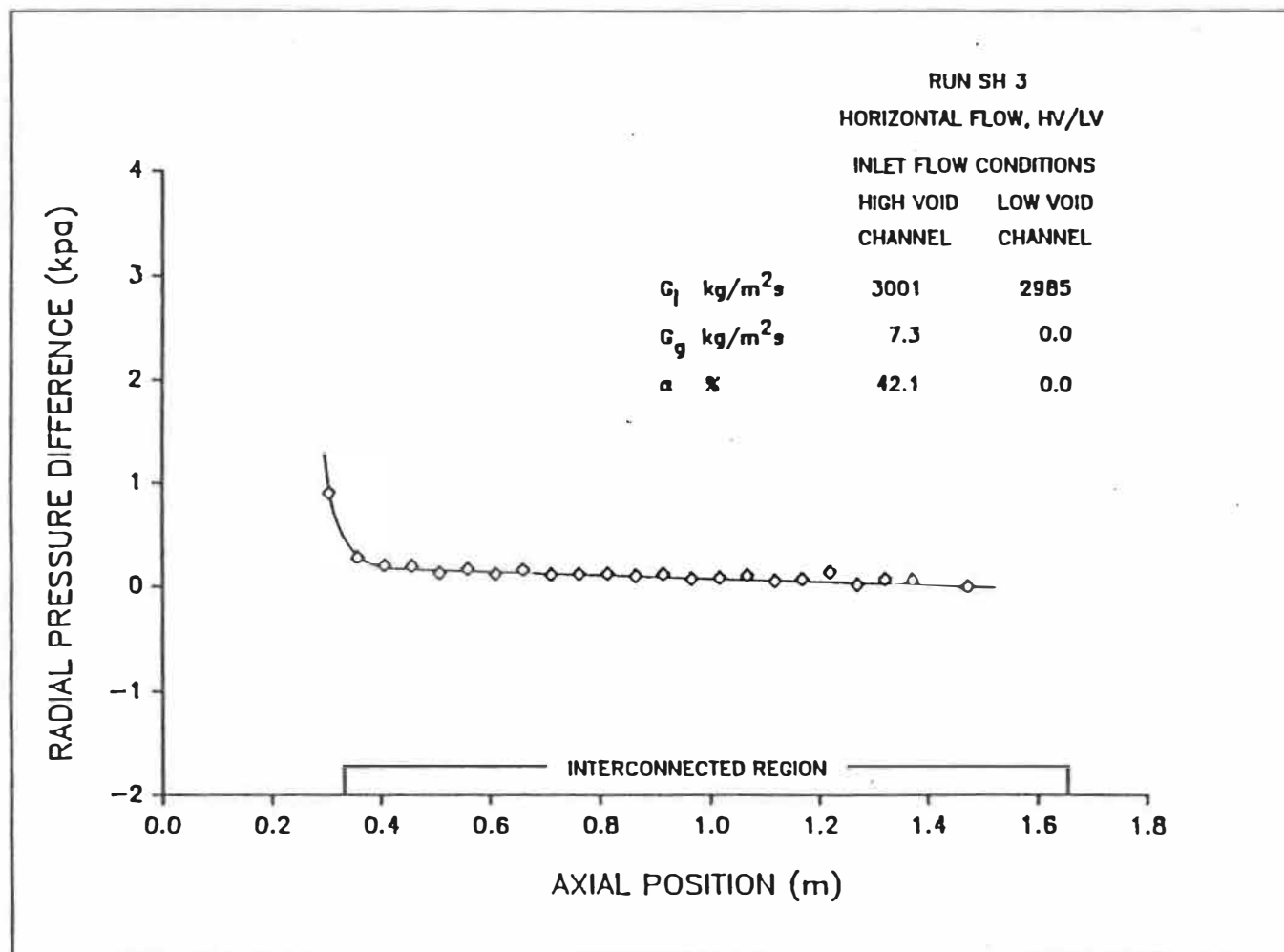
Figure 5.3e: Distribution axiale de la différence des pressions radiales.
