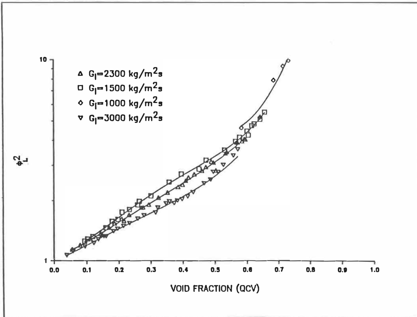
Figure 4.6: Variation du coefficient multiplicatif de deux phases \phi_L^2 .
