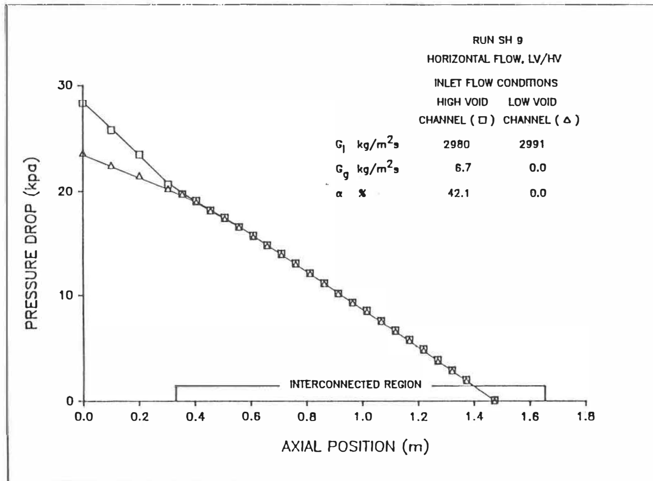
Figure 5.9d: Distribution axiale de la perte de pression axiale.
