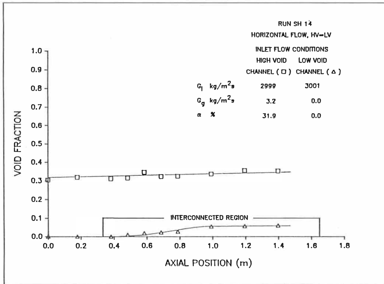
Figure 5.14a: Distribution axiale du taux de vide.
