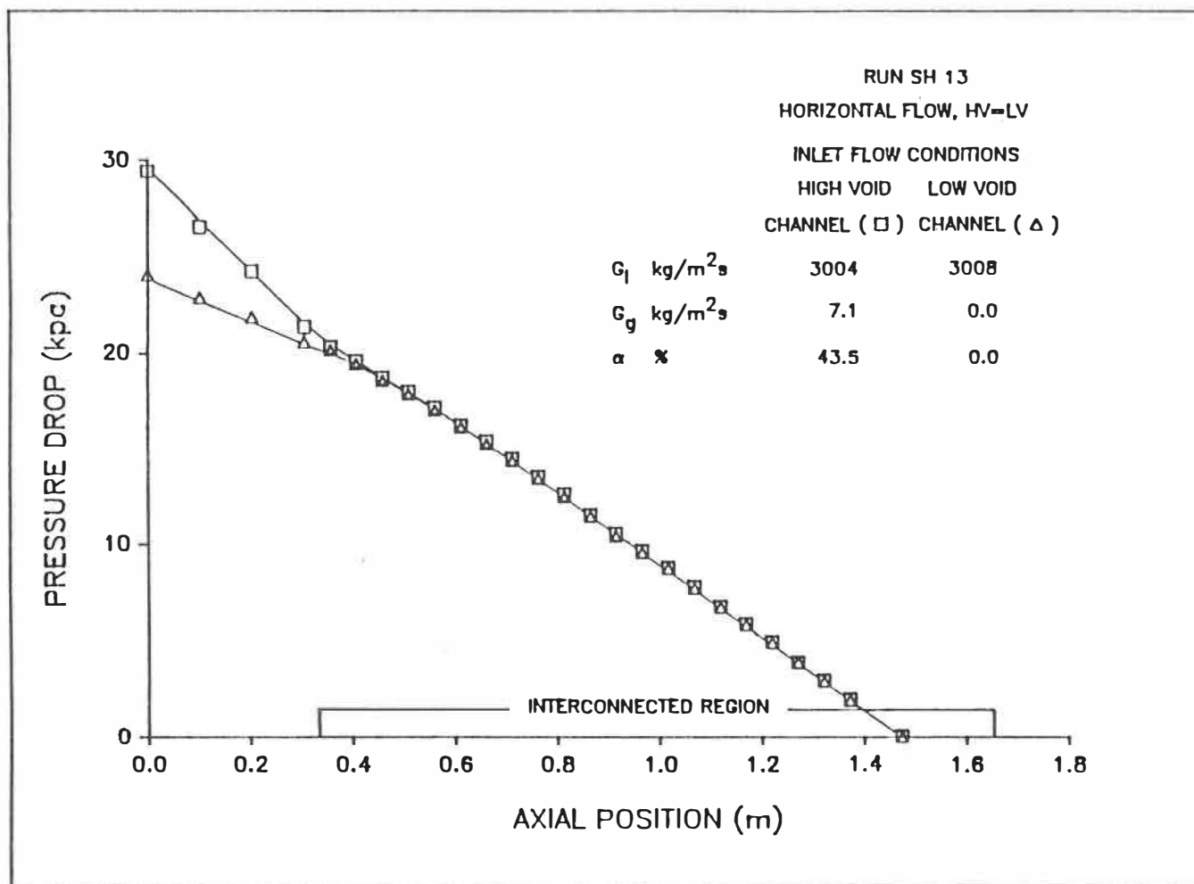
Figure 5.13d: Distribution axiale de la perte de pression axiale.
