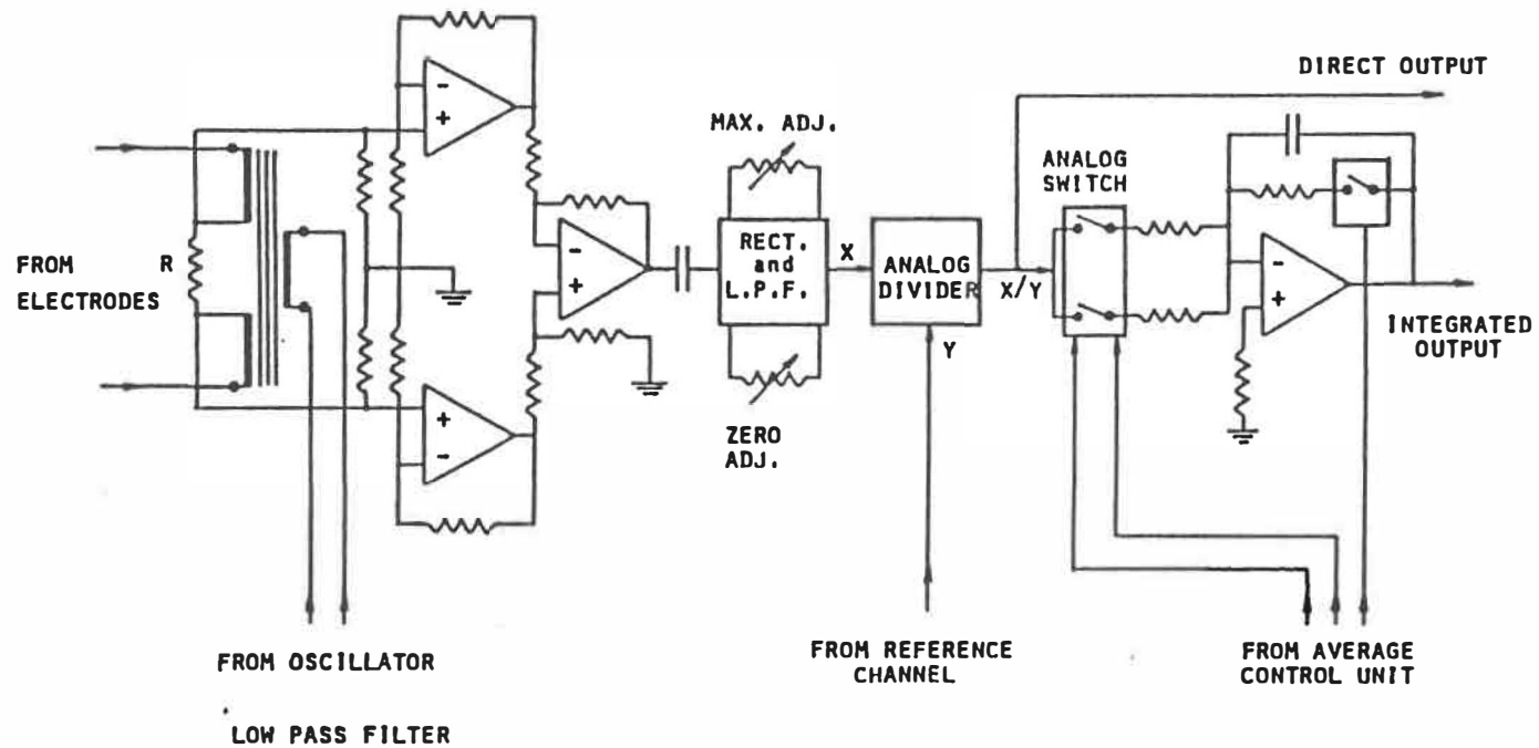
Figure 3.6: Schéma détaillé du circuit électronique associé avec chaque électrode.
