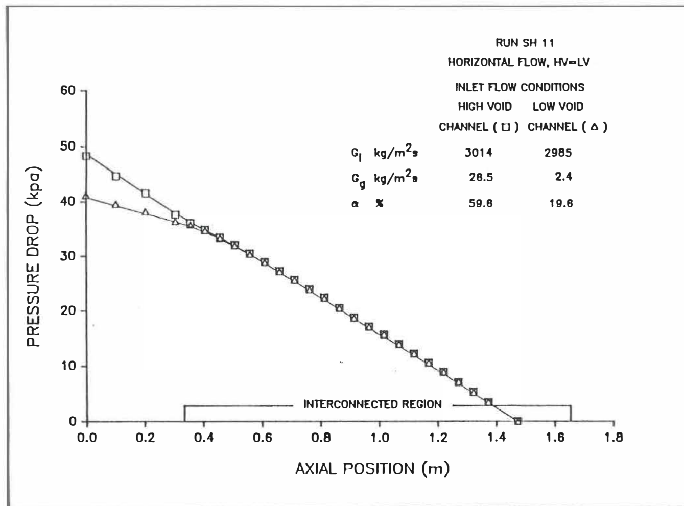
Figure 5.11d: Distribution axiale de la perte de pression axiale.
