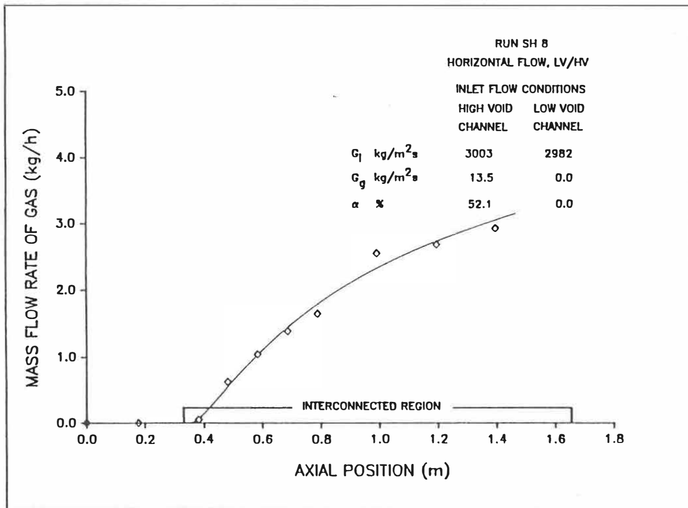
Figure 5.8c: Distribution axiale du débit massique du gaz.
