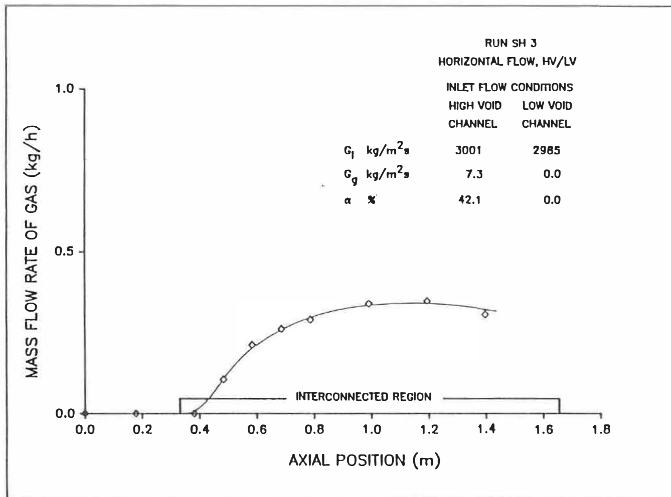
Figure 5.3c: Distribution axiale du débit massique du gaz.
