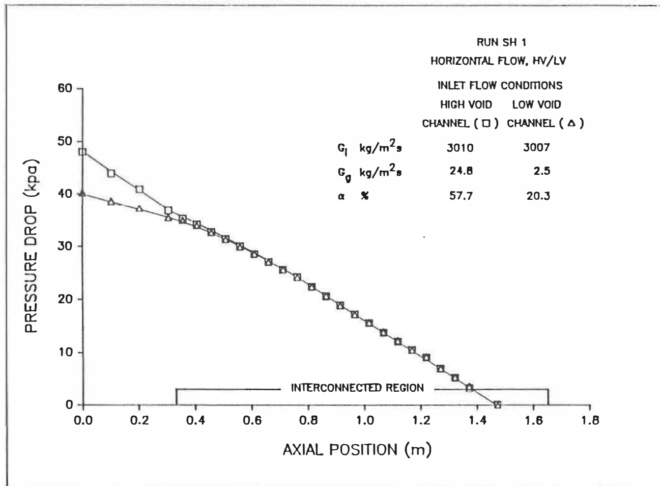
Figure 5.1d: Distribution axiale de la perte de pression axiale.
