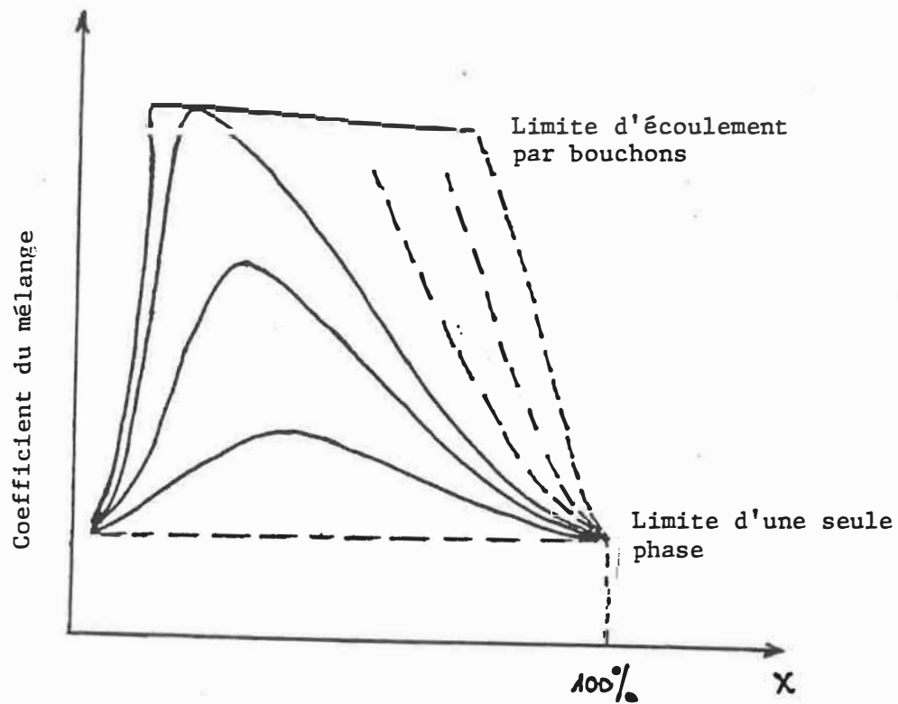
Figure 2.4: Courbe du coefficient de mélange.
