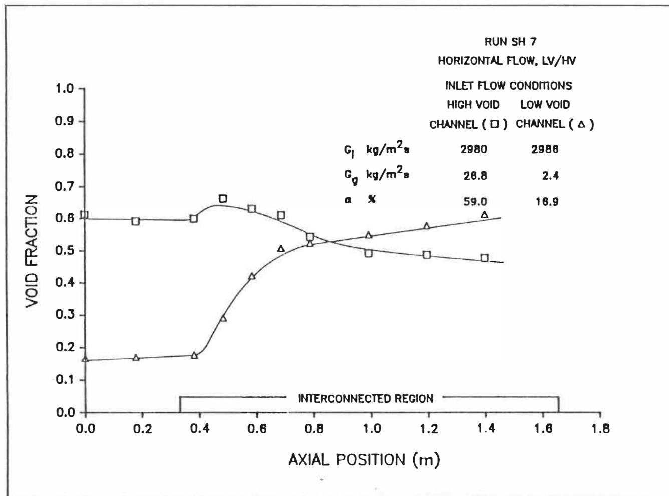
Figure 5.7a: Distribution axiale du taux de vide.
