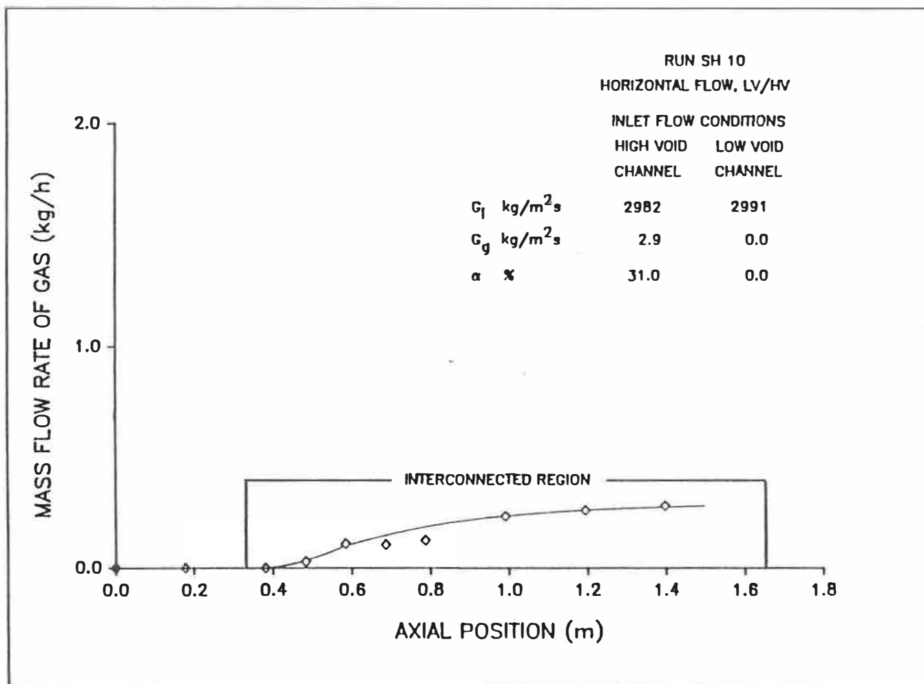
Figure 5.10c: Distribution axiale du débit massique du gaz.
