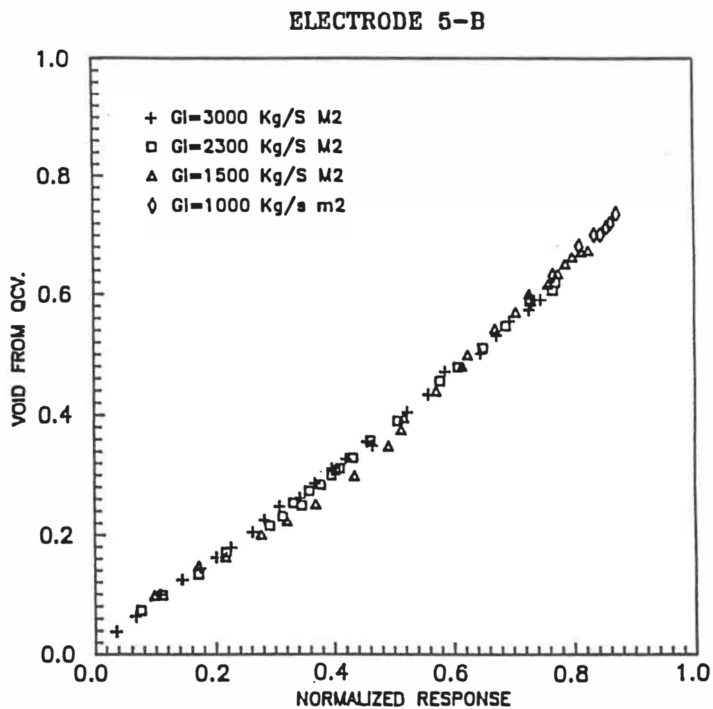
Figure 4.1b: Courbe de calibration de l'électrode (2-5).
