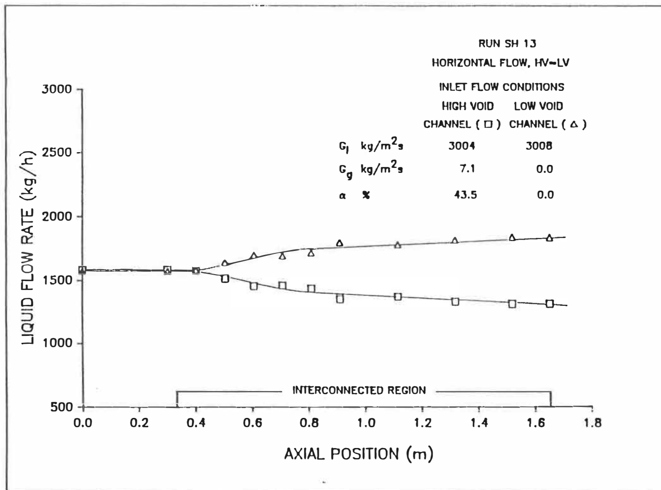
Figure 5.13b: Distribution axiale du débit massique du liquide.
