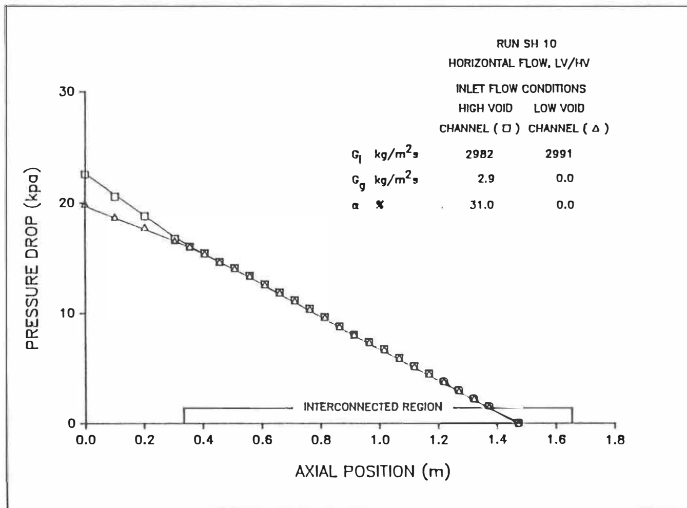
Figure 5.10d: Distribution axiale de la perte de pression axiale.
