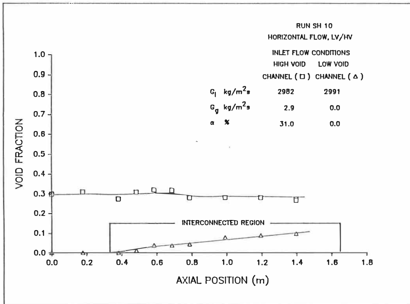
Figure 5.10a: Distribution axiale du taux de vide.
