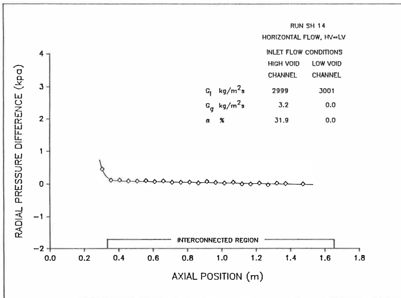
Figure 5.14e: Distribution axiale de la différence des pressions radiales.
