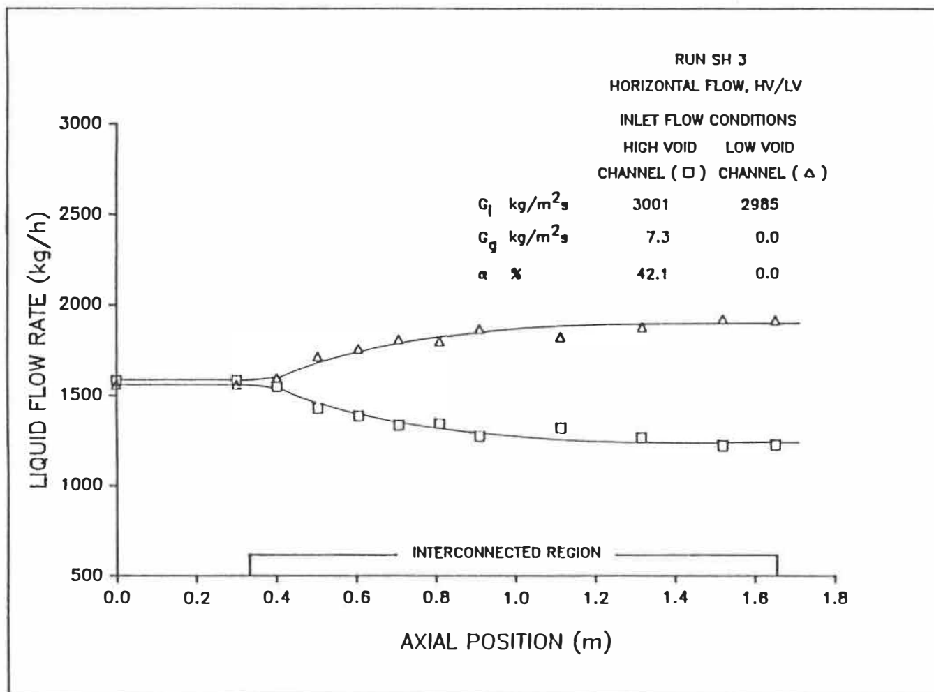
Figure 5.3b: Distribution axiale du débit massique du liquide.
