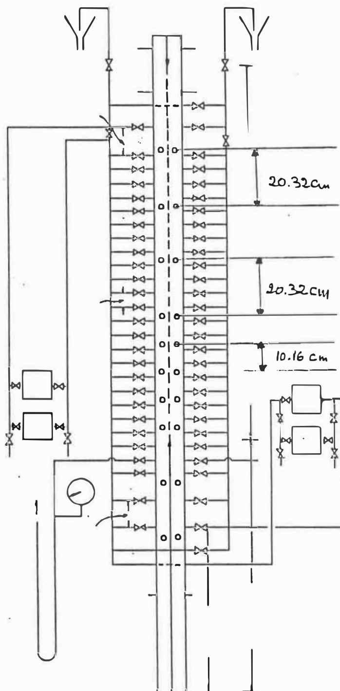
Figure 3.4: Positions des électrodes et des stations d'échantillonnage du traceur.
