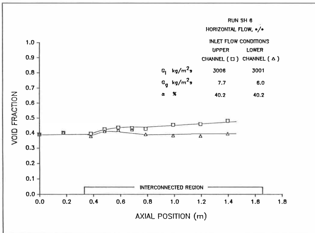
Figure 5.6a: Distribution axiale du taux de vide.
