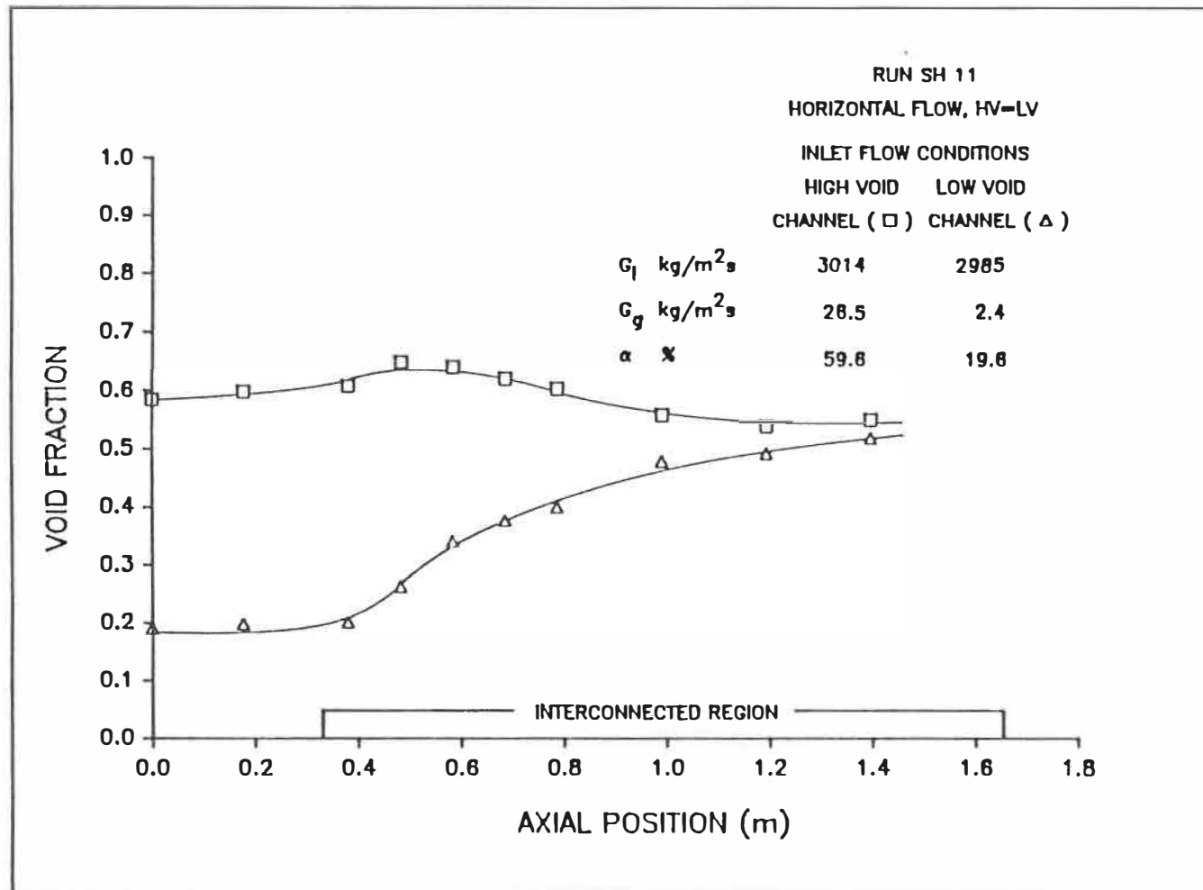
Figure 5.11a: Distribution axiale du taux de vide.
