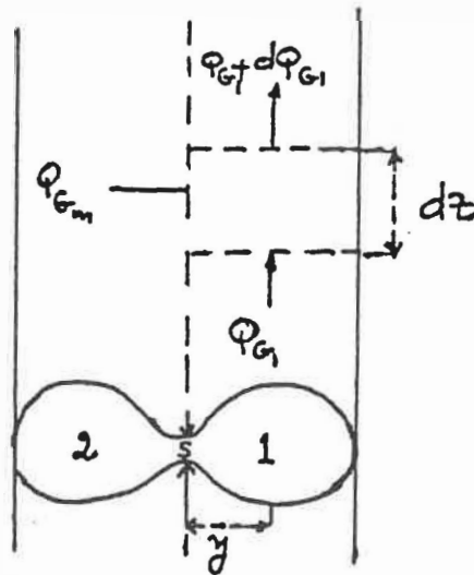
Figure 2.5: Schéma du volume de contrôle.
