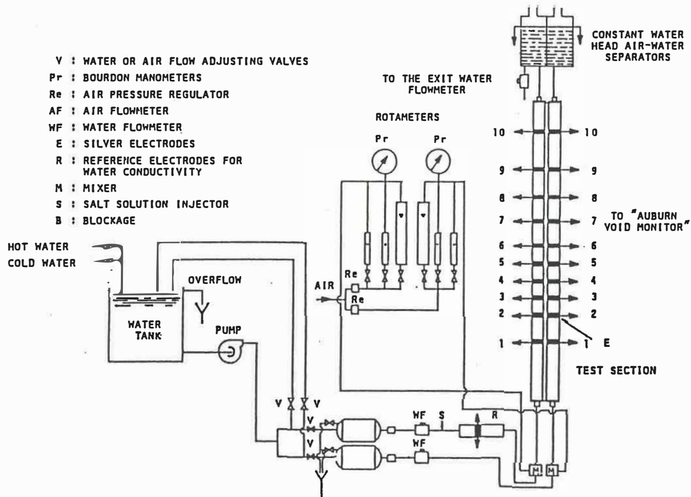
Figure 3.1: Appareils expérimentaux.
