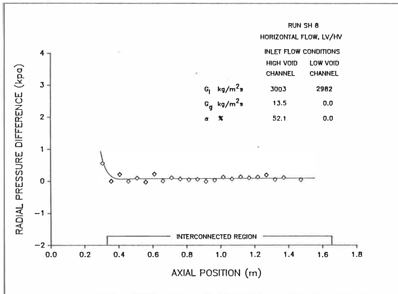
Figure 5.8e: Distribution axiale de la différence des pressions radiales.
