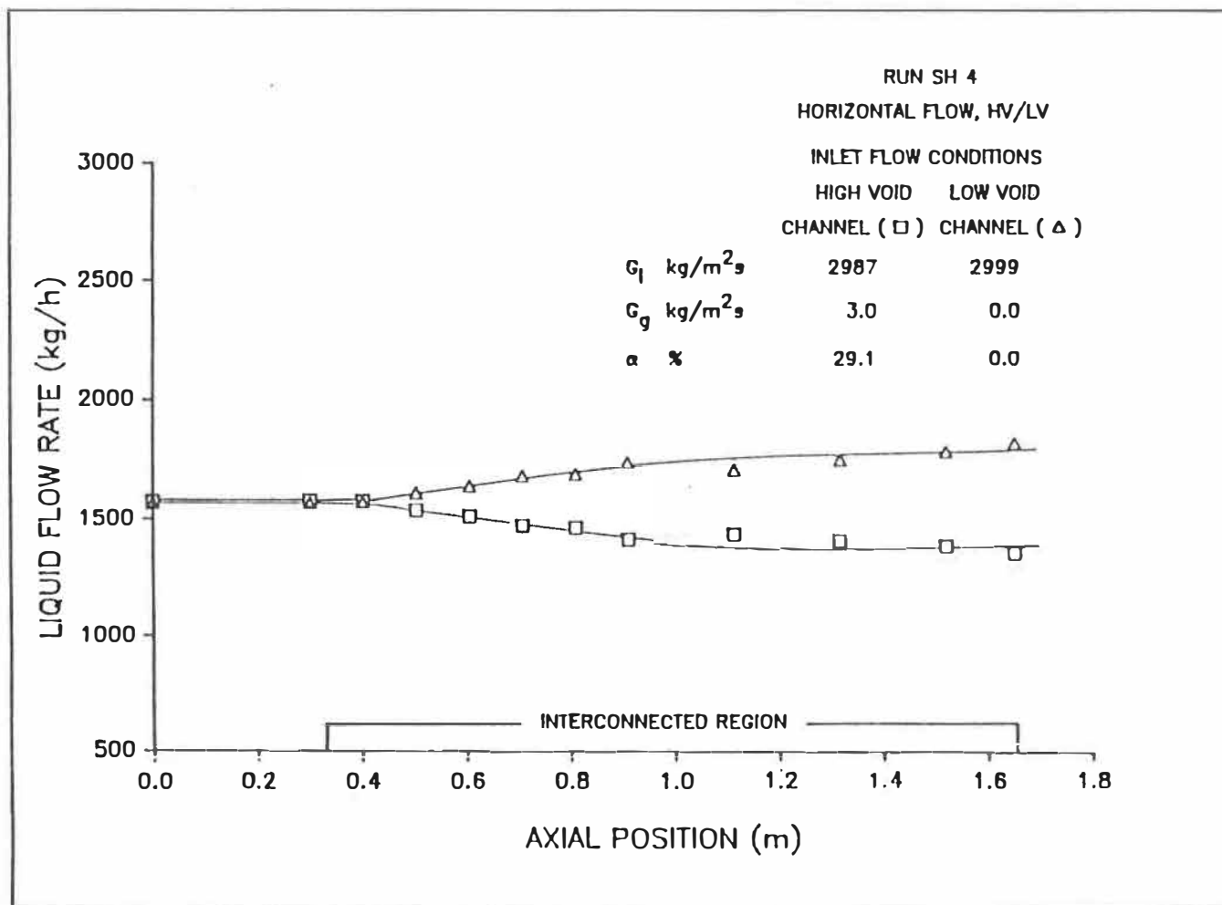
Figure 5.4b: Distribution axiale du débit massique du liquide.
