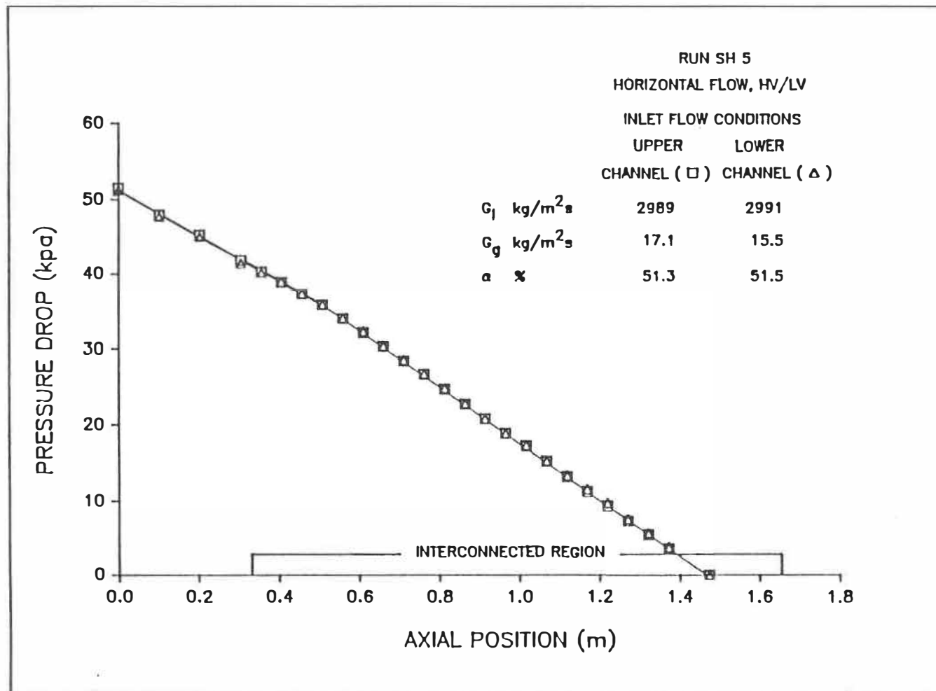
Figure 5.5d: Distribution axiale de la perte de pression axiale.
