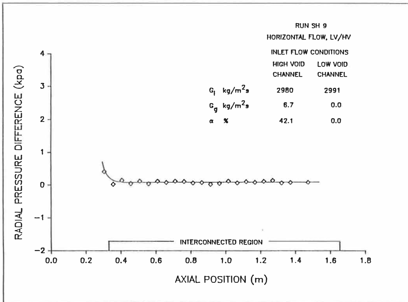
Figure 5.9e: Distribution axiale de la différence des pressions radiales.
