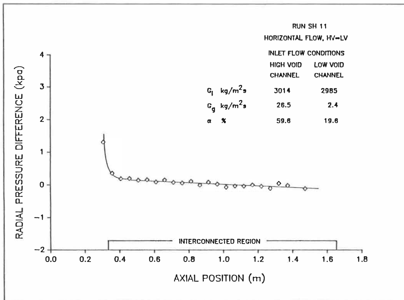
Figure 5.11e: Distribution axiale de la différence des pressions radiales.
