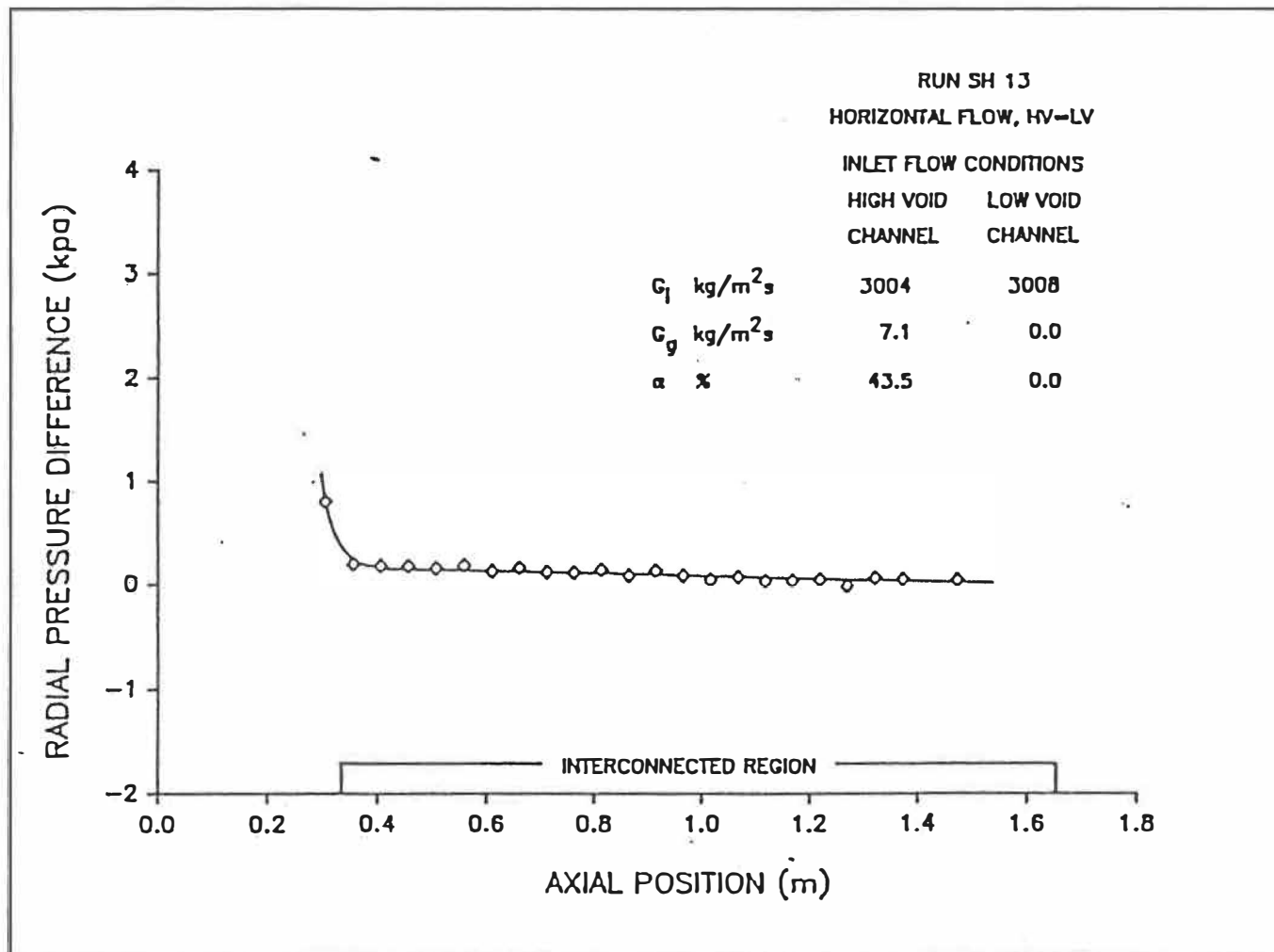
Figure 5.13e: Distribution axiale de la différence des pressions radiales.
