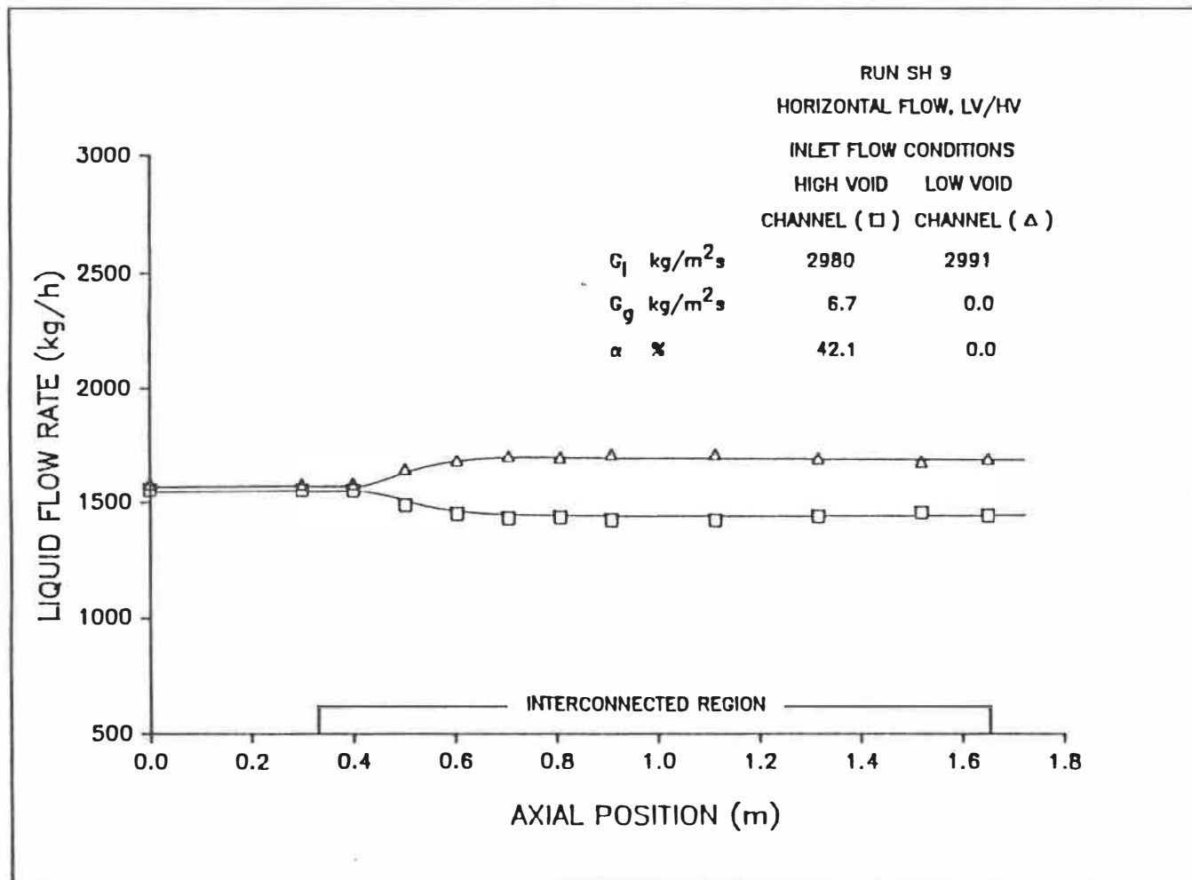
Figure 5.9b: Distribution axiale du débit massique du liquide.
