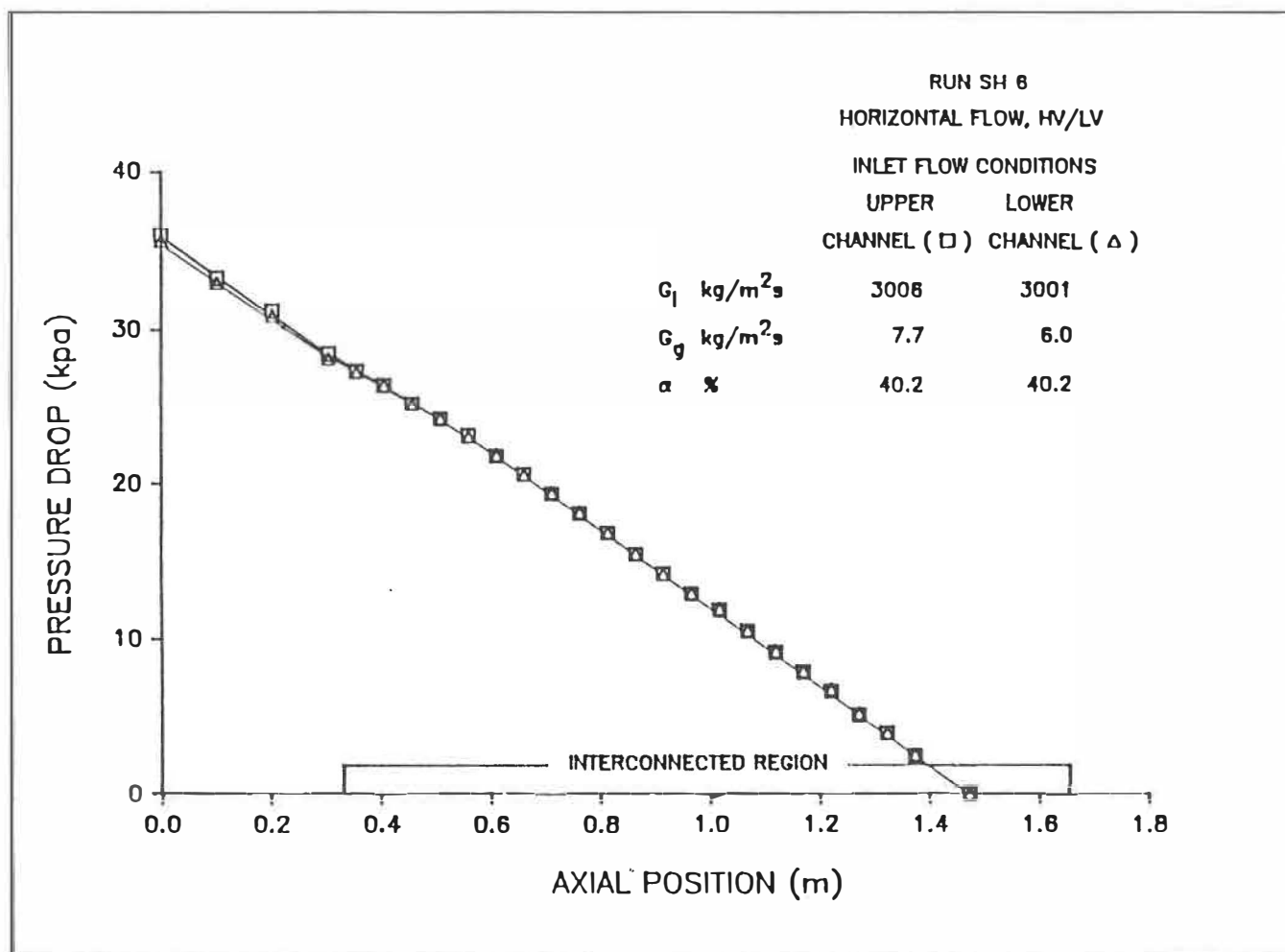
Figure 5.6d: Distribution axiale de la perte de pression axiale.
