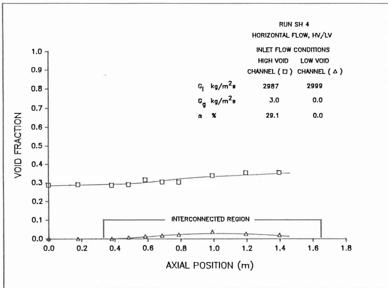
Figure 5.4a: Distribution axiale du taux de vide.
