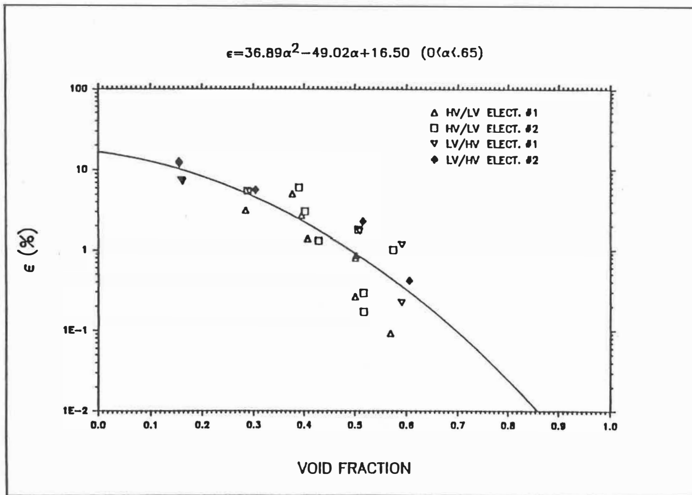
Figure 4.8: Facteur de correction en fonction du taux de vide.
