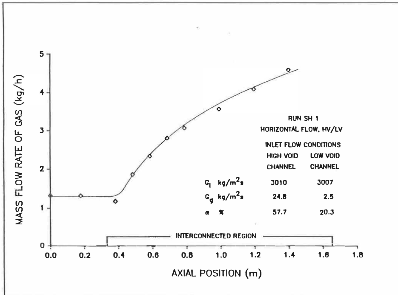
Figure 5.1c: Distribution axiale du débit massique du gaz.
