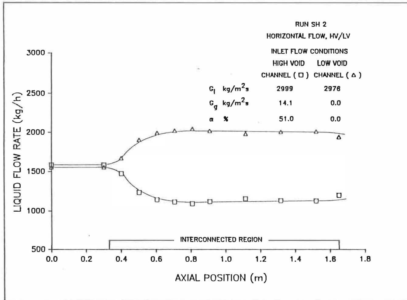
Figure 5.2b: Distribution axiale du débit massique du liquide.
