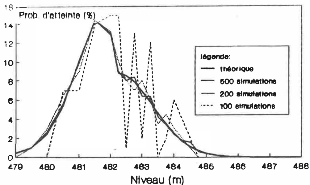
Figure 6.6 Comparaison des probabilités d'atteinte au début de la période 6.
