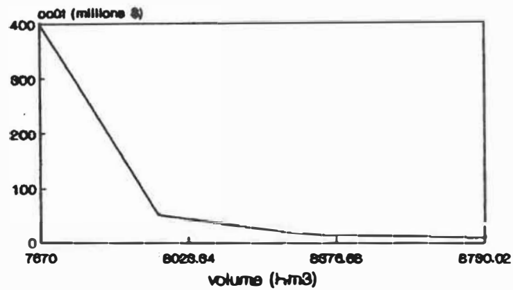
Figure 4.4 Coût de dépassement du niveau minimal acceptable.
