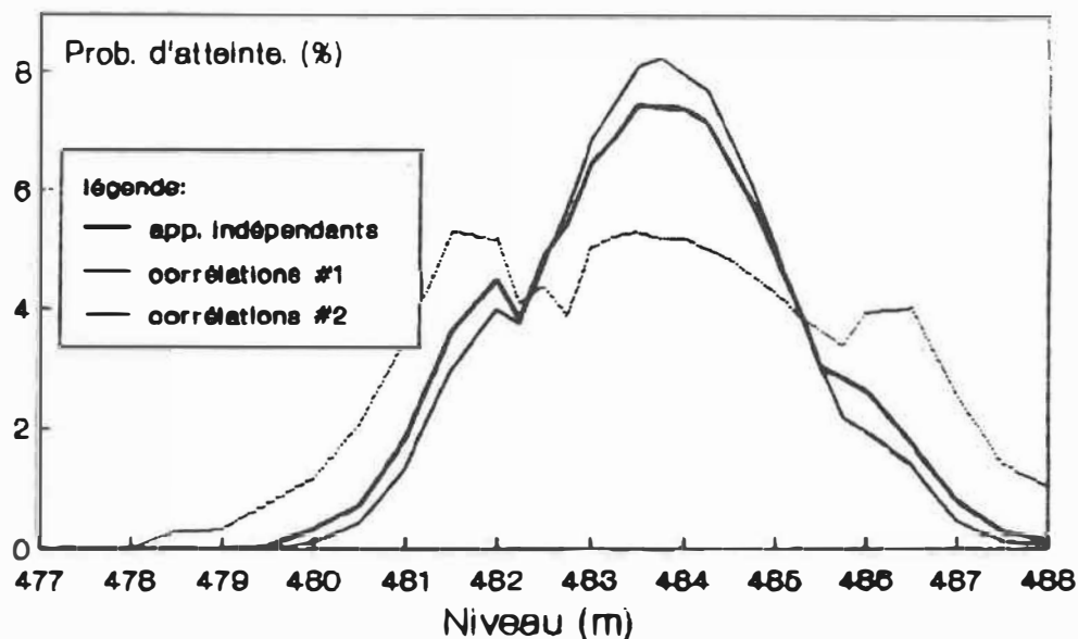
Figure 6.1 Comparaison de la probabilité d'atteinte au début de la période 7.
