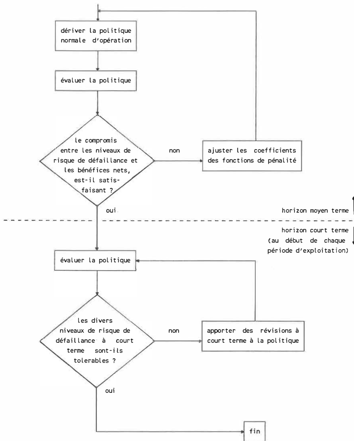
Figure 1.1 Représentation schématique de la méthodologie de gestion.
