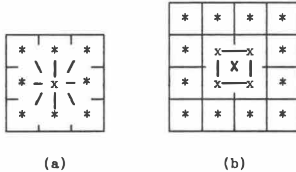
Figure 4.5.1. Bloc de 4 pixels donnant \pi_B = 8 \times 4 - 6 = 26 paires distinctes de pixels: (a) chaque pixel du bloc fait partie de 8 cliques de 2 pixels; (b) les paires formées de 2 pixels appartenant au bloc - ceux marqués par un x - apparaissent 2 fois.
