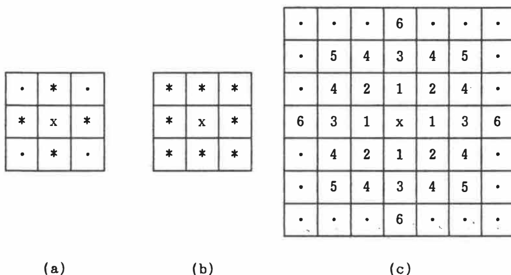
Figure 3.3.1 Système de voisinages: (a) voisinage du 1 er ordre formé des 4 pixels les plus proches (notés *) à l'horizontale et à la verticale; (b) voisinage du 2 ème ordre formé des pixels du voisinage du 1 er ordre plus les 4 pixels aux diagonales; (c) voisinages jusqu'à l'ordre 6, chaque ordre conservant toujours les pixels des ordres inférieurs.
