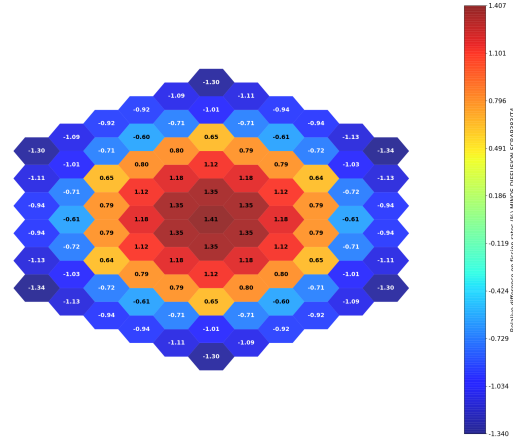
(d) Relative error on fission rates, DOP+VOID configuration.
