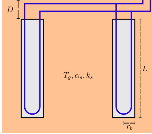
Fig. 1. Borehole geometry and thermal parameters
