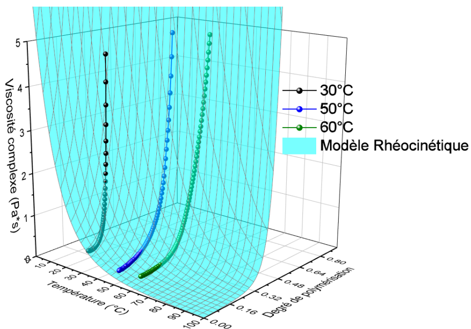
FIGURE 3.8 Viscosité du Bio-PU selon la température et le degré de polymérisation
