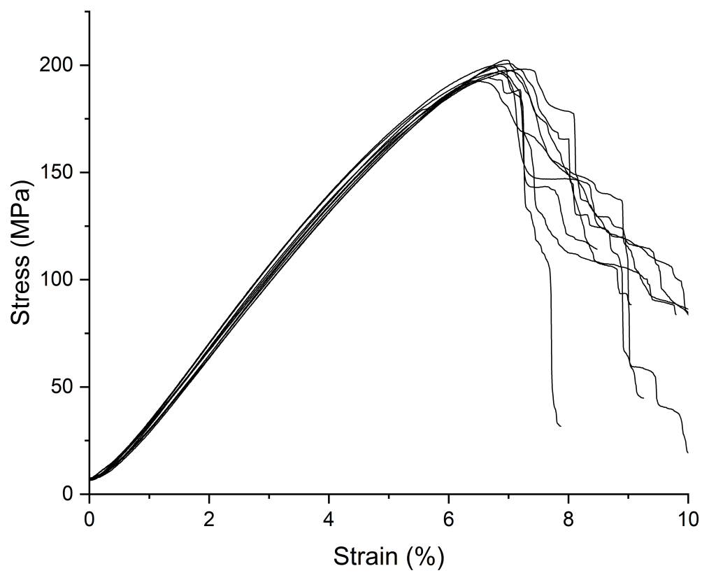
FIGURE B.3 Résultats des essais de cisaillement interlaminaire
