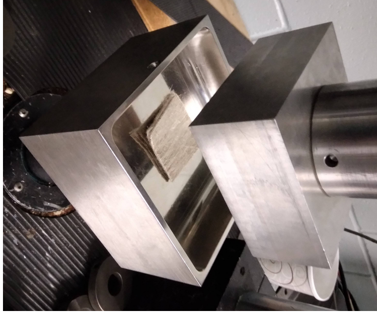
FIGURE 3.12 Montage du test de compaction du renfort de lin lubrifié avec le polyol à base de soya
