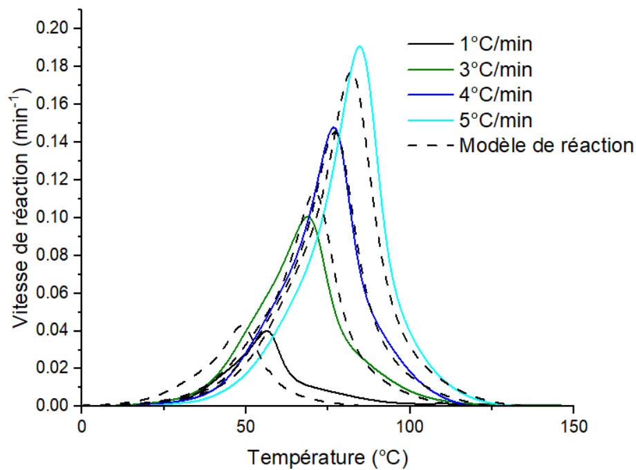
FIGURE 3.5 Vitesse de réaction du Bio-PU selon la rampe de température
