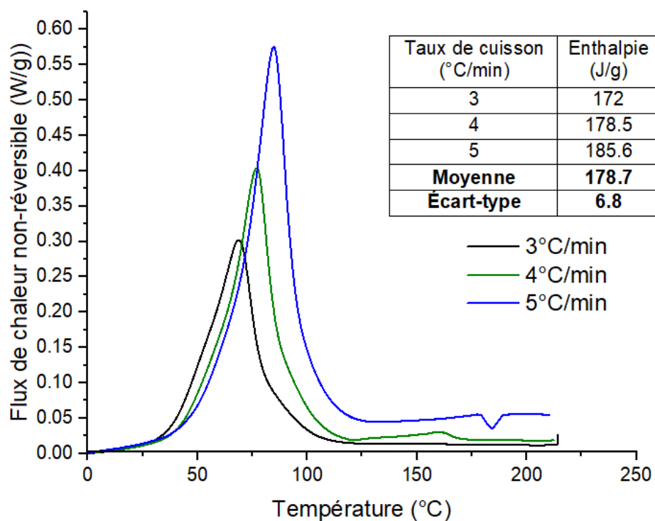
FIGURE 3.3 Flux de chaleur non réversible du Bio-PU selon le taux de température
