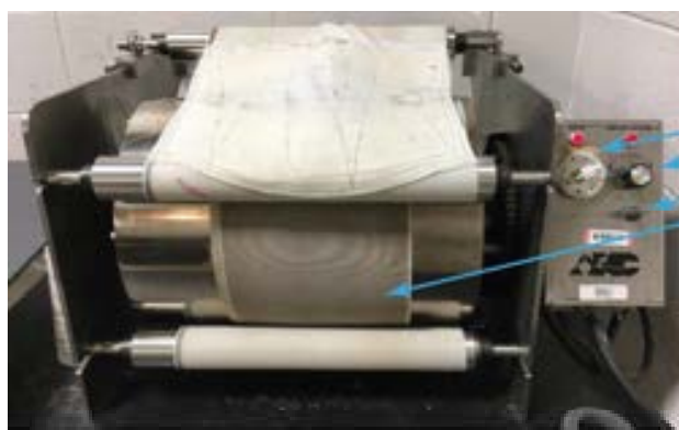
bouton température bouton vitesse bouton Marche/Arrêt mat de lin
