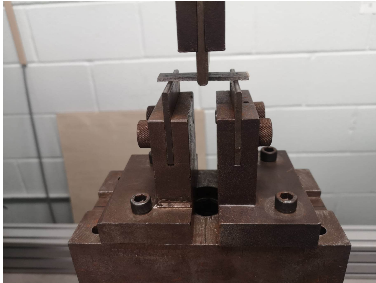
FIGURE 2.18 Montage ASTM D790 pour les essais de flexion
