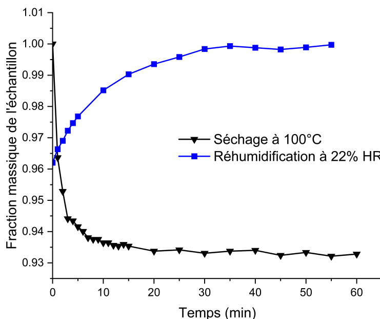
FIGURE 3.16 Fraction massique du renfort de lin lors d'un cycle de séchage à 100°C suivi d'une réhumidification à 22% d'humidité relative.
