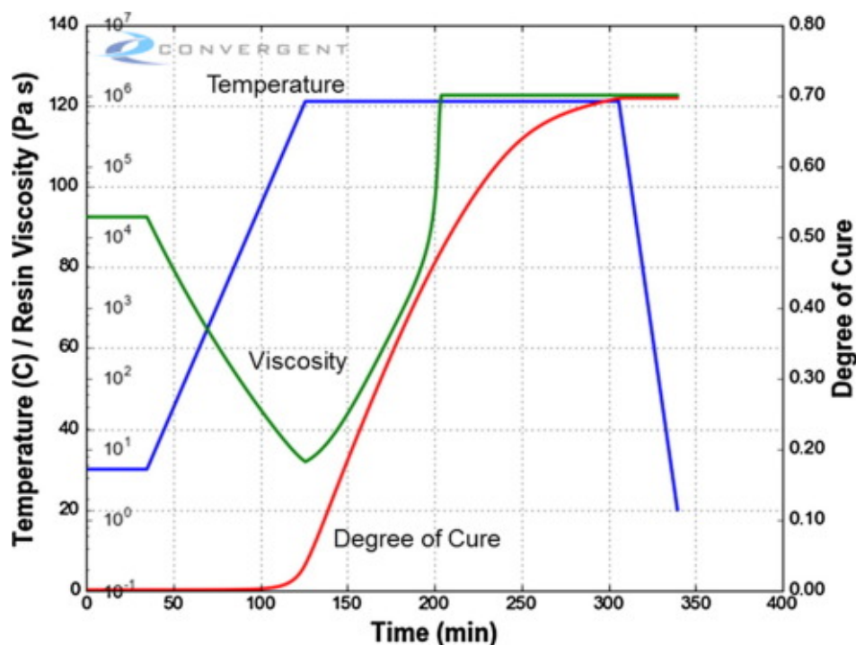
FIGURE 2.12 Courbe de la viscosité et du degré de polymérisation lors d'un cycle de cuisson [51]
