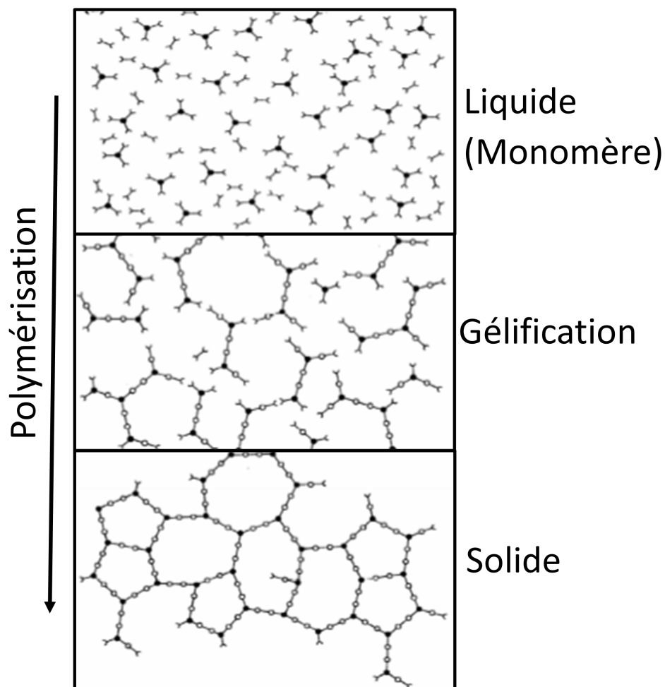
FIGURE 2.2 Polymérisation d'une matrice thermodurcissable (adapté de [17])
