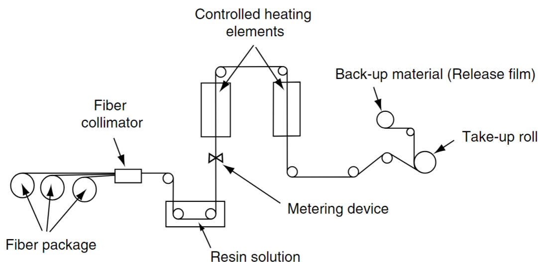
FIGURE 2.15 Schéma de la mise en forme d'un préimprégné [5]
