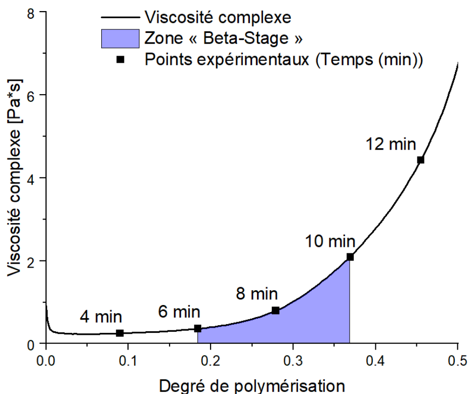
FIGURE 3.15 Zone de processabilité du préimprégné selon des essais expérimentaux à 60°C
