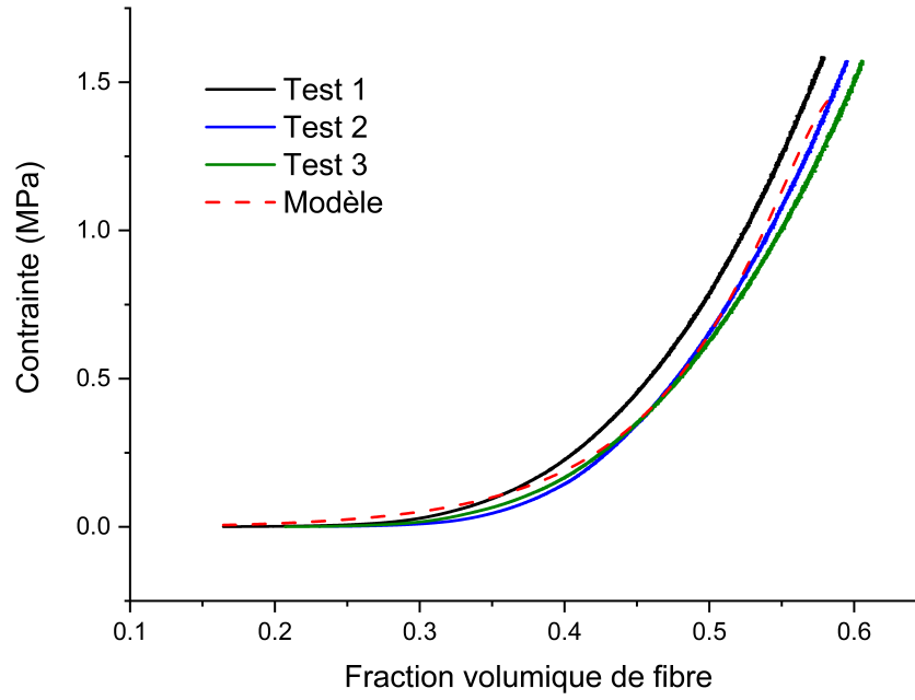
FIGURE 3.13 Modèle de Gutowski [46] pour la compaction de 6 plies de renfort de lin unidirectionnel
