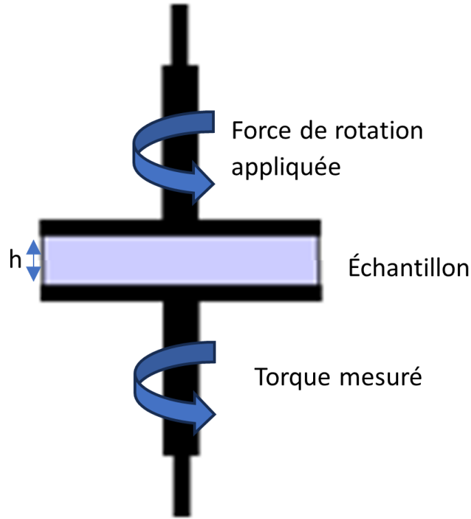
FIGURE 2.13 Configuration plaque parallèle d'un rhéomètre
