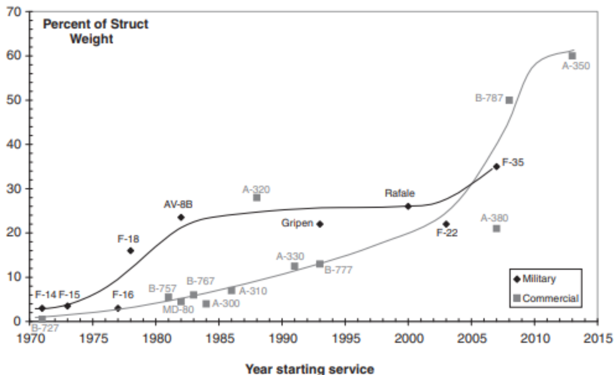
FIGURE 1.1 Application des composites dans les structures de l'aviation civile et militaire [6]
