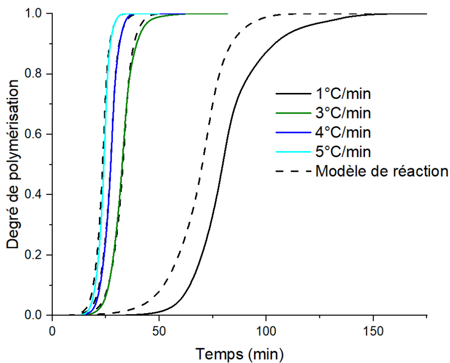
FIGURE 3.4 Degré de polymérisation du Bio-PU selon le temps à différentes rampes de température
