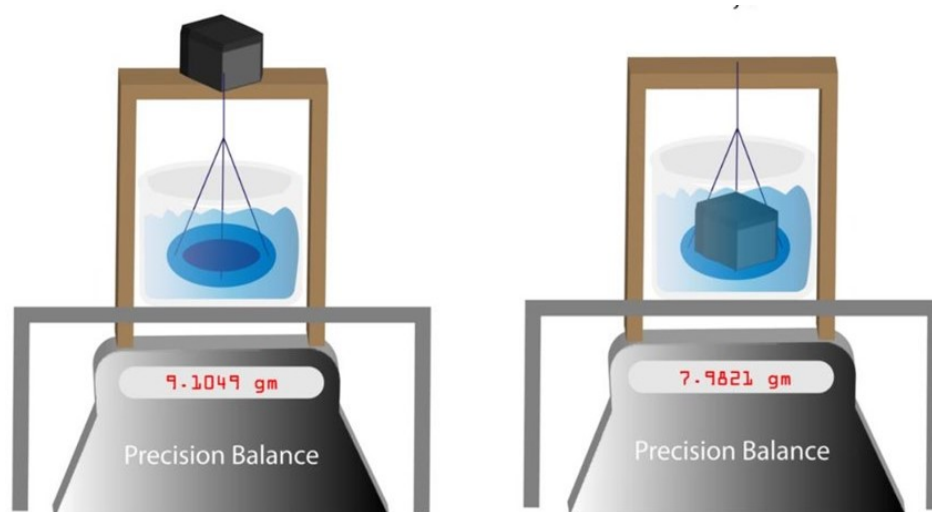
FIGURE 2.16 Montage ASTM D792 pour la mesure de la densité [55]
