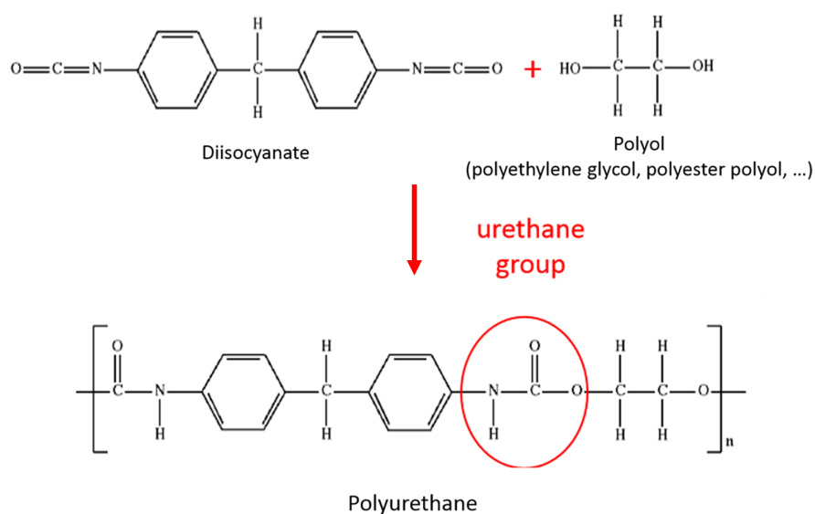
FIGURE 2.7 Synthèse du polyuréthane (adapté de [17])
