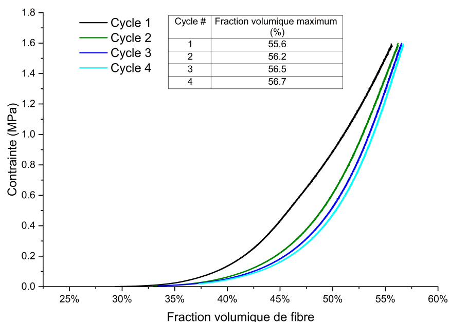
FIGURE 3.14 Effet d'imbrication des fibres lors de la compaction cyclique de 6 plis de renfort de lin
