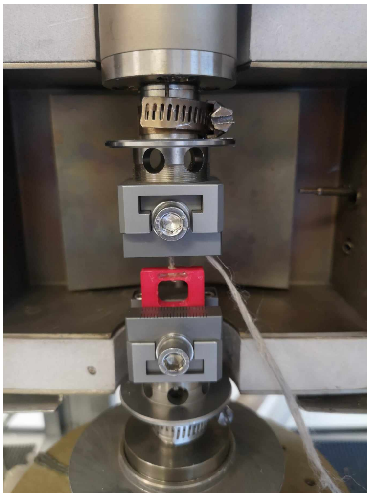
FIGURE 3.17 Montage de fiber pull-out pour tester la résistance au cisaillement de l'interface fibre/matrice
