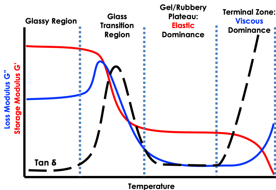
FIGURE 2.14 Courbes du module de stockage et de perte du composite sous un chargement dynamique [53]
