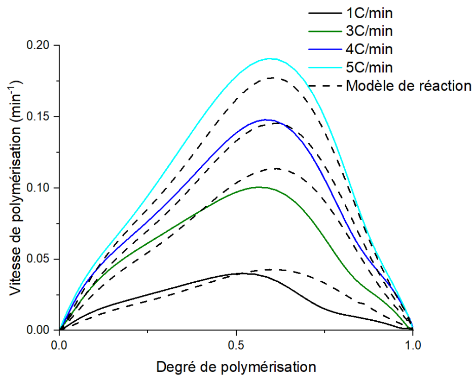
FIGURE 3.6 Vitesse de réaction du Bio-PU selon le degré de polymérisation
