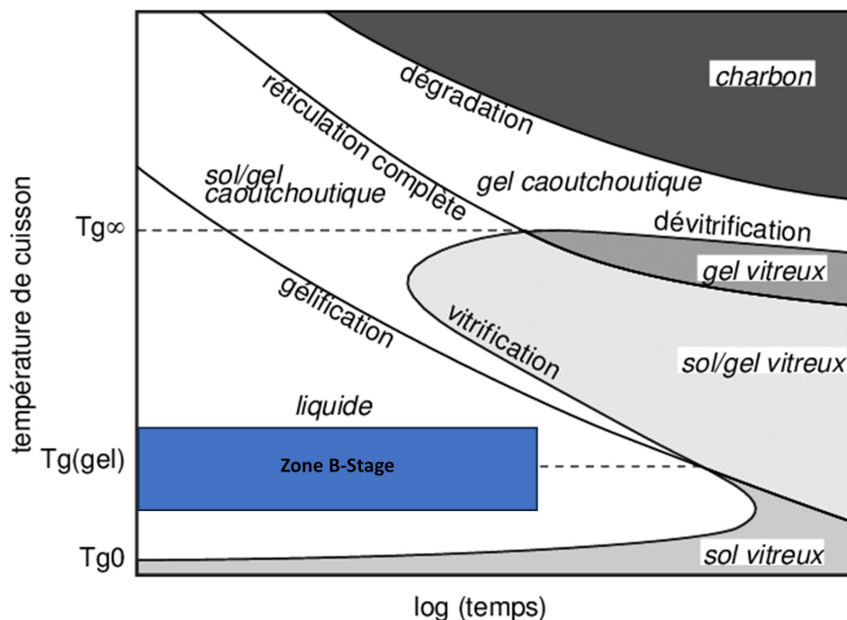
FIGURE 2.3 Diagramme TTT d'un polymère lors de la polymérisation (adapté de [18])
