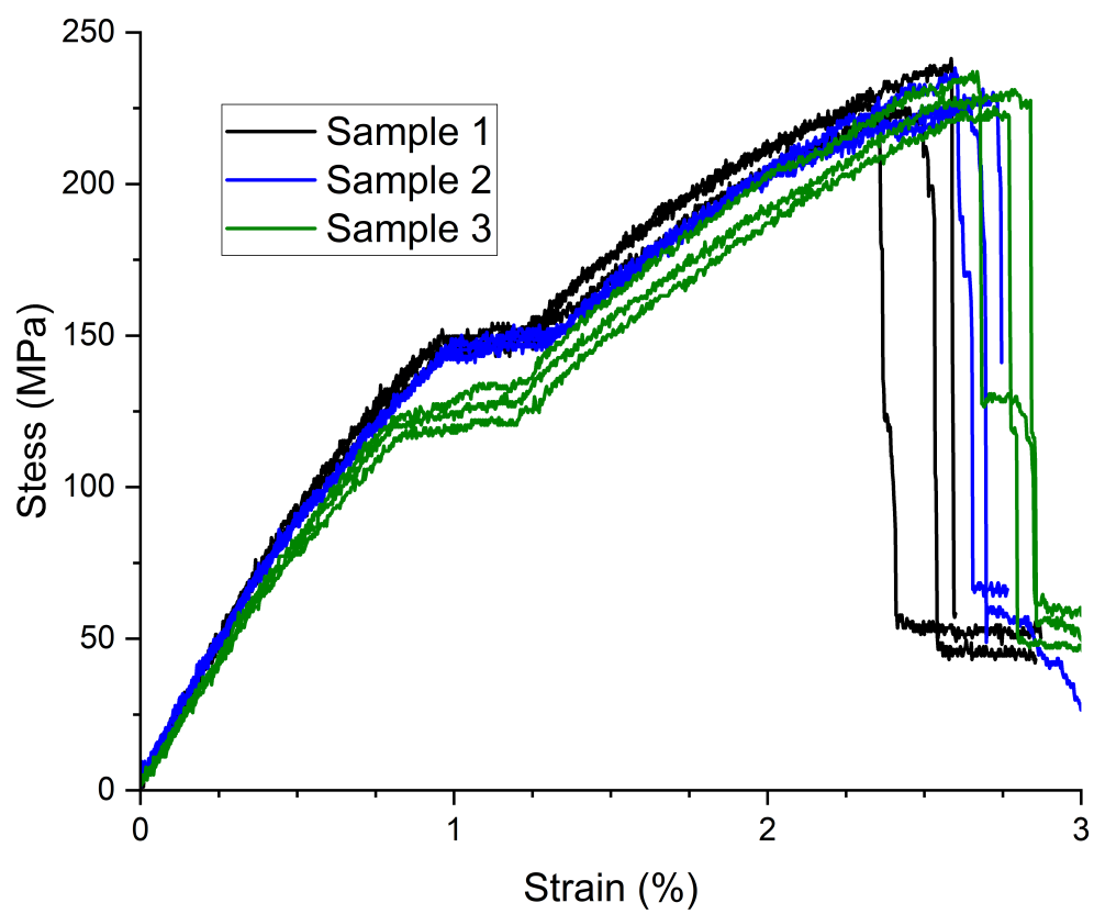
FIGURE B.2 Résultats des essais de flexion
