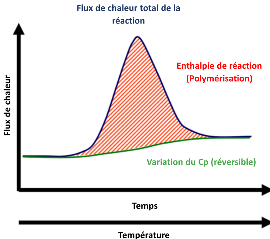
FIGURE 2.11 Courbe du flux de chaleur selon la température et le temps d'une DSC (adapté de [17])
