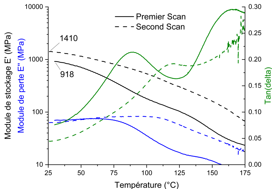
FIGURE 3.11 DMA du Bio-PU avant la post-cuisson, premier et second scan
