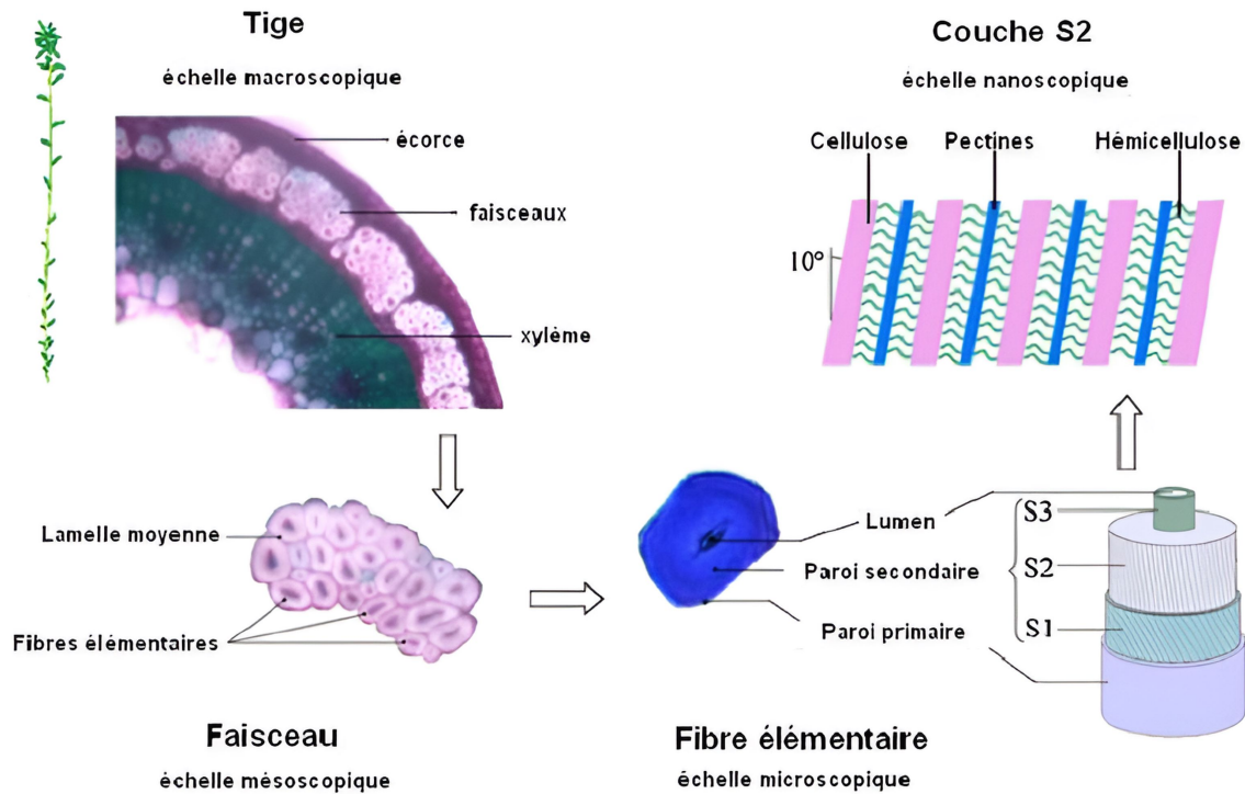
FIGURE 2.5 Structure du lin à l'échelle macroscopique et microscopique [26]
