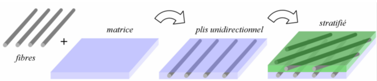
FIGURE 2.1 Constituants d'un matériau composite (adapté de [16])
