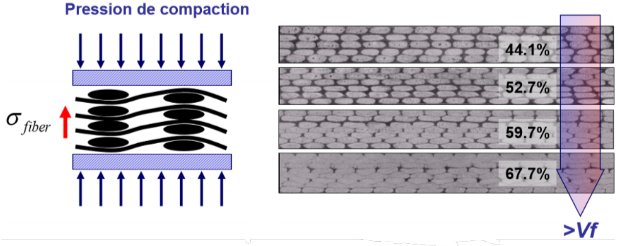
FIGURE 2.8 Effet de la compaction sur le taux volumique de fibre [17]
