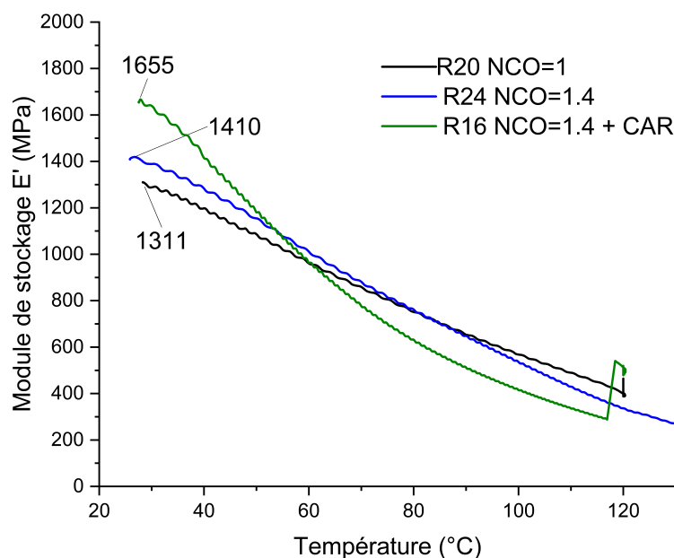
FIGURE 3.10 DMA des différentes formulations de Bio-PU de la section 3.3.1
