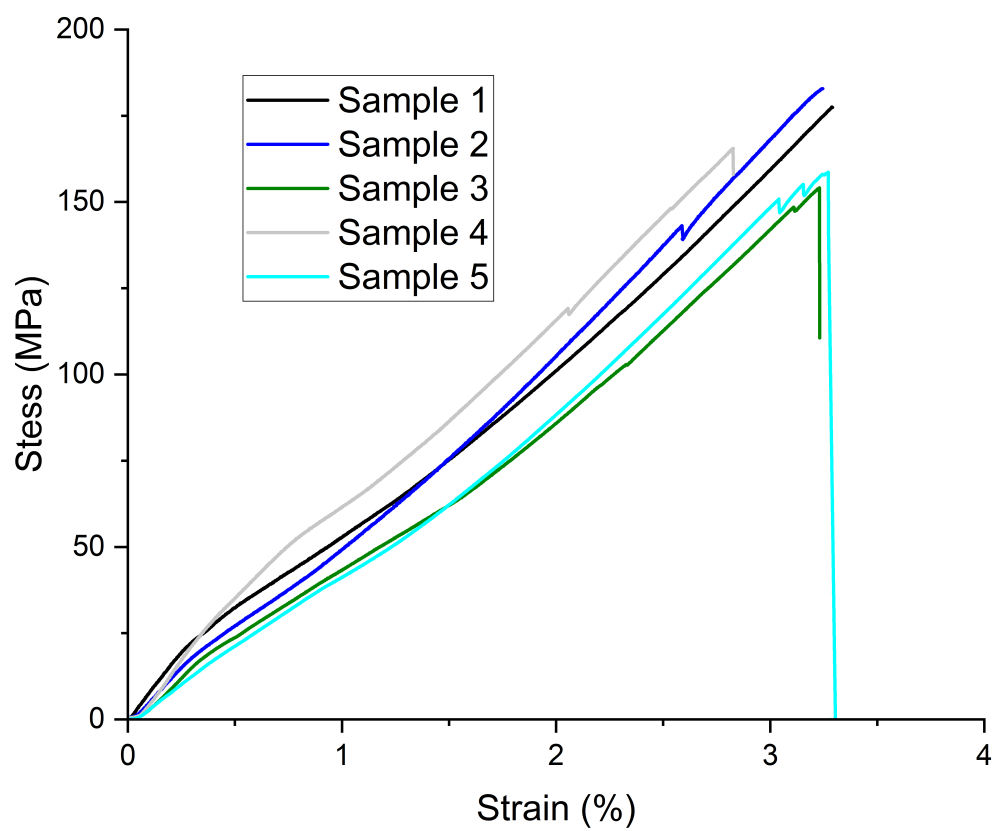
FIGURE B.1 Résultats des essais de tractions
