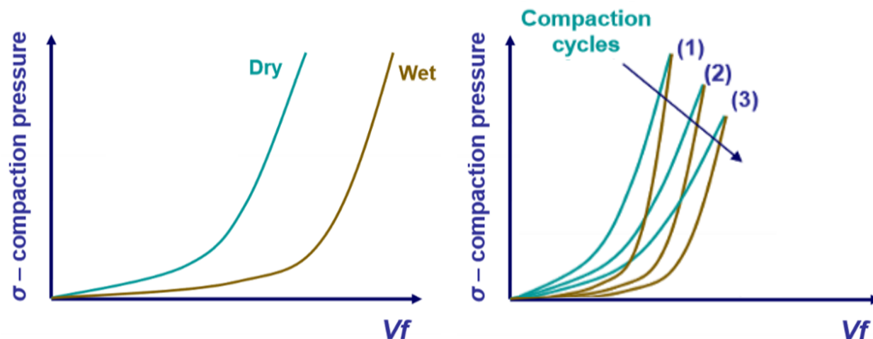
FIGURE 2.9 Exemple de courbes de compaction de renforts [17]
