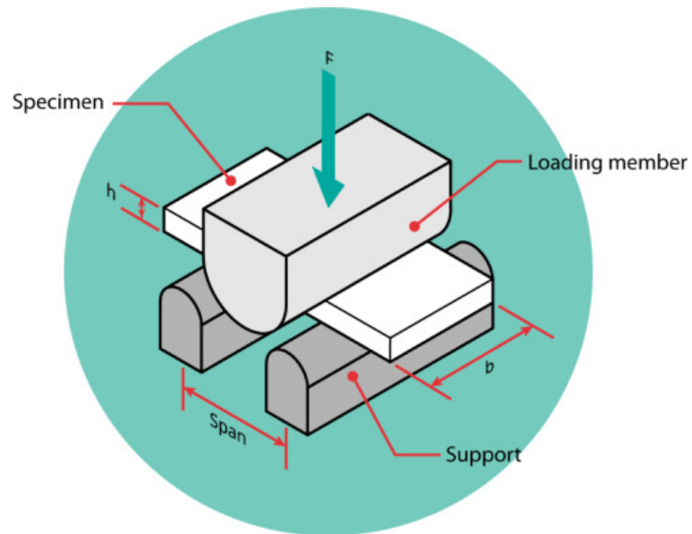
FIGURE 2.19 Montage ASTM D2344 pour les essais de « SBS » [62]
