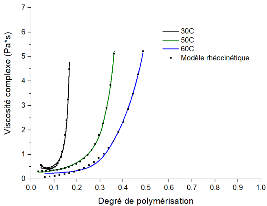
FIGURE 3.7 Viscosité du Bio-PU selon son degré de polymérisation
