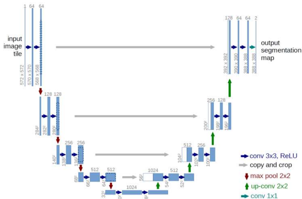
FIGURE 2.14 Architecture U-Net. Des connexions raccourcies entre l’encodeur et le décodeur du réseau de segmentation permettent de mieux reconstituer l’information spatiale perdue lors de l’encodage. Image extraite de [16].
