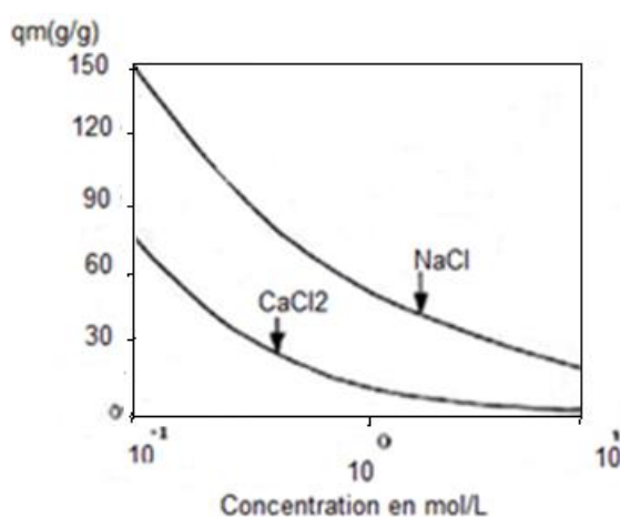
Figure 2.9: Absorbance de l'acide polyacrylique dans des solutions de NaCl et de \text{CaCl}_2 (d'après Shimomura et Hymen, 1991).
