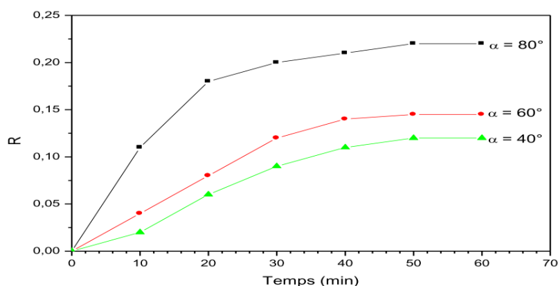
Figure 2.14: La cinétique d'extraction de Zn 2+ par le gel d'acide polyacrylique de sodium pour différents taux d'ionisation (α de 40 à 80) (d'après Taouil et al., 2014).
