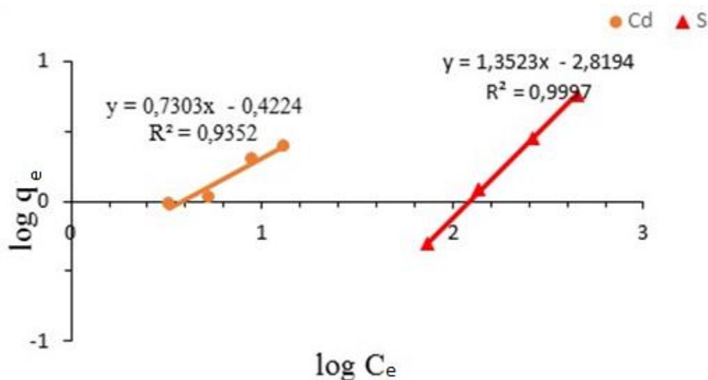
Figure 5.11: Exemple d'isotherme de Freundlich pour la séquestration de Cd et As par les PSAs.
