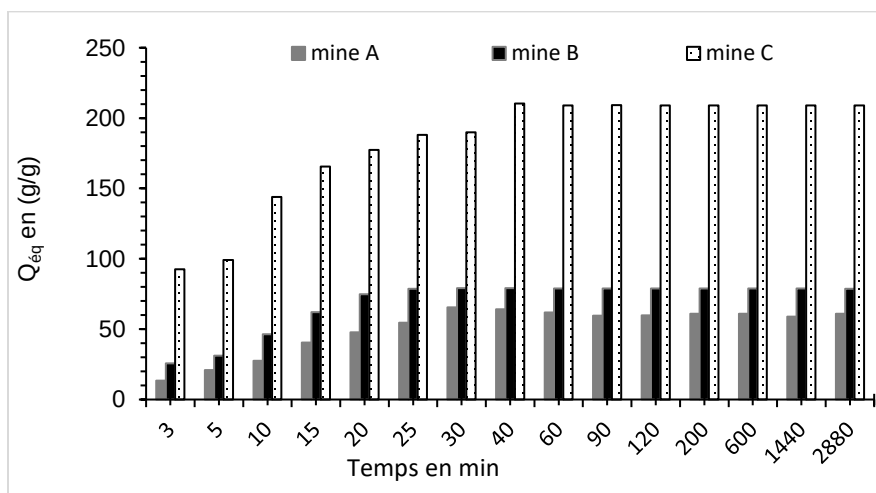
Figure 4.2: Taux d'absorption des PSAs grossiers dans les eaux minières ayant différentes compositions chimiques.
