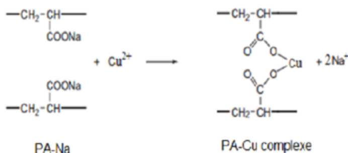
Figure 2.13: Complexation entre les ions carboxylate et les ions \text{Cu}^{2+} (d'après Ismi et al., 2014).
