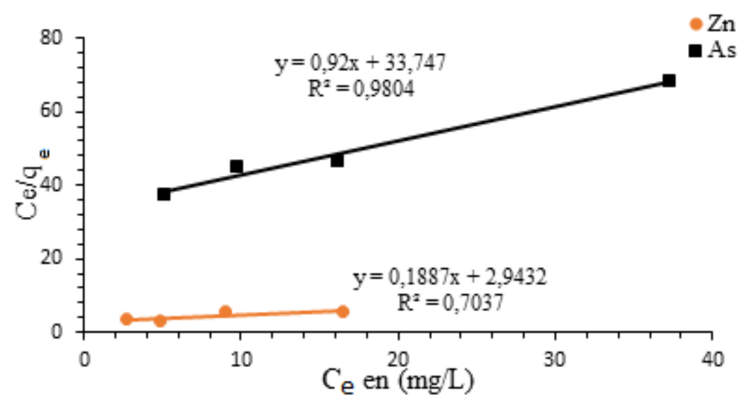
Figure 5.12: Exemple d'isotherme de Langmuir pour la séquestration de As et de Zn par le PA-Na.
