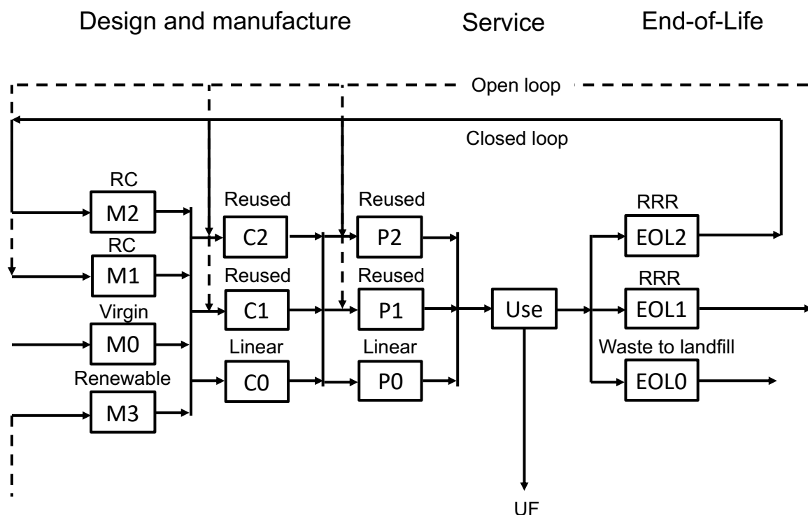
Figure D.1: Arbre de processus circulaire.
