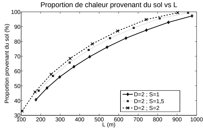
Figure 5.12 Proportion de l'énergie en chauffage du bâtiment fournie par l'échangeur géothermique pour 3 différents espacements à D=2 m.
