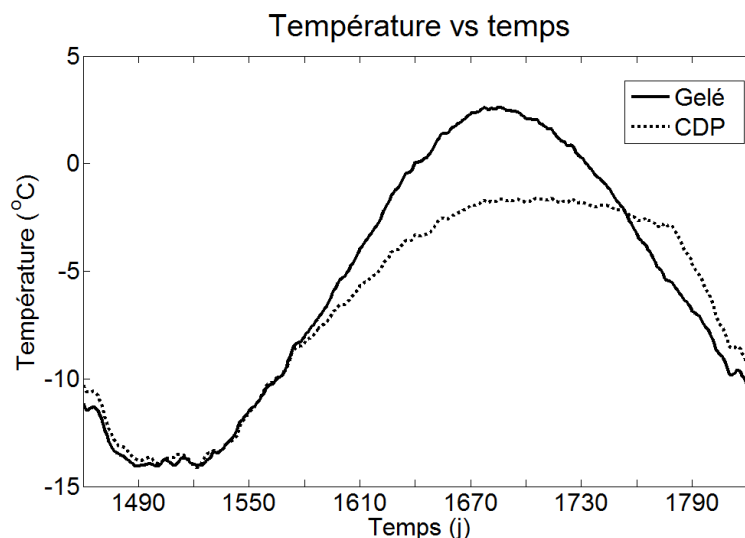
Figure 5.6 Comparaison des températures calculées au point 4 avec des modèles numériques avec CDP, sans CDP et sol gelé et sans CDP et sol dégelé pour 2 tuyaux pour la cinquième année.
