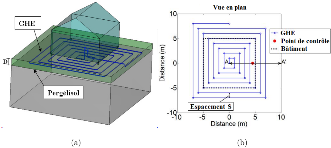
Figure 5.1 Représentation schématique de la disposition de l'échangeur géothermique.
