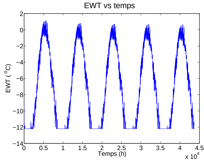
Figure 5.10 EWT pour un dimensionnement de D = 2,5\text{ m} , L = 446,25\text{ m} et S = 1,5\text{ m} calculé heure par heure sur 5 ans.
