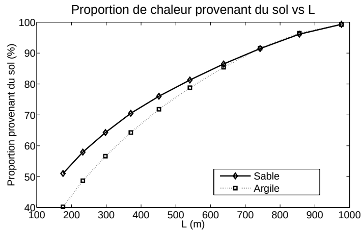
Figure 6.1 Proportion de l'énergie en chauffage du bâtiment donnée par l'échangeur géothermique pour S=1 m et D=2,5 m. Comparaison des résultats obtenus avec le sable et l'argile.
