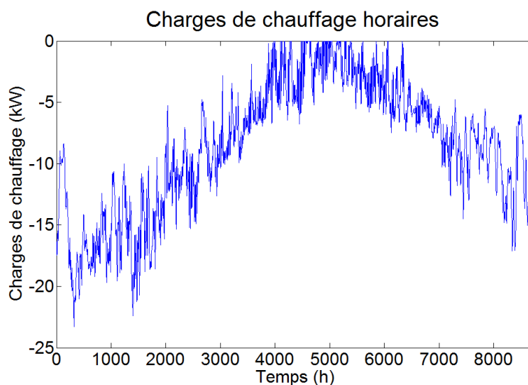
Figure 5.9 Profil des charges horaires utilisées pour les calculs
