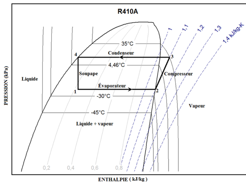
Figure 3.2 Diagramme de la variation de la pression et de l'enthalpie du réfrigérant dans une pompe à chaleur.
