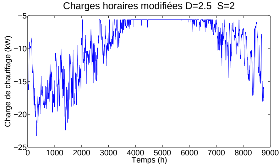
Figure 5.17 Énergie de chauffage d'un bâtiment avec charge minimum limitée à 5,6 kW durant l'été pour garder le sol gelé. D = 2,5 m, L = 903 m et S = 2 m.
