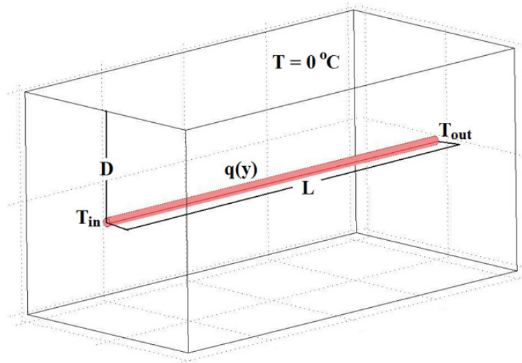
Figure 3.8 Illustration des paramètres utilisés dans les équations du régime permanent de Claesson et Dunand (1983) pour un tuyau horizontal.
