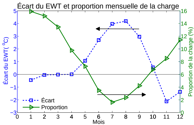
Figure 5.8 Écarts moyens mensuels entre les EWTs de la figure 5.7 et la proportion de chauffage mensuelle sur 75 MWh.
