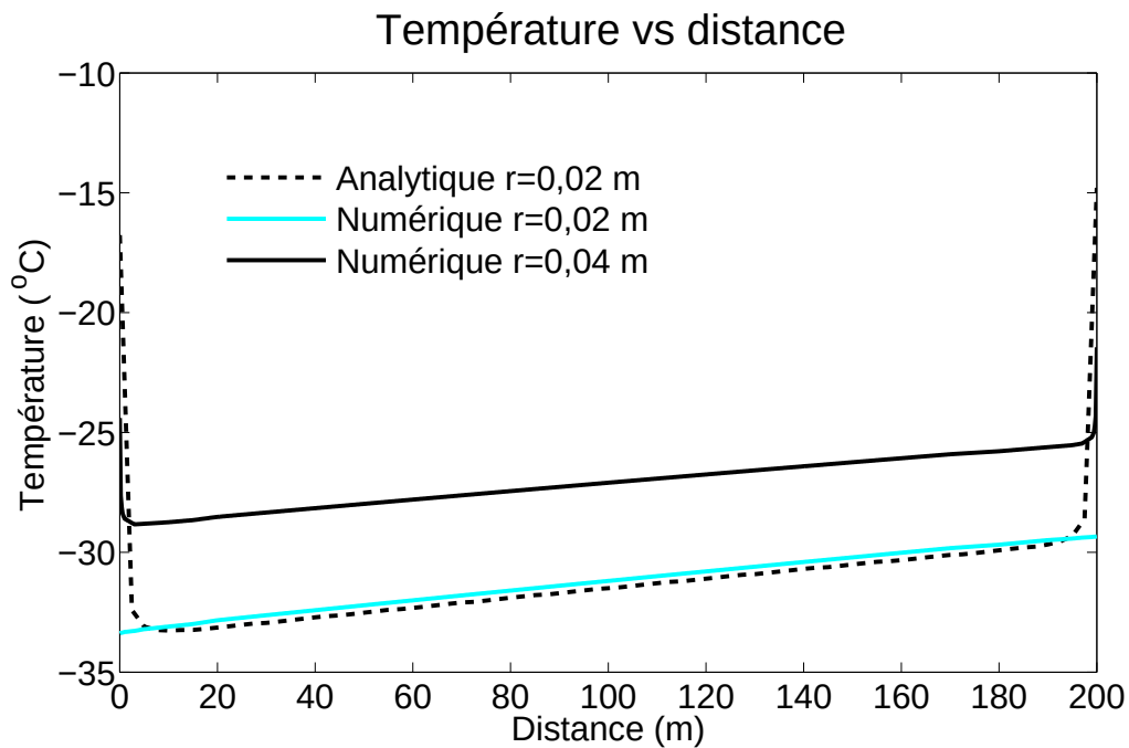
Figure II.1 Profil de température le long d'un tuyau pour trois cas ; fin de la 5 e année d'une charge constante.
