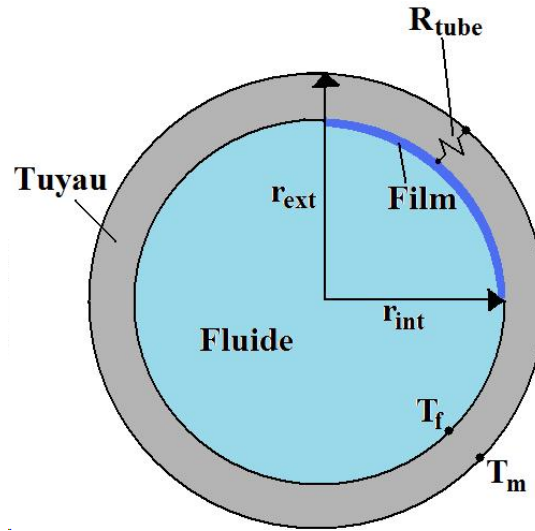
Figure 3.4 Coupe d'un tuyau perpendiculairement au débit de circulation
