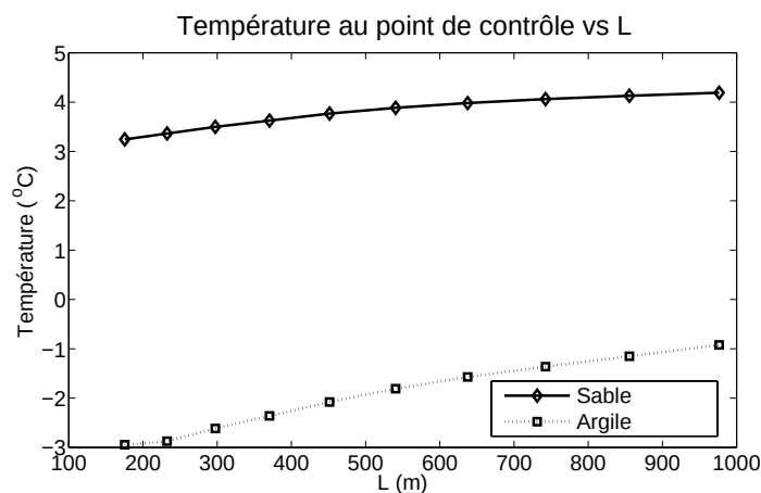
Figure 6.2 Température maximale au point de contrôle pour la 5 e année de simulation, pour S=1 m et D=2,5 m. Comparaison des résultats obtenus avec le sable et l'argile.
