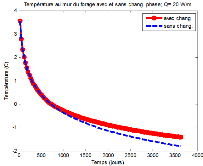
Figure 3.10 Température au mur du forage par rapport au temps en considérant le changement de phase et en ne le considérant pas pour une charge de 20 W/m ; porosité de 25%.
