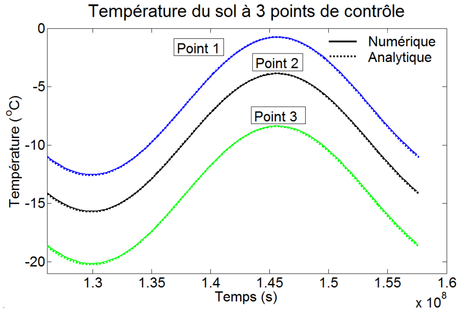
Figure 4.5 Réponses numériques et analytiques de température aux points de contrôle 1 à 3 (voir figure 4.3) ; charge constante dans le sol (-15 kW) et température variable en surface avec A=12,5 °C et T_s = -2 °C.
