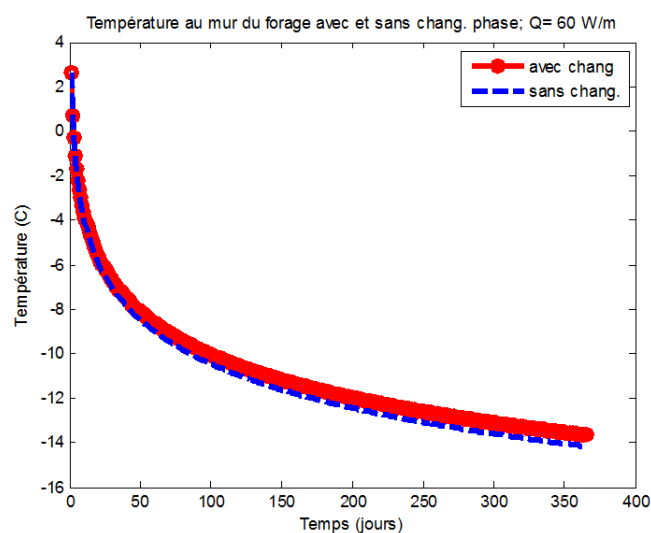
Figure 3.12 Température au mur du forage par rapport au temps en considérant le changement de phase et en ne le considérant pas pour une charge de 60 W/m ; porosité de 3%.
