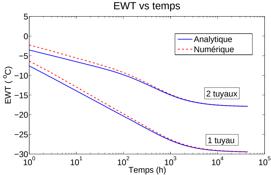
Figure 4.9 Réponses numériques et analytiques de température à la sortie du tuyau (EWT) ; charge constante dans le sol (-15 kW) avec température constante en surface.
