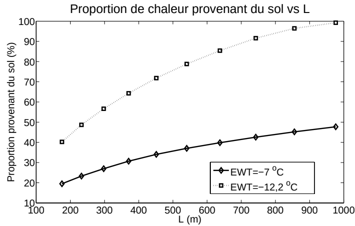
Figure 6.5 Proportion de l'énergie en chauffage du bâtiment donnée par l'échangeur géothermique pour S = 1\text{ m} et D = 2,5\text{ m} . EWT limite de -7\text{ }^{\circ}\text{C} et de -12,2\text{ }^{\circ}\text{C} .
