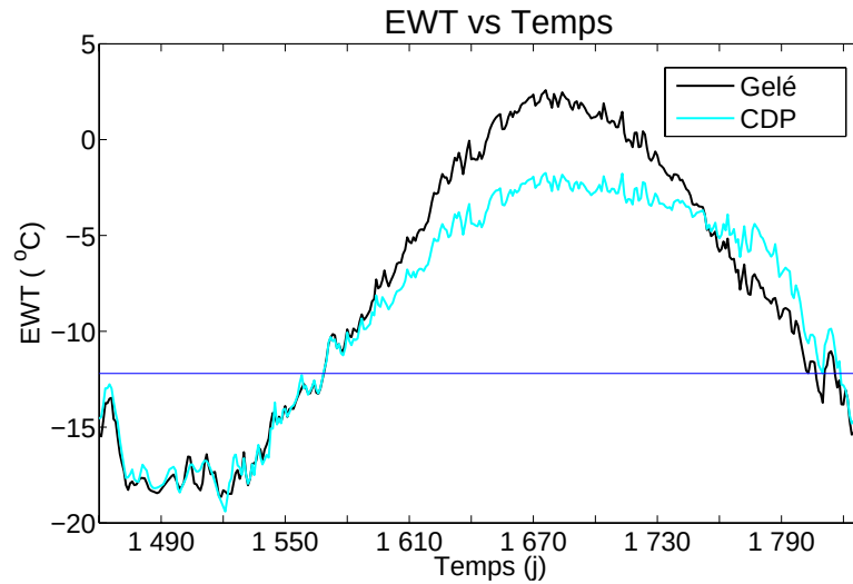
Figure 5.7 EWT des modèles numériques avec CDP et sans CDP avec sol gelé pour la 5 e année. Modèle avec 2 tuyaux.
