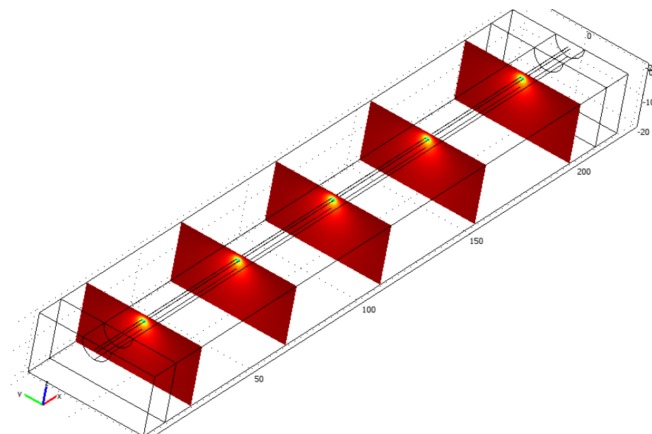
Figure 4.6 Modèle numérique 3D avec 2 tuyaux.
