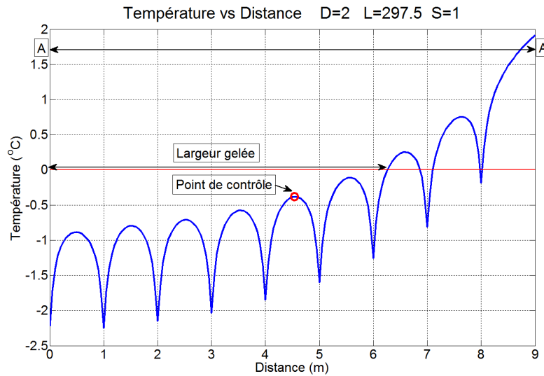
Figure 5.11 Profil de température le long de la section A-A' pour le temps le plus chaud à D=2 m. L'échangeur géothermique est de dimension L = 297,5 m et S=1 m. La limite extérieure du bâtiment est à une distance de 5 m.
