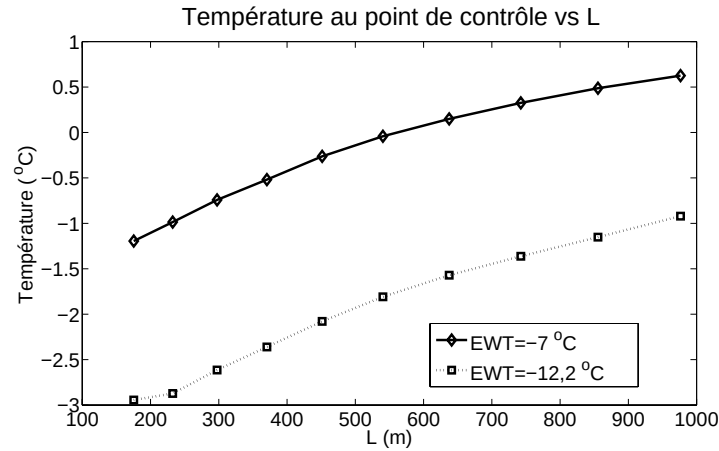
Figure 6.6 Température maximale au point de contrôle pour la 5 e année de simulation, pour S = 1 m et D = 2,5 m. EWT limite de -7 °C et de -12,2 °C.
