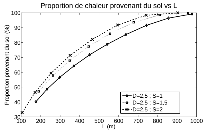
Figure 5.13 Proportion de l'énergie en chauffage du bâtiment donnée par l'échangeur géothermique pour 3 différents espacements à D=2,5 m.
