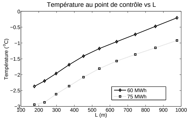
Figure 6.4 Température maximale au point de contrôle pour la 5 e année de simulation, pour S=1 m et D=2,5 m. Charges de chauffage de 60 MWh et de 75 MWh.
