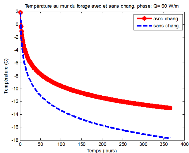
Figure 3.11 Température au mur du forage par rapport au temps en considérant le changement de phase et en ne le considérant pas pour une charge de 60 W/m ; porosité de 25%.
