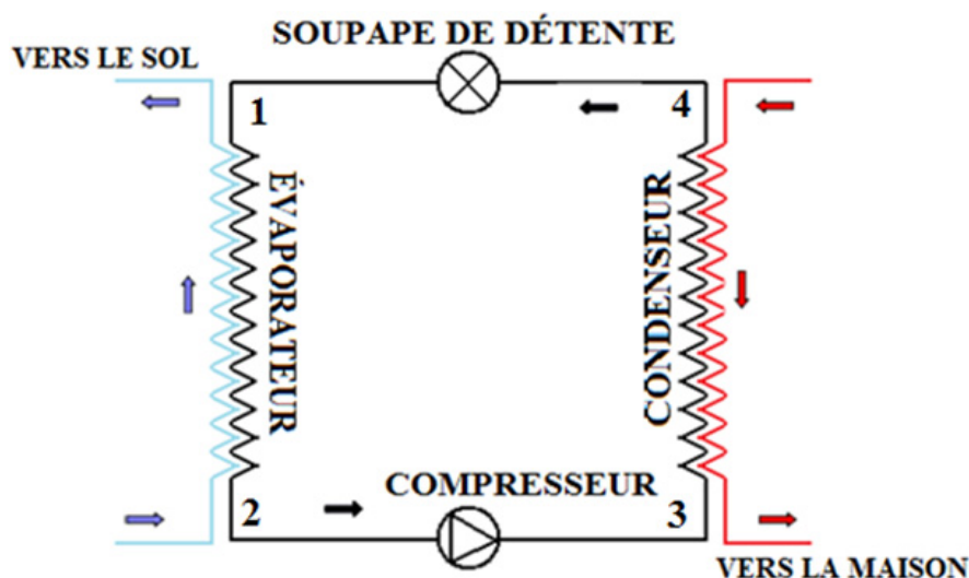
Figure 3.1 Représentation schématique des principales parties d'une pompe à chaleur.
