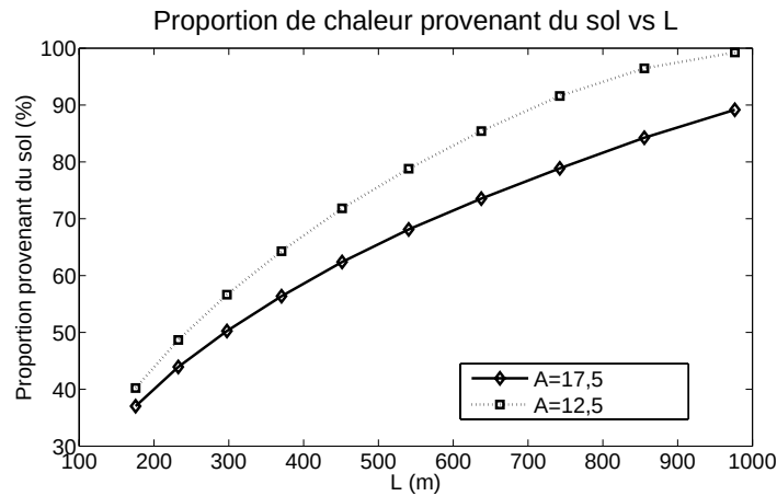
Figure 6.9 Proportion de l'énergie en chauffage du bâtiment donnée par l'échangeur géothermique pour S = 1\text{ m} et D = 2,5\text{ m} . Comparaison des résultats obtenus avec A = 17,5\text{ }^{\circ}\text{C} et A = 12,5\text{ }^{\circ}\text{C} .
