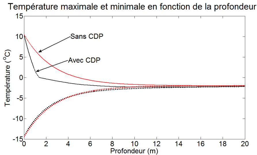
Figure 5.2 Températures maximales (lignes continues) et minimales (lignes pointillées) à chaque profondeur durant la 5 e année. Calculées avec CDP et sans CDP (paramètres sol gelé) ; modèle numérique 1D.
