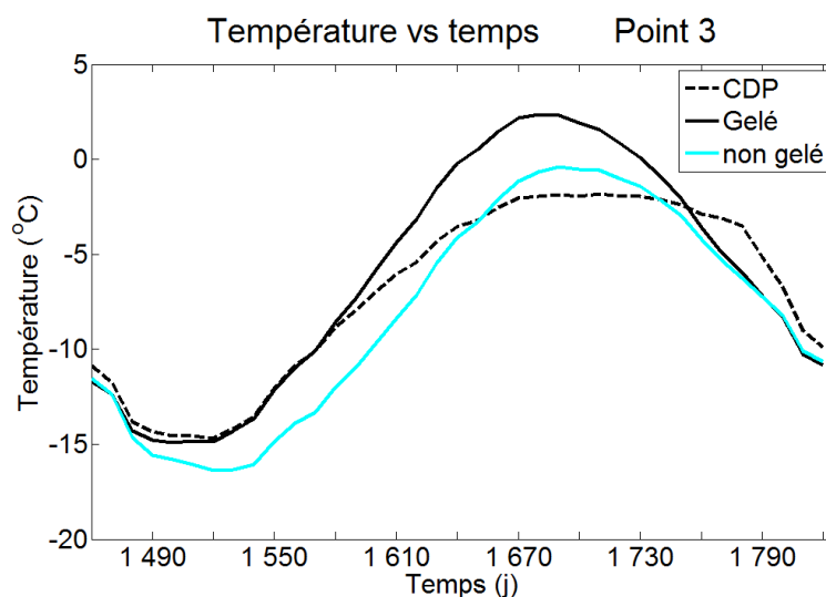
Figure 5.5 Comparaison des températures calculées au point 3 avec des modèles numériques avec CDP, sans CDP et sol gelé et sans CDP et sol dégelé pour 1 tuyau pour la cinquième année.
