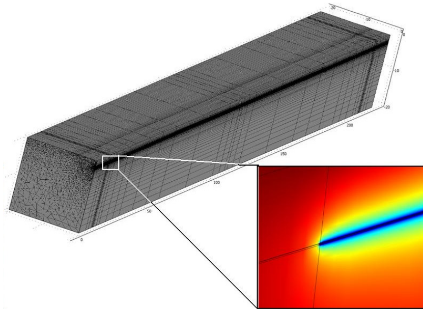
Figure 4.2 Modèle numérique 3D avec 1 tuyau et agrandissement sur le tuyau une fois les calculs effectués
