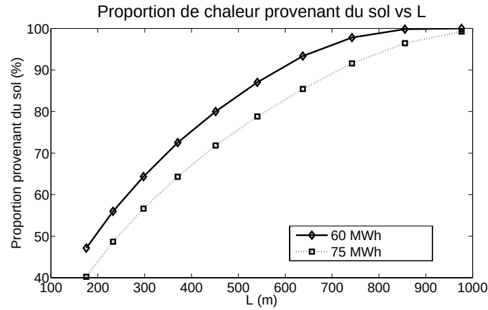
Figure 6.3 Proportion de l'énergie en chauffage du bâtiment donnée par l'échangeur géothermique pour S=1 m et D=2,5 m. Charges de chauffage de 60 MWh et de 75 MWh.
