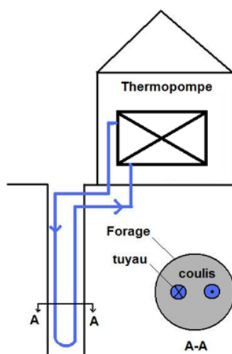
Figure 3.3 Illustration d'un échangeur géothermique vertical couplé à une pompe à chaleur.
