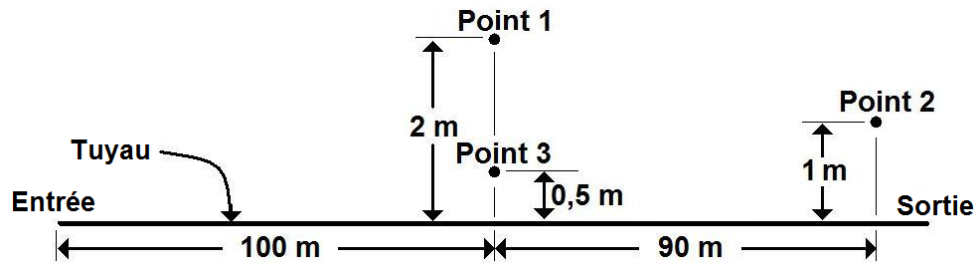
Figure 4.3 Localisation des points de contrôle pour la validation du modèle analytique pour 1 tuyau.
