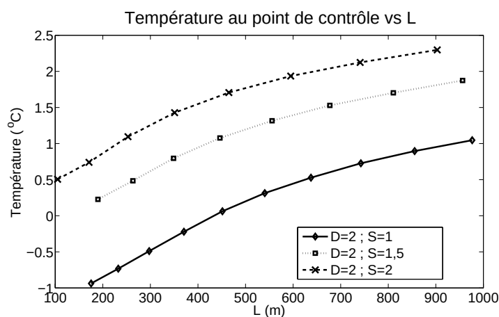
Figure 5.14 Température maximale aux points de contrôle pour la 5 e année de simulation, pour 3 différents espacements à D=2 m
