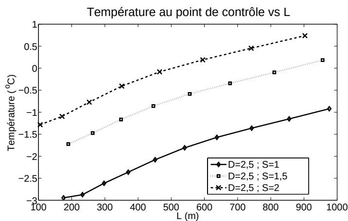
Figure 5.15 Température maximale aux points de contrôle pour la 5 e année de simulation, pour 3 différents espacements à D=2,5 m
