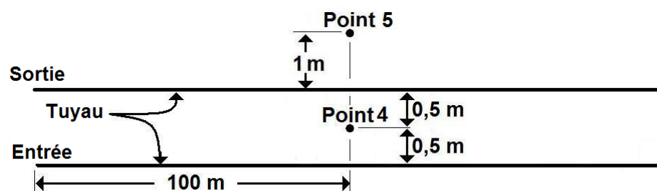
Figure 4.7 Localisation des points de contrôle utilisé pour la comparaison des modèles à deux tuyaux.
