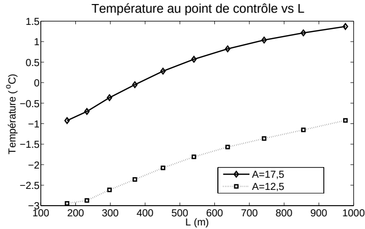
Figure 6.10 Température maximale au point de contrôle pour la 5 e année de simulation, pour S=1 m et D=2,5 m. Comparaison des résultats obtenus avec A = 17,5 °C et A = 12,5 °C.
