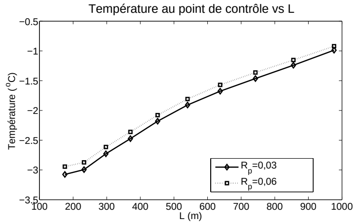
Figure 6.12 Température maximale au point de contrôle pour la 5 e année de simulation, pour S = 1 m et D = 2,5 m. Comparaison des résultats obtenus avec R_p = 0,03 et R_p = 0,06 .
