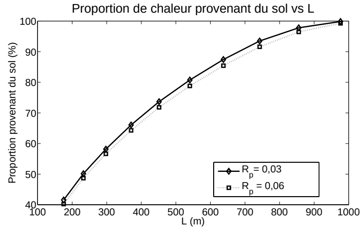
Figure 6.11 Proportion de l'énergie en chauffage du bâtiment donnée par l'échangeur géothermique pour S = 1 m et D = 2,5 m. Comparaison des résultats obtenus avec R_p = 0,03 et R_p = 0,06 .
