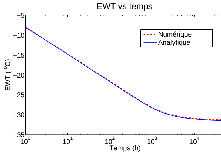
Figure III.1 Réponses numériques et analytiques de température à la sortie du tuyau (EWT) ; charge constante dans le sol (-15 kW) avec température constante en surface. Modèle à 1 tuyau avec un débit égale à 947,5 \text{ l/s} .
