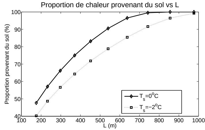
Figure 6.7 Proportion de l'énergie en chauffage du bâtiment donnée par l'échangeur géothermique pour S = 1 m et D = 2,5 m. T_s = 0^\circ\text{C} et T_s = -2^\circ\text{C} .
