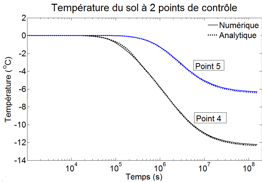
Figure 4.8 Réponses numériques et analytiques de température aux points de contrôle 4 et 5 (voir figure 4.7) ; charge constante dans le sol (-15 kW) et température de 0 °C constante en surface.
