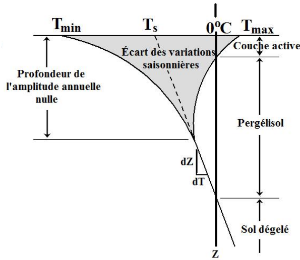
Figure 3.13 Représentation des variations saisonnières de température dans le sol. Figure modifiée de Andersland et Ladanyi (2004).
