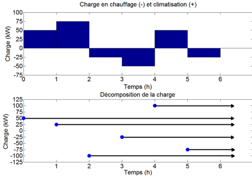
Figure 3.6 Illustration du principe de superposition temporelle avec charge variant sur 6 heures. Figure modifiée de Marcotte et al. (2010).
