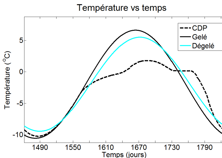
Figure 5.3 Comparaison des températures calculées avec des modèles numériques avec CDP, sans CDP et sol gelé et sans CDP et sol dégelé avec un modèle 1D sans tuyau pour la cinquième année. Température à une profondeur de 1 m.
