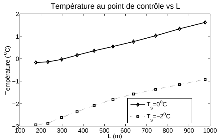
Figure 6.8 Température maximale au point de contrôle pour la 5 e année de simulation, pour S = 1 m et D = 2,5 m. T_s = 0^\circ\text{C} et T_s = -2^\circ\text{C} .
