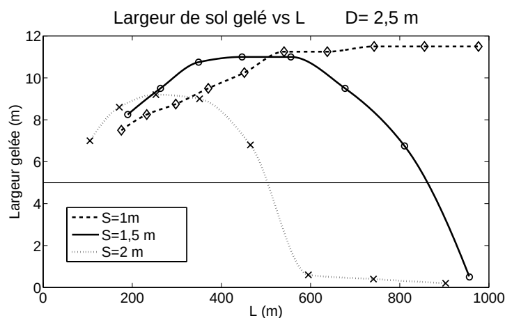
Figure 5.16 Largeur de sol gelé pour différents espacements à D = 2,5 m. Résultats pour la 5 e année.
