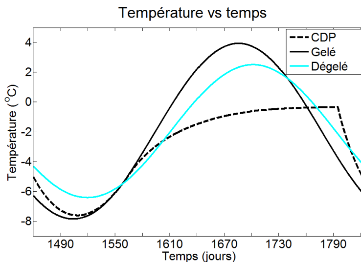
Figure 5.4 Comparaison des températures calculées avec des modèles numériques avec CDP, sans CDP et sol gelé et sans CDP et sol dégelé avec un modèle 1D sans tuyau pour la cinquième année. Température à une profondeur de 2 m.
