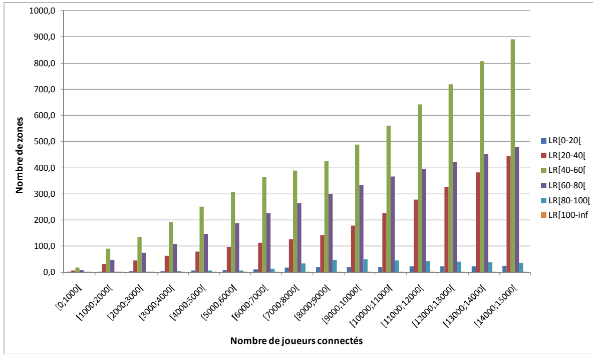
(a) Nombre moyen de zones par classe de ratio de charge en fonction du nombre de joueurs
