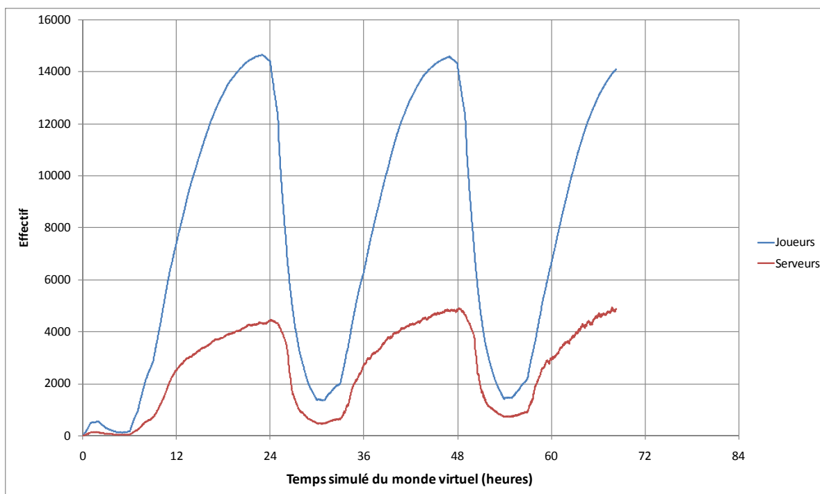
(a) Nombre de joueurs et de serveurs (zones) en fonction du temps
