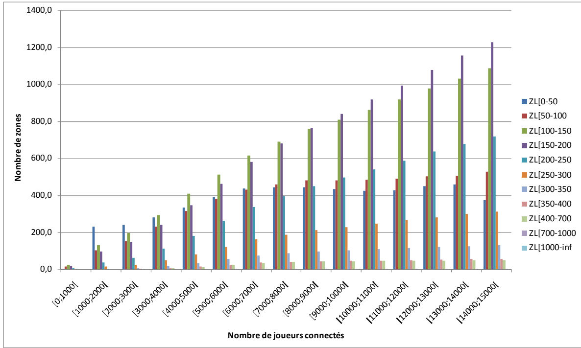
(a) Nombre moyen de zones par classe de latence en fonction du nombre de joueurs
