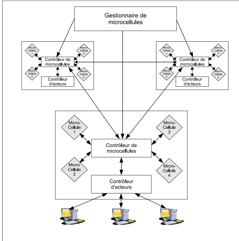
FIGURE 2.3 Architecture logicielle de redéploiement dynamique de microcellules
