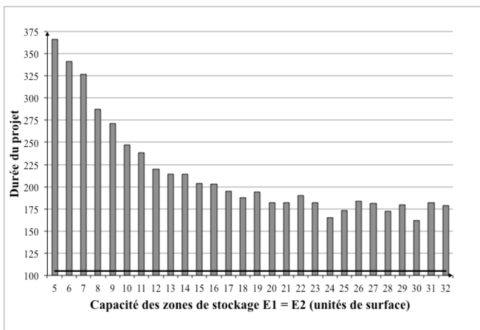
Figure 3.11 : Variation de la durée totale de projet en fonction de la capacité de stockage (120 activités)
