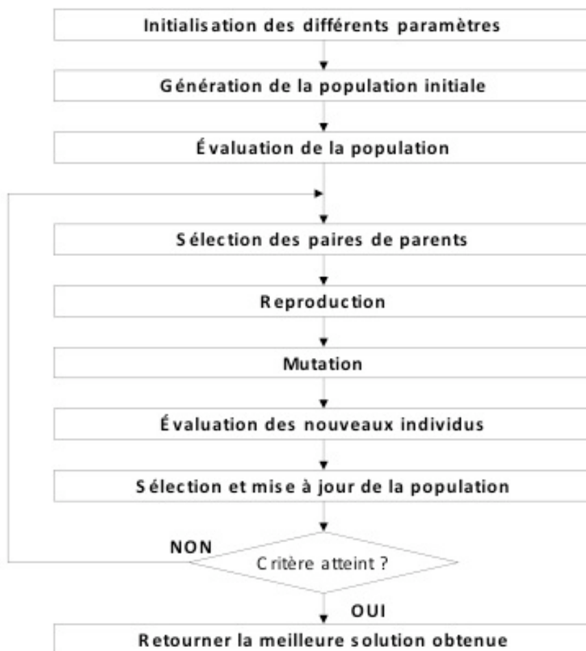
Figure 2.2 : Schéma de principe de l'algorithme génétique
