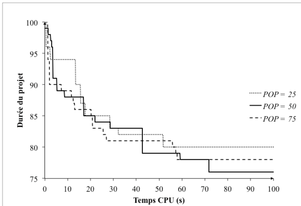
Figure 3.3 : Convergence de la durée de projet en fonction de POP ( C_p = 0,50 et M_p = 0,10 )
