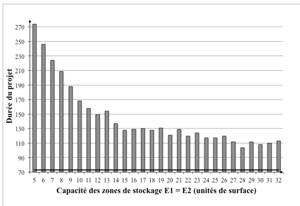
Figure 3.10 : Variation de la durée totale de projet en fonction de la capacité de stockage (90 activités)
